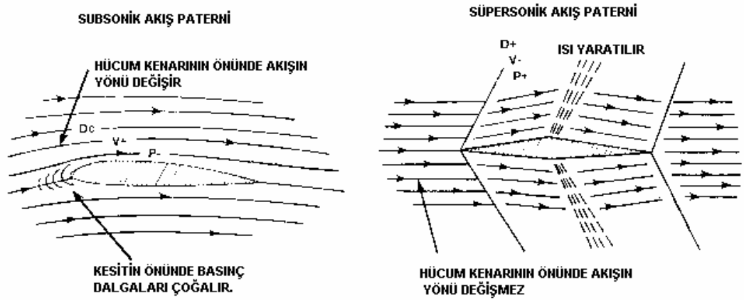
Şekil 2.10. Subsonik ve Süpersonik Akış Paternlerinin Karşılaştırılması.
