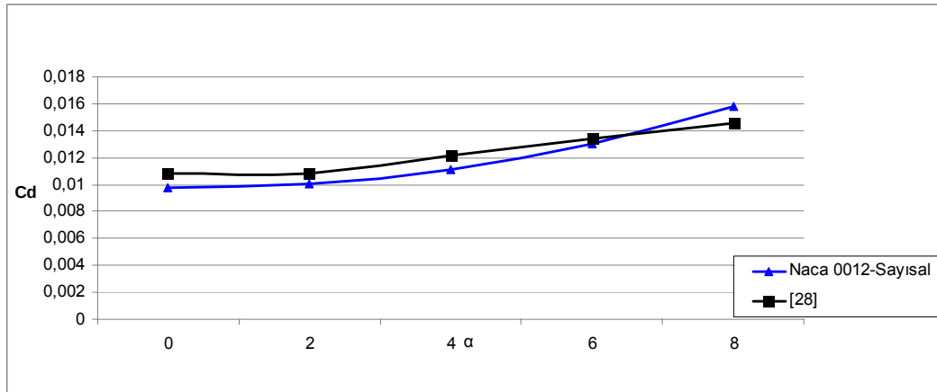
Şekil 5. 2. Naca 0012 kanat profili için Abbott ve Doenhoff ile tez çalışmasındaki C_D değerinin karşılaştırılması
