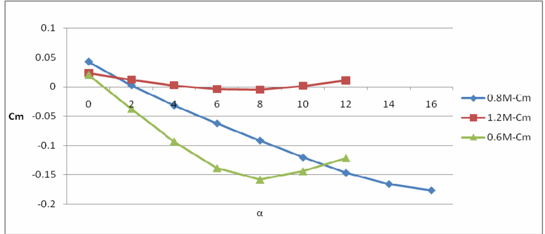
Şekil 5.10. RAE Kanat Profiline Moment Katsayısı Değişimi.
