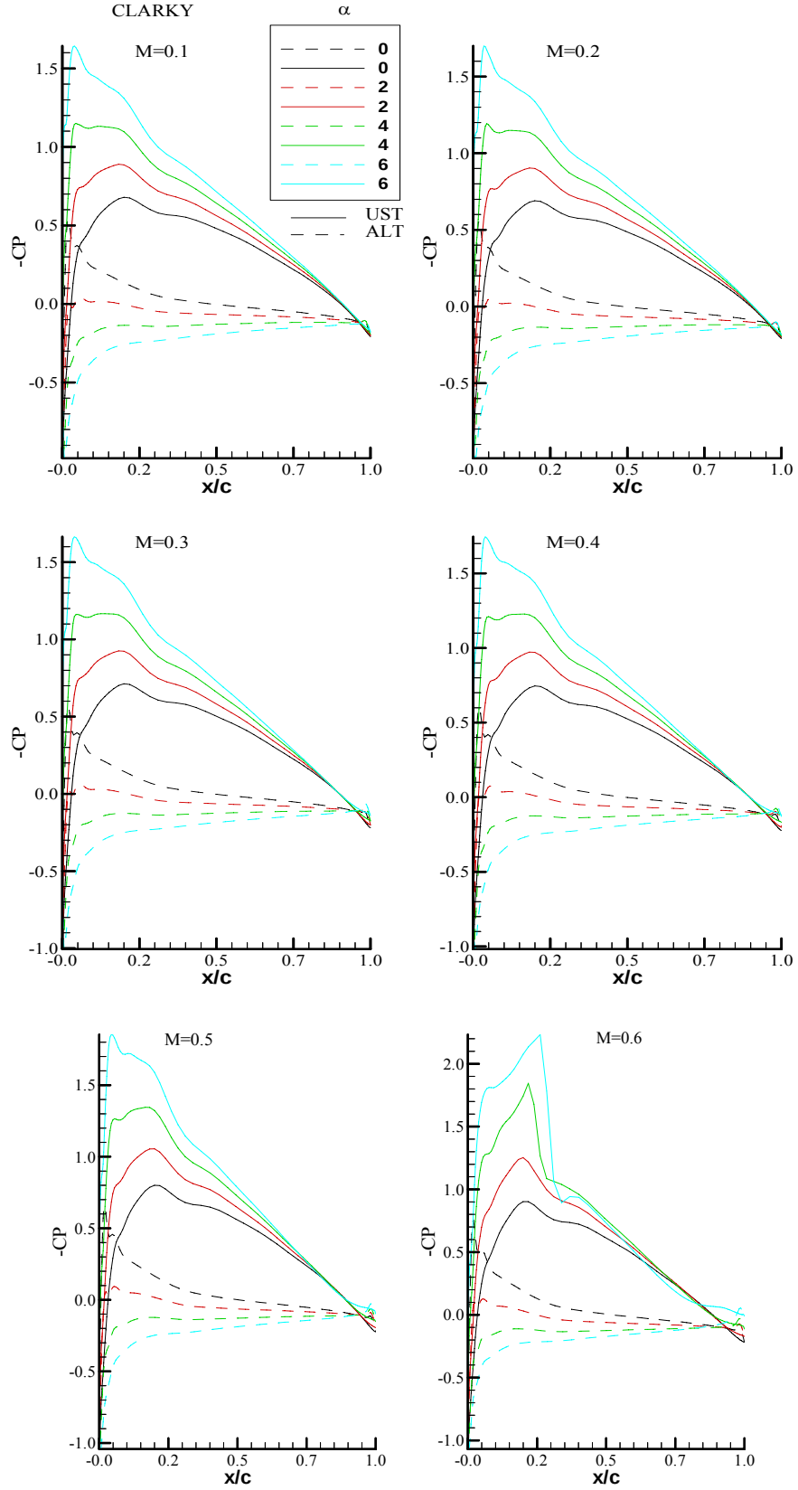
Şekil 5.25. Clark-Y Kanat Profili İçin 0.1 Mach' Dan 0.6 Mach'a Kadar C_p ' nin Hücum Açısıyla Değişimi.
