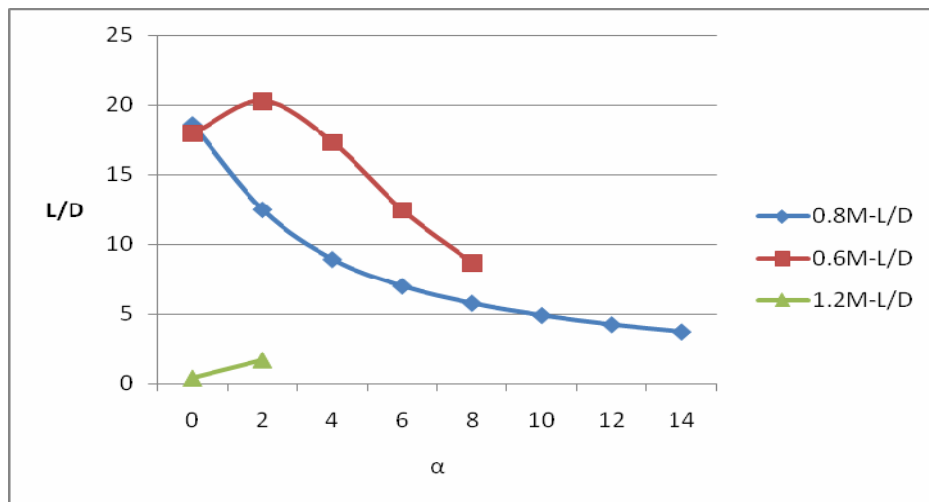
Şekil 5.13. Whitcomb Kanat Profilinin Kaldırma ve Sürüklenme Oranı Değişimi.
