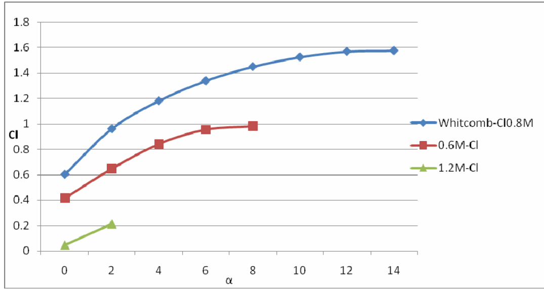
Şekil 5.7. Whitcomb Kanat Profilinin Kaldırma Katsayısı Değişimi.
