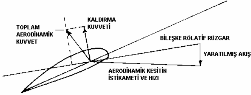
Şekil 2.5. Aerodinamik Kesite Etki Eden Kaldırma Kuvveti.
