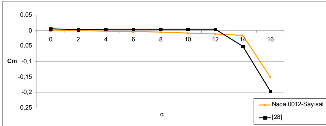
Şekil 5.3. Naca 0012 kanat profili için Abbott ve Doenhoff ile tez çalışmasındaki C_D değerinin karşılaştırılması.
