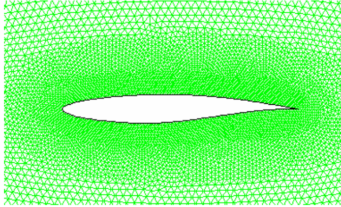
Şekil 4.7. RAE (Transonik) Kanat Profili.
