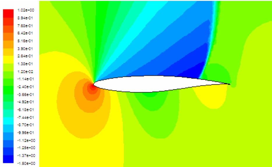
Şekil 5.28.b. RAE Profili 0.8 Mach Sayısında 6^\circ Hücum Açısında Basınç Katsayısı Dağılımı.
