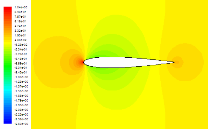
Şekil 5.26.a. Naca 0012 Profili 0.4 Mach Sayısında 0^\circ Hücüm Açısında Basınç Katsayısı Dağılımı.
