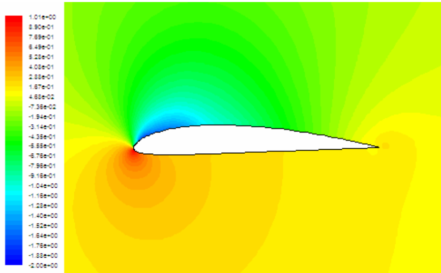
Şekil 5.27.b. Clark-Y Profili 0.4 Mach Sayısında 6^\circ Hücum Açısında Basınç Katsayısı Dağılımı.
