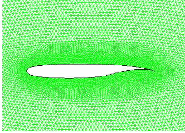
Şekil 4.6. Whitcomb (Süperkritik) Kanat Profili.
