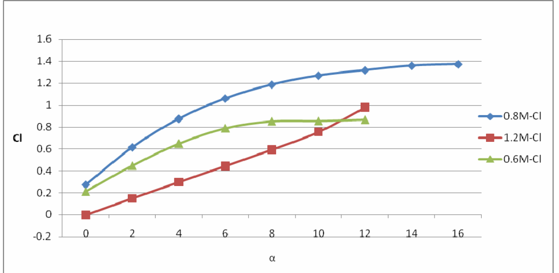
Şekil 5.6. RAE Kanat Profilinin Kaldırma Katsayısı Değişimi.
