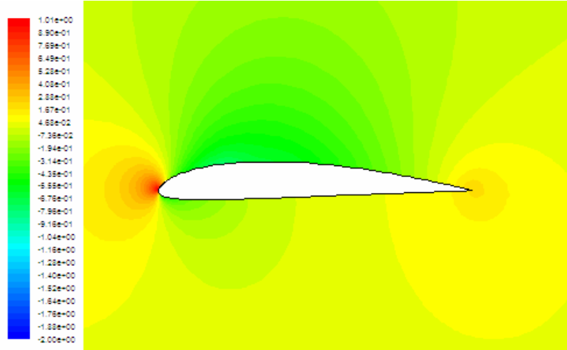
Şekil 5.27.a. Clark-Y Profili 0.4 Mach Sayısında 0^\circ Hücum Açısında Basınç Katsayısı Dağılımı.
