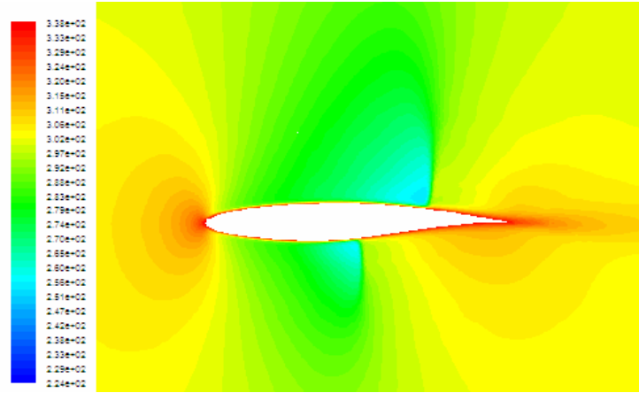
Şekil 5.18.a. RAE Profili 0.8 Mach Sayısında 0^\circ Hücum Açısında Sıcaklık Dağılımı.
