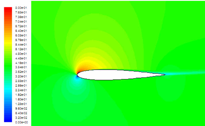
Şekil 5.20.b. Naca 0012 Profili 0.4 Mach Sayısında 6^\circ Hücum Açısında Mach Sayısı Değişimi.
