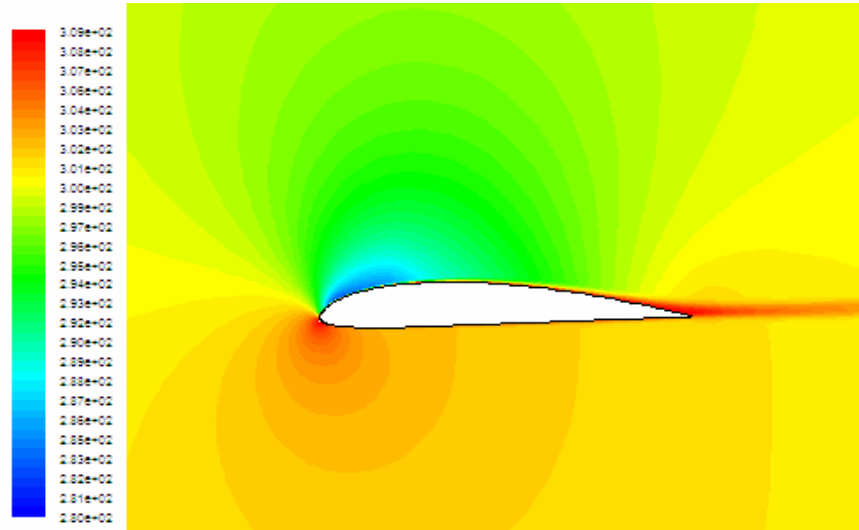
Şekil 5.17b. Clark-Y Profili 0.4 Mach Sayısında 6° Hücum Açısında Sıcaklık Dağılımı.
