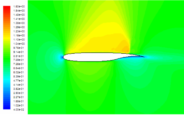
Şekil 5.23.a. Whitcomb Profili 0.8 Mach Sayısında 0^\circ Hücum Açısında Mach Sayısı Değişimi.
