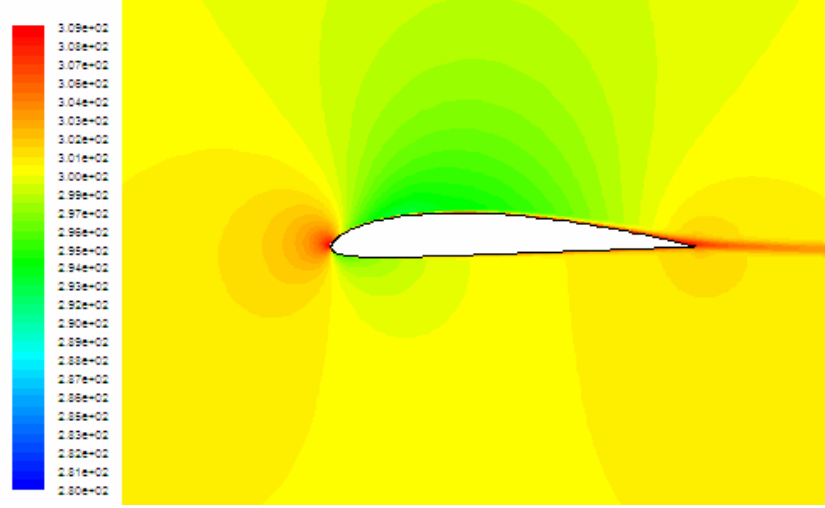
Şekil 5.17a. Clark-Y Profili 0.4 Mach Sayısında 0° Hücum Açısında Sıcaklık Dağılımı.
