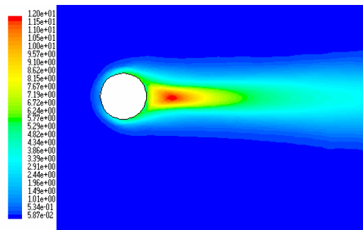
Şekil 4.1. Dairenin Türbülans Yoğunluğu Değişimi.
