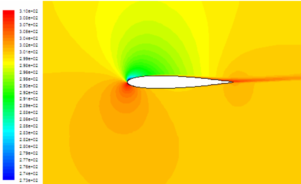
Şekil 5.16b. Naca 0012 Profili 0.4 Mach Sayısında 6° Hücüm Açısında Sıcaklık Dağılımı.
