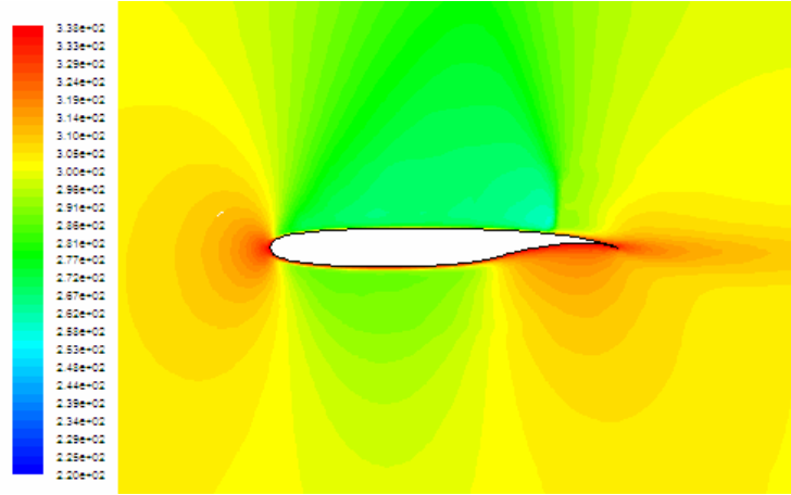
Şekil 5.19.a. Whitcomb Profili 0.8 Mach Sayısında 0^\circ Hücum Açısında Sıcaklık Dağılımı.
