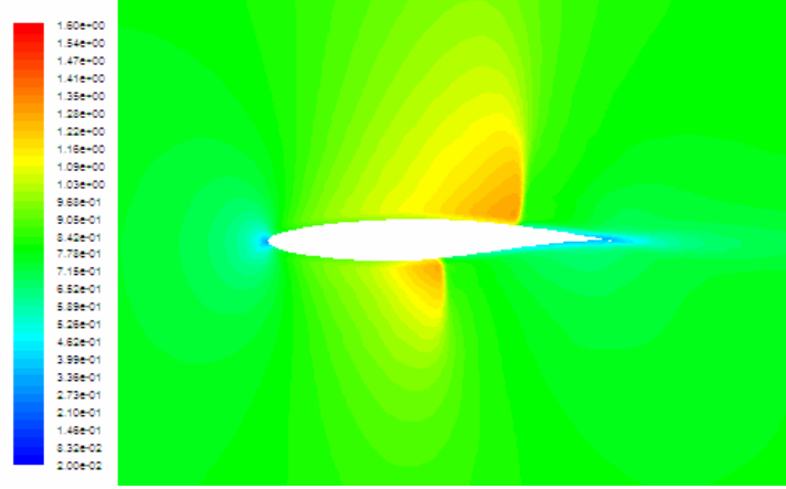
Şekil 5.22.a. RAE Profili 0.8 Mach Sayısında 0^\circ Hücum Açısında Mach Sayısı Değişimi.
