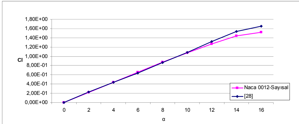
Şekil 5.1. Naca 0012 kanat profili için Abbott ve Doenhoff ile tez çalışmasındaki C_L değerinin karşılaştırılması.
