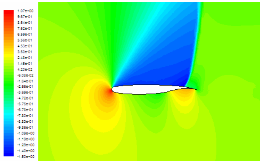
Şekil 5.29.b. Whitcomb Kanat Profili 0.8 Mach Sayısında 6^\circ Hücum Açısında Basınç Katsayısı Dağılımı.
