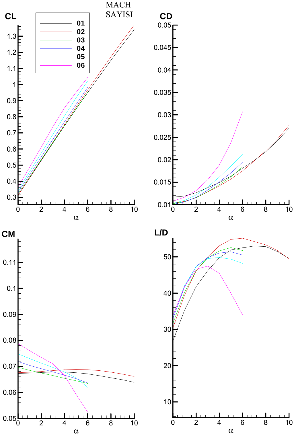
Şekil 5.5. Clark-Y Kanat Profiline Ait Aerodinamik Katsayılar Ve Taşıma/ Sürüklenme Kuvveti Oranı.
