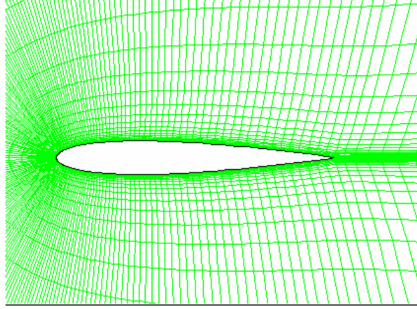
Şekil 4.4. Naca0012 (Simetrik) Kanat Profili.
