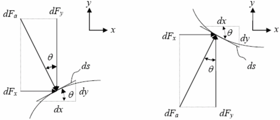
Şekil 2.9. Aerodinamik Kuvvetlerin Yüzeye Etkisi.
