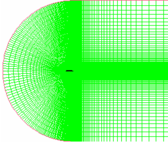
Şekil 4.8. Clark-Y Kanat Profilinde Modellenen Serbest Akım Bölgesi.
