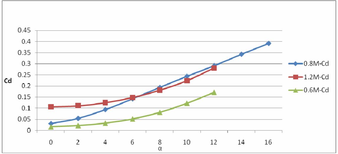
Şekil 5.8. RAE Kanat Profilinin Sürüklenme Katsayısı Değişimi.
