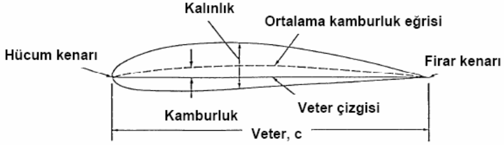
Şekil 2.1. Temel Kanat Profili Geometrisi.
