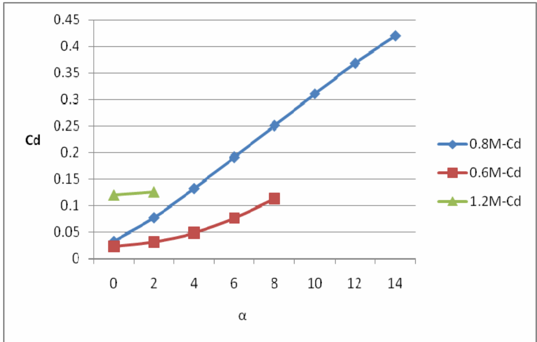
Şekil 5.9. Whitcomb Kanat Profilinin Sürüklenme Katsayısı Değişimi.
