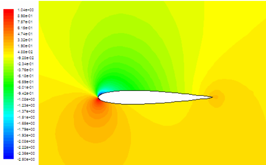
Şekil 5.26.b. Naca 0012 Profili 0.4 Mach Sayısında 6^\circ Hücüm Açısında Basınç Katsayısı Dağılımı.
