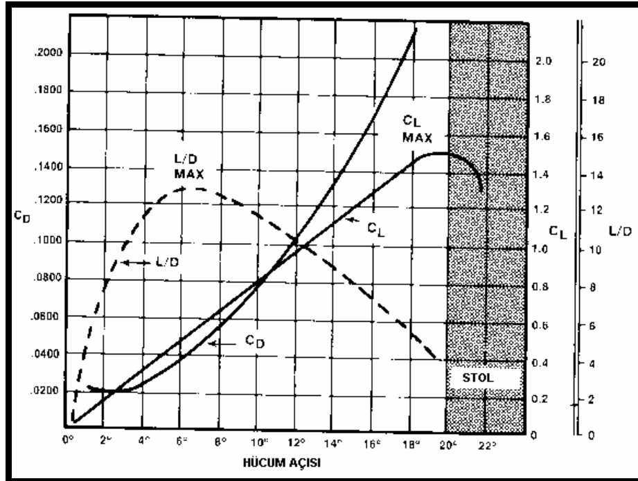
Şekil 2.7. Kaldırma Kuvveti - Sürüklenme Kuvveti İlişkisi.
