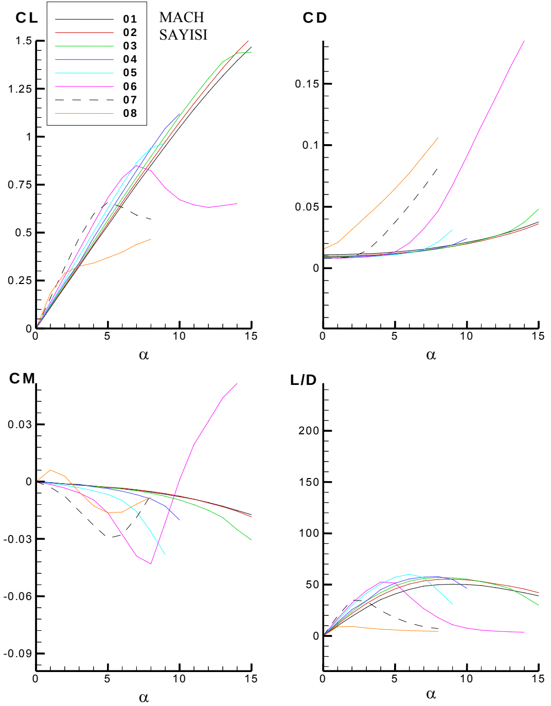
Şekil 5.4. NACA0012 Kanat Profiline ait Aerodinamik Katsayılar ve Taşıma/Sürüklenme Kuvveti Oranı.
