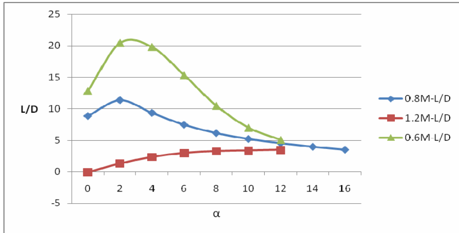
Şekil 5.12. RAE Kanat Profilinin Kaldırma Ve Sürüklenme Oranı Değişimi.
