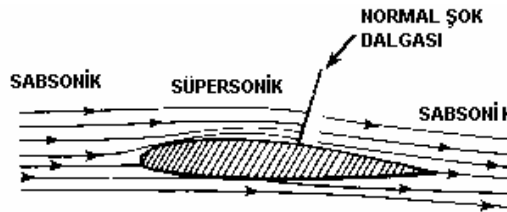
Şekil 2.11. Normal şok dalgasının şekli.
