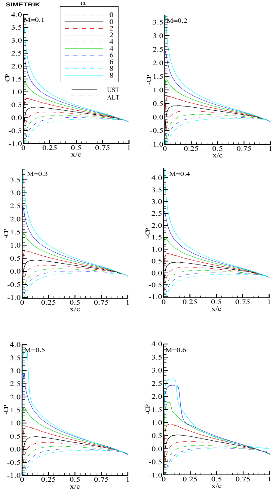
Şekil 5.24. Simetrik Kanat Profili İçin 0.1 Mach' dan 0.6 Mach'a Kadar C_p ' nin Hücum Açısıyla Değişimi.
