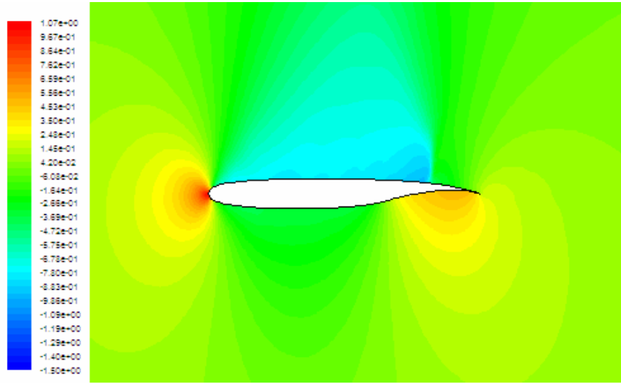
Şekil 5.29.a. Whitcomb Kanat Profili 0.8 Mach Sayısında 0^\circ Hücum Açısında Basınç Katsayısı Dağılımı.
