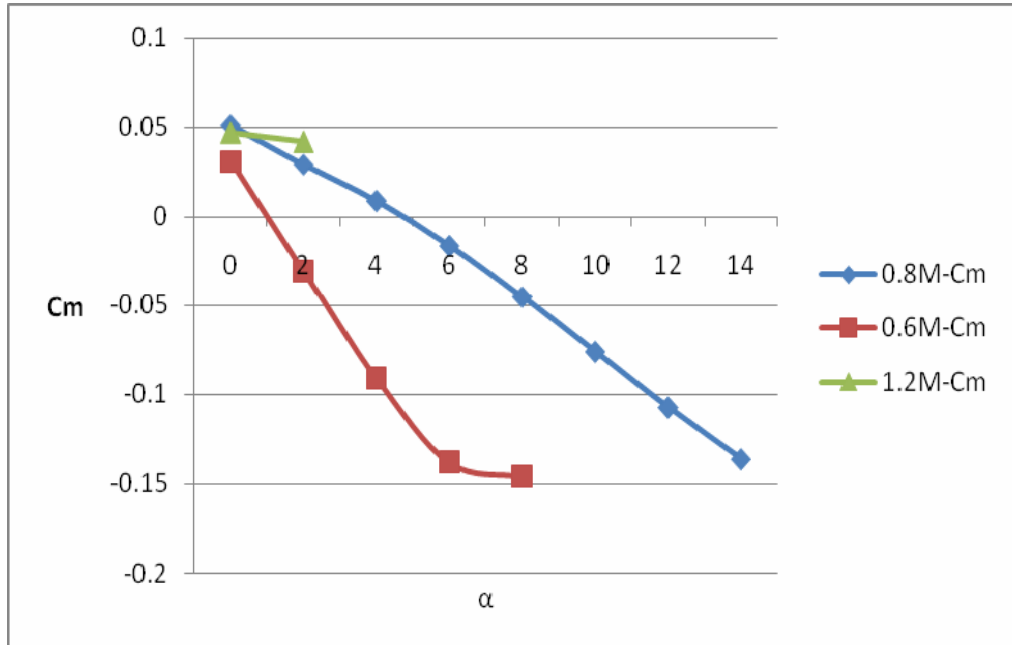
Şekil 5.11. Whitcomb Kanat Profiline Moment Katsayısı Değişimi.
