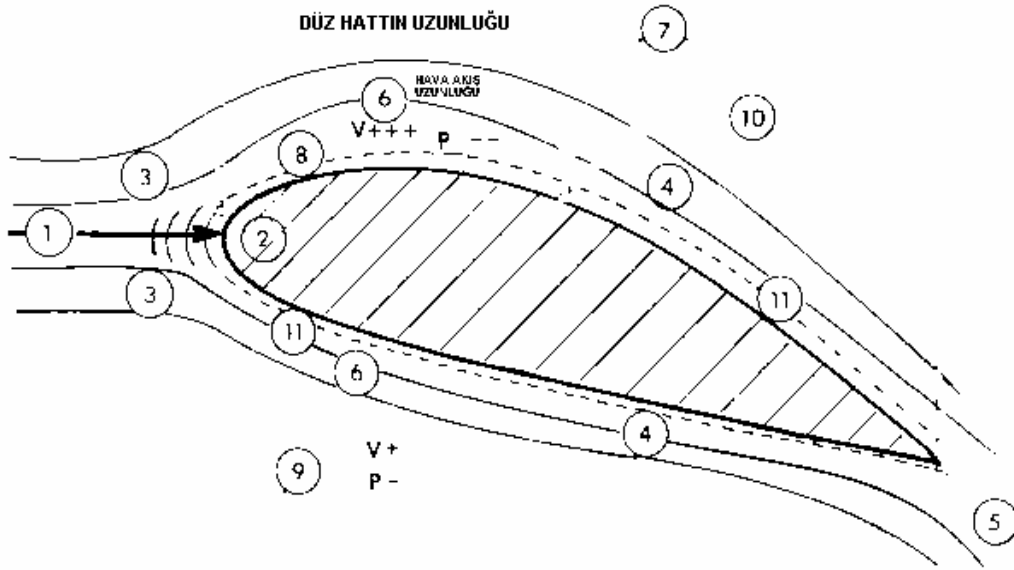
Şekil 2.2. Aerodinamik Kesit Boyunca Hava Akışı.
