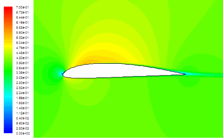
Şekil 5.21.a. Clark-Y Profili 0.4 Mach Sayısında 0^\circ Hücum Açısında Mach Sayısı Değişimi.
