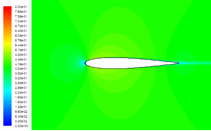
Şekil 5.20.a. Naca 0012 Profili 0.4 Mach Sayısında 0^\circ Hücum Açısında Mach Sayısı Değişimi.
