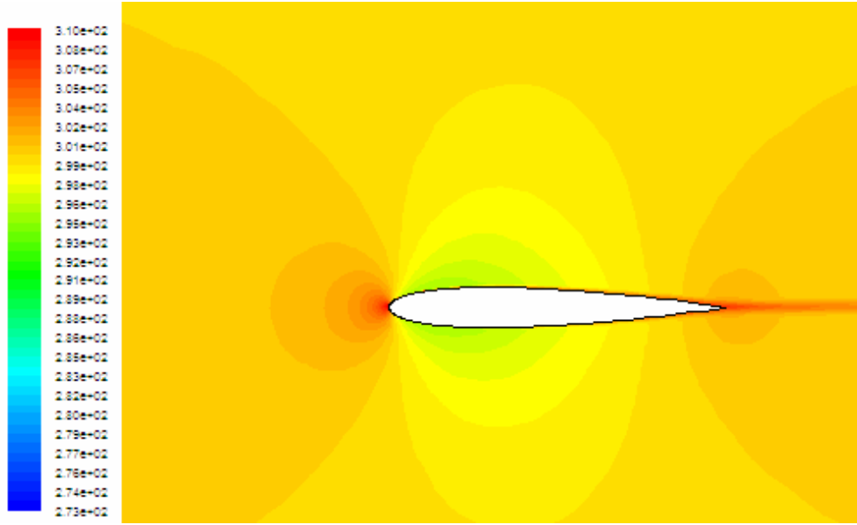
Şekil 5.16a. Naca 0012 Profili 0.4 Mach Sayısında 0° Hücüm Açısında Sıcaklık Dağılımı.
