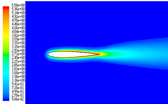
Şekil 4.3. Kanat Profilinin Türbülans Yoğunluğu Değişimi.
