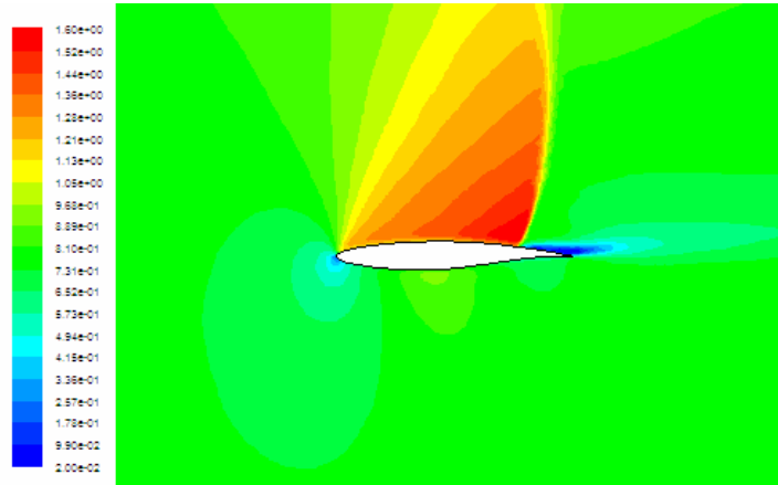
Şekil 5.22.b. RAE Profili 0.8 Mach Sayısında 6^\circ Hücum Açısında Mach Sayısı Değişimi.
