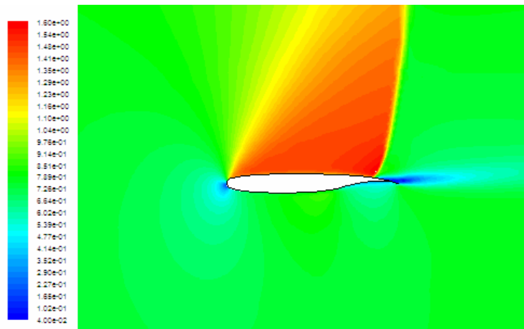
Şekil 5.23.b. Whitcomb Profili 0.8 Mach Sayısında 6^\circ Hücum Açısında Mach Sayısı Değişimi.
