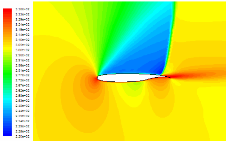
Şekil 5.19.b. Whitcomb Profili 0.8 Mach Sayısında 6^\circ Hücum Açısında Sıcaklık Dağılımı.
