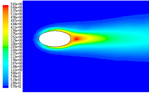
Şekil 4.2. Elipsin Türbülans Yoğunluğu Değişimi.
