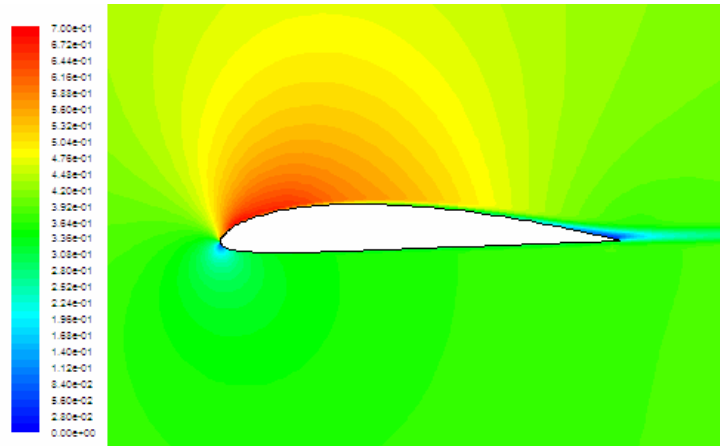
Şekil 5.21.b. Clark-Y Profili 0.4 Mach Sayısında 6^\circ Hücum Açısında Mach Sayısı Değişimi.
