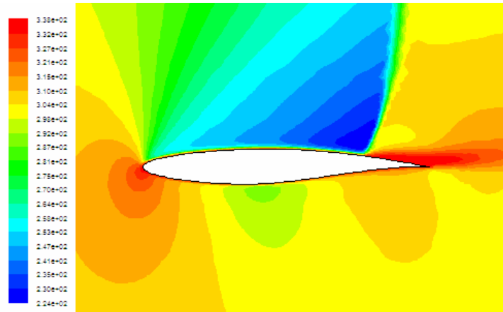
Şekil 5.18.b. RAE Profili 0.8 Mach Sayısında 6^\circ Hücum Açısında Sıcaklık Dağılımı.
