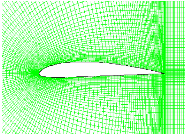
Şekil 4.5. Clark-Y (Kambur) Kanat Profili.
