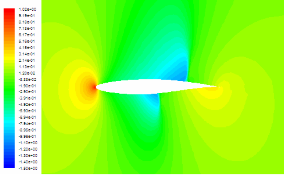
Şekil 5.28.a. RAE Profili 0.8 Mach Sayısında 0^\circ Hücum Açısında Basınç Katsayısı Dağılımı.
