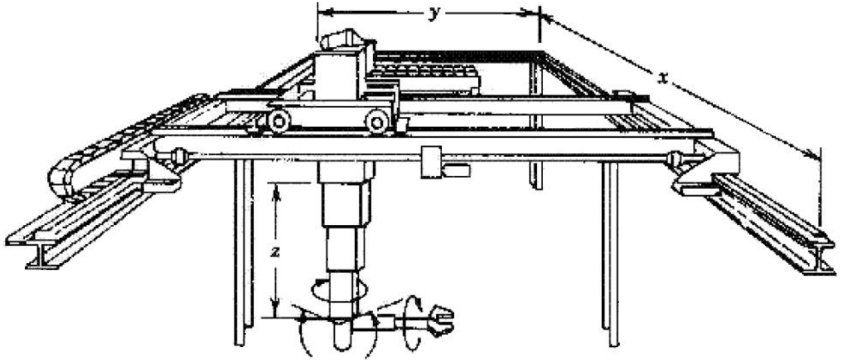
Şekil 3.5 Kartezyen robot
