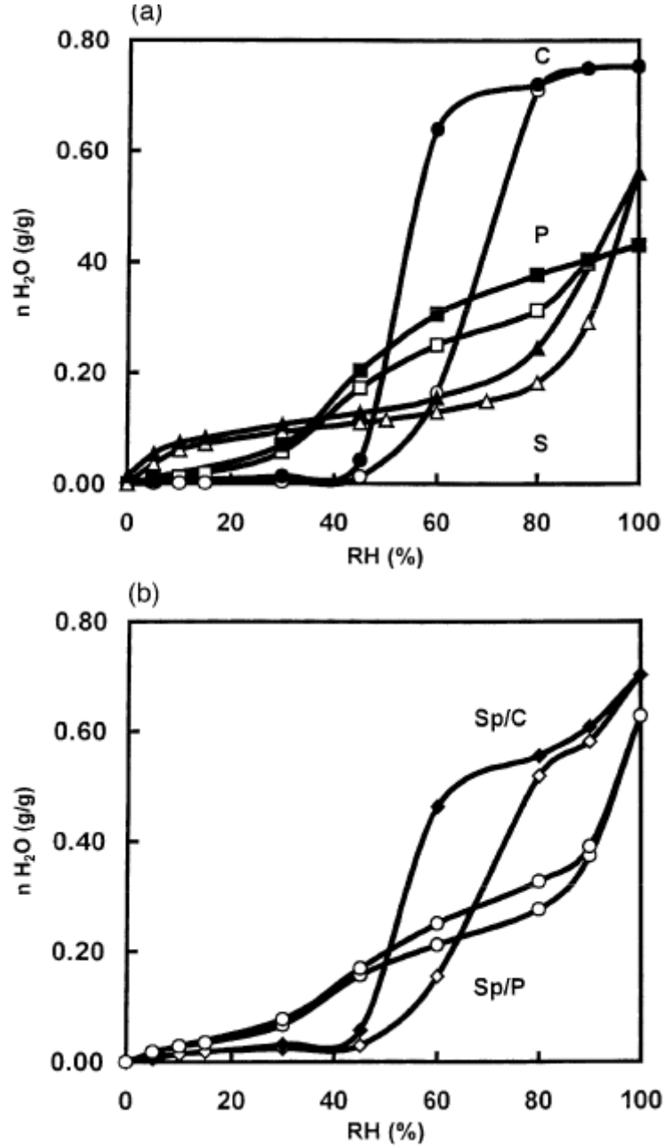
Şekil 5.12. 23°C’de havadaki su buharının adsorpsiyon/desorpsiyon izotermi (a) Sepiyolit ve aktiflenmiş karbon için, (b) Pellets Sp/P ve Sp/C [93]
