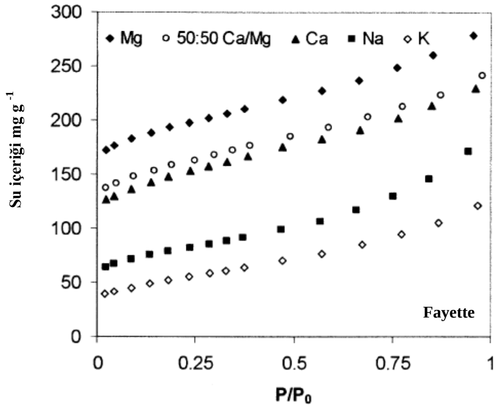
Şekil 5.3. \text{Ca}^{2+} , 50:50 \text{Ca}^{2+}/\text{Mg}^{2+} , \text{Mg}^{2+} , \text{K}^{+} , ve \text{Na}^{+} ile değiştirilmiş Blount ve Fayette toprak killeri için su adsorpsiyon izotermeleri [71]
