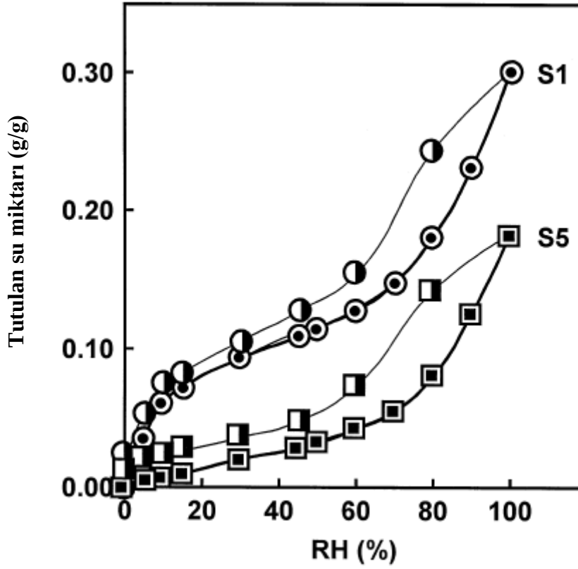
Şekil 5.7. 23°C’de (açık semboller) ve 40°C’de (kapalı semboller) havadaki su buharının adsorpsiyon/desorpsiyon izotermi. Yarı-kapalı semboller, desorpsiyon kollarına karşılık gelmektedir [75]
