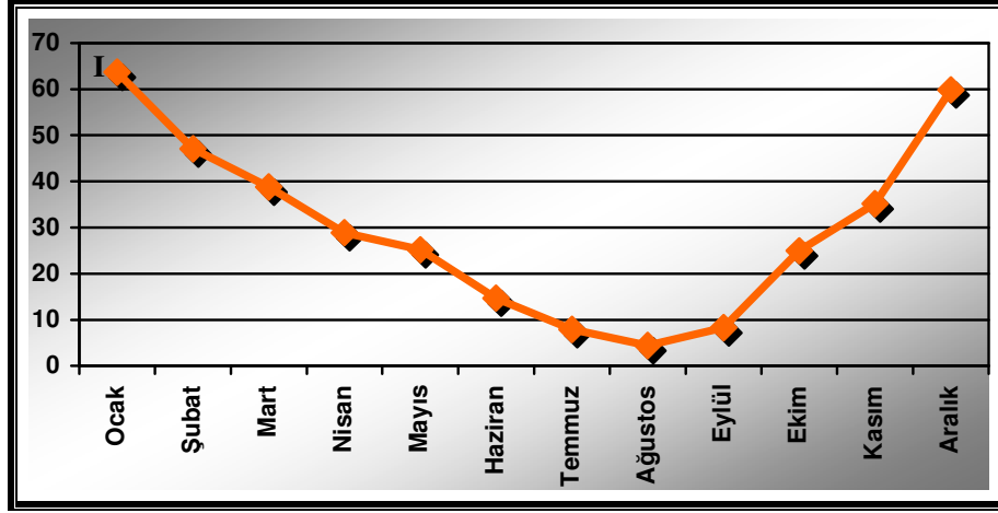
Şekil 1.11. De Martonne'nin aylık kuraklık indisinin Bozüyük'e uygulanması.
