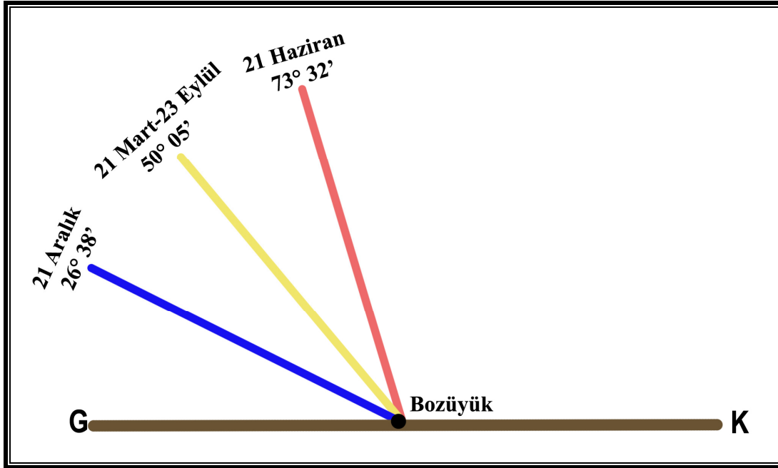
Şekil 1.1. Bozüyük'e güneş ışınlarının belirli tarihlerde geliş açıları.
