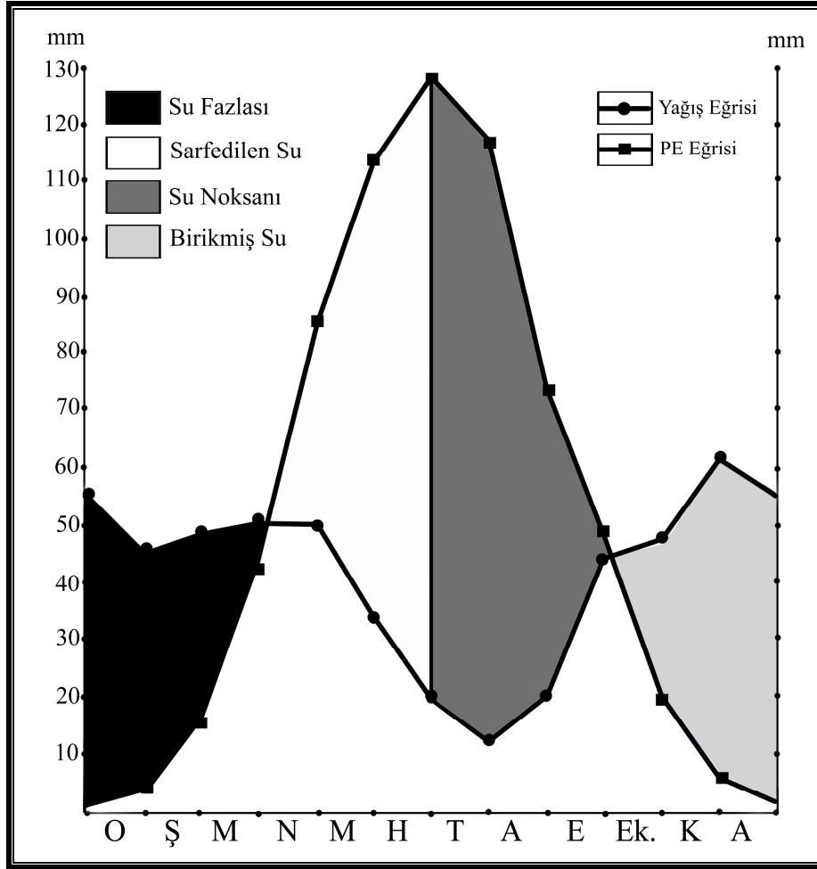
Şekil 1.12. Thornthwaite' a göre Bozüyük'ün su bilançosu.
