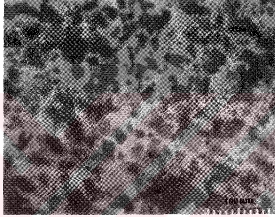
Şekil 6.22. Doğal hammaddelerden hazırlanmış ve 1350 °C'de 1 saat sinterlenmiş D1 numunesinin optik mikroskop görüntüsü (X160 büyütme)
