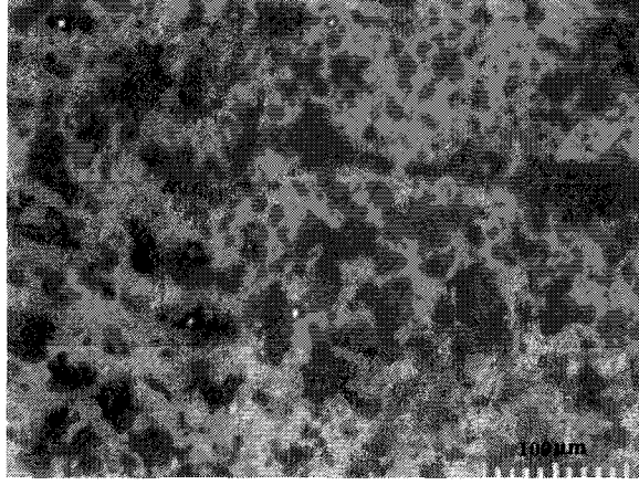
Şekil 6.27. Doğal hammaddelerden hazırlanmış ve 1350 °C’de 3 saat sinterlenmiş D2 numunesinin optik mikroskop görüntüsü (X160 büyütme)
