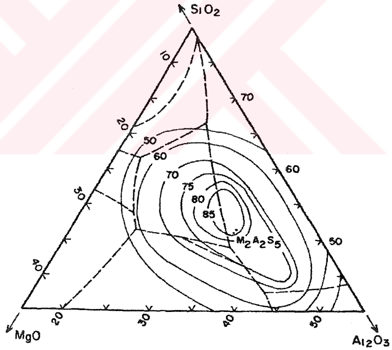
Şekil 4.6. Sinterlenmiş çeşitli oksit kompozisyonlarındaki bünyelerdeki kordiyerit yüzdesi [34]
