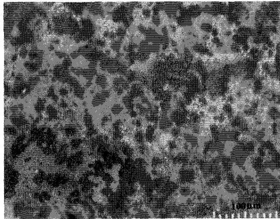
Şekil 6.23. Doğal hammaddelerden hazırlanmış ve 1350 °C'de 3 saat sinterlenmiş D1 numunesinin optik mikroskop görüntüsü (X160 büyütme)
