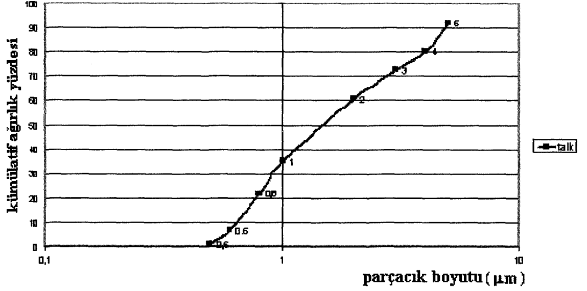
Şekil 6.8. Talkın parçacık boyut dağılımı grafiği
