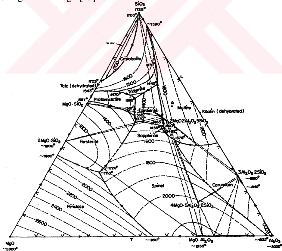
Şekil 4.1. \text{MgO}-\text{Al}_2\text{O}_3-\text{SiO}_2 Üçlü Denge Diyagramı [27]
