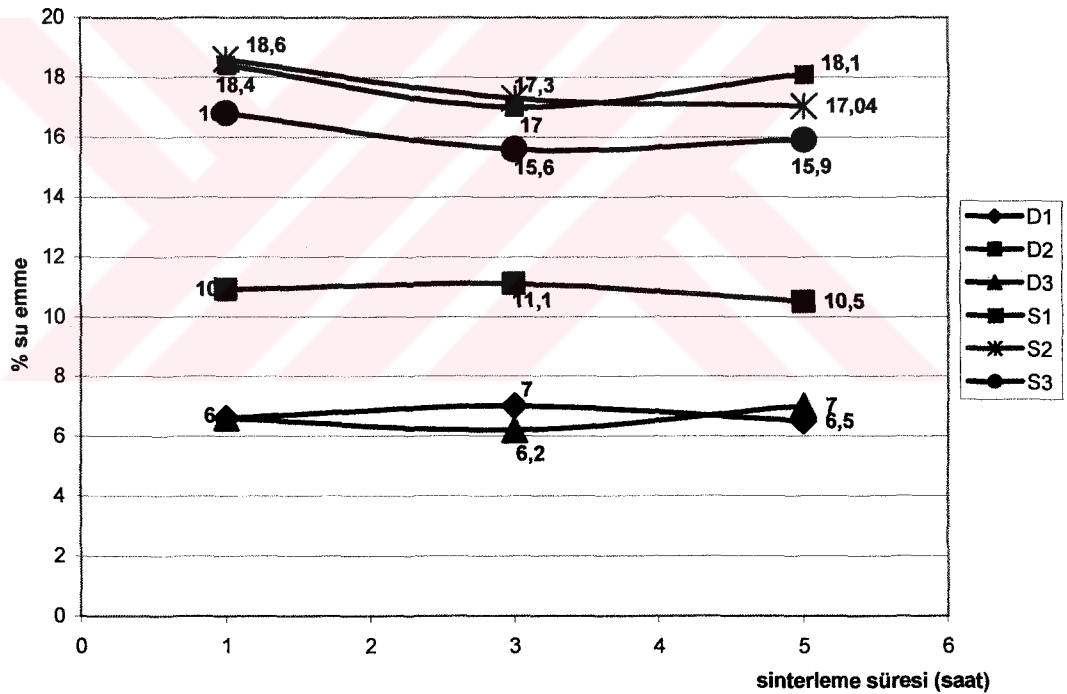
Şekil 6.15. Doğal hammaddelerden ve sentetik tozlardan hazırlanmış numunelerin su emme değerleri
