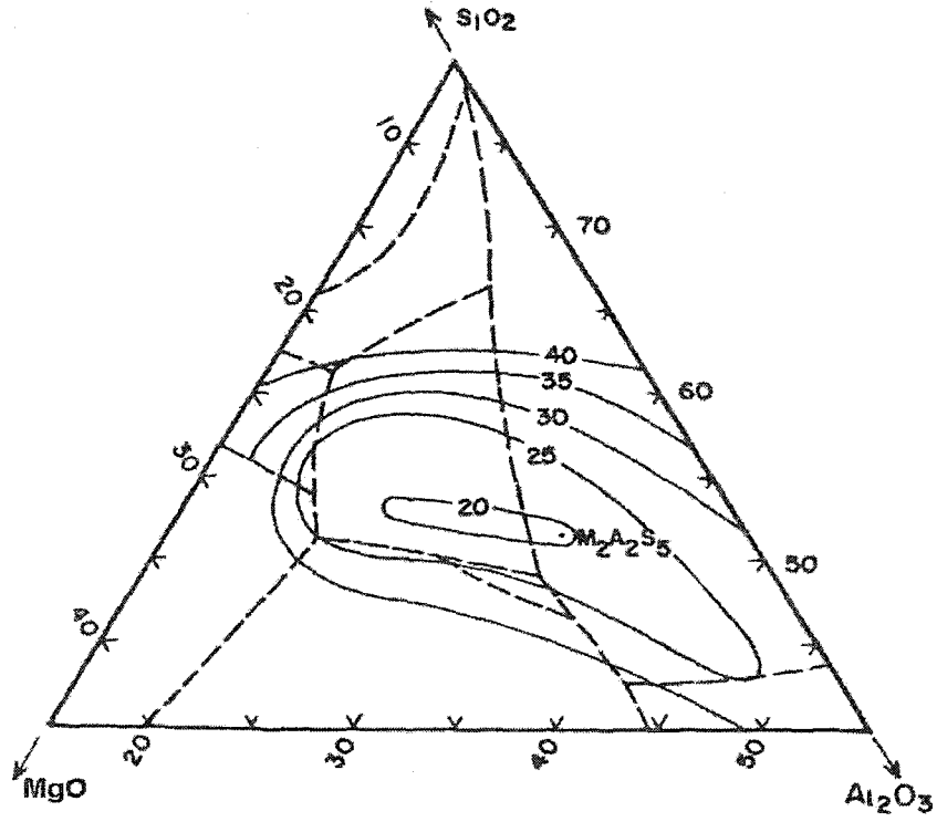
Şekil 4.5. 1300 °C’de sinterlenmiş çeşitli oksit kompozisyonlarındaki bünyelerin ısı genleşme katsayıları [34]
