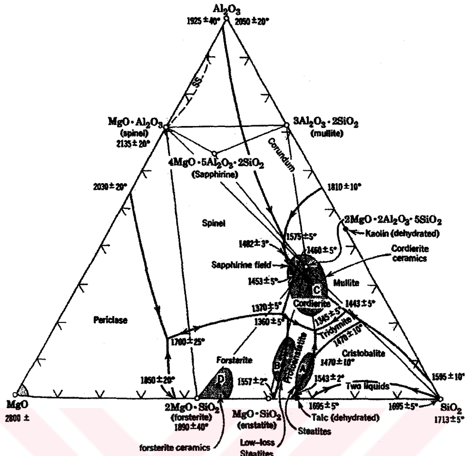
Şekil 4.2. MgO-Al 2 O 3 -SiO 2 üçlü faz sisteminde yeralan çeşitli bileşimler [25]
