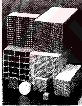
Şekil 4.8. Şekillendirilmiş kordiyerit bal peteği yapıları [18]
