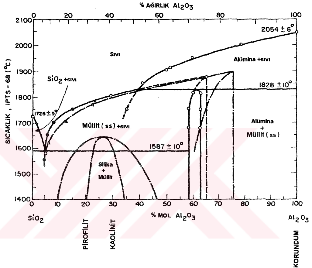
Şekil 4. 9. \text{SiO}_2\text{-Al}_2\text{O}_3 İkili denge diyagramında hammaddelerin konumu [46]
