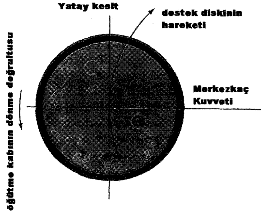
Şekil 5.4. Gezen tipi değirmenin çalışma prensibi
