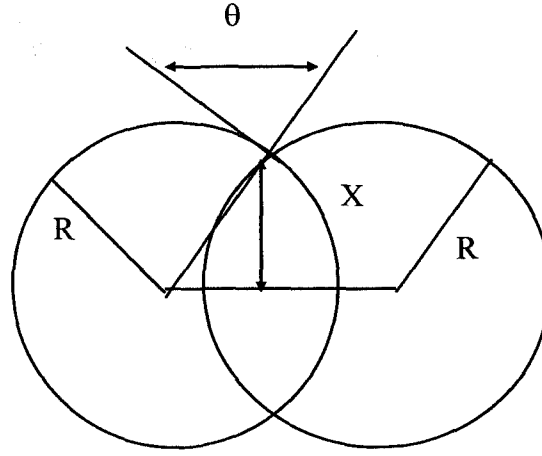
Şekil 2. Boyun Büyüklüğü ve Dihedral Açısı [25]
