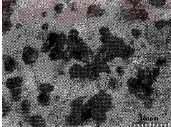
Şekil 26. Doğal hammaddelerden hazırlanmış ve 1350 °C'de 5 saat sinterlenmiş D3 numunenin optik mikroskop görüntüsü (X160 büyütme)
