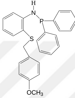
Şekil 4:3 Ligand(L 3 )'in Yapısı
