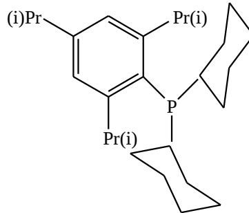
Şekil 2:8 (2,4,6triizopropilfenil)disiklopentilfosfin( www.alpha.chem.umb.edu )
