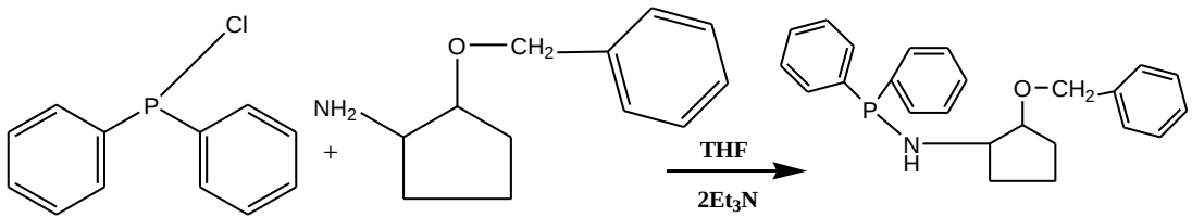
řekil 3:5 Ph 2 PNHC 5 H 8 OCH 2 C 6 H 5 Sentezi
