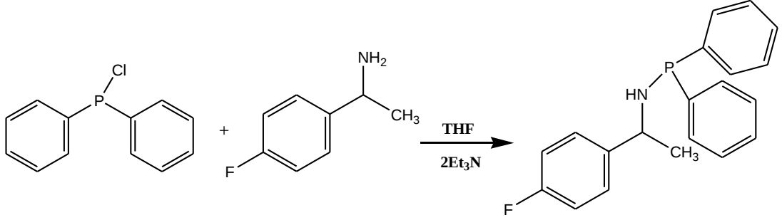
řekil 3:4 Ph 2 PNHCHCH 3 C 6 H 4 F Sentezi
