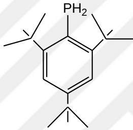
Şekil 2:4 2,4,6-tri-t-bütilfenilfosfin (Brynda 2005)
