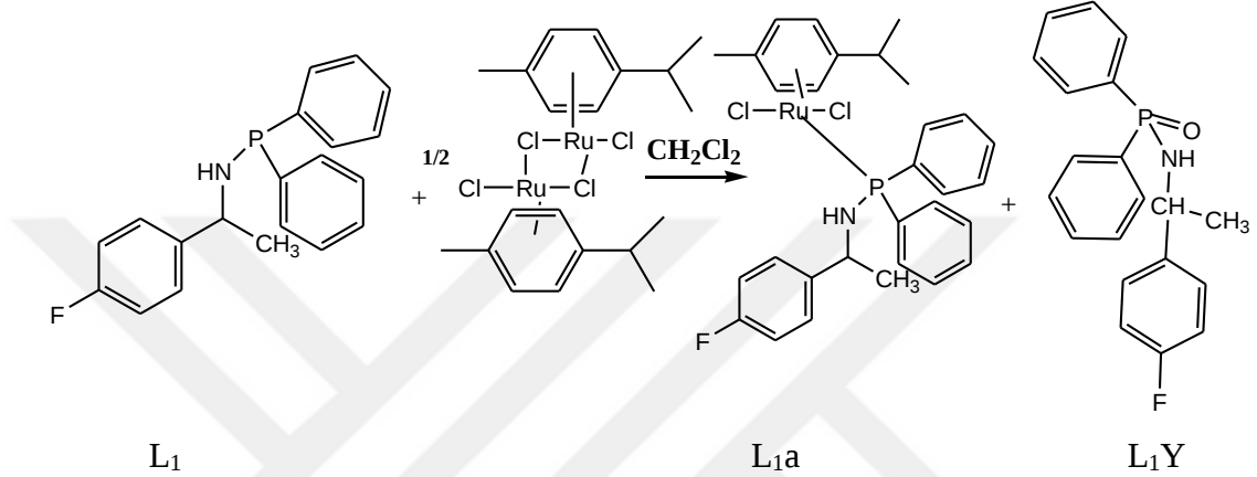
Şekil 3:7 (L 1a ) Kompleksinin Sentezi
