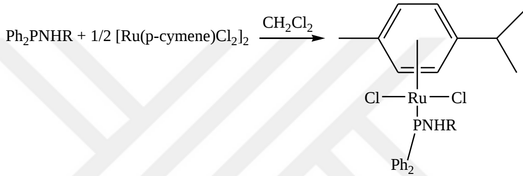
Şekil 2:16 Aminofosfinin Sentezlenme Reaksiyonu (Kayan ve diğ.2011)
