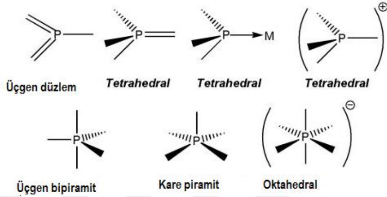
Şekil 1:1 Fosforun Geometrik Yapıları (Gopalakrishnan, 2009).
