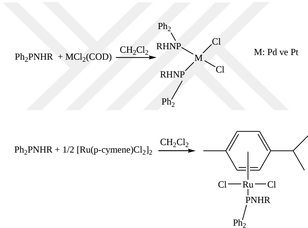
Şekil 3:1 Aminofosfinin Sentezlenme Reaksiyonu (Kayan ve diğ.2011)
