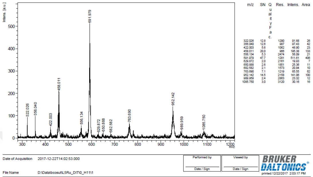
Şekil 6.3.4. (L 1 a) Kompleksin Kütle Spektrumu
