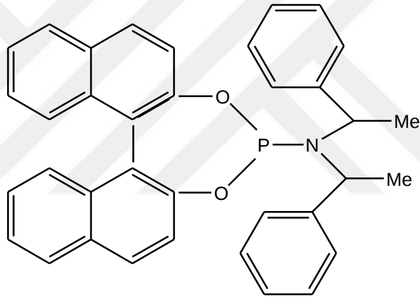
Şekil 2:13 (R)-2,2'-Binaftol-(S,S)-di-(1-fenilsetil)aminyilfosfin(Smith ve diğ. 2008)
