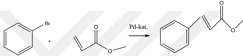
Şekil 2:22 Heck Reaksiyonu
