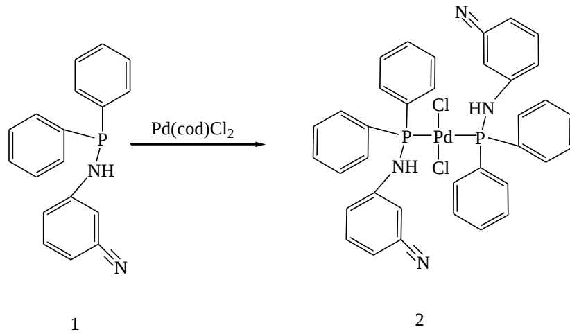
Şekil 2:27 Aminofosfin Palladyum(II) Kompleksinin Sentezi
