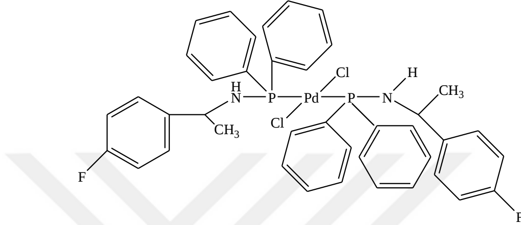
Şekil 4:8 L 1b kompleksinin yapısı
