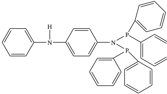
Şekil 2:11 N,N-bis(difenilfosfino)-4-aminodifenilamin (Kayan ve diğ. 2011)
