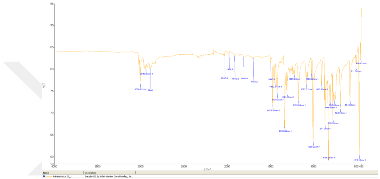
Şekil 6.1.1: Dikloro(1,5-siklooktadien)platin(II) [Pt(COD)Cl 2 ] FT-IR spektrumu
