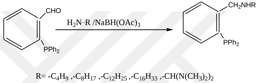
Şekil 2:26 Aminofosfinlerin Sentezi
