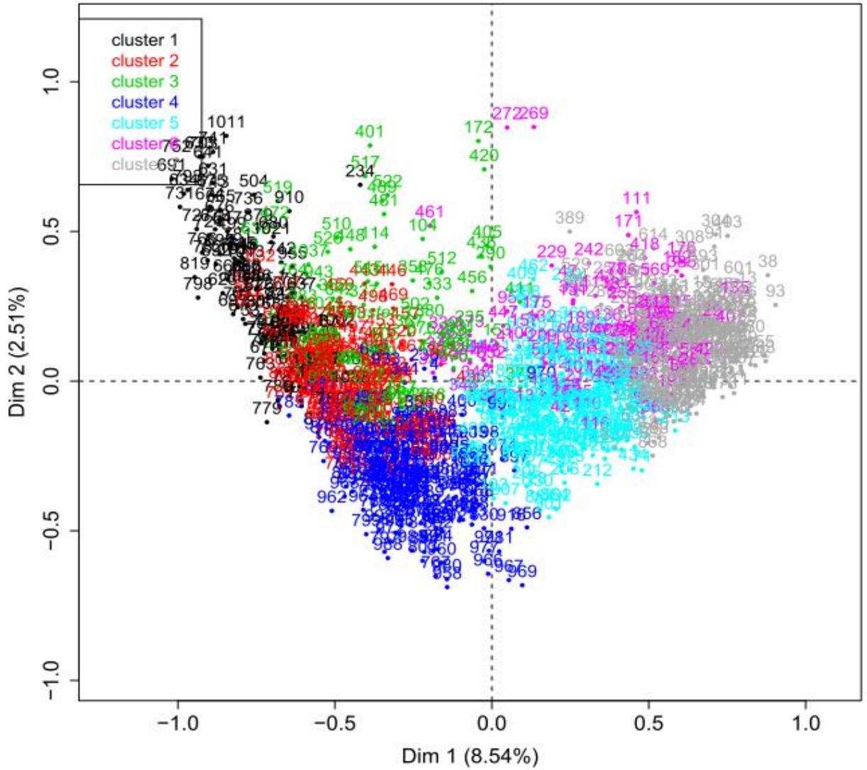
Şekil 4.4. Katmanlar Programının Kullanılması Sonucunda Ortaya Çıkan Grupların İki Boyutlu Düzlemde Dağılımı
