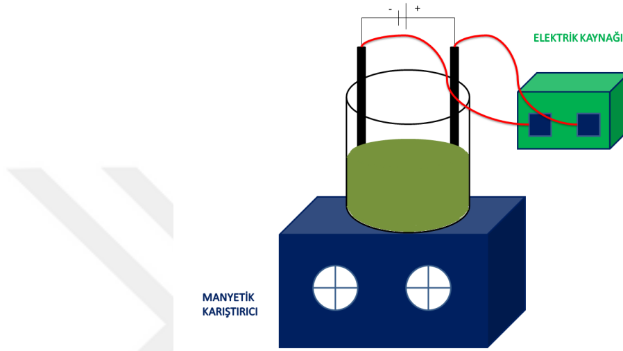
Şekil 5.2. Anodik oksidasyon liç ünitesi.
