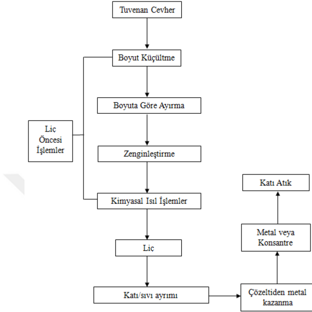
Şekil 3.1. Liç işlemi genel akım şeması [3].
