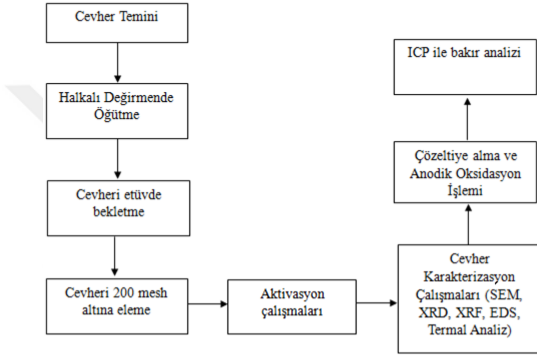
Şekil 6.1. Deneysel çalışmaların akış şeması.
