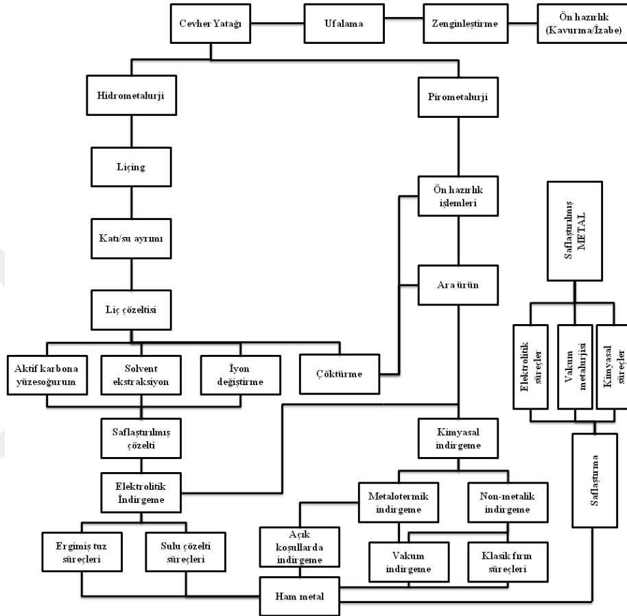
Şekil 2.3. Metal üretimi için genel bir akım şeması [14].
