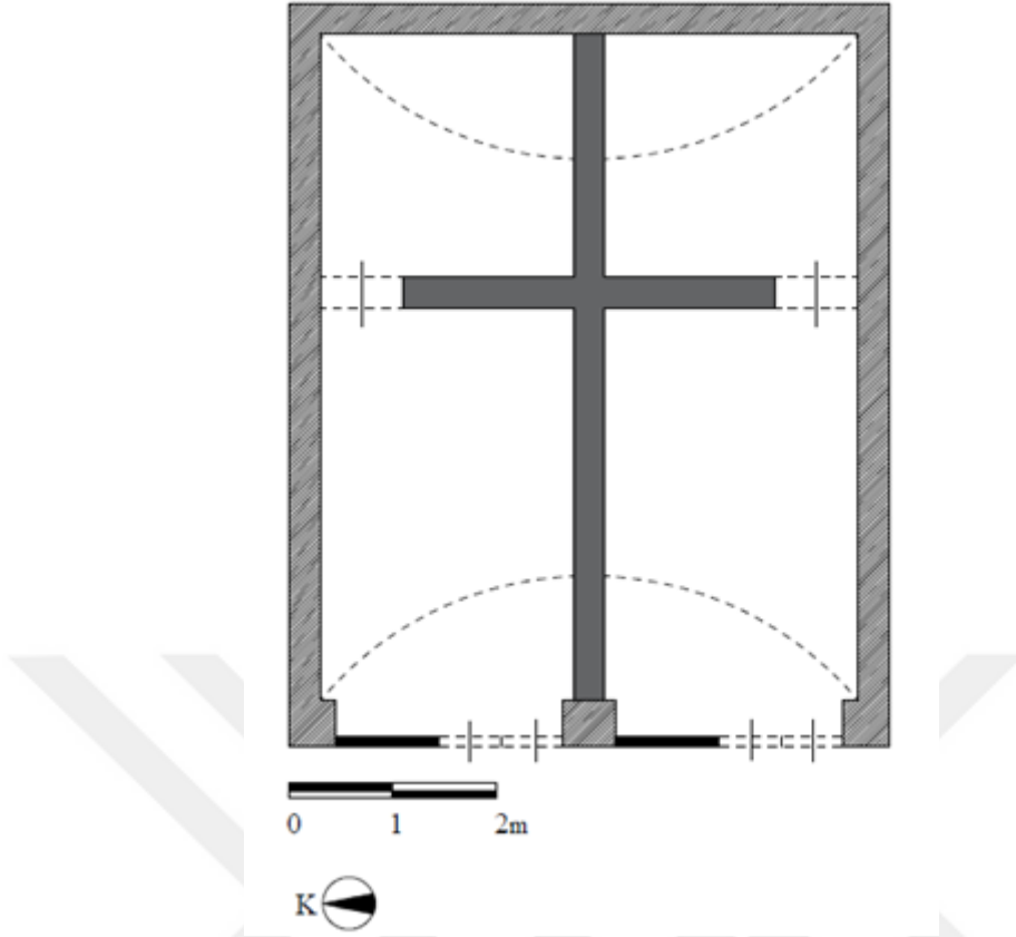
Şekil 15: Uşak/ Ulubey 11. Dükkan Röleve Planı (2018).
