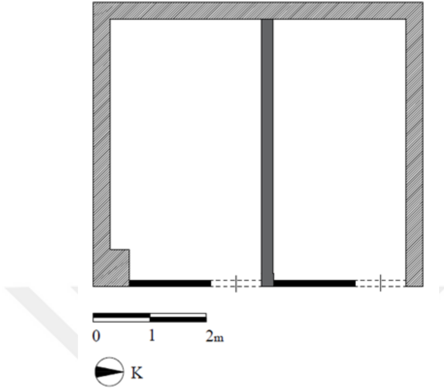
Şekil 3: Uşak/ Ulubey 2. Dükkan Röleve Planı (2018).
