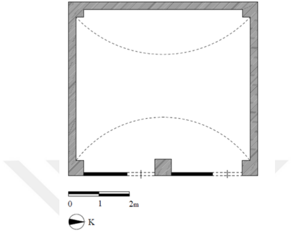
Şekil 1: Uşak/ Ulubey 1. Dükkan Röleve Planı (2018).
