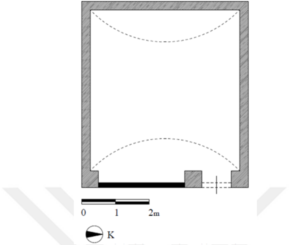
Şekil 7: Uşak/ Ulubey 4. Dükkan Röleve Planı (2018).
