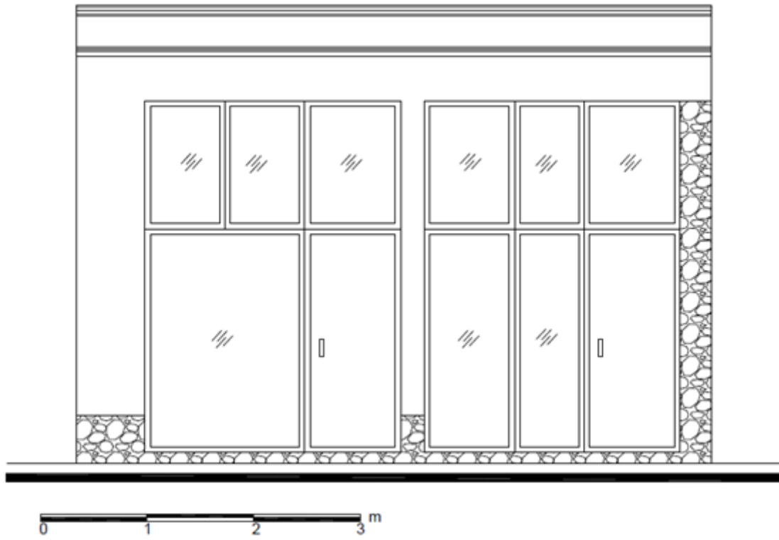
Şekil 4: Uşak/ Ulubey 2. Dükkan Doğu Cephesi Çizimi (2018).
