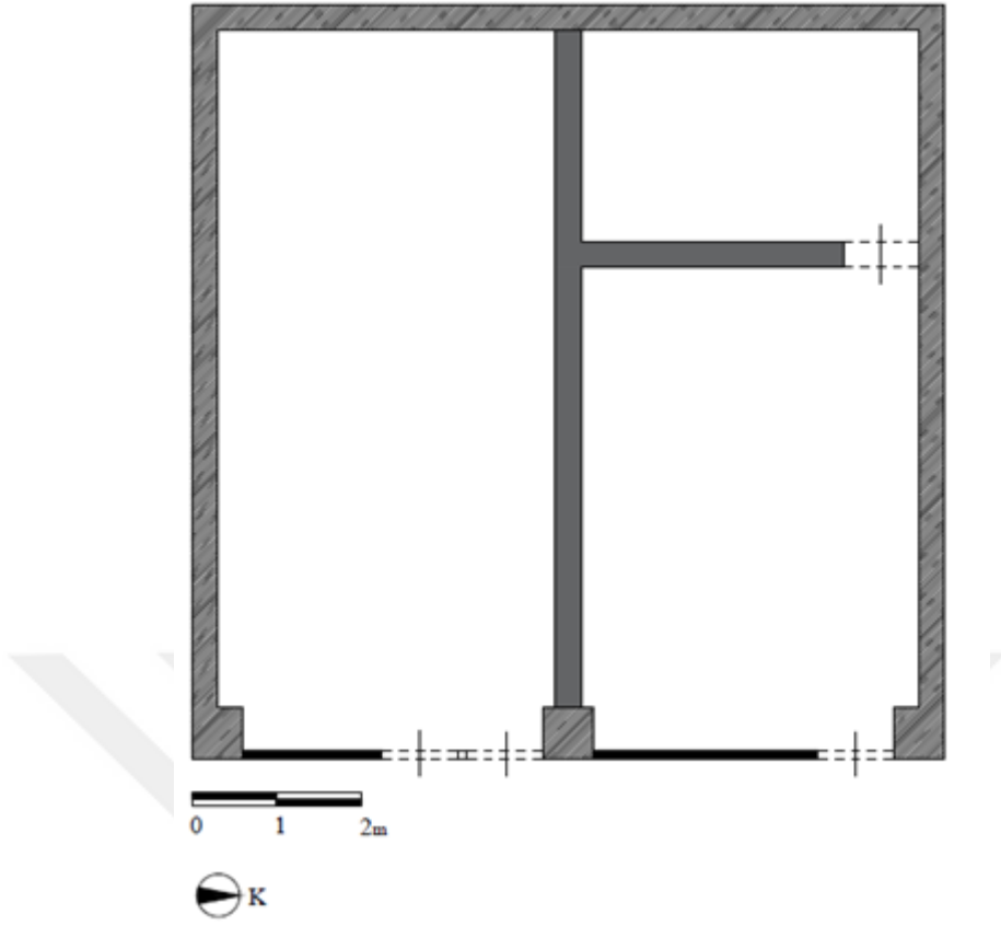
Şekil 24: Uşak/ Ulubey 18. Dükkan Röleve Planı (2018).
