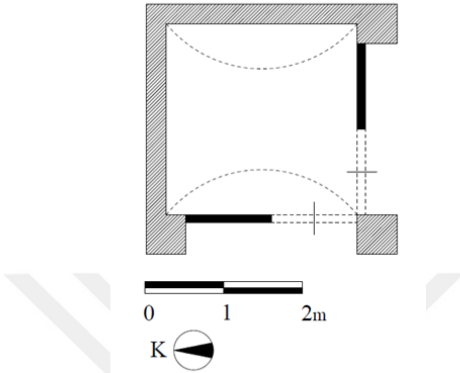
Şekil 9: Uşak/ Ulubey 5. Dükkan Röleve Planı (2018).
