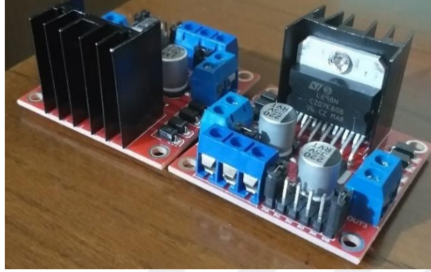
Şekil 3.9. L298N Motor sürücü devre kartı ön ve arka görünümü
