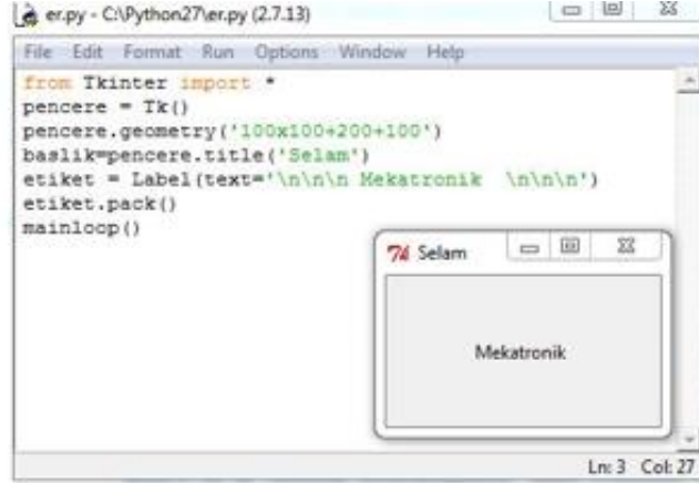
Şekil 3.16. Python simgesi(Python, 2001-2019) ve basit bir program yapısı
