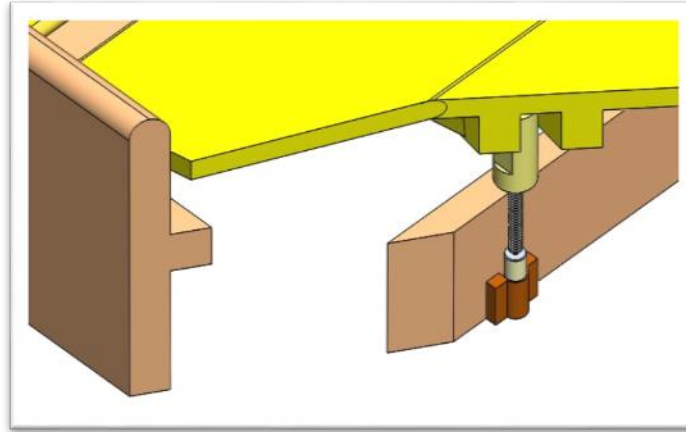
Şekil 3.14. Hasta yatađı orta kısmının DC motor bağlantısı SolidWorks tasarımı
