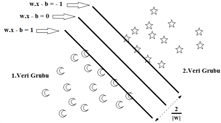
Şekil 3.40. Sınıflandırmada sınır belirlenmesi
