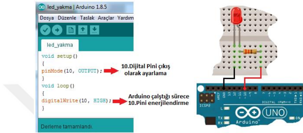
Şekil 3.7. Led yakma kod yapısı ve kart bağlantısı(Yaman, 2016)
