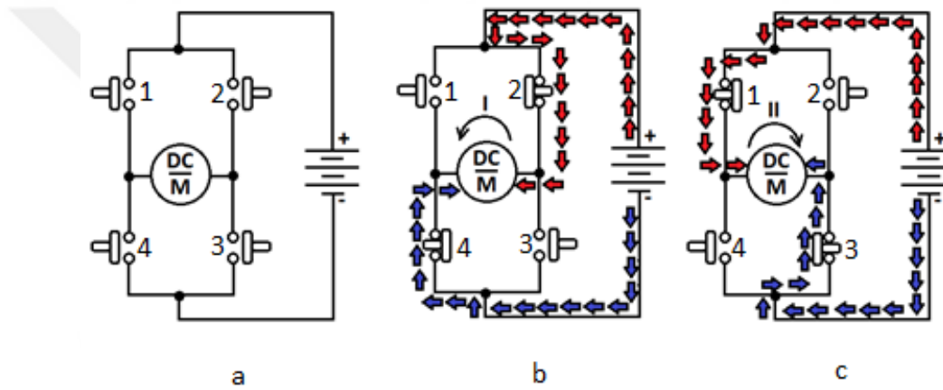
Şekil 3.8. H Köprüsü yöntemi
