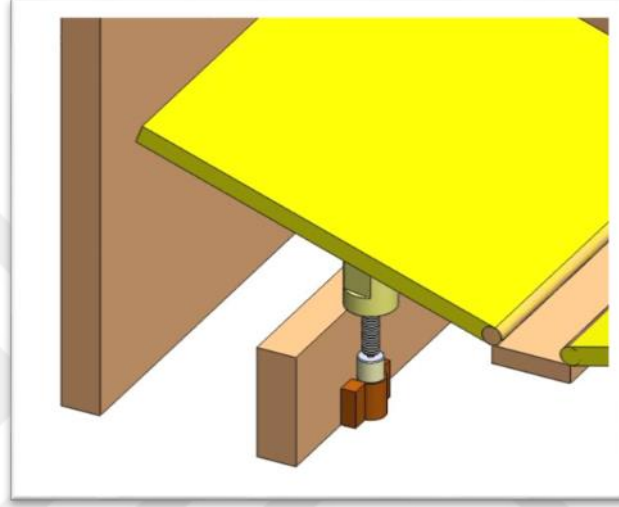
Şekil 3.13. Hasta yatađı baş kısmının DC motor bağlantısı SolidWorks tasarımı
