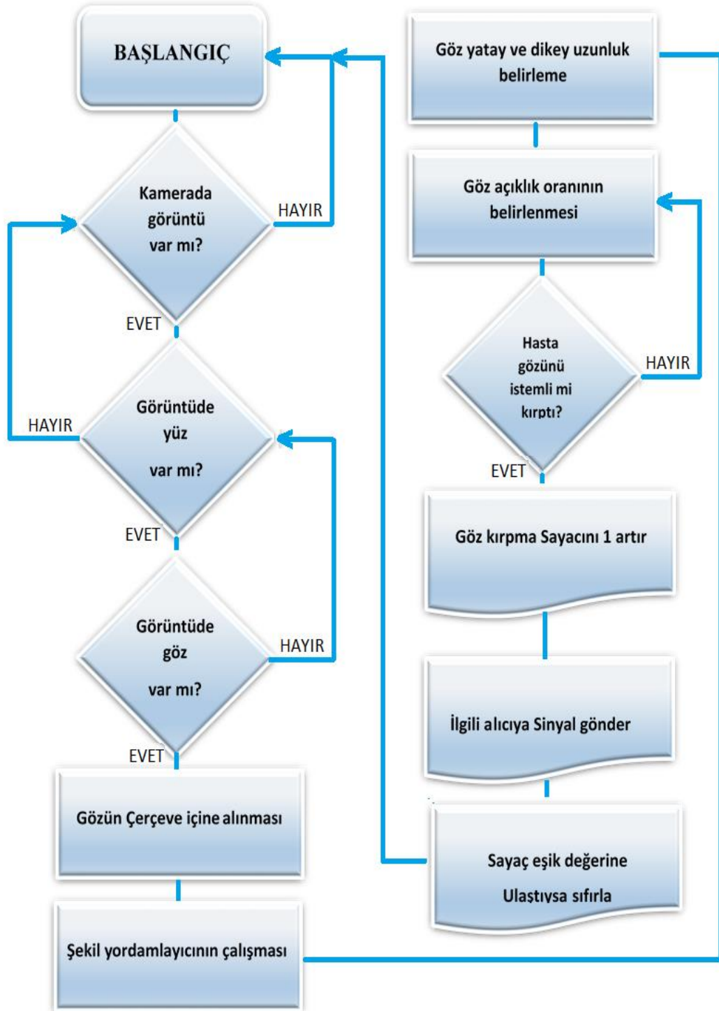
Şekil 3.48 Yazılım Algoritması
