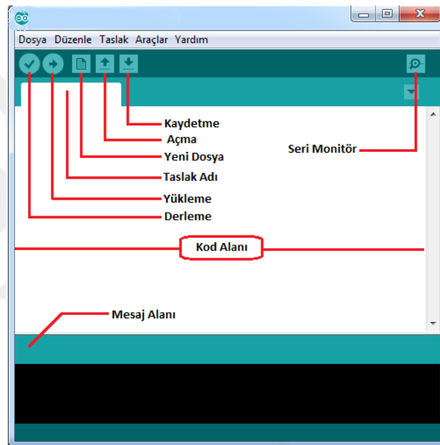
Şekil 3.6. Arduino IDE program arayüzü
