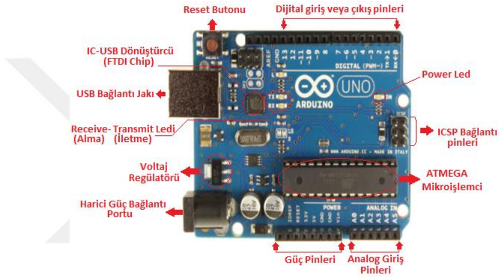
Şekil 3.5 Arduino UNO Kontrol Kartı Pin Yapısı
