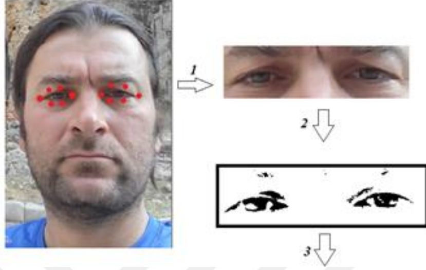
Şekil 3.45. Göz kırpma tespit işlem sıralaması
