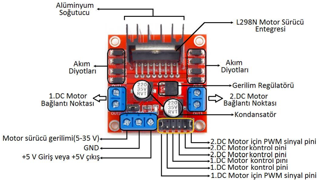
Şekil 3.10. L298N Motor sürücü devre kartı bağlantı noktaları
