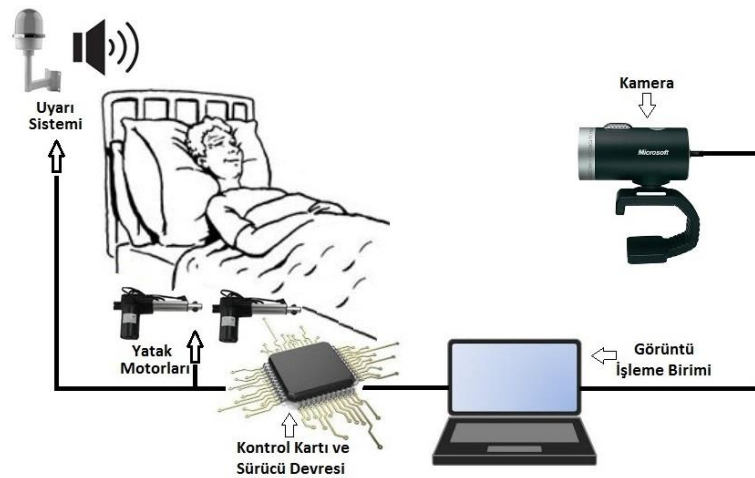
Şekil 3.1. Akıllı yatak sistemin genel yapısı
