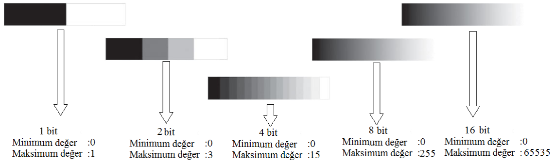
Şekil 3.25. Farklı çözünürlük gri tonlama değerleri
