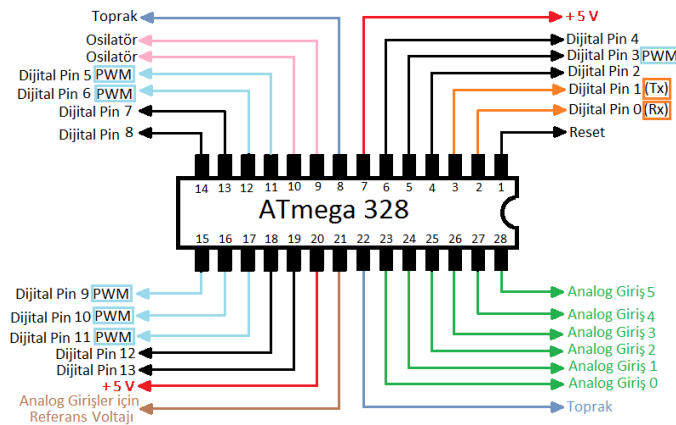
Şekil 3.4. ATmega 328 Mikrodenetleyici
