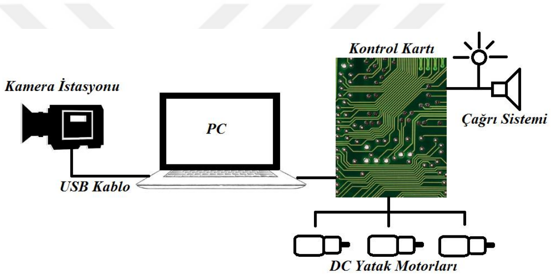
Şekil 4.1. Sistem Yapısı
