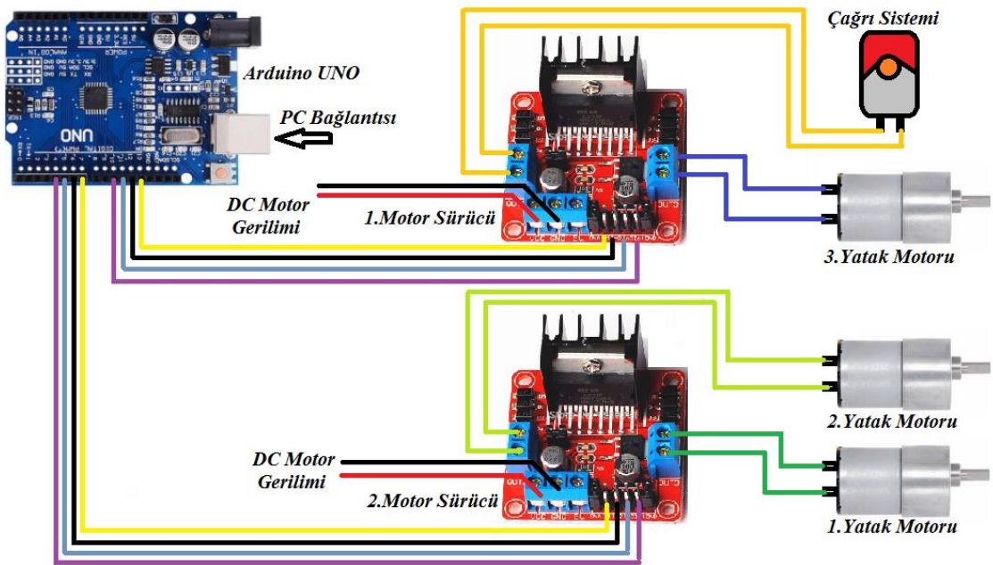
Şekil 3.53. Tez çalışması kontrol devresi
