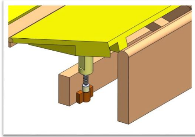
Şekil 3.15. Hasta yatağı orta kısmının DC motor bağlantısı SolidWorks tasarımı
