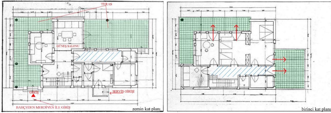
Şekil-4. 28: İhsan Sami Evi Plan Şeması İncelemesi
