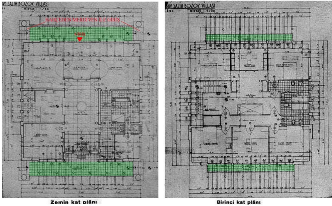
Şekil-4. 33: Suadiye’de Bir Villa Plan Şeması İncelemesi
