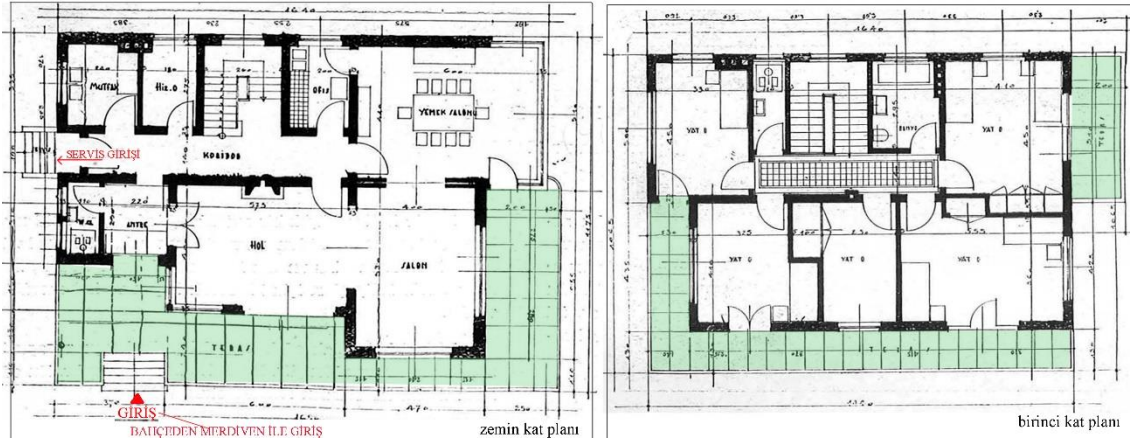
Şekil-4. 29: Kalamış'ta Bir Villa Plan Şeması İncelemesi
