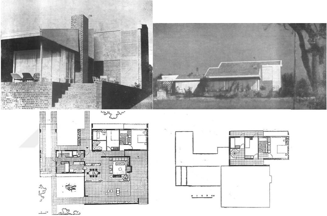
Şekil-3. 32: Enis Korkan "Yelkenci Villası", Tuzla, 1962
