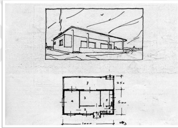
Şekil-2.8 : Mimar Abidin Yazlık Ev Taslağı (Abidin, 1933).
