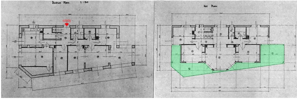
Şekil-4. 32: Cemil Filmer Evi Plan Şeması İncelemesi
