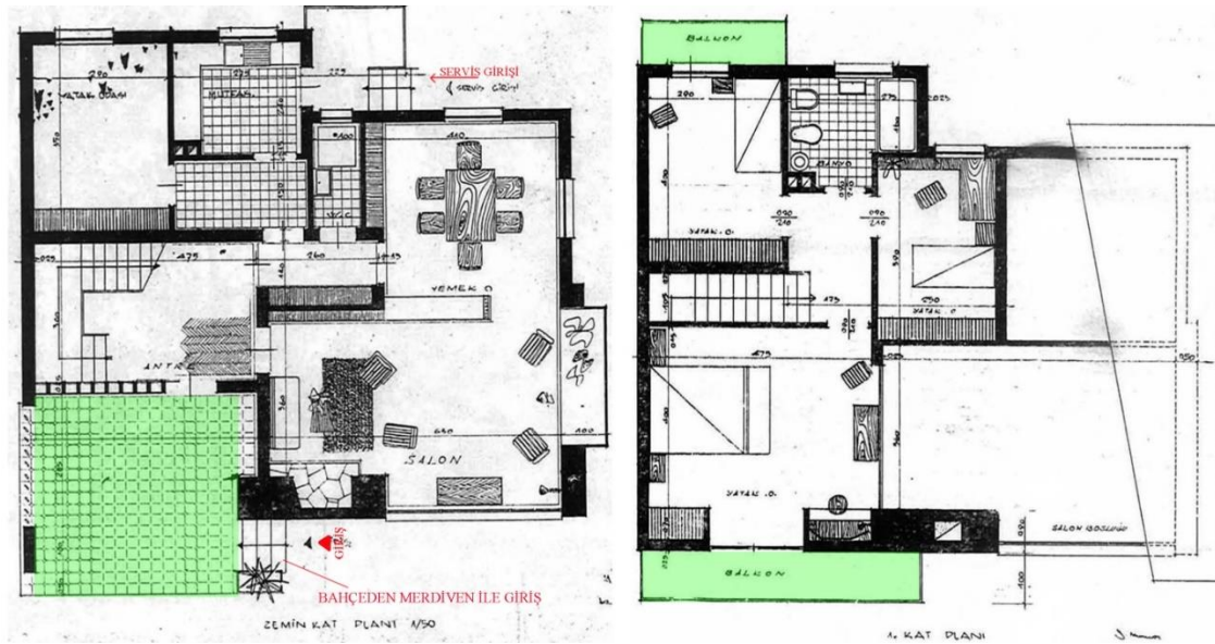
Şekil-4. 36: Mithat Güldü Evi Plan Şeması İncelemesi
