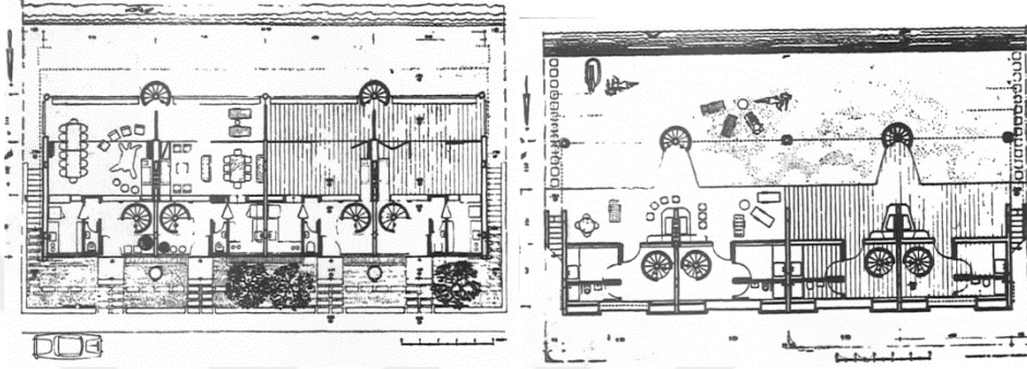
Şekil-3. 33: Yılmaz Sanlı Dört Bloklı Yaz Evi, Kumburgaz, 1969
