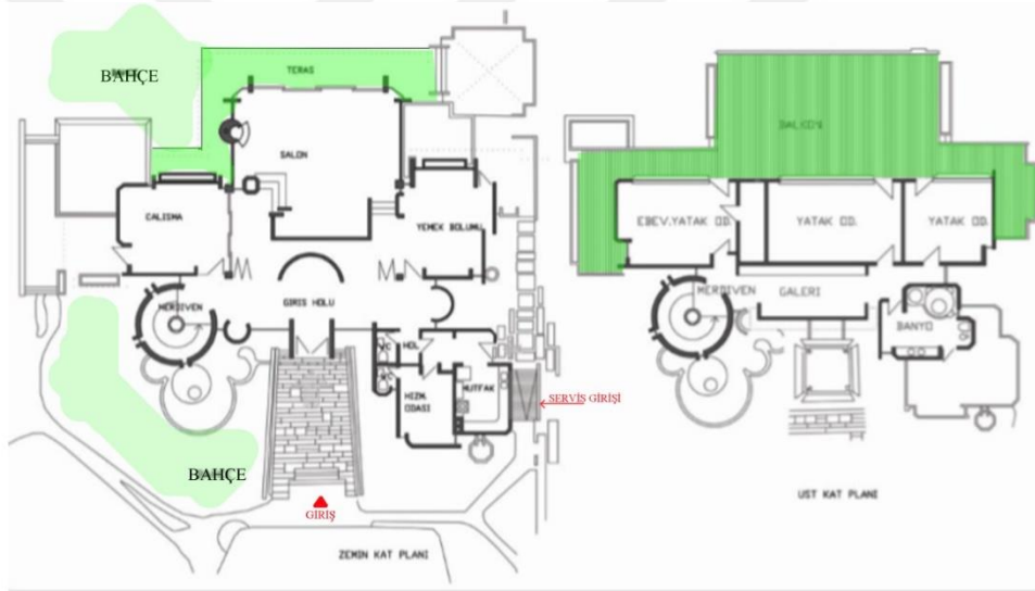
Şekil-4. 38: Özdemiroğlu Yalısı Plan Şeması İncelemesi
