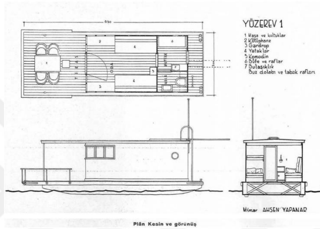
Şekil-2.3 : 1947 Y. Mimar Muallim Ahsen Yapanar'ın "Yüzer ev" Tasarımı Plan Şeması (Arkitekt, 1939).
