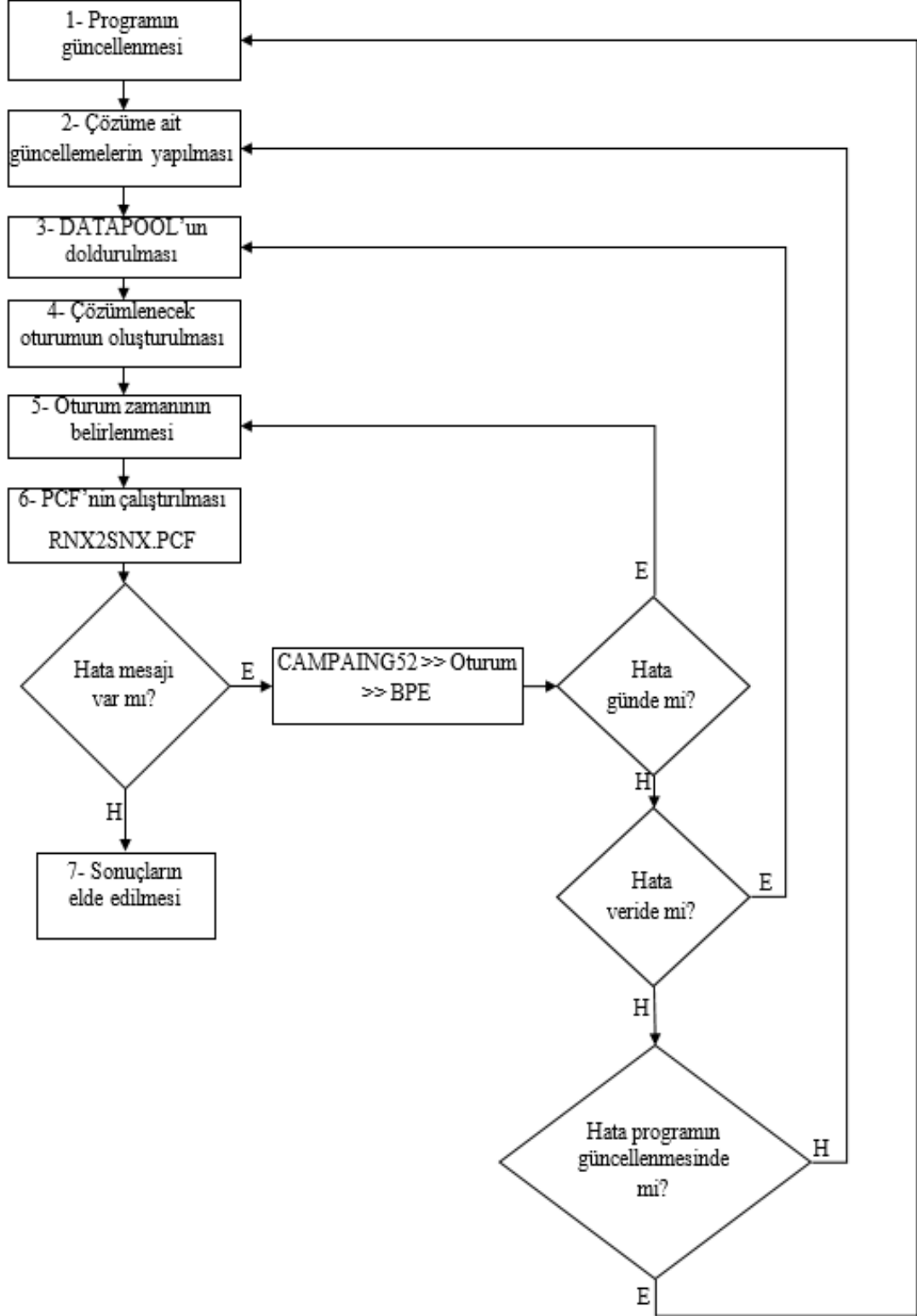
Şekil 6.15 RNX2SNX.PCF iş akış diyagramı
