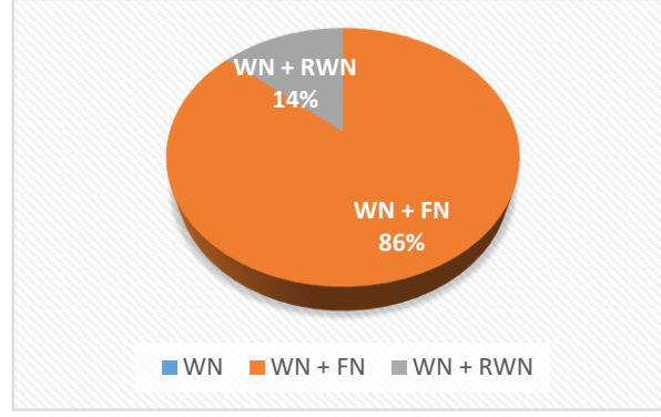
Şekil 6.22 Düşey koordinat bileşeni gürültü dağılımı
