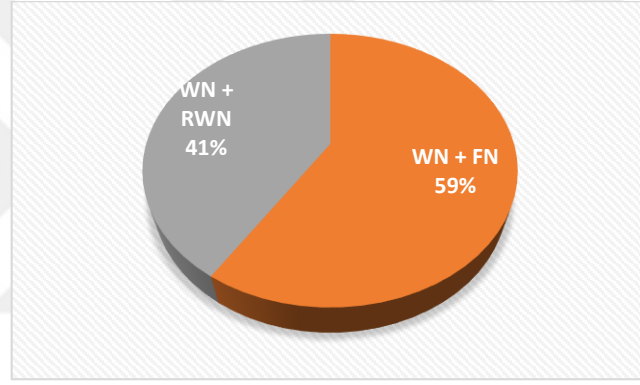
Şekil 6.20 Kuzey bileşeni gürültü dağılımı
