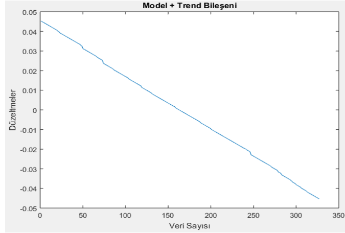
Şekil 6.24 ADAN istasyonu X koordinatı için Trend ‘in gösterimi
