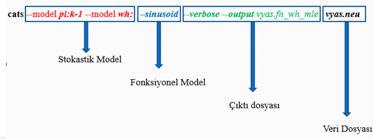
Şekil 4.3 CATS yazılımı çalışma prensibi
