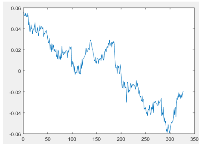
Şekil 6.26 ADAN istasyonu X koordinatı için Gürültü + Trend ‘in gösterimi
