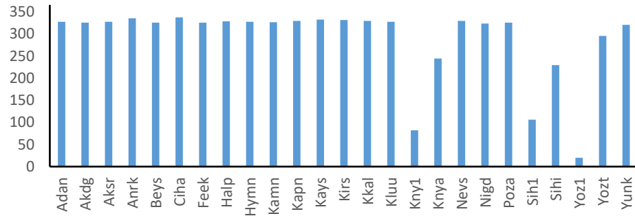
Şekil 6.5 TUSAGA-Aktif istasyonları veri uzunluğu
