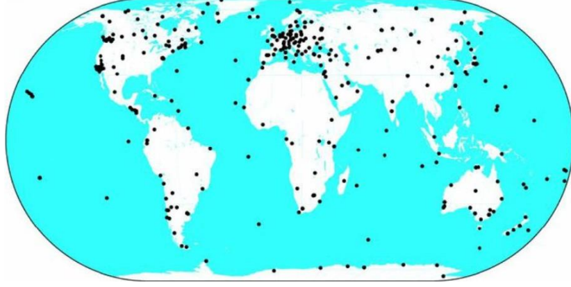
Şekil 2.1. IGS istasyonlarının dağılımı
