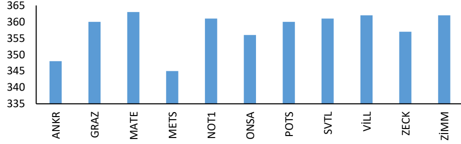
Şekil 6.4 IGS istasyonları veri uzunluğu
