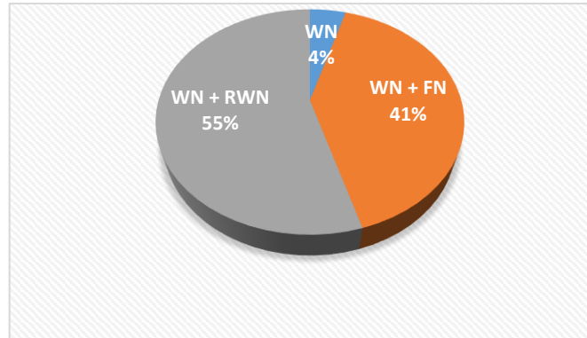
Şekil 6.21 Doğu bileşeni gürültü dağılımı
