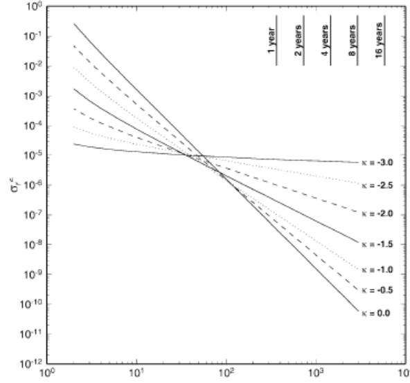
Şekil 4.1 Veri sayısı ve gürültü modeli ilişkisi
