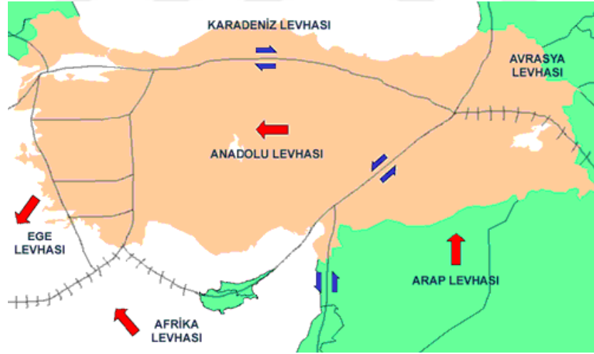
Şekil 3.1 Türkiye'nin üzerinde bulunduğu tektonik plakalar ve hareketleri
