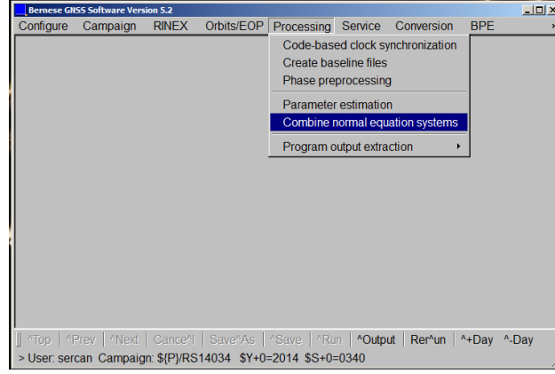
Şekil 5.13. Hız kestirimi ADDNEQ2
