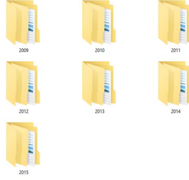
Şekil 6.14 Yıllık olarak temin edilen verilerin gösterimi
