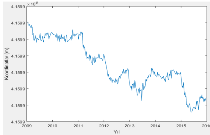
Şekil 6.23 ADAN istasyonu X koordinatının seriye açılması
