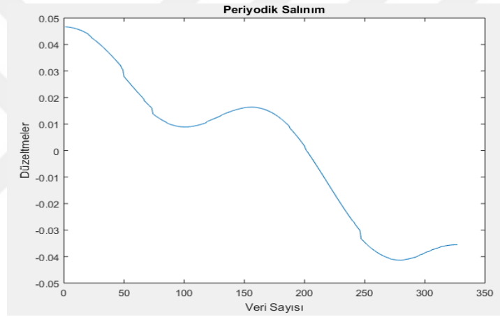
Şekil 6.25 ADAN istasyonu X koordinatı için periyodik etkinin gösterimi
