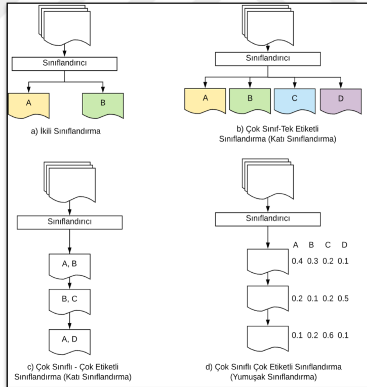
Şekil 1.3. Sınıflandırma Türleri
