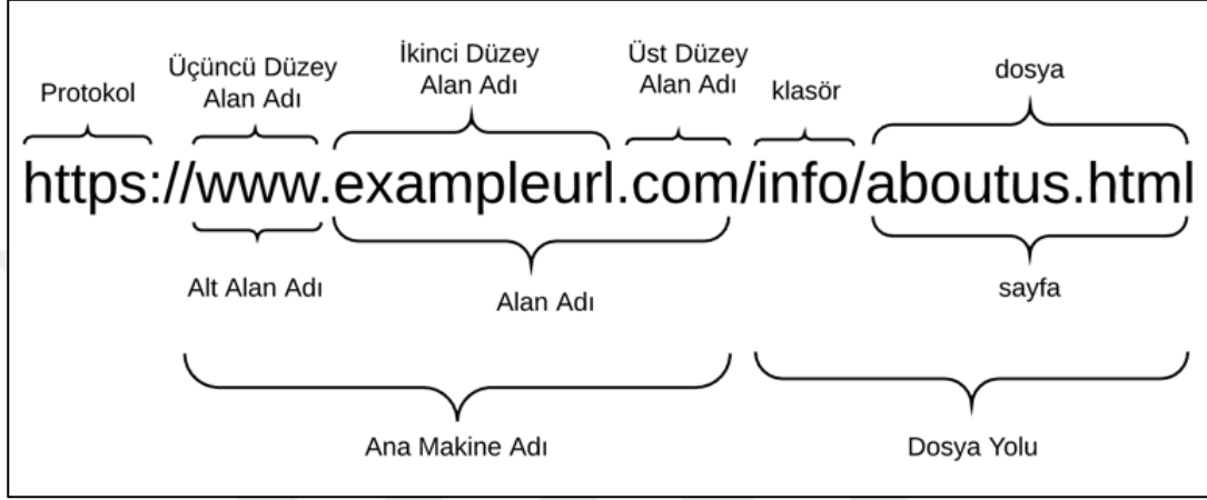
Şekil 1.6. URL Bileşenleri
