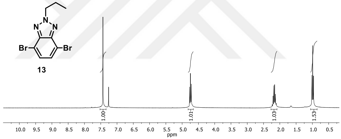
EK 26: 13 bileşığının 1 H NMR (300 MHz, CDCl 3 ) spektrumu
