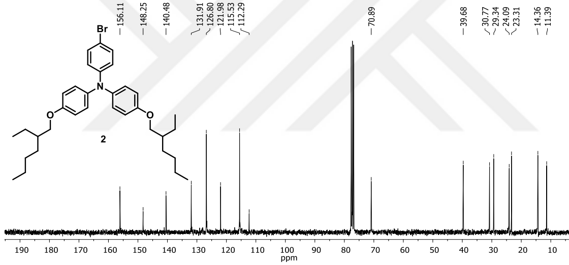
EK 4: 2 bileşğinin 13 C NMR (75 MHz, CDCl 3 ) spektrumu
