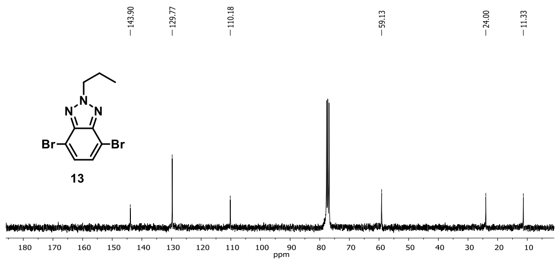
EK 27: 13 bileşiğinin 13 C NMR (75 MHz, CDCl 3 ) spektrumu
