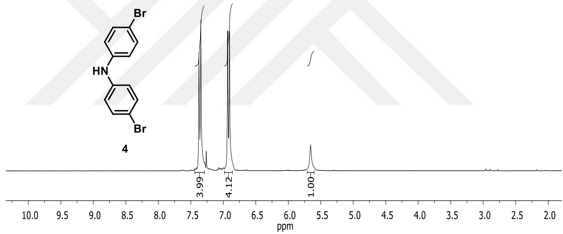
EK 6: 4 bileşığının 1 H NMR spektrumu (300 MHz, CDCl 3 )
