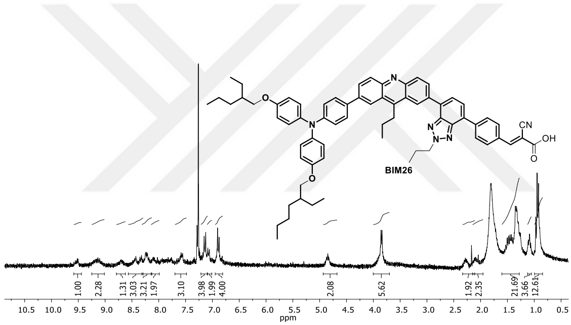
EK 44: BIM26 bileşığının ^1\text{H} NMR spektrumu (300 MHz, \text{CDCl}_3 )
