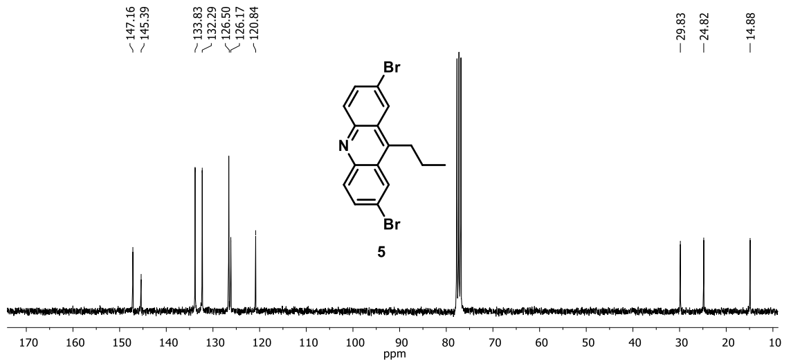
EK 9: 5 bileşiğinin 13 C NMR (75 MHz, CDCl 3 ) spektrumu
