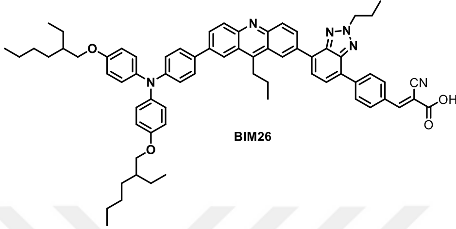
Şekil 3.19. 3-(4-(7-(7-(4-(bis(4-((2-etilhekzil)oksi)fenil)amino)fenil)-9-propilakridin-2-il)-2-propil-2H-benzo[d][1,2,3]triazol-4-il)fenil)- 2-siyanoakrilik asit (BIM26) bileşığının sentezi
