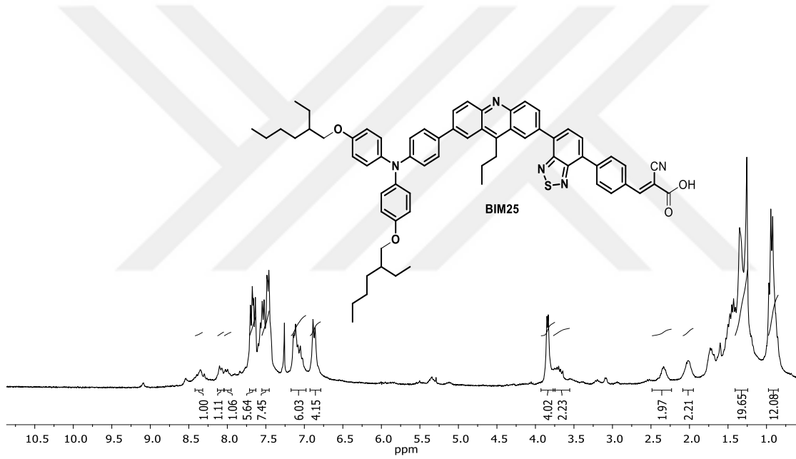
EK 40: BIM25 bileşığının ^1\text{H} NMR spektrumu (300 MHz, \text{CDCl}_3 )
