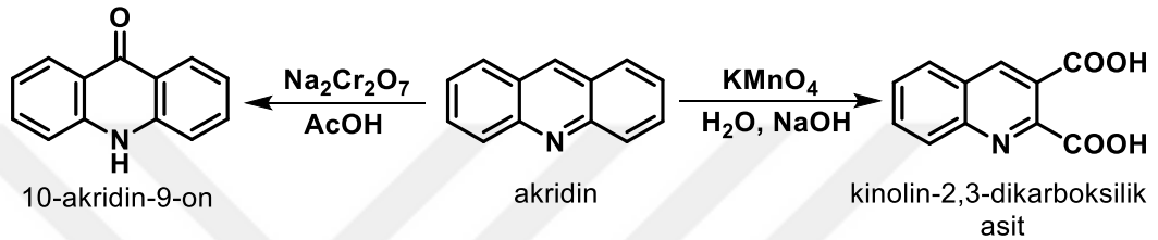
Şekil 2.9. Akridinin yükseltgenmesi
