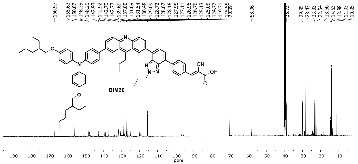
EK 45: BIM26 bileşiğinin ^{13}\text{C} NMR (176 MHz, DMSO-d 6 ) spektrumu
