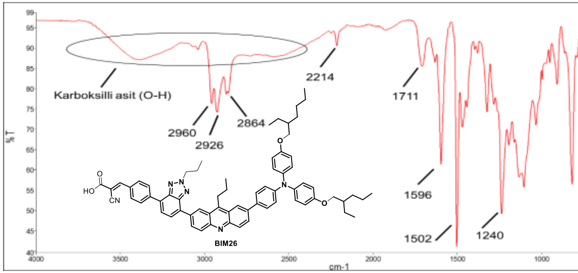
EK 43: BIM26 bileşığının FT-IR spektrumu ( \text{cm}^{-1} )
