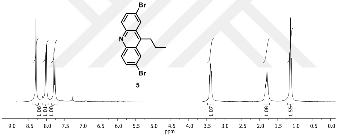
EK 8: 5 bileşğinin 1 H NMR spektrumu (300 MHz, CDCl 3 )
