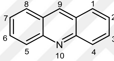
Şekil 2.1. Akridinin yapısı
