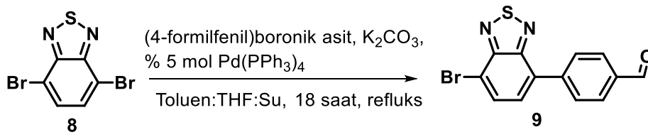
Şekil 3.9. 4-(7-bromobenzo[c][1,2,5]tiyadiazol-4-il)benzaldehit (9) bileşiğinin sentezi
