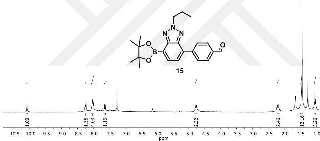
EK 32: 15 bileşiğinin ^1\text{H} NMR spektrumu (300 MHz, \text{CDCl}_3 )
