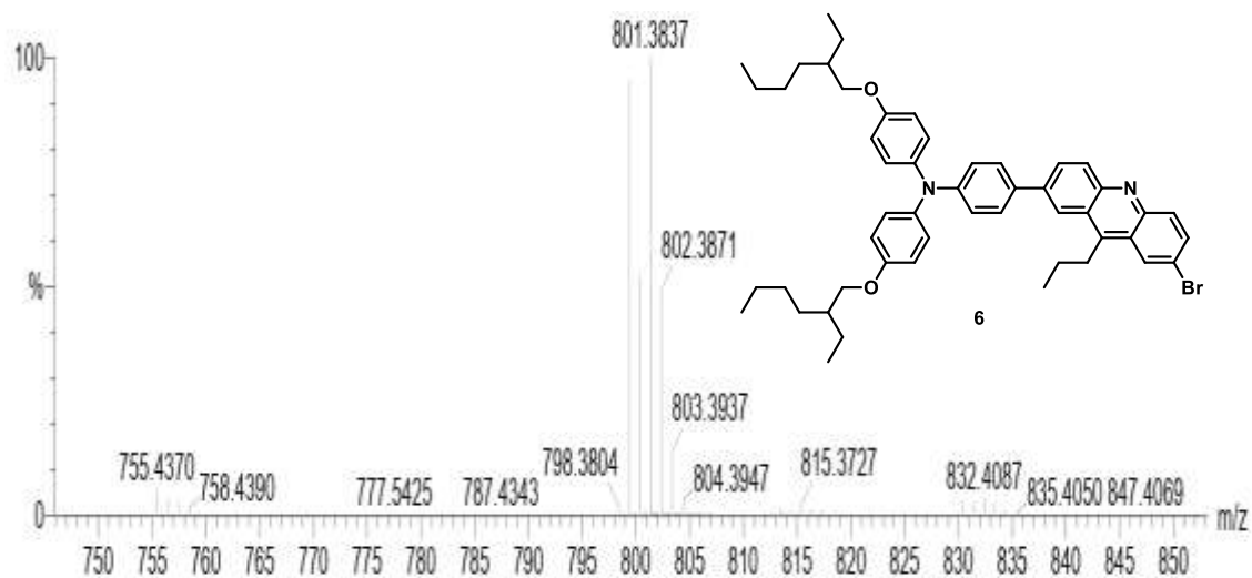
EK 13: 6 bileşığının HRMS-ESI(+) spektrumu
