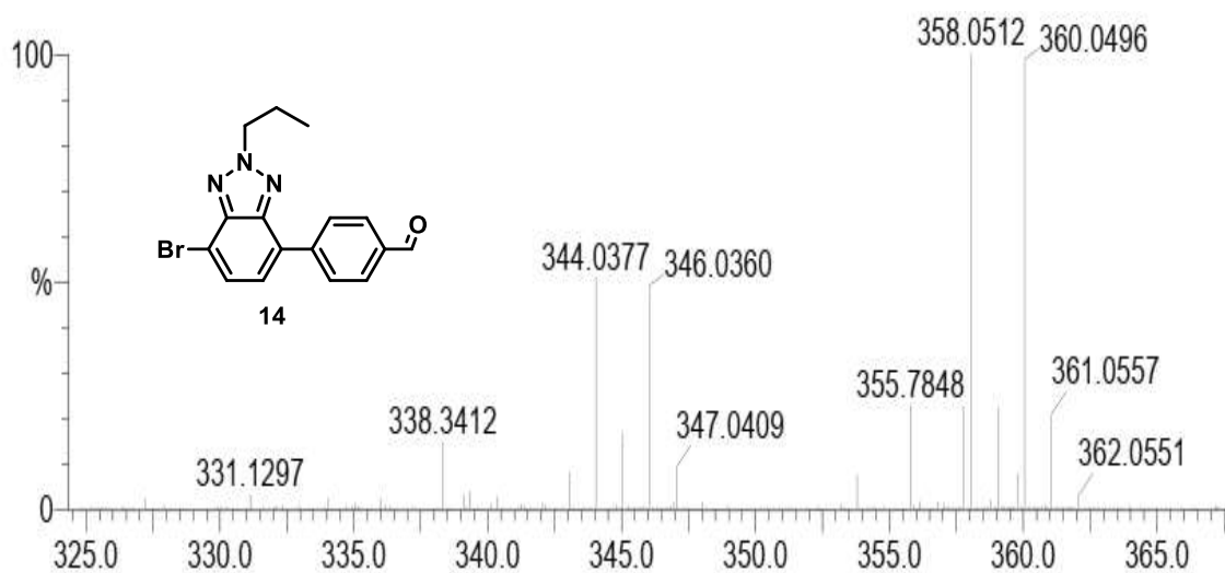
EK 31: 14 bileşiğinin HRMS-ESI(+) spektrumu
