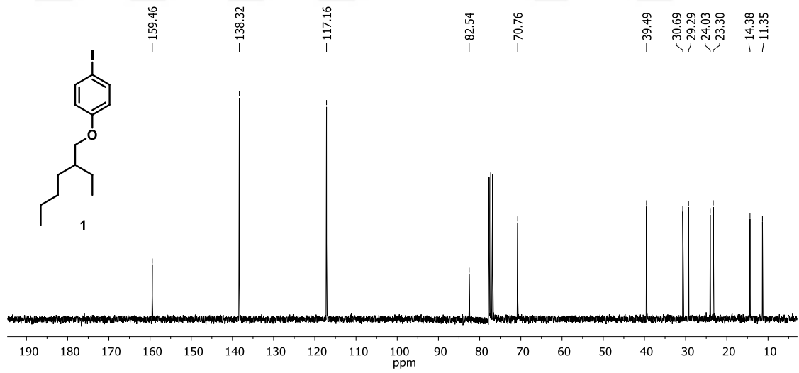
EK 2: 1 bileşığının 13 C NMR spektrumu (75 MHz, CDCl 3 )
