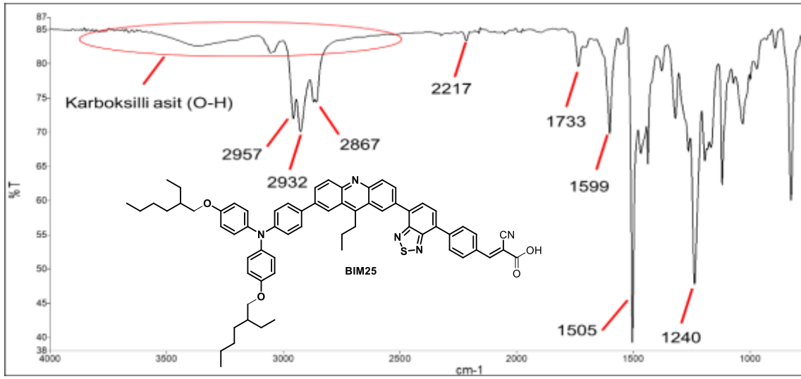
EK 39: BIM25 bileşığının FT-IR spektrumu ( \text{cm}^{-1} )
