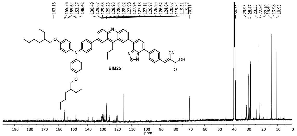
EK 41: BIM25 bileşiğinin ^{13}\text{C} NMR (176 MHz, DMSO- d_6 ) spektrumu
