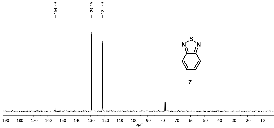
EK 15: 7 bileşiğinin ^{13}\text{C} NMR (75 MHz, \text{CDCl}_3 ) spektrumu
