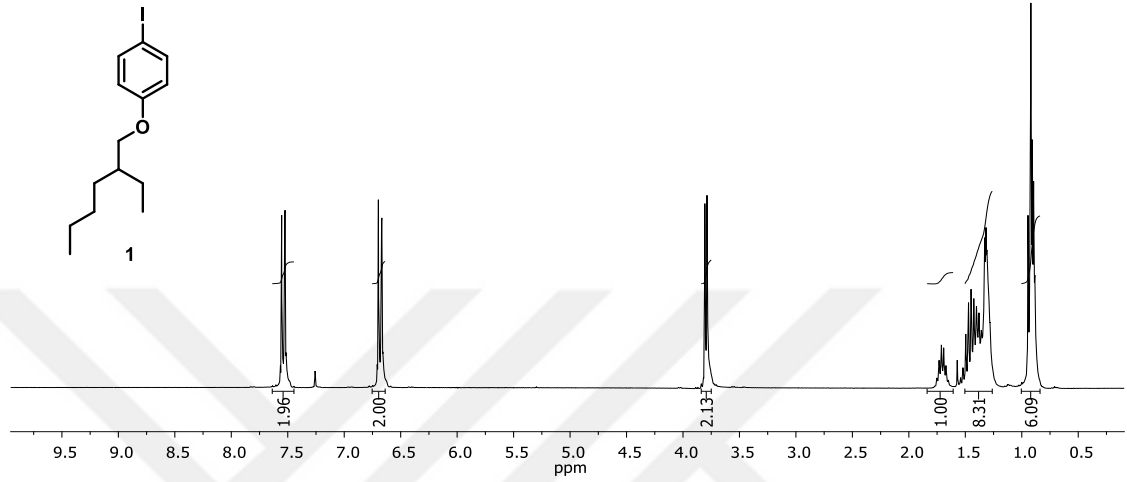
EK 1: 1 bileşığının 1 H NMR spektrumu (300 MHz, CDCl 3 )
