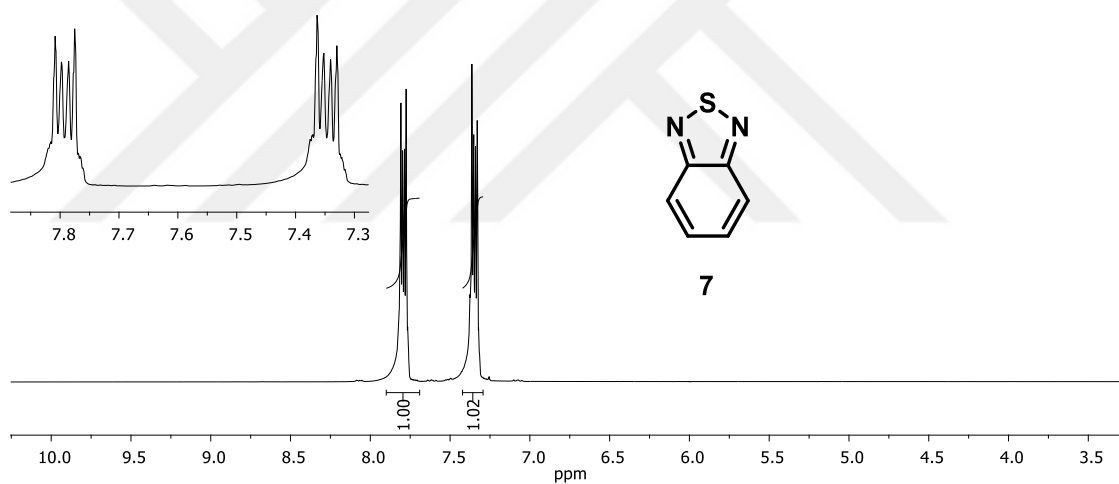
EK 14: 7 bileşığının 1 H NMR spektrumu (300 MHz, CDCl 3 )
