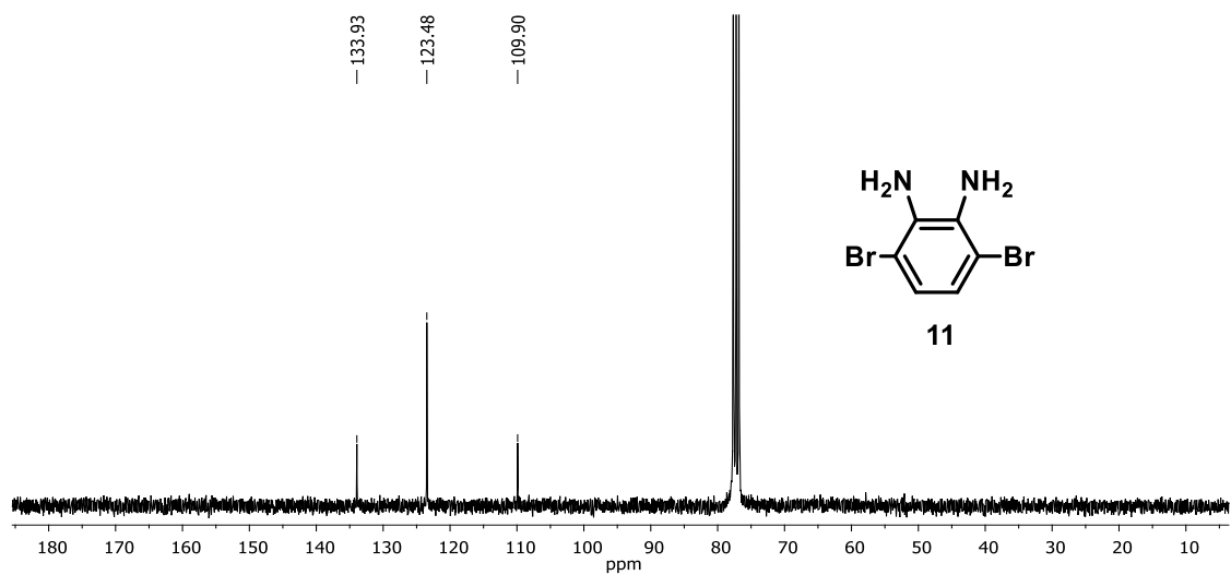
EK 23: 11 bileşiğinin ^{13}\text{C} NMR (75 MHz, \text{CDCl}_3 ) spektrumu
