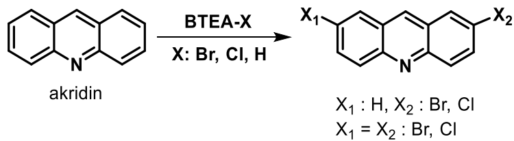
Şekil 2.10. Akridinin halojenlenmesi
