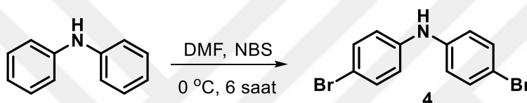
Şekil 3.4. bis(4-bromofenil)amin (4) bileşiğinin sentezi
