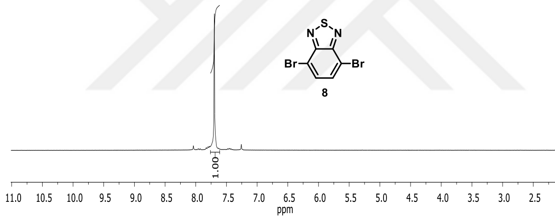
EK 16: 8 bileşiğinin ^1\text{H} NMR (300 MHz, \text{CDCl}_3 ) spektrumu
