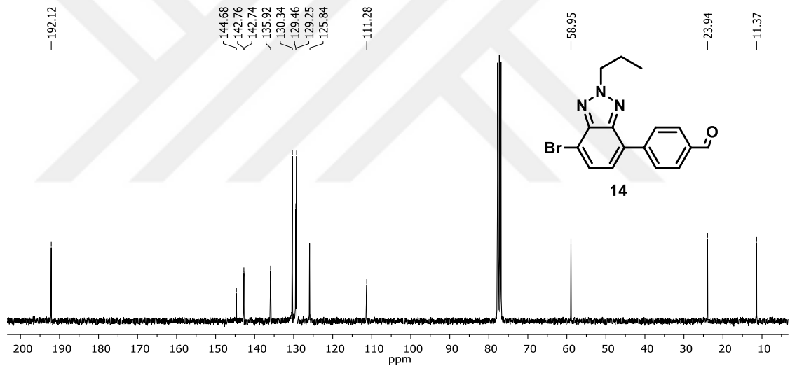
EK 30: 14 bileşığının 13 C NMR (75 MHz, CDCl 3 ) spektrumu
