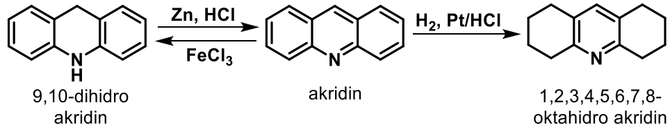
Şekil 2.8. Akridinin indirgenmesi
