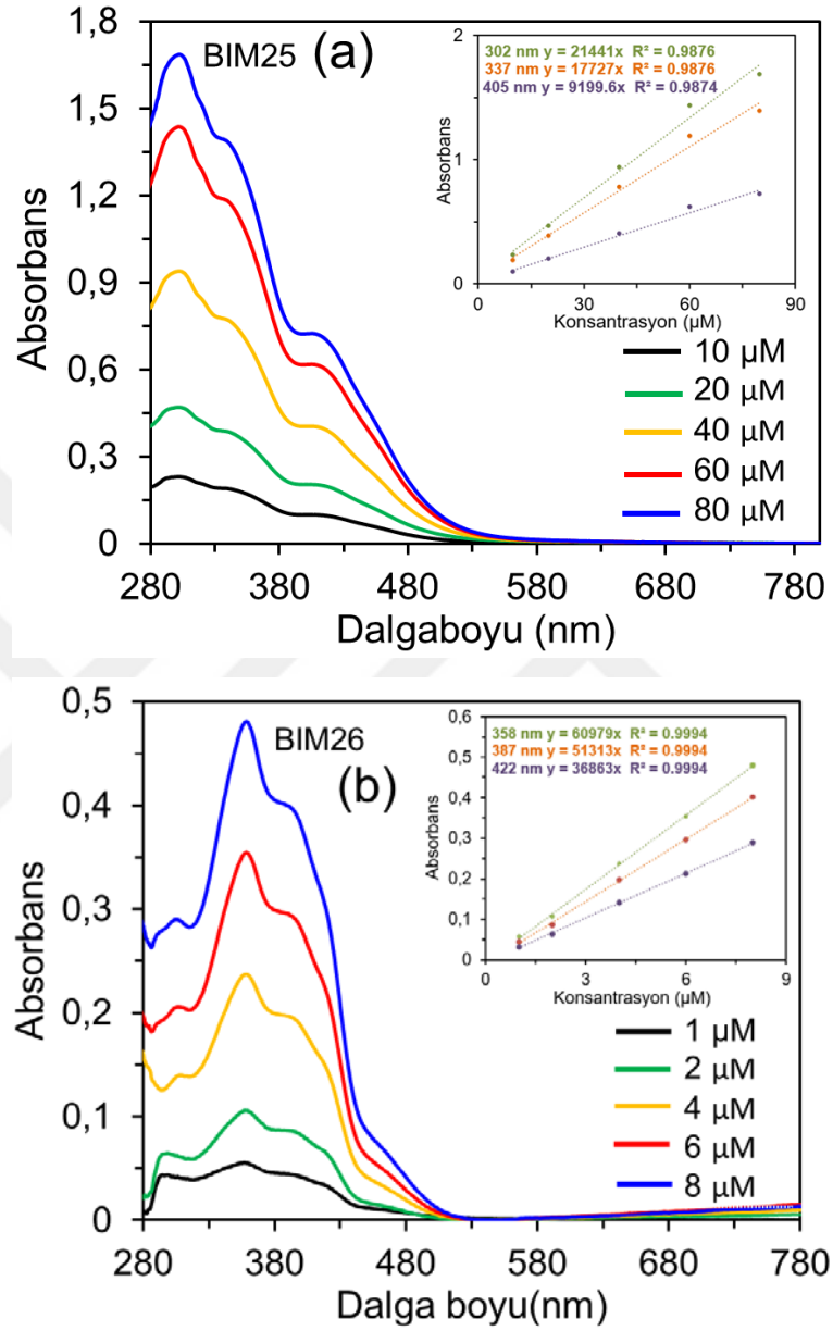
Şekil 4.3. Çeşitli konsantrasyonlarda THF içinde BIM25 ve BIM26 boyaalarının absorpsiyon spektrumları. Grafik içindeki kısım, konsantrasyona karşı absorpsiyon grafiklerini gösterir.
