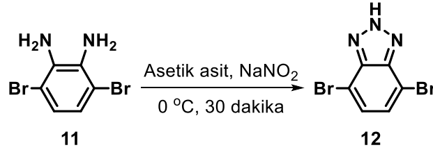
Şekil 3.12. 4,7-dibromo-2H-benzo[d][1,2,3]triazol ( 12 ) bileşiğinin sentezi
