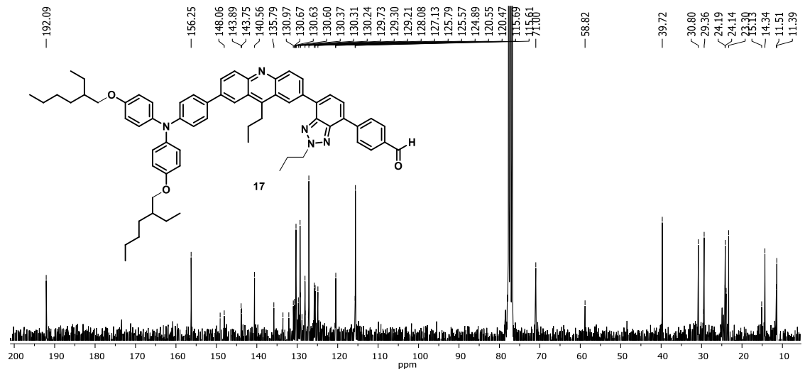
EK 37: 17 bileşiğinin ^{13}\text{C} NMR (75 MHz, \text{CDCl}_3 ) spektrumu
