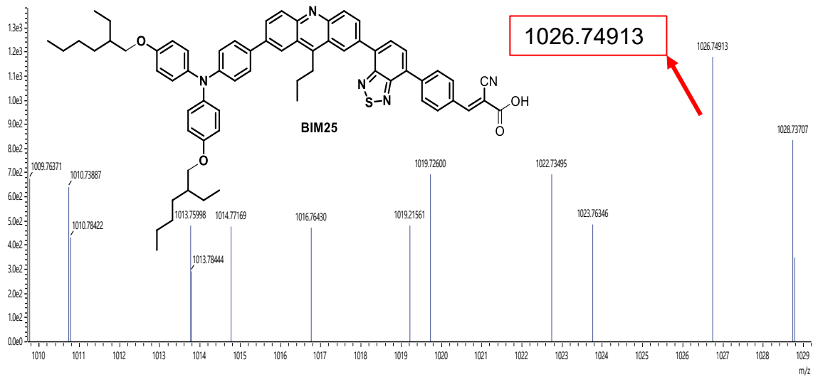
EK 42: BIM25 bileşiğinin bileşiğinin LC-MS spektrumu
