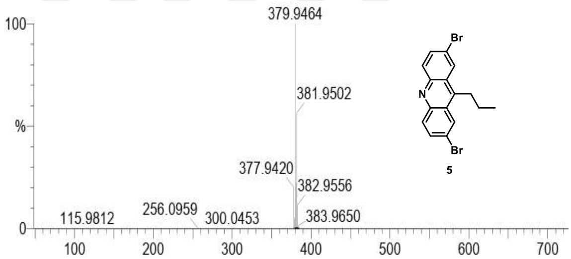
EK 10: 5 bileşiğinin HRMS-ESI(+) spektrumu
