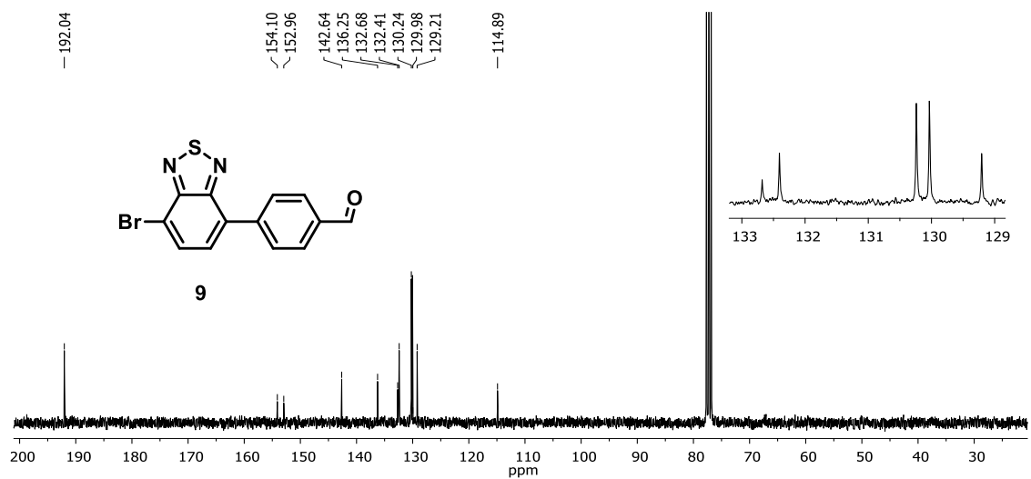
EK 19: 9 bileşiğinin 13 C NMR (75 MHz, CDCl 3 ) spektrumu
