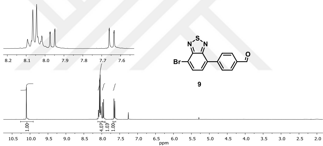
EK 18: 9 bileşığının ^1\text{H} NMR (300 MHz, \text{CDCl}_3 ) spektrumu
