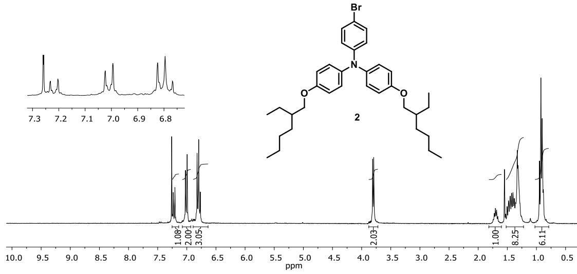
EK 3: 2 bileşğinin 1 H NMR spektrumu (300 MHz, CDCl 3 )
