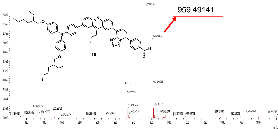
EK 35: 16 bileşiminin bileşiminin LC-MS spektrumu
