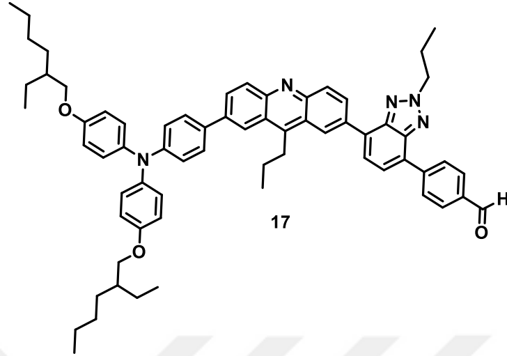
Şekil 3.17. 4-(7-(7-(4-(bis(4-((2-etilhekzil)oksi)fenil)amino)fenil)-9-propilakridin-2-il)-2-propil-2H-benzo[d][1,2,3]triazol-4-il)benzaldehit (17) bileşığının sentezi
