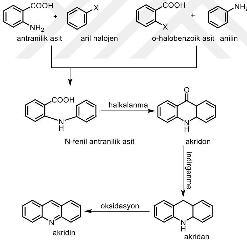
Şekil 2.2. Ullman sentezi
