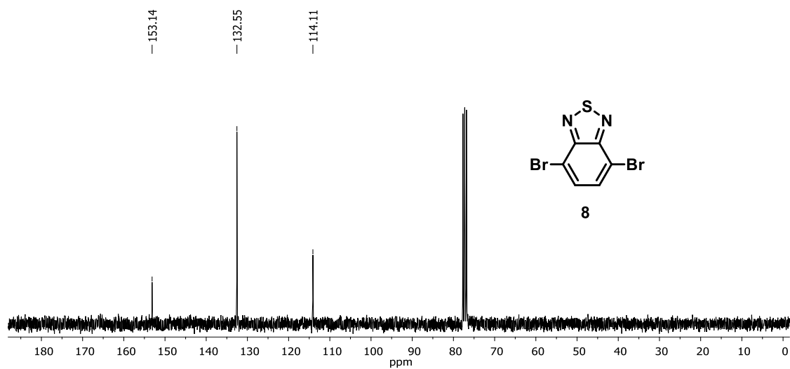
EK 17: 8 bileşığının ^{13}\text{C} NMR (75 MHz, \text{CDCl}_3 ) spektrumu
