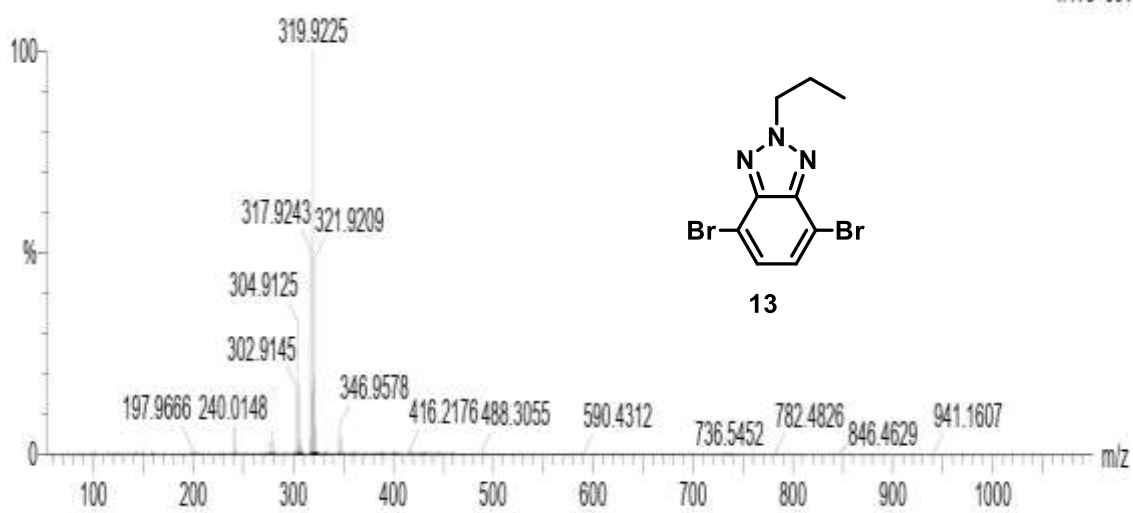
EK 28: 13 bileşiğinin HRMS-ESI(+) spektrumu
