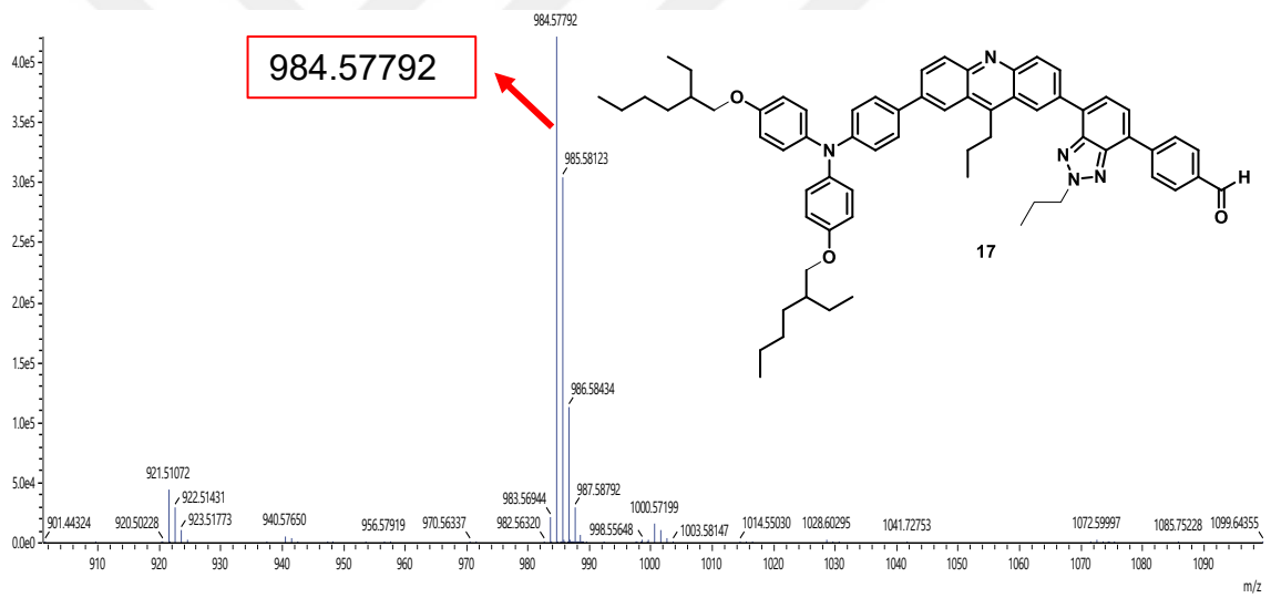
EK 38: 17 bileşiğinin bileşiğinin LC-MS spektrumu
