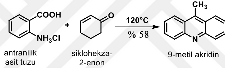
Şekil 2.4. Friedlander sentezi
