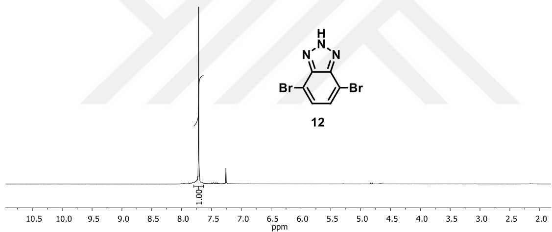
EK 24: 12 bileşiğinin ^1\text{H} NMR spektrumu (300 MHz, \text{CDCl}_3 )
