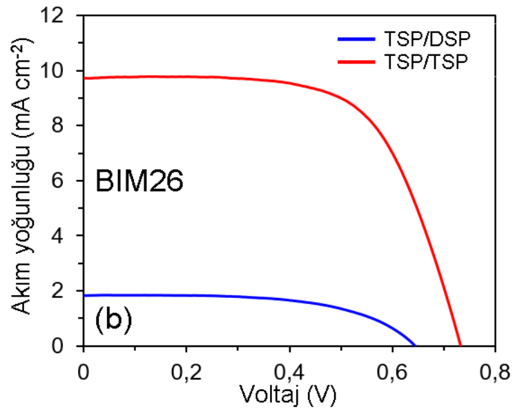
Şekil 4.6. TSP/TSP ve TSP/DSP TiO 2 fotoanotlarında hassaslaştırılmış BIM25 (a) ve BIM26 (b) boyalarının akım-voltaj grafikleri.
