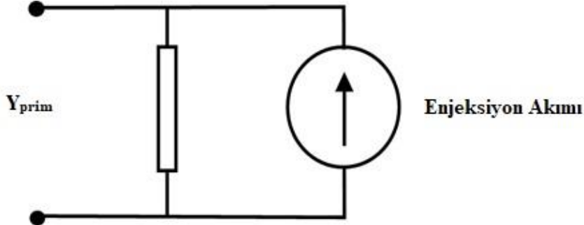
Şekil 3.1. Güç dönüşüm elemanlarının Enjeksiyon Akım Modeli [30].
