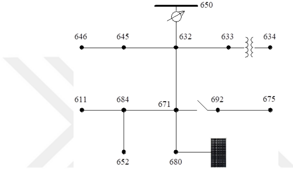
Şekil 2.2. Modifiye edilmiş IEEE 13 baralı test fideri [59].
