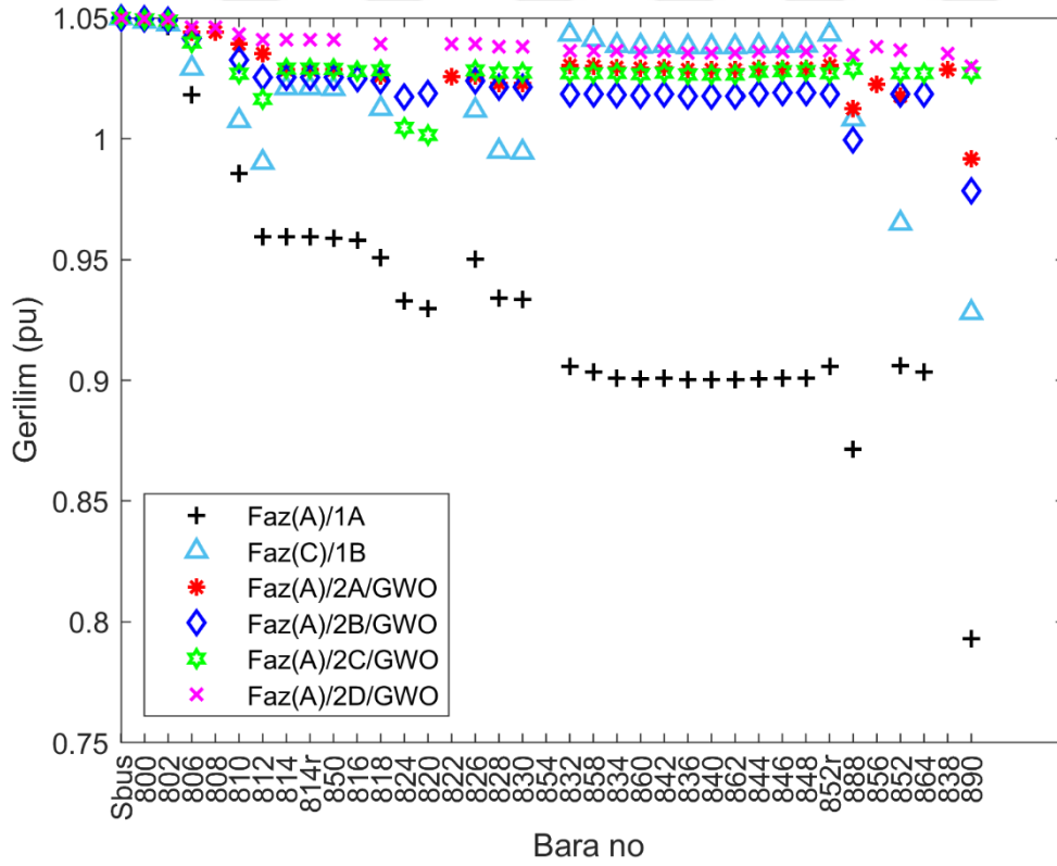
Şekil 5.2. Senaryo 1-GWO ve Senaryo 2-GWO için gerilim profili.
