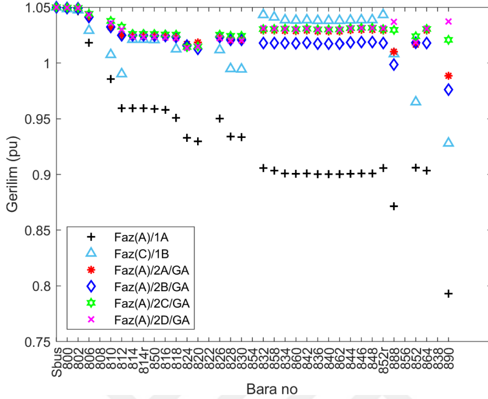
Şekil 5.1. Senaryo 1-GA ve Senaryo 2-GA için gerilim profili.
