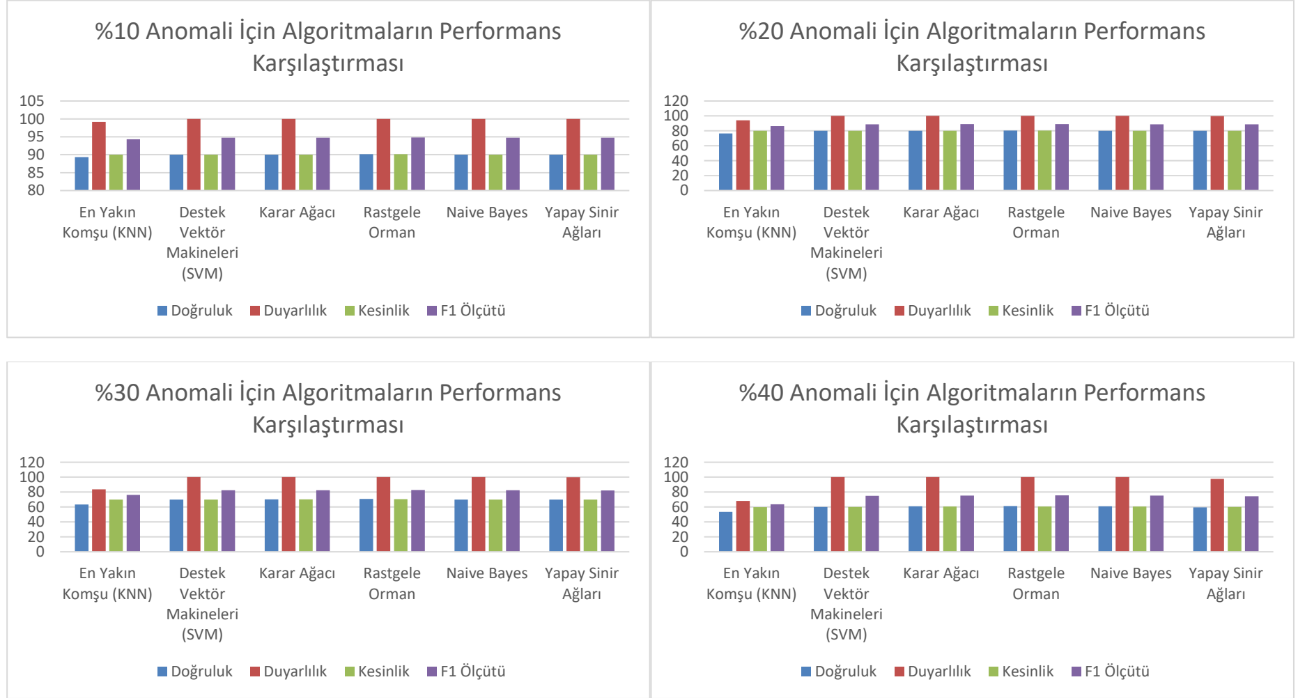
Şekil 4.4. Algoritmaların performans karşılaştırması.
