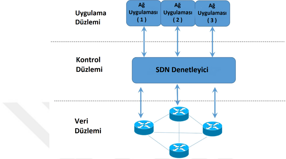
Şekil 2.3. Yazılım tanımlı ağ mimarisi.
