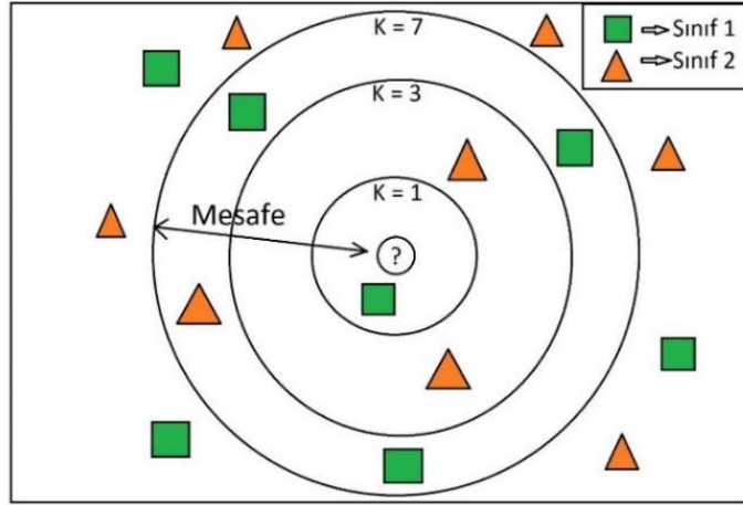
Şekil 4.1. En yakın komşu algoritması modeli [92].
