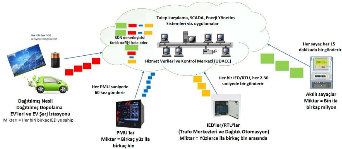
Şekil 2.4. Yazılım tanımlı akıllı şebeke mimarisi [1].
