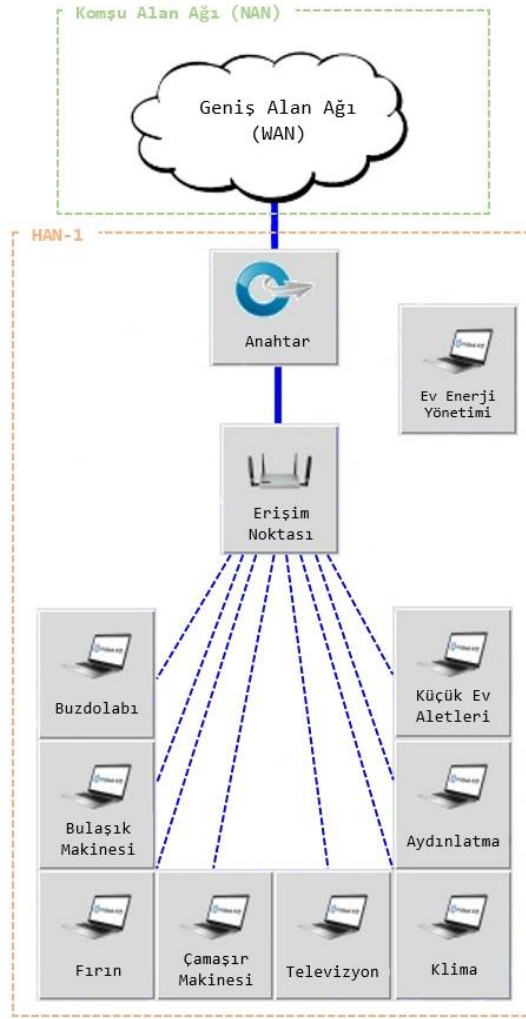
Şekil 3.2. Simülasyon ortamında oluşturulan akıllı ev topolojisi.
