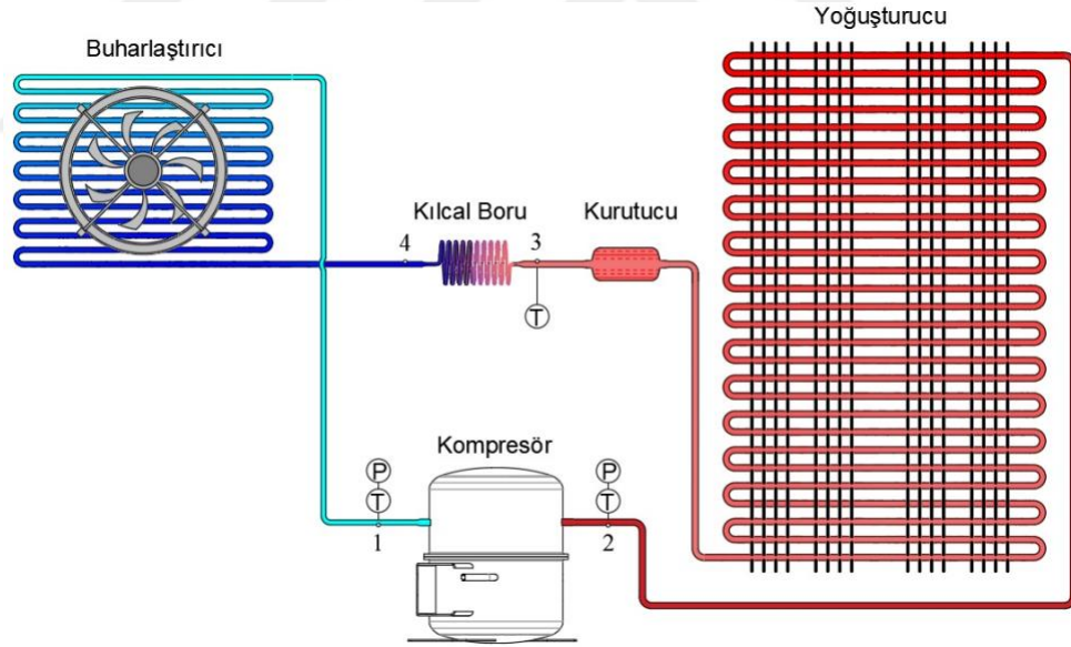
Şekil 3.1. Buhar sıkıştırırmalı soğutma çevriminin şematik görüntüsü [38].
