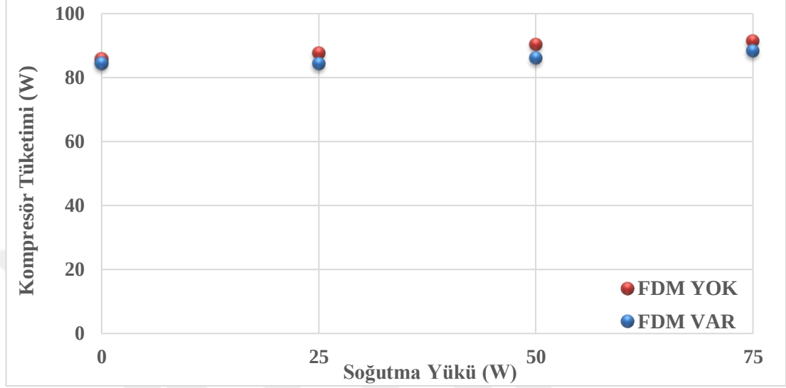
Şekil 4.3. FDM kullanılan ve kullanılmayan sistemlerin Kompresör Tüketimlerinin soğutma yüklerine bağlı değişimi.
