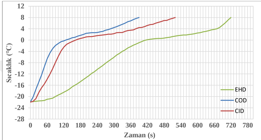
Şekil 4.11. FDM kullanılmayan defrost yöntemlerinin defrost sürelerine etkileri
