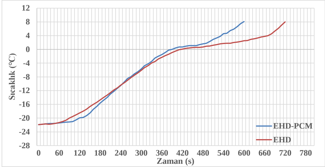
Şekil 4.10. Elektrikli ısıtıcılı FDM kullanılan ve kullanılmayan sistemlerde defrost sürelerinin zamana bağlı değişimi (Soğutma Yüğü: 0W)
