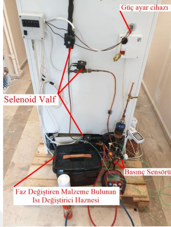
Şekil 3.5. Deney sistemi ve ölçüm elemanlarının yerleşimleri
