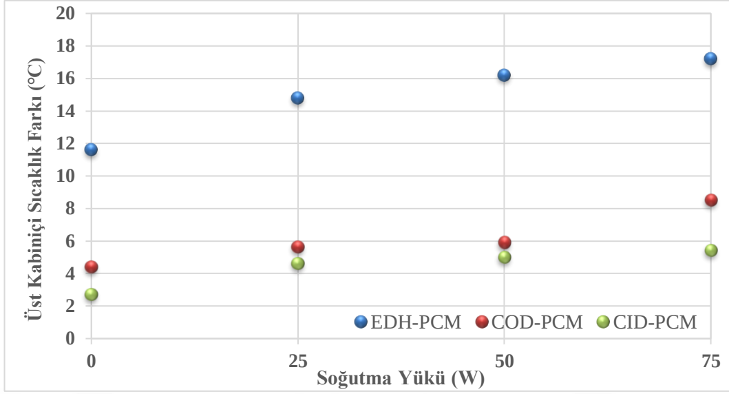
Şekil 4.19. FDM kullanılan soğutma sistemlerinde kabiniçi sıcaklık artışlarının soğutma yüküne bağlı değişimi
