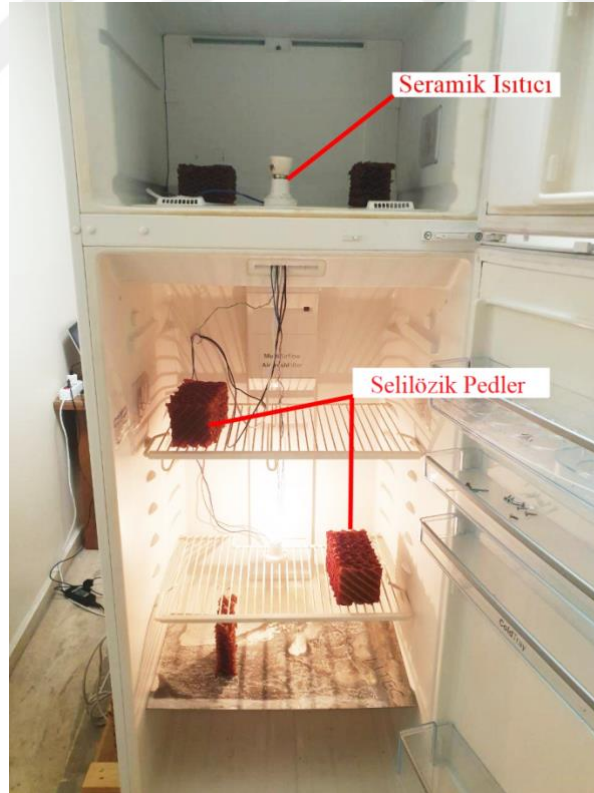
Şekil 3.6. Soğutma kabini içerisine yerleştirilen selilözik pedlerin görüntüsü
