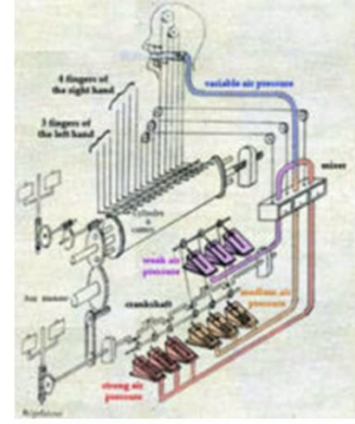
Vaucanson'un mekanik flütistinin çizimi
