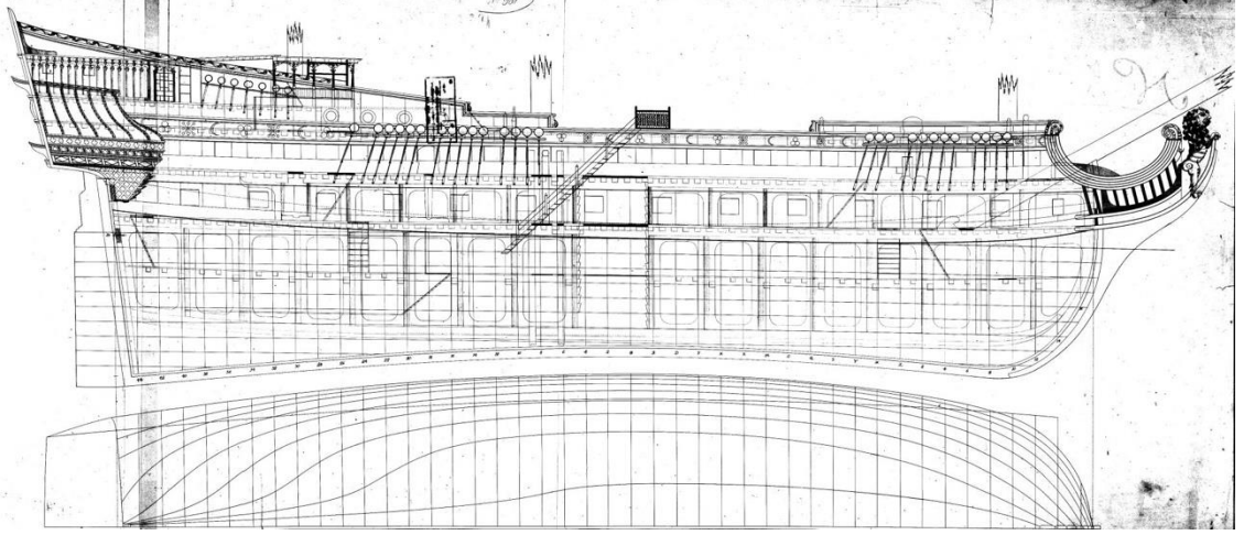
Görsel 8: Ruslar tarafından ele geçirildikten sonra Ioann Predtechka adını alan Peleng-i Bahri kalyonunun planı
