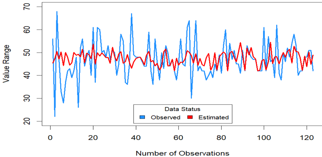
Şekil 3: RF yöntemi ile Aşıya Yönelik Tutumun Test Verileri Tahmini
