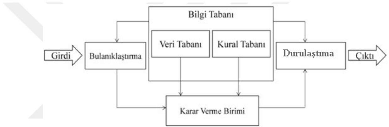
Şekil 7. Durulaştırma Sistemi
