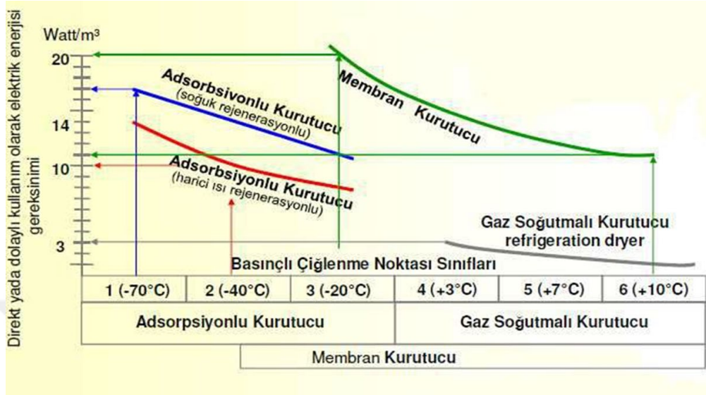
Şekil 13 Kurutucu Basınçlı Çiğlenme Noktası Sınıfları (Kanoğlu,2010)
