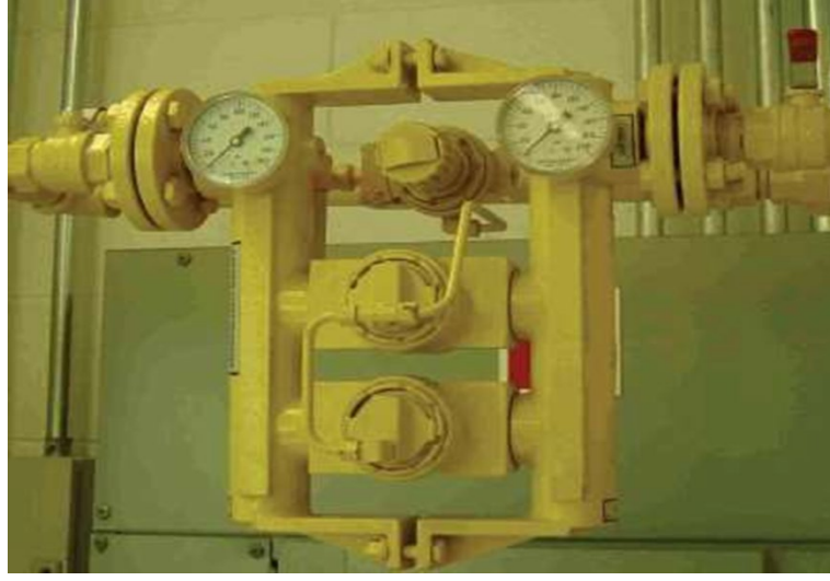
Şekil 18 Pnömatik Debi Kontrolörü
