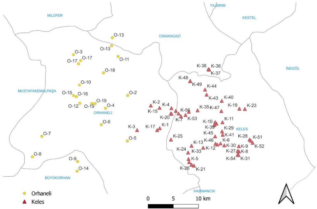
Şekil 3.3. Orhanlı ve Keleş ilçelerine ait örnekleme noktalarının yer aldığı harita.
