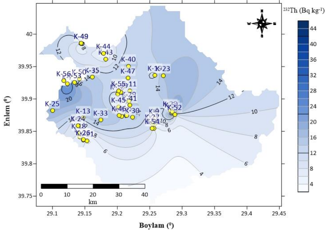
Şekil 4.2. Keleş ilçesi, çalışma bölgesindeki ^{232}\text{Th} spesifik aktivite dağılımı.
