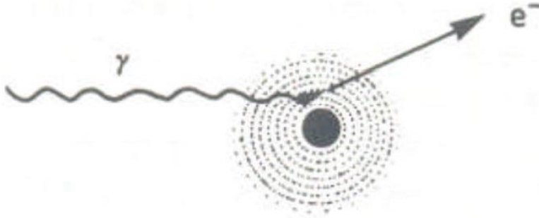
Şekil 2.7. Fotoelektrik olay [52].
