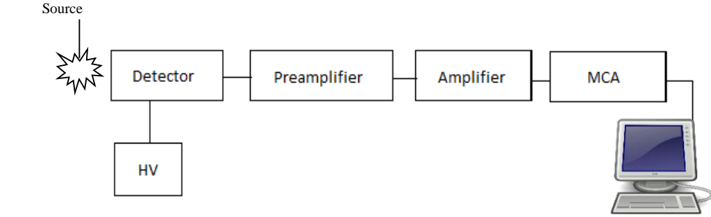
Şekil 3.5. Gama spektroskopisi sistemi genel şeması.
