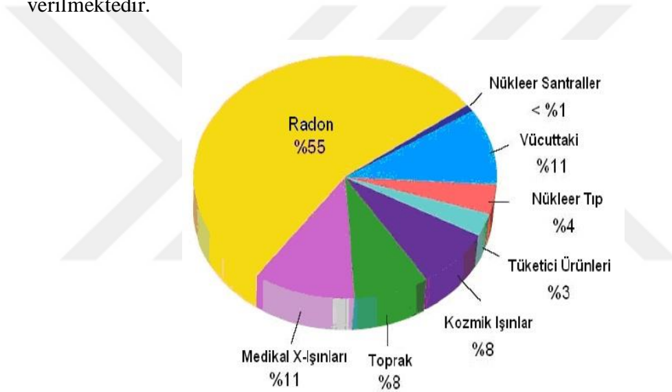
Şekil 2.1. Radyasyon kaynakları [36].
