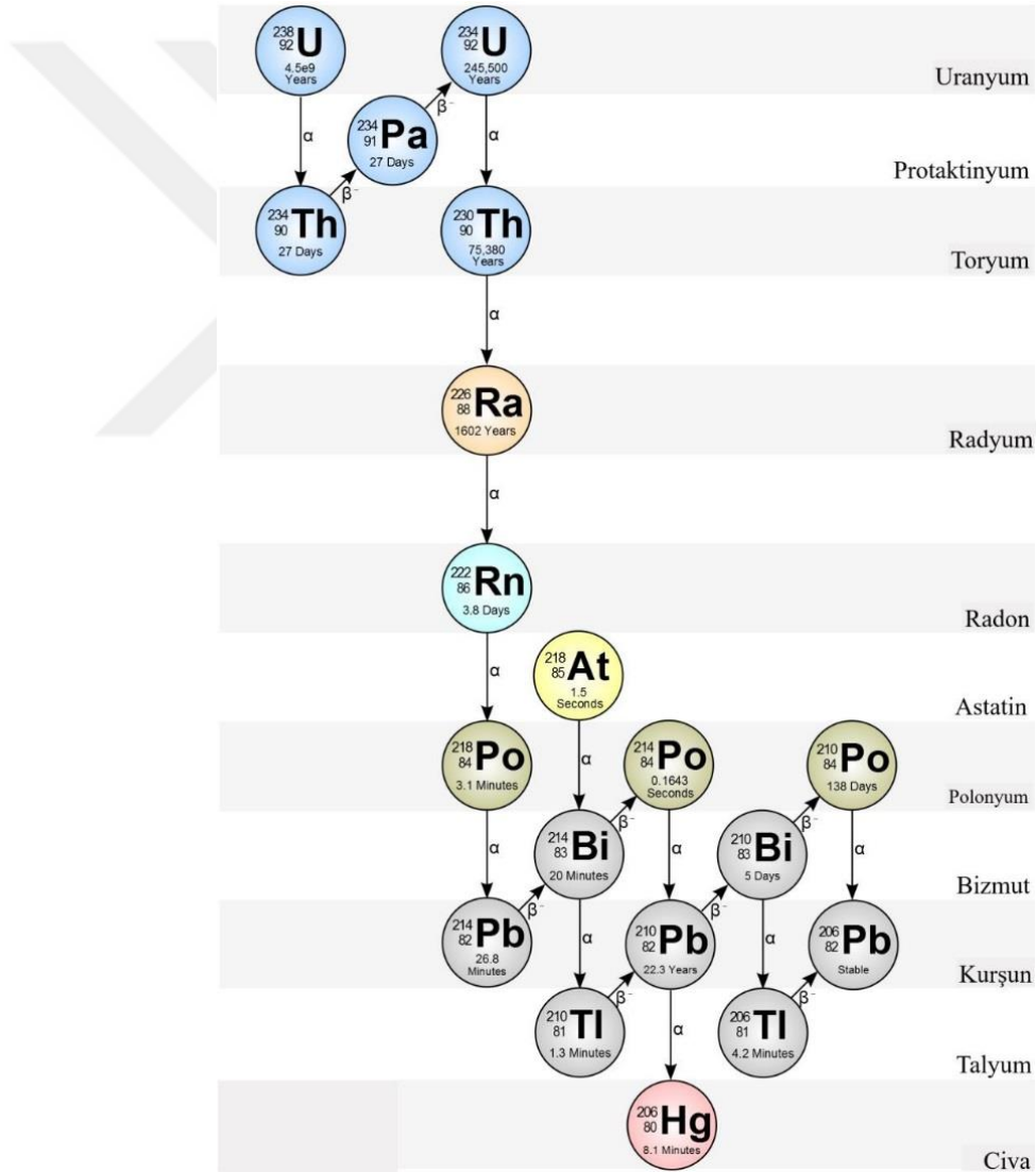
Şekil 2.2. ^{238}\text{U} bozunma serisi [44]
