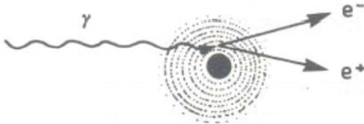
Şekil 2.9. Çift oluşumu [52].
