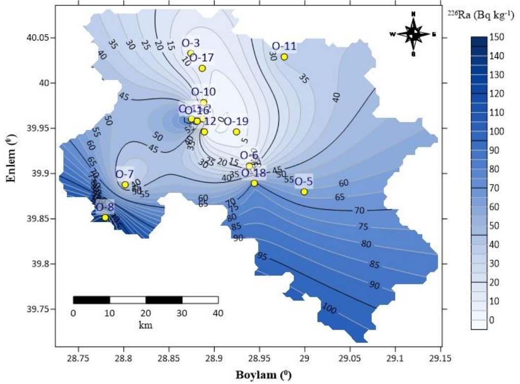
Şekil 4.4. Orhanlı ilçesi, çalışma bölgesindeki ^{226}\text{Ra} spesifik aktivite dağılımı.
