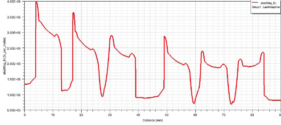
Şekil 7.45: Silindirik iki takoz ile yapılan deneyin Maxwell analizinde takoz üzerindeki elektrik alan değışimi grafiđi.
