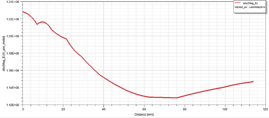
Şekil 7.36: Üç leplast takoz ile yapılan deneyin Maxwell analizinde takoz üzerindeki elektrik alan değışimi grafiđi.
