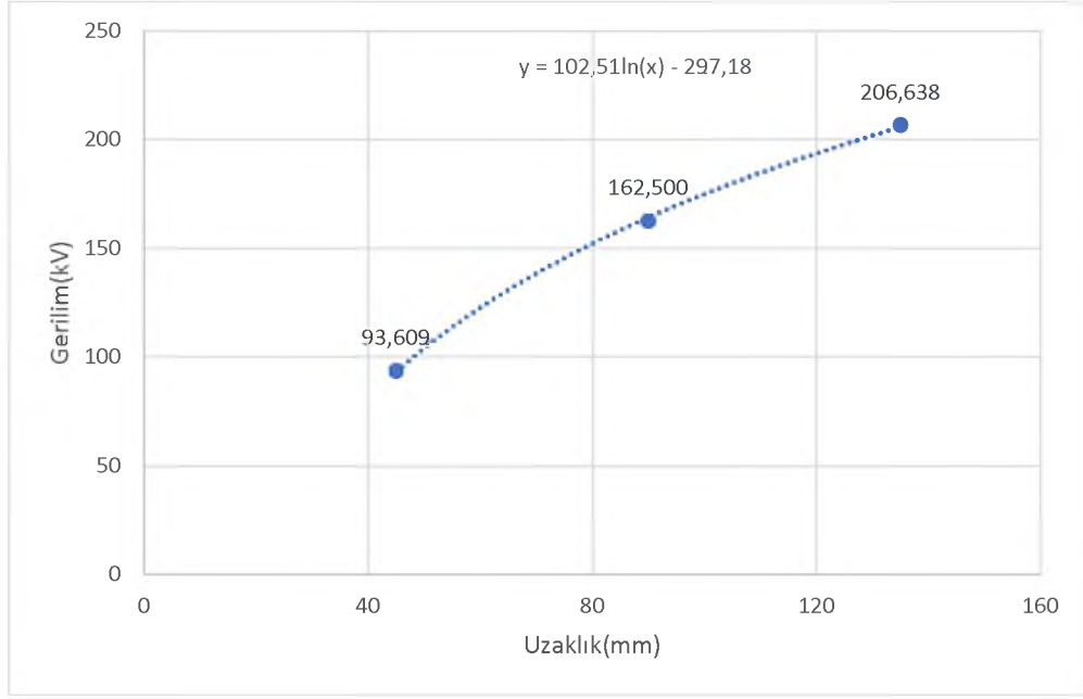
Şekil 7.51: Kuru hava ortamında silindirik takoz deney sonuçlarına göre oluşturulan grafik ve denklemi.
