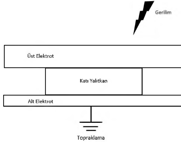
Şekil 7.4: Deney düzeneği basit modeli.
