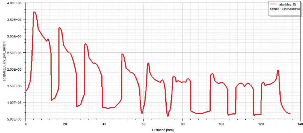
Şekil 7.49: Silindirik uç takoz ile yapılan deneyin Maxwell analizinde takoz üzerindeki elektrik alan değişimi grafiği.
