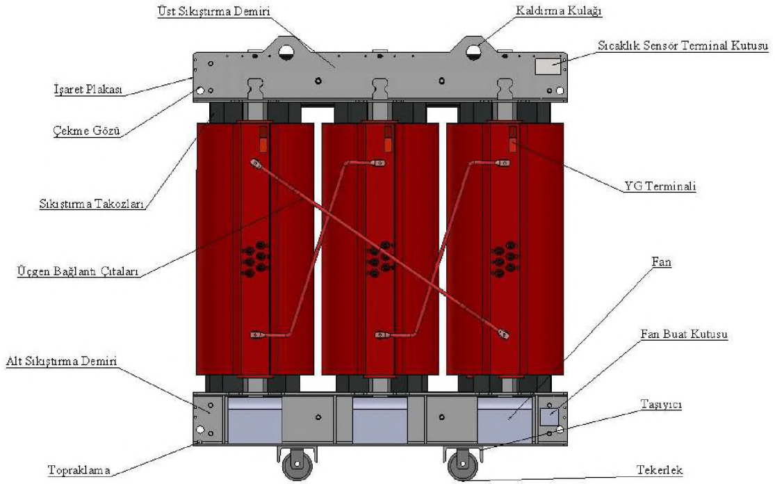
Şekil 3.1: Kuru tip transformatör önden genel görünüş.
