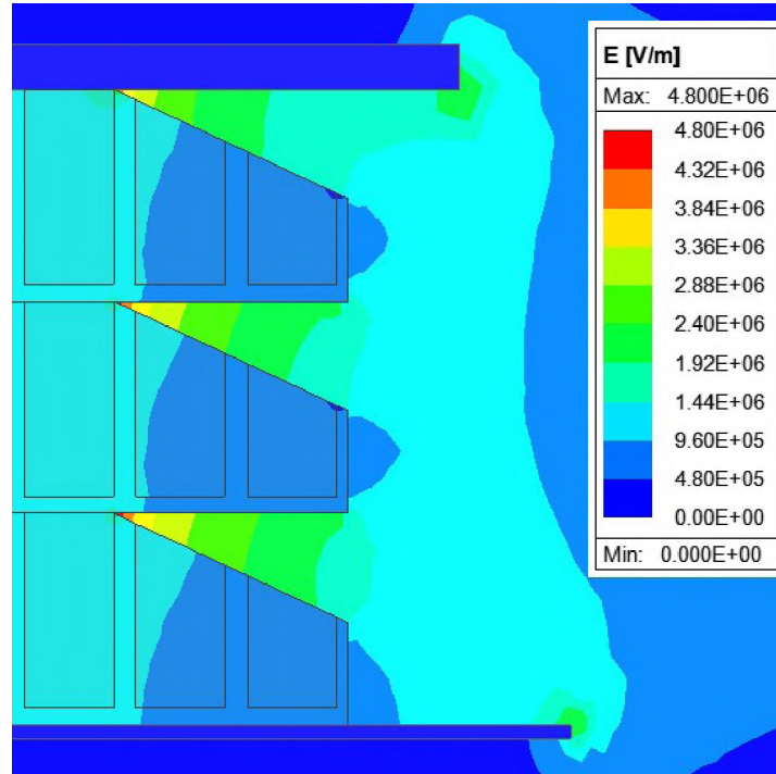
Şekil 7.37: Takozun gerilim verilen elektroda yakın olduđu dar alan ve takozlar arası dar alanlar.
