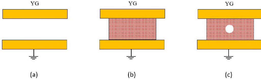
Şekil 6.4: Kısmi deşarj tipi modelleri (a) Korona deşarjı, (b) Yüzey deşarjı, (c) Dahili(iç) deşarj [9].
