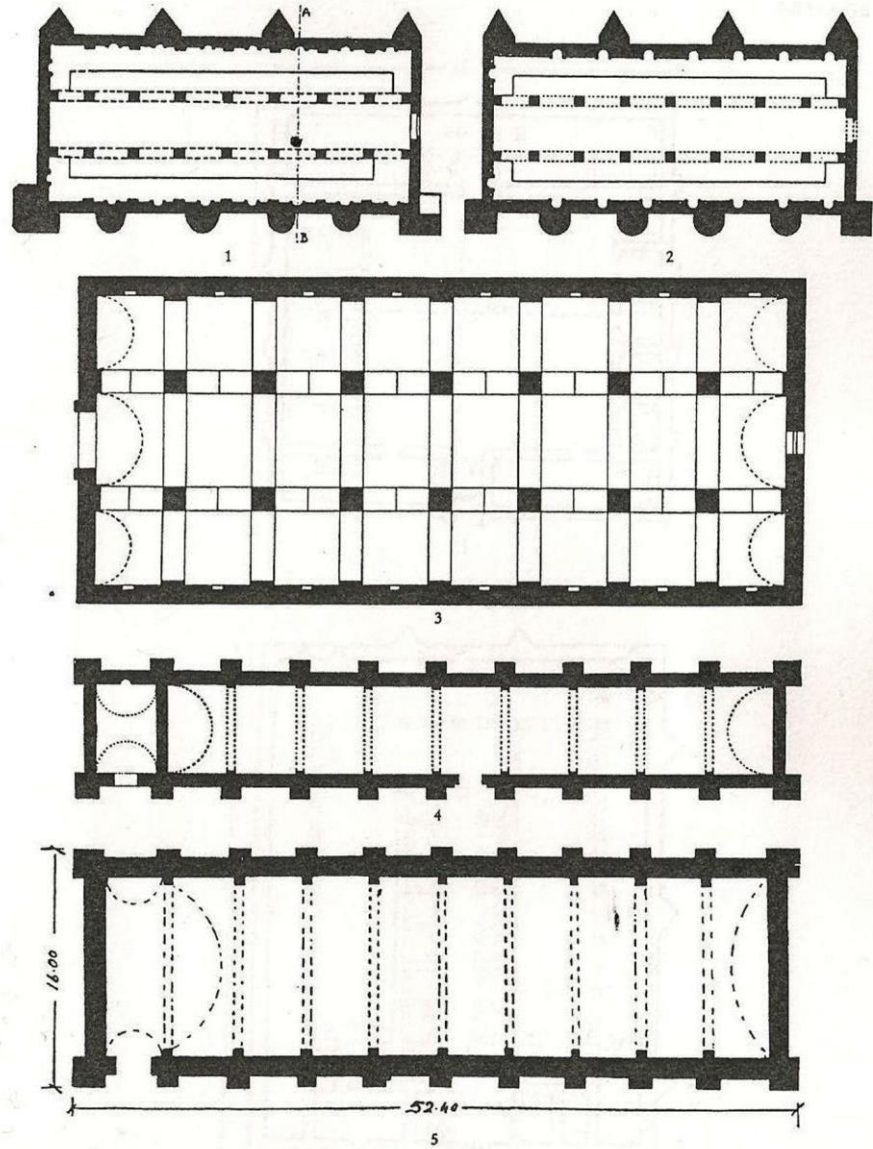
fig. 1 Ezinepazar Han (No. 45), Jerphanion 1928 nach Riondel — fig. 2 Ezinepazar Han (No. 45), nach Gabriel 1934 — fig. 3 Ezinepazar Han (No. 45), nach Riefstahl , unveröffentlicht, 1926 — fig. 4 Sarafşa Han (No. 53), nach Riefstahl 1931 — fig. 5 Sarafşa Han (No. 53), nach Fikri Erten 1940
