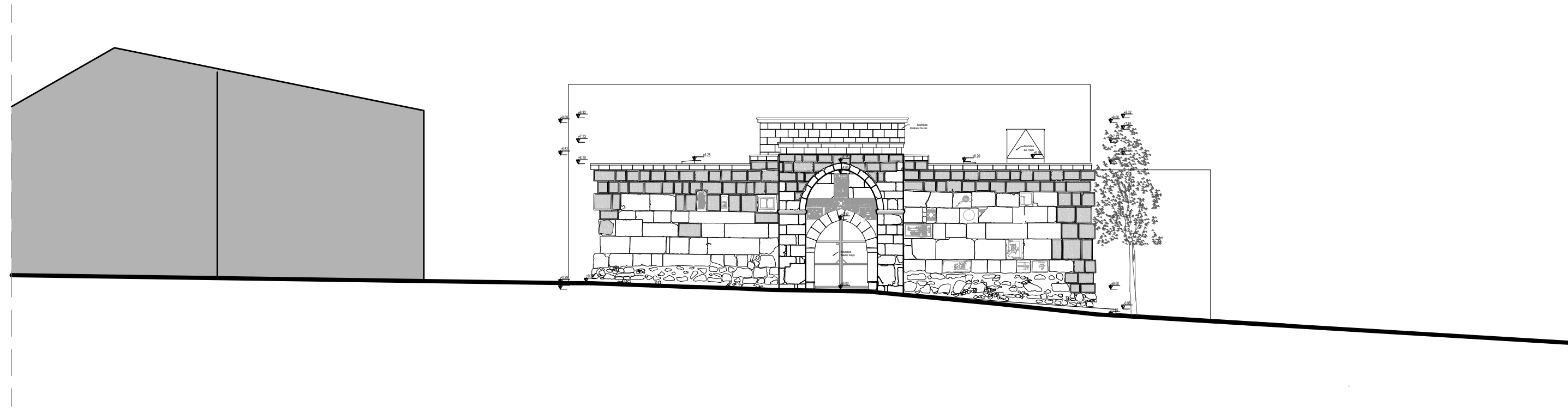
SİLÜET (DOĞU CEPHE)
