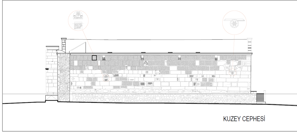
Şekil 3.8: Raziye Sultan Kervansarayı rölöve kuzey cephesi (Bayram, 2022)
