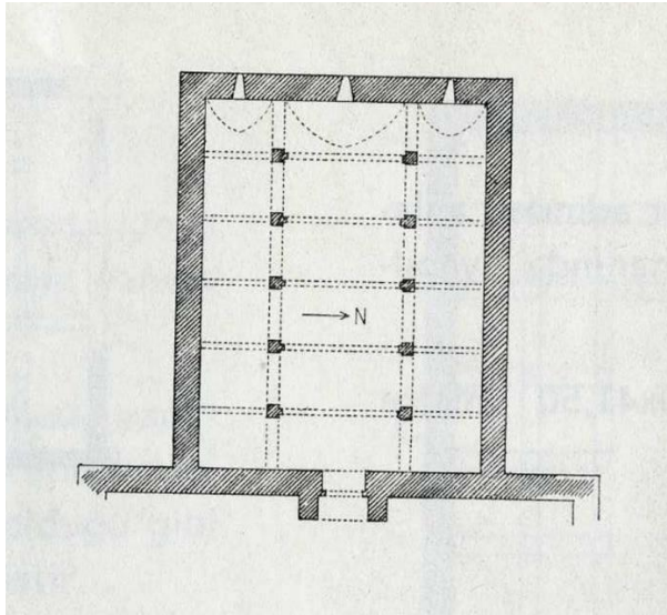
Şekil 4.9: Kadın Hanı planı (Erdmann, 1976)
