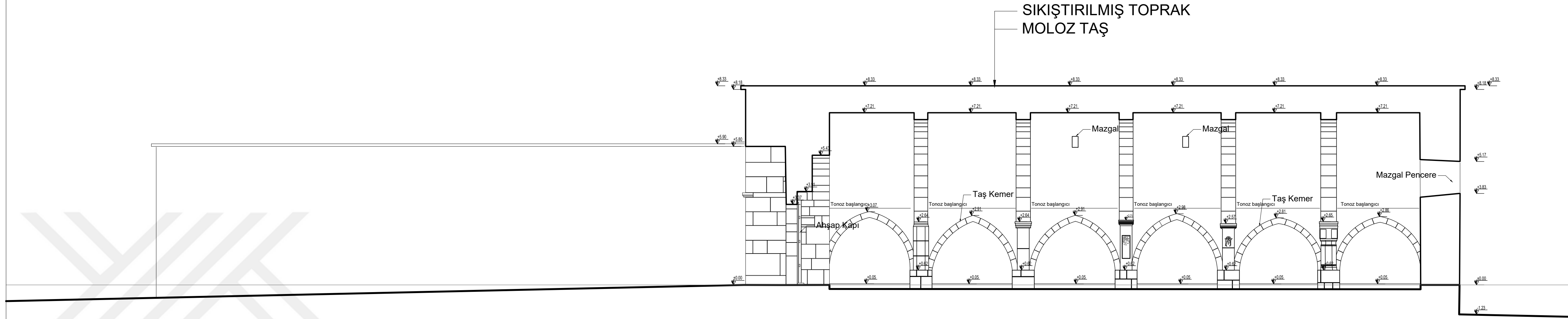
B-B KESİTİ
