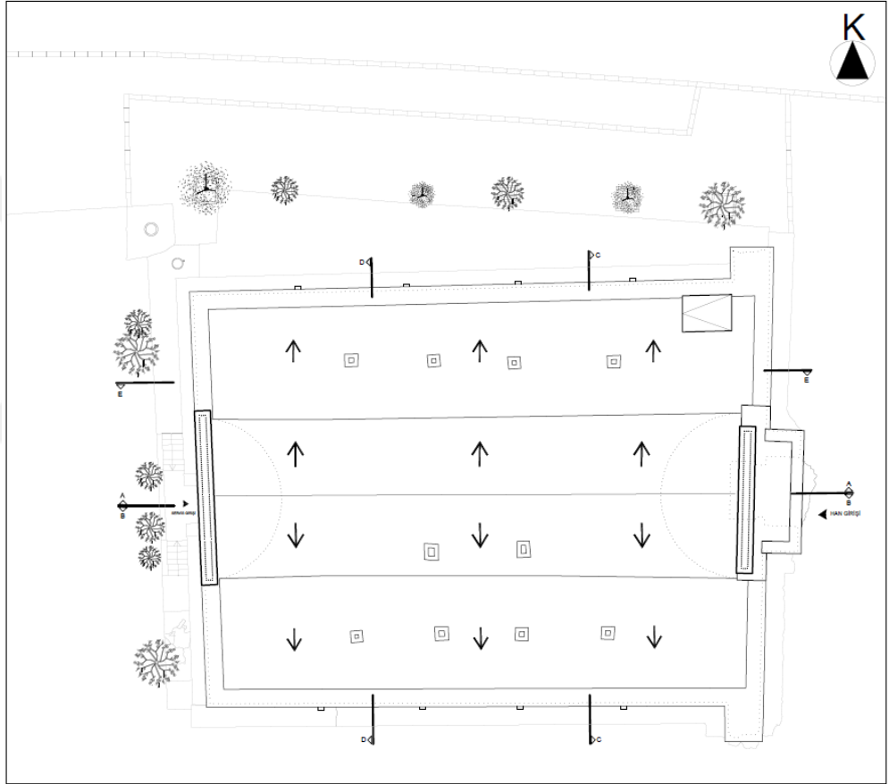
Şekil 3.7: Raziye Sultan Kervansarayı rölöve çatı planı (Bayram, 2022)
