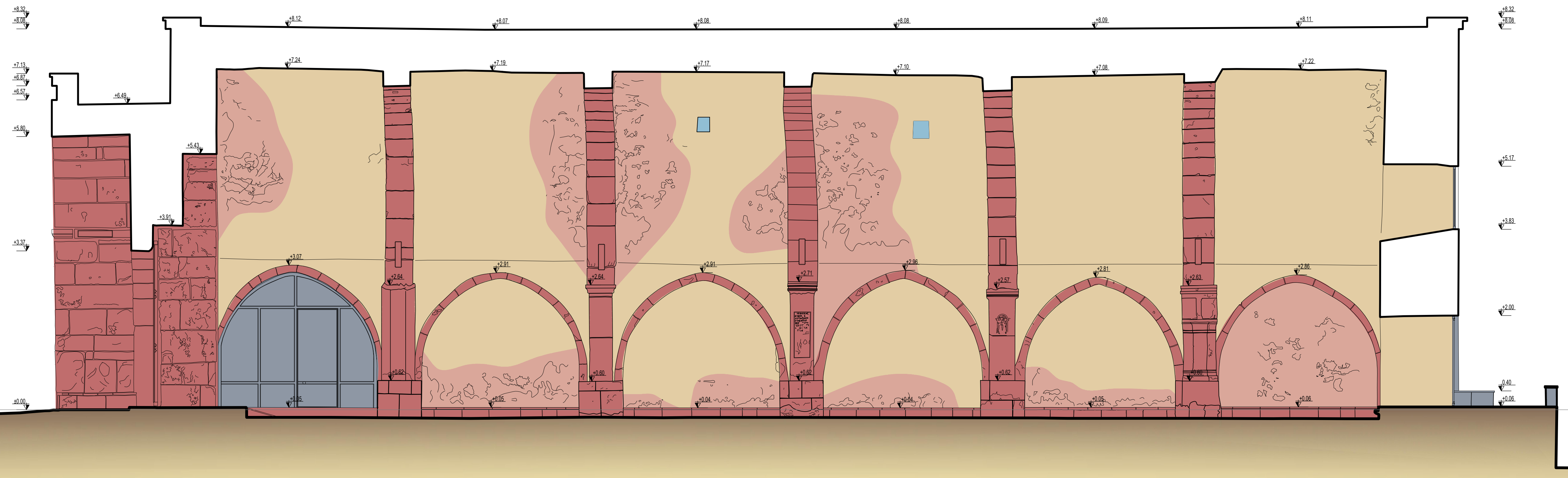
B-B KESİTİ
