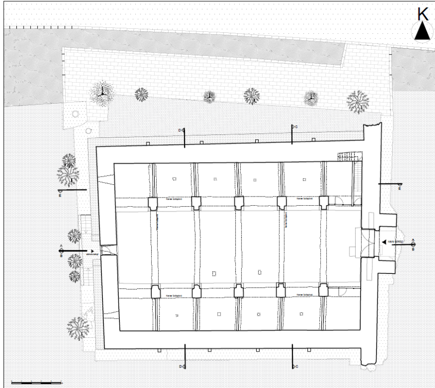
Şekil 3.6: Raziye Sultan Kervansarayı rölöve planı (Bayram, 2022)
