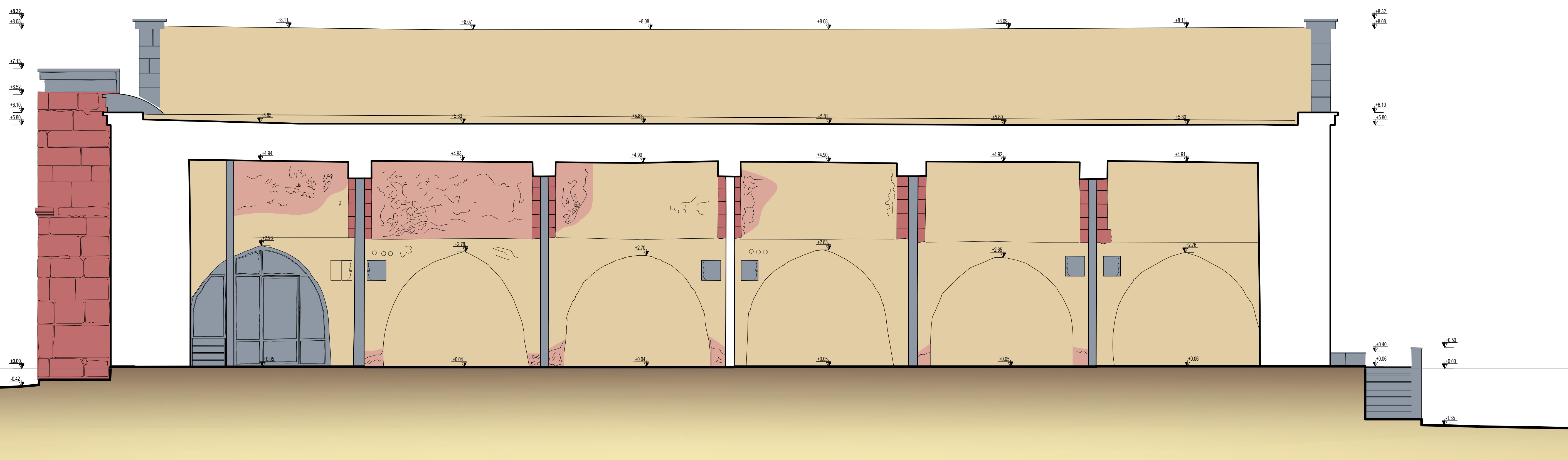
E-E KESİTİ
