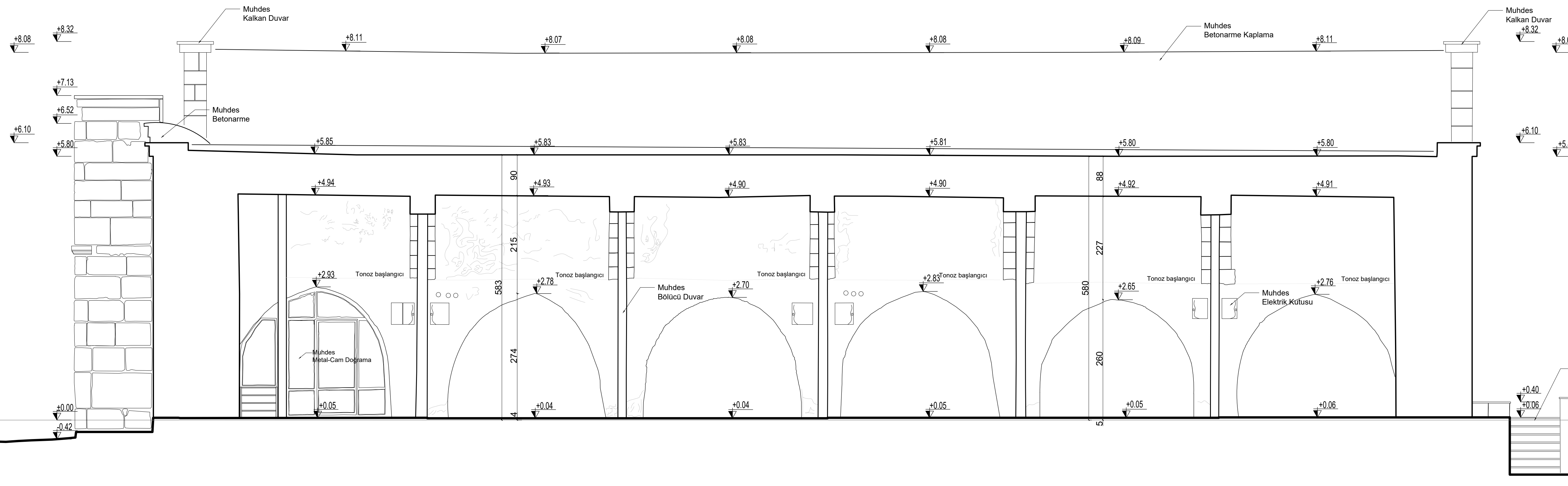
E-E KESİTİ
