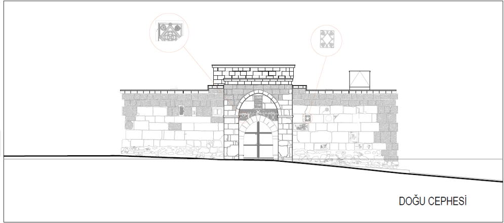
Şekil 3.10: Raziye Sultan Kervansarayı rölöve doğu cephesi (Bayram, 2022)
