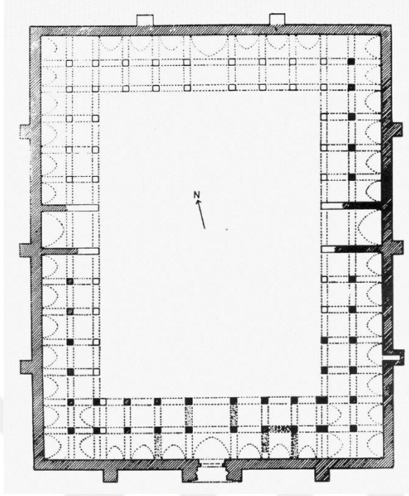
Şekil 2.9: Evdir Han planı, (Erdmann, 1961)
