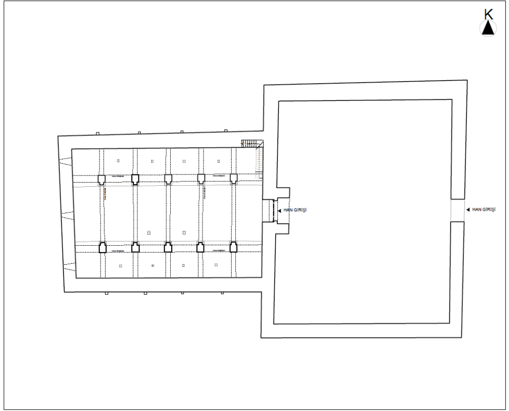
Şekil 3.5: Raziye Sultan Kervansarayı restirüsyon planı (Bayram, 2022)
