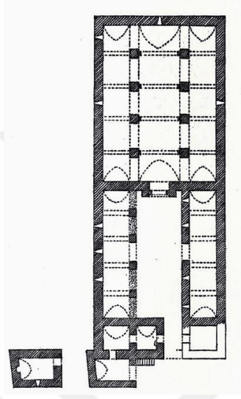
Şekil 2.1: Altınapa Han planı (Erdmann, 1961)
