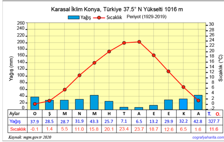
Şekil 1.2: Konya karasal iklim grafiği (URL-2)
