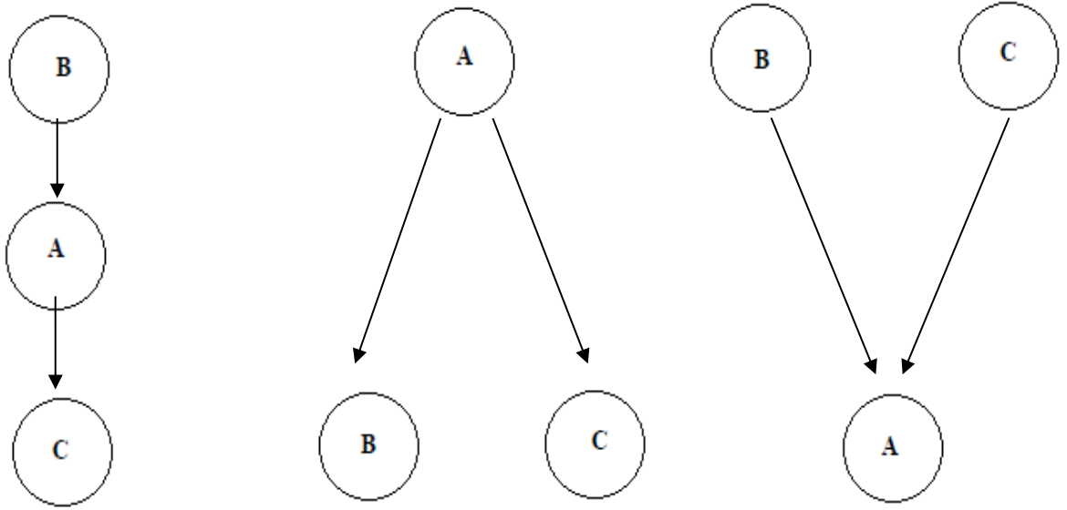
Şekil 2. 5. Bir Bayes Ağı'nda serisel, ıraksayan ve yakınsayan bağlantılar
