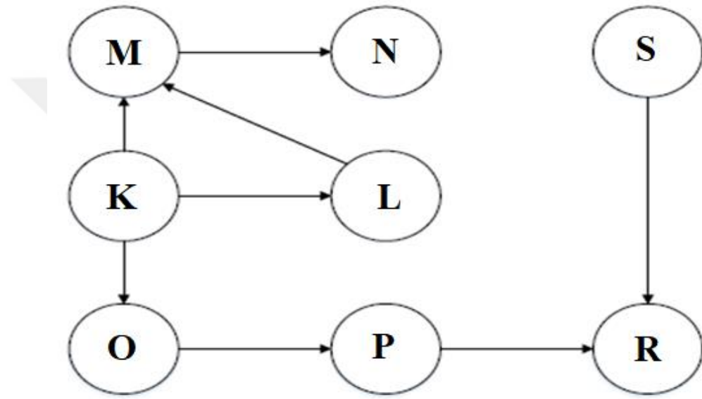
Şekil 2. 8. Aile ebeveyn, çocuk ve torun dışı düğümler için verilen Bayes Ağı örneği Bu ağ için her bir düğüm ile ilgili Çizelge 2.1 ortaya çıkarılmıştır.
