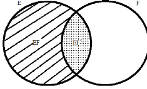
Şekil 2. 10. EF= Taralı alan, EFC = Noktalı alan gösterimi
