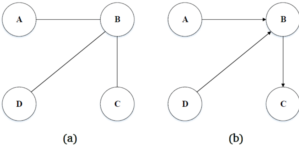
Şekil 2. 3. Dört düğümden oluşan yön verilmiş ve yön verilmemiş grafik örnekleri
