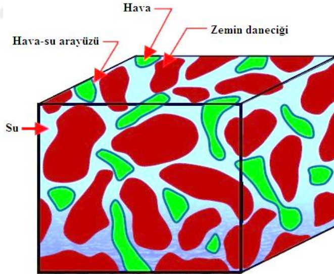
Şekil 3.3. Doygun olmayan bir zemin daneciğine ait dört fazlı bir elementin temsili gösterimi (Fredlund, 2005).
