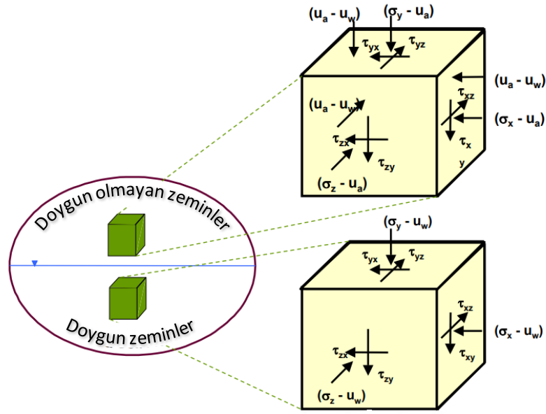
Şekil 3.8. Doygun ve doymun olmayan zemin değişkenleri küp formu (Fredlund ve Rahardjo, 1993).
