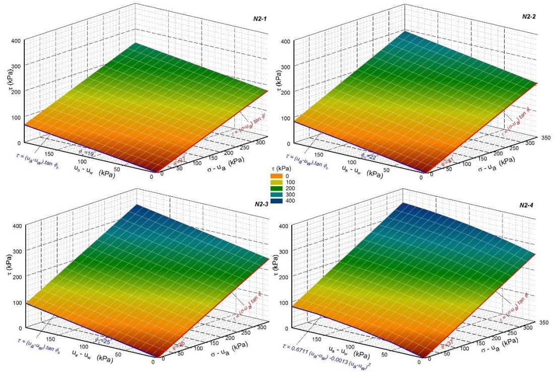
Şekil 4.36. 2. seri kayma yüzeyi çizimlerinin 3 boyutta gösterimi.
