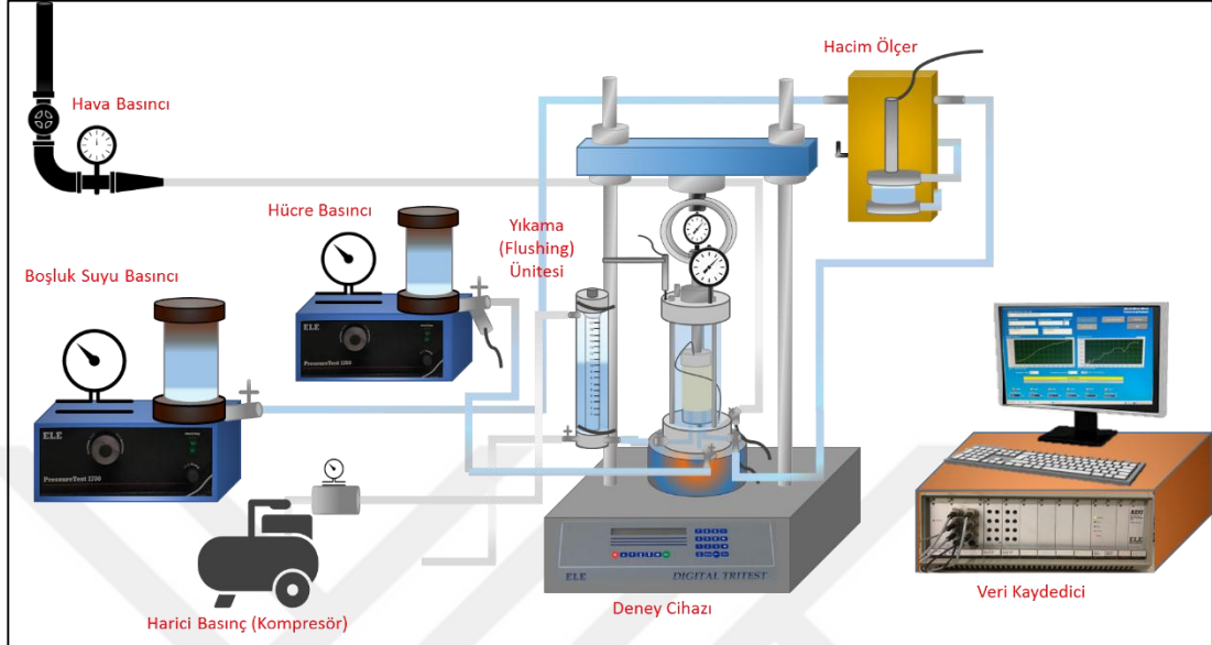
Şekil 4.23. Çalışmada doymayan deneyler için kullanılan üç eksenli hücre kesme deney cihazı.
