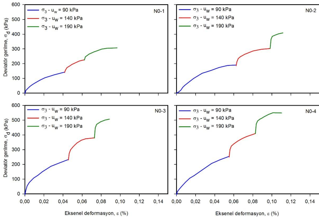
Şekil 4.20. Doygun zeminler için çok aşamalı hücre kesme deneyi gerilme-şekil değiştirme eğrileri.
