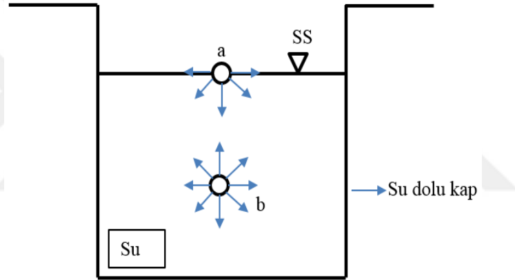
Şekil 3.4. (a) Hava-su arayüzü kuvvetleri, (b) Su içindeki moleküller arası kuvvetler (Özocak, 2003).
