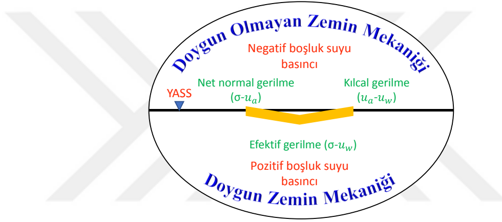
Şekil 1.1. Doymun ve doymun olmayan zeminlerin genel gösterimi (Fredlund ve ark., 2012).
