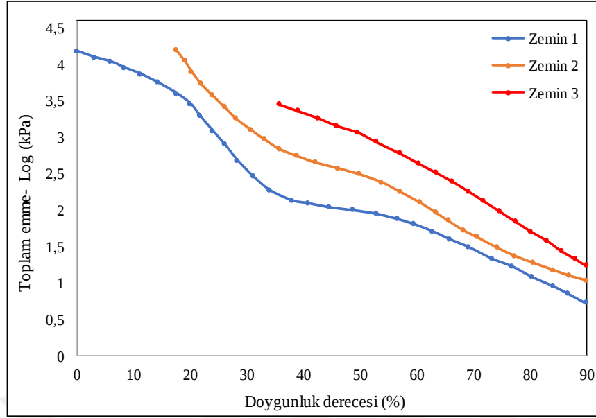
Şekil 2.8. %0 tuz oranına sahip üç zemin için toplam emme ve doygunluk derecesi arasındaki ilişki (Fattah ve ark., 2013).
