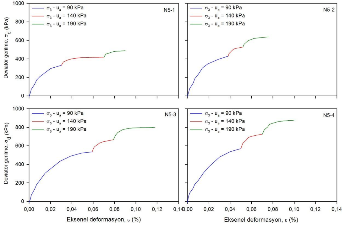
Şekil 4.42. 5. seri emme kontrollü gerilme-şekil değiştirme eğrileri.
