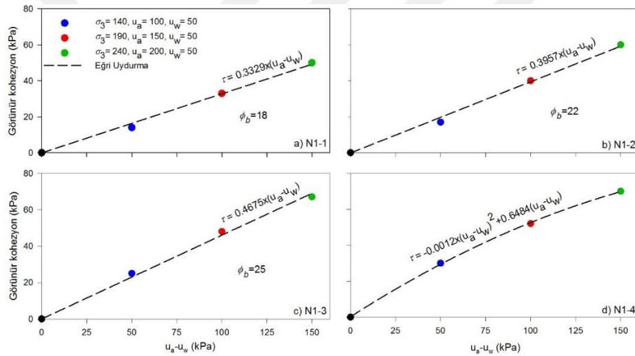
Şekil 4.30. 1. seri kılcal gerilmeye karşılık görünür kohezyon değerleri (Doygun durumda kohezyon değerleri 0'dır).
