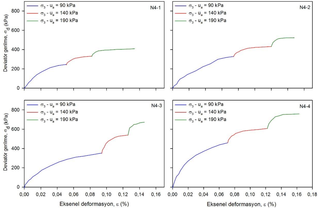
Şekil 4.40. 4. seri emme kontrollü gerilme-şekil değiştirme eğrileri.
