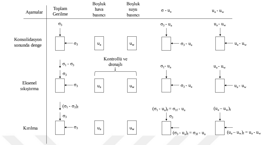
Şekil 3.20. Konsolidasyonlu-Drenajlı (CD) üç eksenli hücre kesme testinin çeşitli aşamalarındaki gerilme koşulları.
