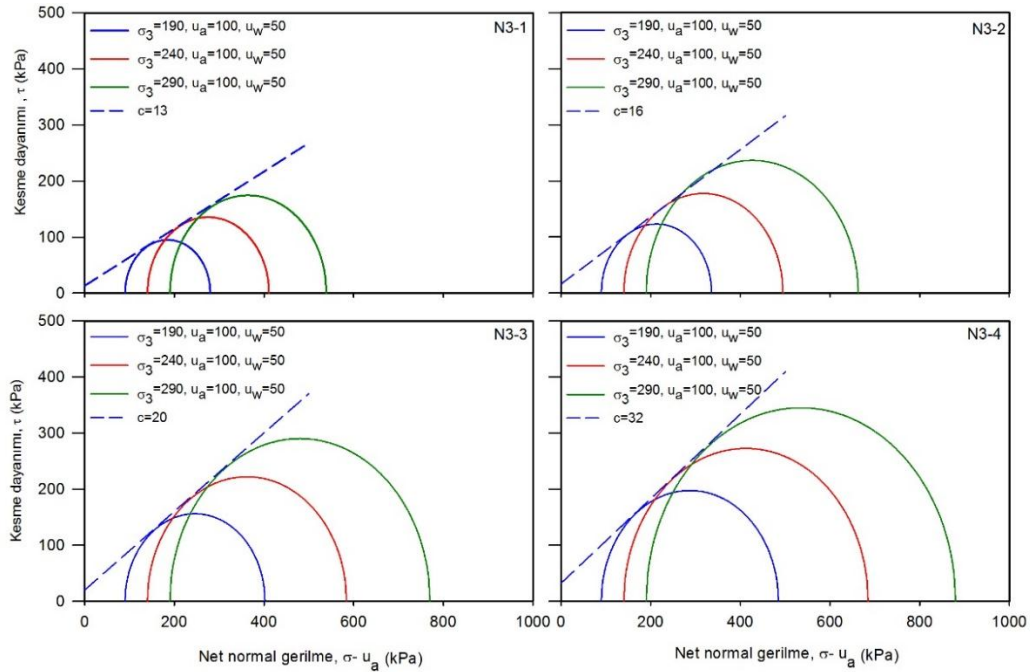
Şekil 4.39. 3. seri net normal gerilme ile kayma direnci arasındaki ilişki.
