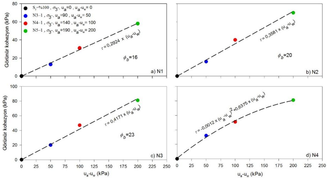
Şekil 4.44. Yöntem 2 deneylerine ait kılcal gerilmeye karşılık görünür kohezyon değerleri (Doygun durumda kohezyon değerleri 0'dır).
