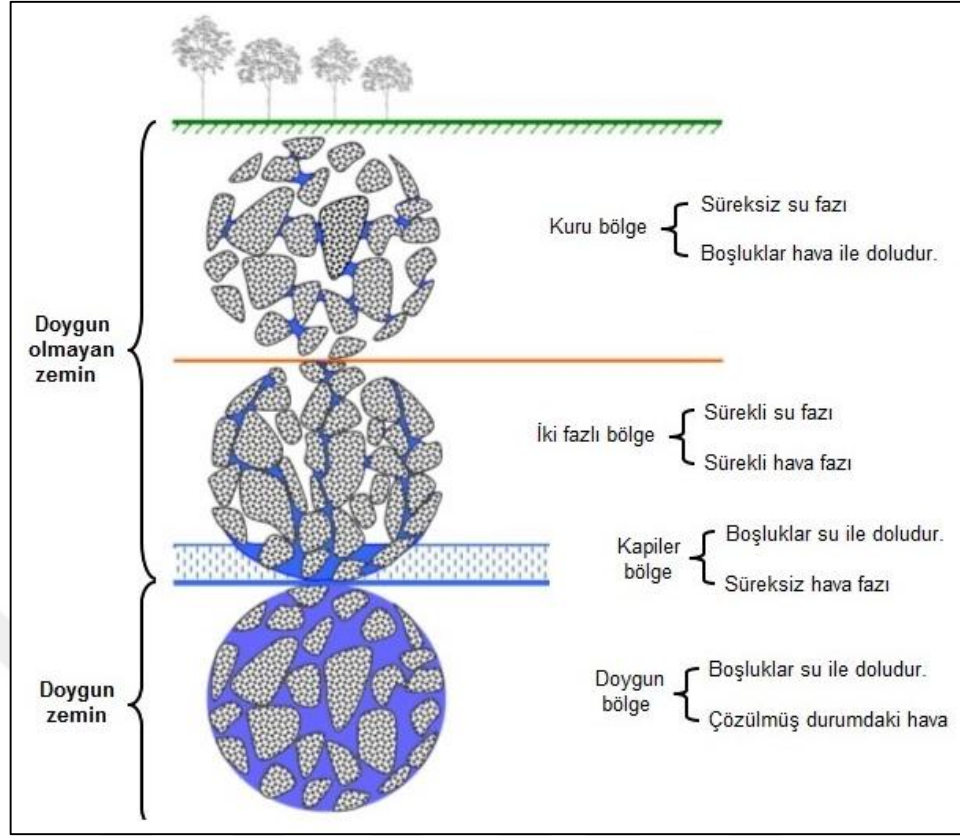
Şekil 3.1. Doygun olmayan zemin profili (Rasool, 2014).
