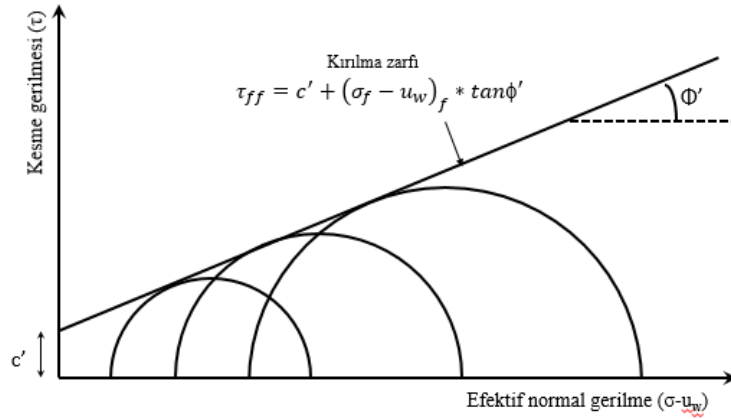
Şekil 3.7. Doygun zeminler için Mohr Coulomb kırılma zarfı.
