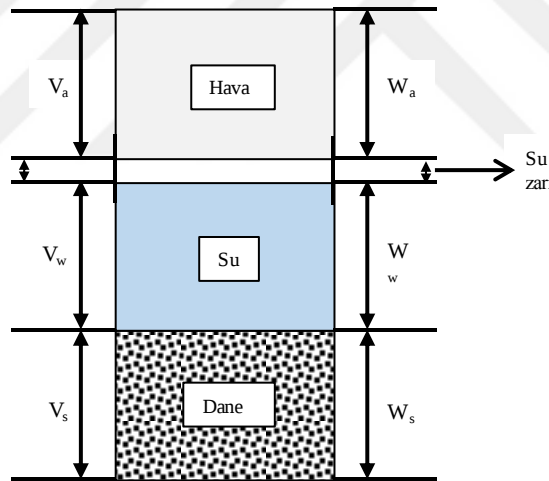
Şekil 3.5. Doygun olmayan zemin için dört fazlı blok diyagramı (Fredlund ve Rahardjo, 1993; Özocak, 2003).
