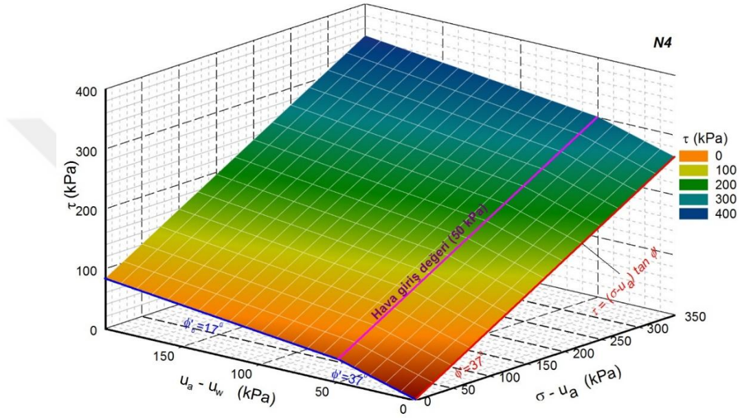
Şekil 4.46. Yöntem 2 numunelerine ait çift düzlem ile kayma yüzeyi çizimi.
