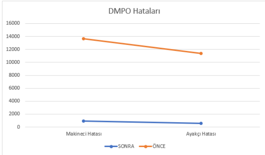
Şekil 4.28. DMPO hataları.
