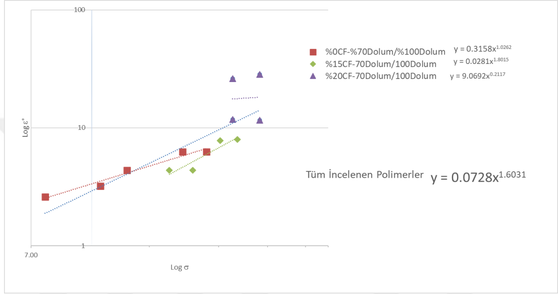
Şekil 5.10. İncelenen polimerlerin “log \epsilon^\circ -log \sigma ” grafiği.
