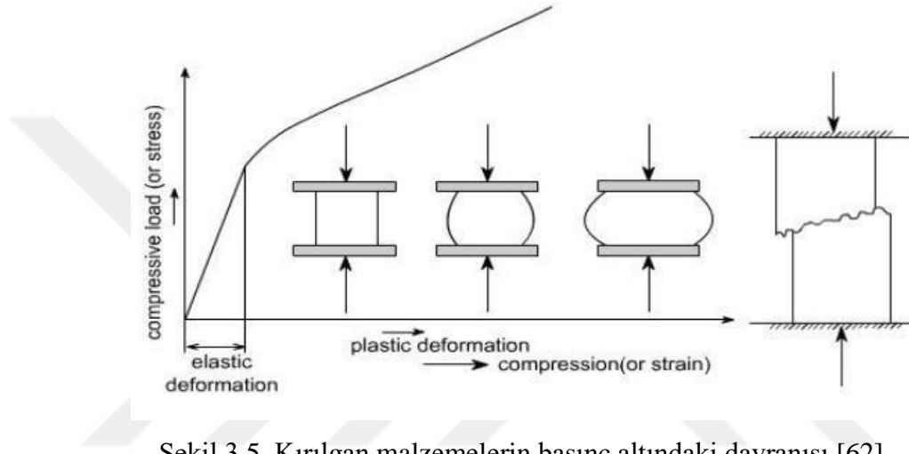
Şekil 3.5. Kırılmalı malzemelerin basınç altındaki davranışı [62].
