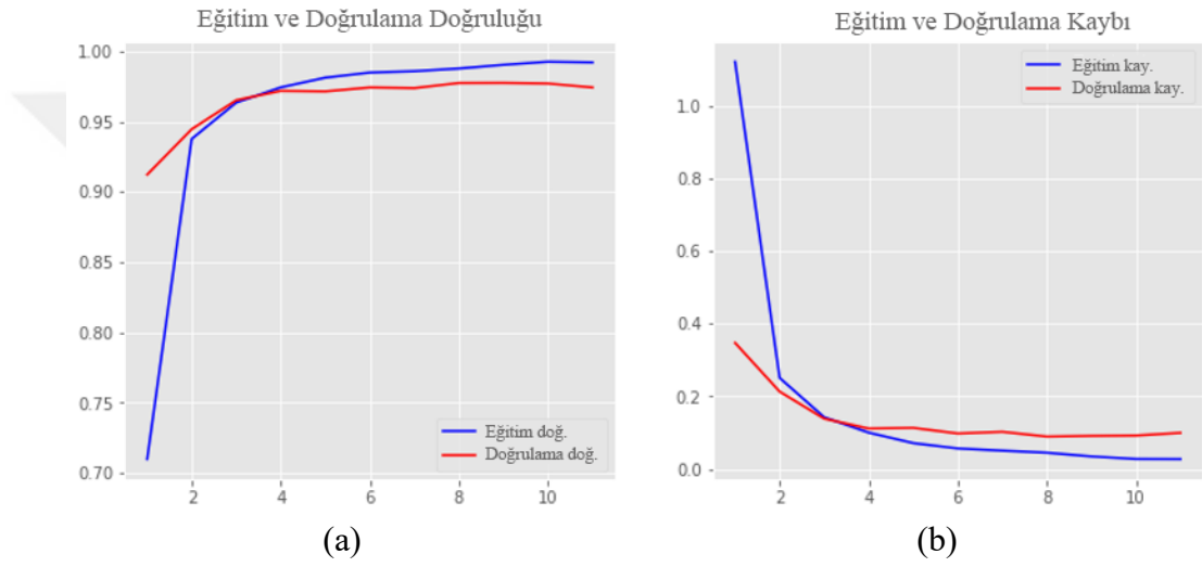
Şekil 5.2. Çift katmanlı, çift yönlü LSTM modelinin eğitim ve doğrulama sonuç grafikleri.
