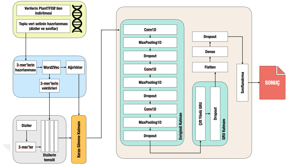
Şekil 6.3. Çalışmanın akış şeması.
