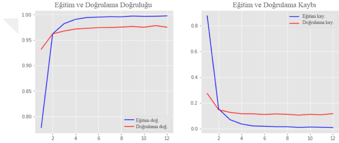
(d) M-2-4 modelinin eğitim ve doğrulama sonuç grafikleri.
