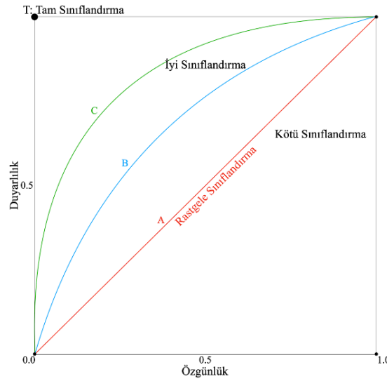
Şekil 4.24. Çeşitli durumları gösteren örnek bir ROC eğrisi.
