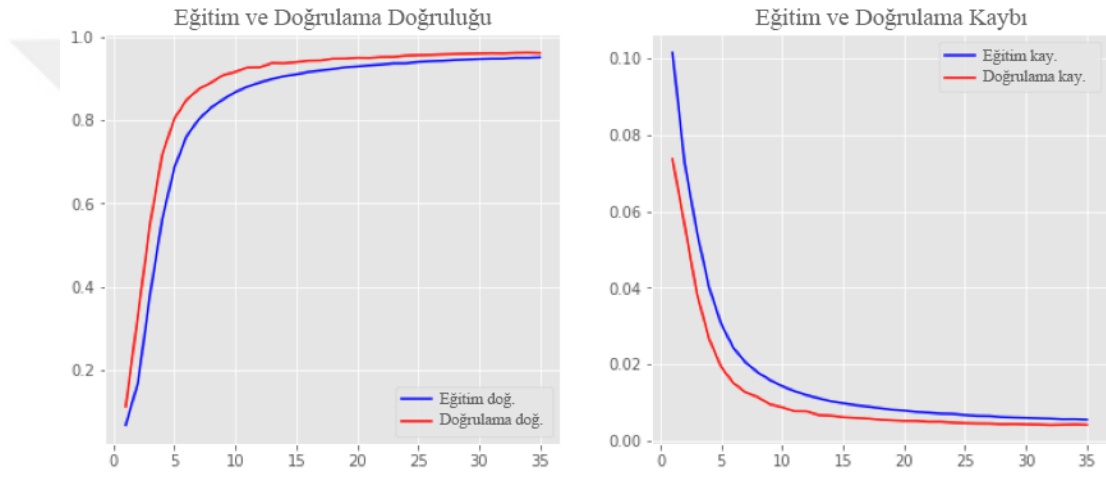
(a) M-6-1 modelinin eğitim ve doğrulama sonuç grafikleri.
