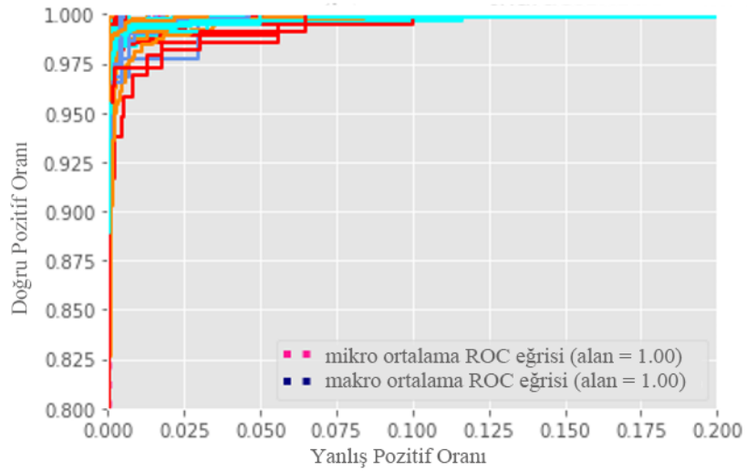
(b) ROC grafiğinin yakınlaştırılmış hali.
