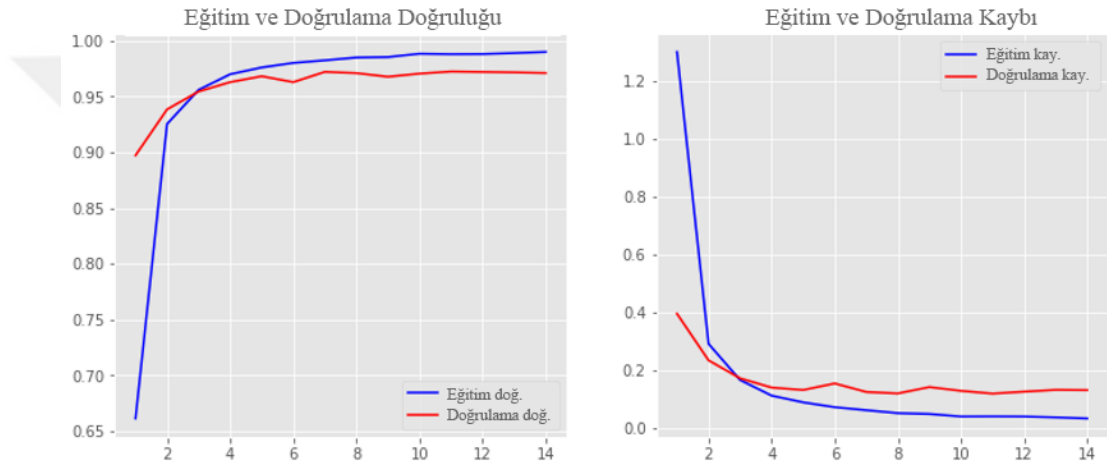
(a) Çift Yönlü LSTM modelinin eğitim ve doğrulama sonuç grafikleri.
