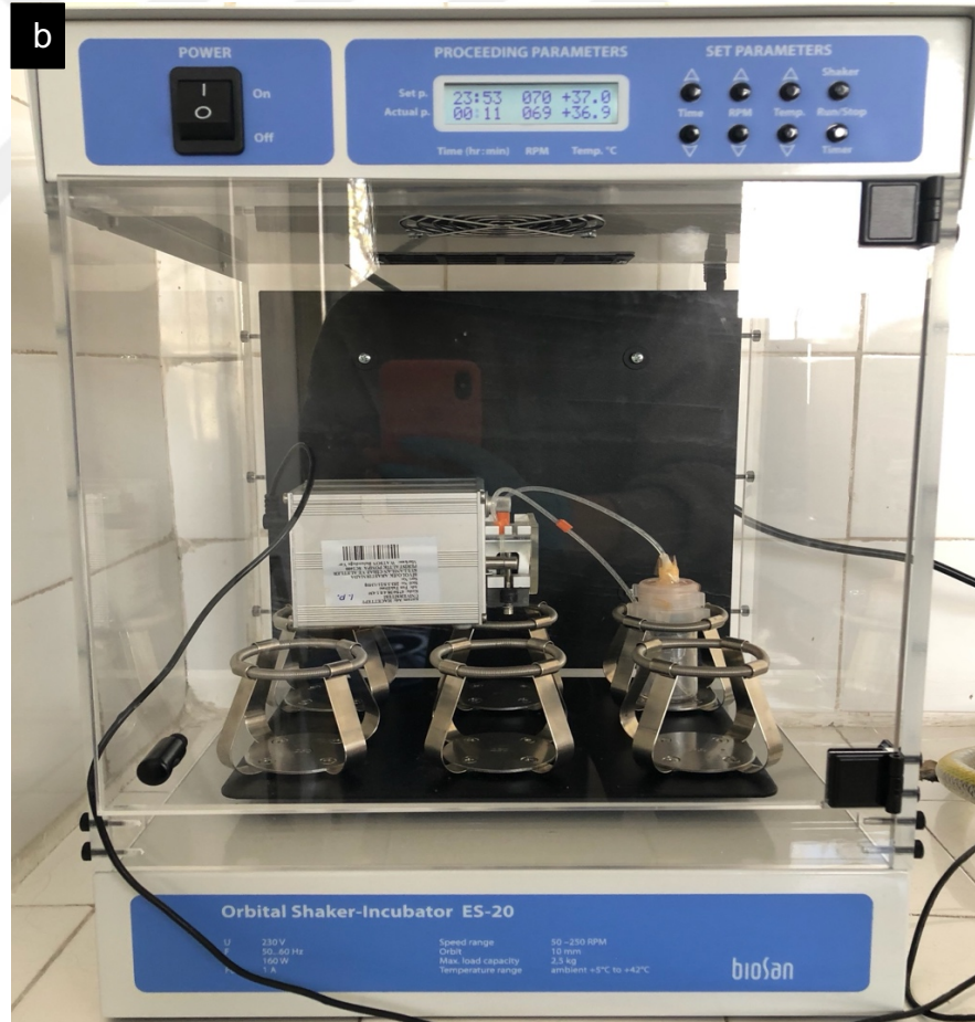
Şekil 3.6. a) Devamlı sistem için kartuş ve peristaltik pompanın kurulması, b) Deney düzeneğinin kurularak hücre süspansiyonunun kartuştan geçirilmesi.
