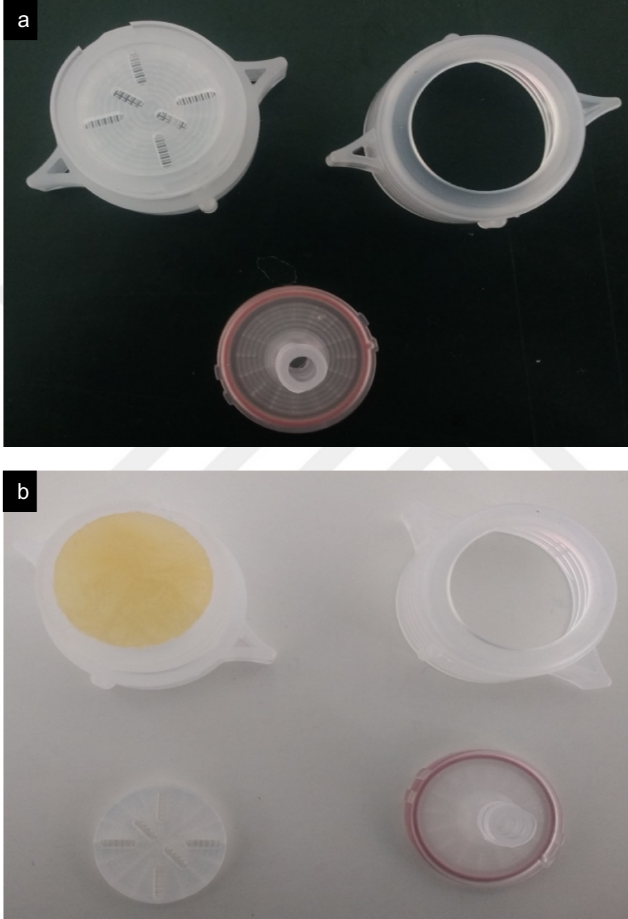
Şekil 3.5. a) Devamlı sistemde kullanılacak kartuş sisteminin hazırlanması, b) Kartuş sistemine çalışılacak kriyojel grubunun yerleştirilmesi.
