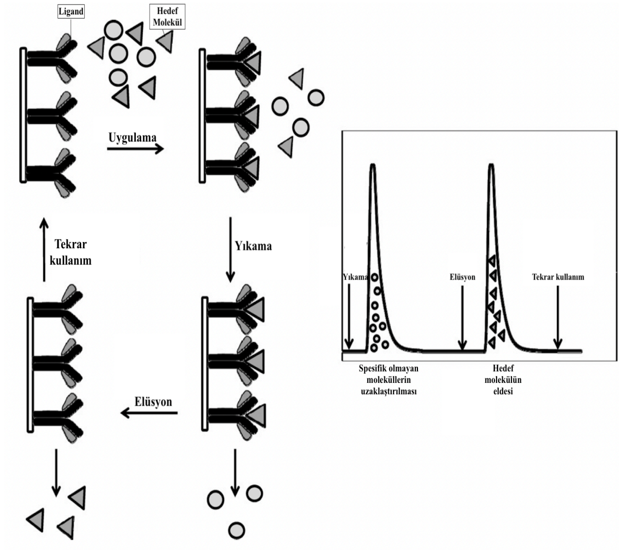
Şekil 2.4. Affinite kromatografisi [103].
