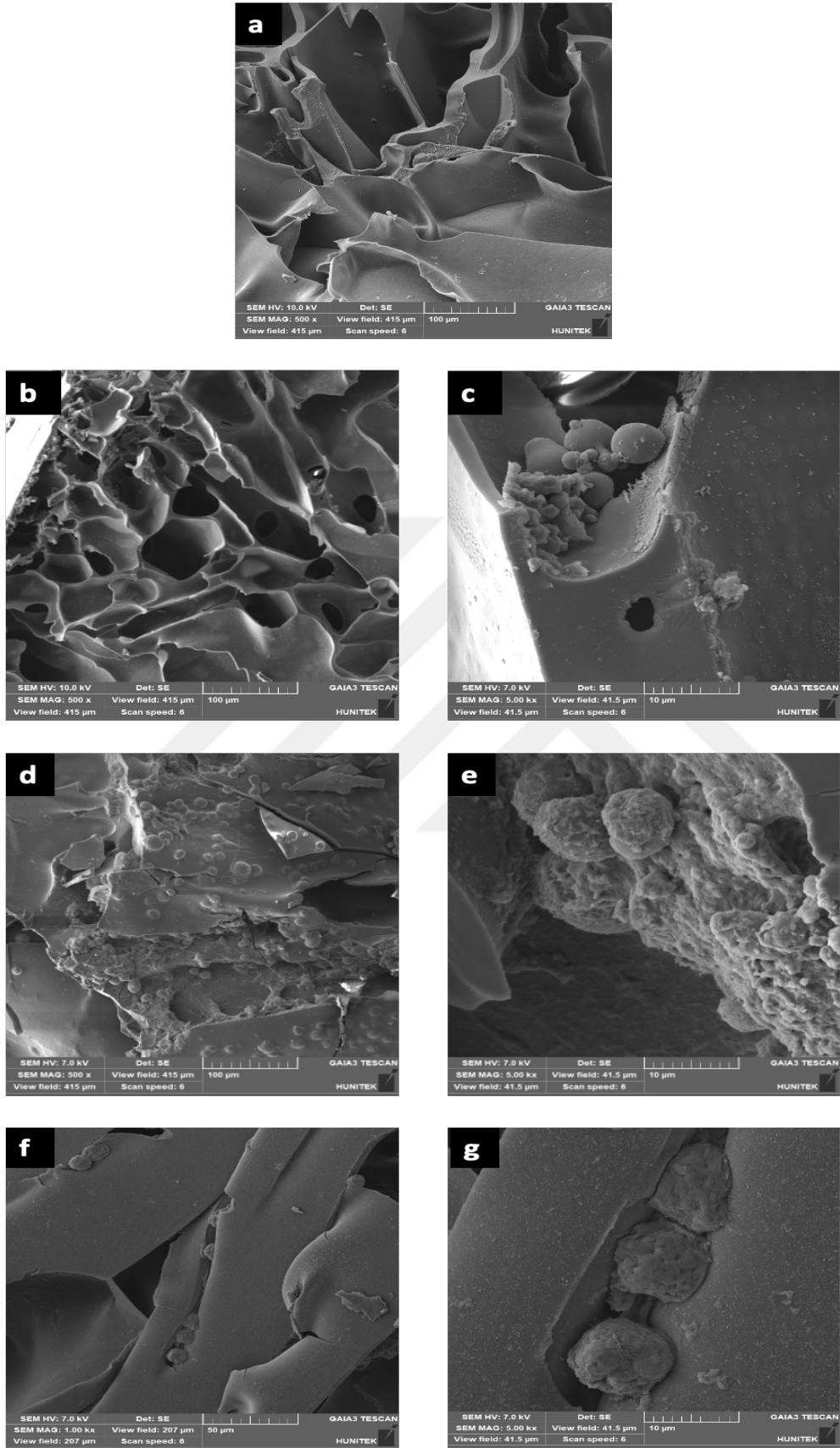
Şekil 4.7. SEM görüntüleri: a) MDA-MB-231, PHEMA-G, b,c) MCF-7, PHEMA-G, d,e) MDA-MB-231, PHEMA-G-BSA100-ConA, f,g) MCF-7, PHEMA-G-BSA100-ConA.
