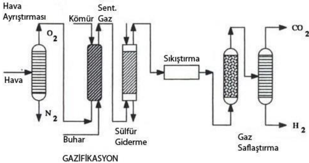
Şekil 2.2. Kömürün gazlaştırılması [40]
