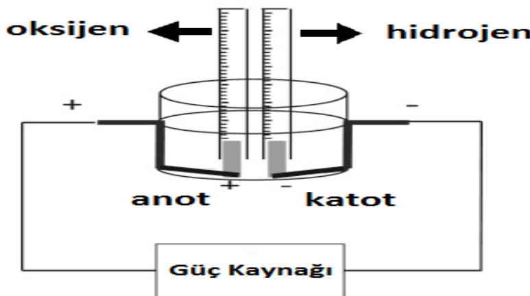
Şekil 2.4. Elektroliz yöntemi [45]
