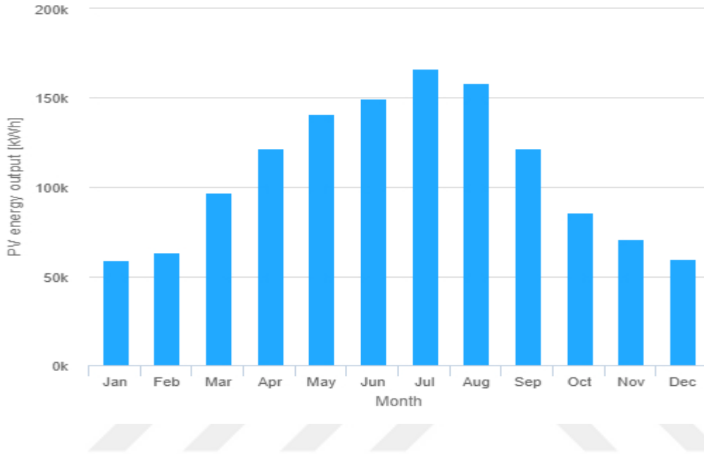
Şekil 5.17. Sakarya ilinde tasarlanan PV sisteminin aylık enerji üretimi
