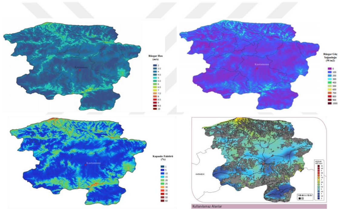
Harita 5.22. Kastamonu ilinin rüzgar enerji potansiyel atlası [77]
