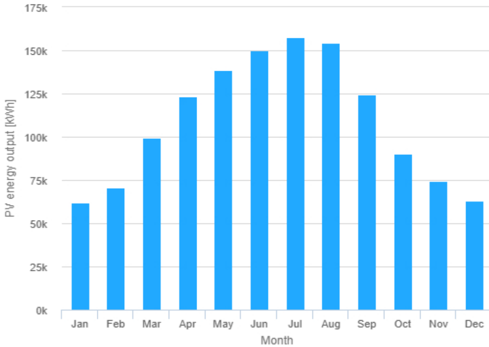
řekil 5.7. Sinop ilinde tasarlanan PV sisteminin aylık enerji retimi
