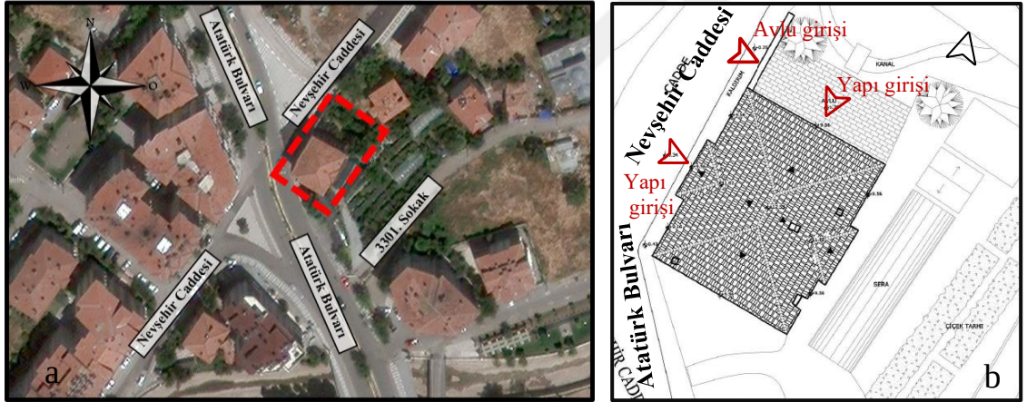
Şekil 4.9. a) Yapı konumu (Yandex Maps görüntüsü üstüne işlenmiştir.), b) Konut-1 rölöve vaziyet planı (Karadayı Yenice, 2012)
