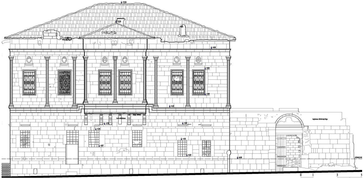
Şekil 4.21. Konut-1 doğu cephesi rölöve çizimi (Karadayı Yenice, 2012)
