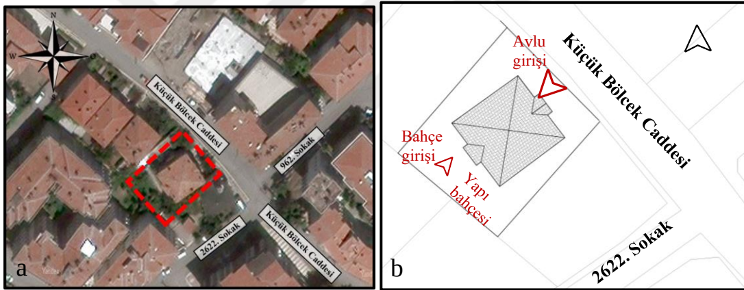
Şekil 4.108. a) Yapı konumu (Yandex Maps görüntüsü üstüne işlenmiştir.), b) yapı vaziyet planı
