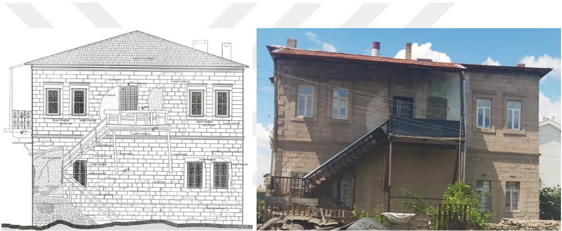
Şekil 4.171. Konut-15 doğu cephesi rölöve çizimi (Karadayı Yenice, 2012) ve doğu cephesi
