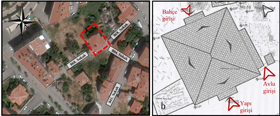
Şekil 4.162. a) Yapı konumu (Yandex Maps görüntüsü üstüne işlenmiştir.), b) yapı vaziyet planı rölöve çizimi (Karadayı Yenice, 2012)
