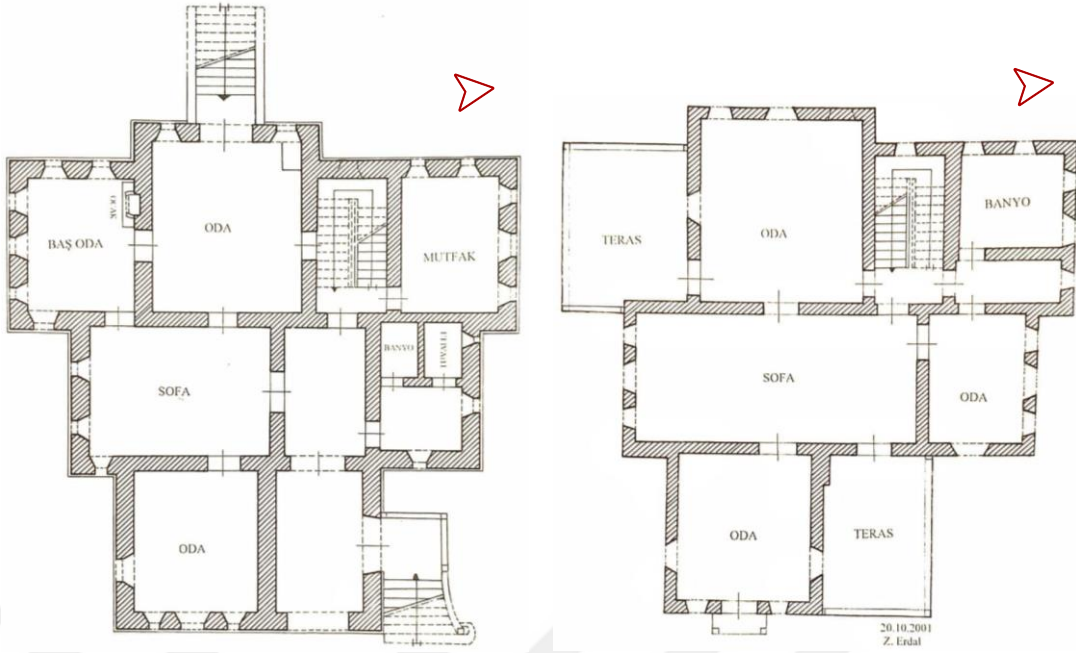
Şekil 4.96. Konut-8 zemin kat ve Birinci kat planı rölövesi (Erdal, 2016)
