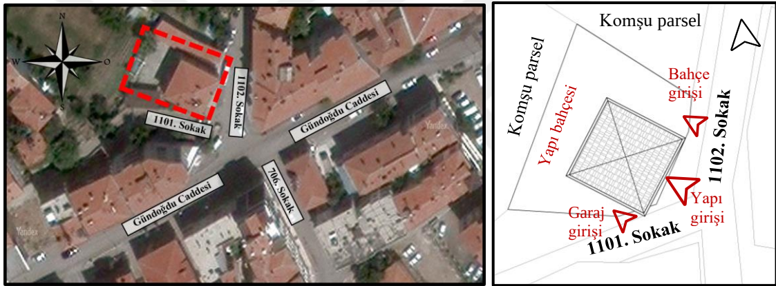
Şekil 4.35. a) Yapı konumu (Yandex Maps görüntüsü üstüne işlenmiştir.), b) yapı vaziyet planı
