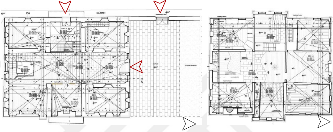
Şekil 4.10. Konut-1 zemin kat (solda) ve birinci kat (sağda) rölöve planı (Karadayı Yenice, 2012)
