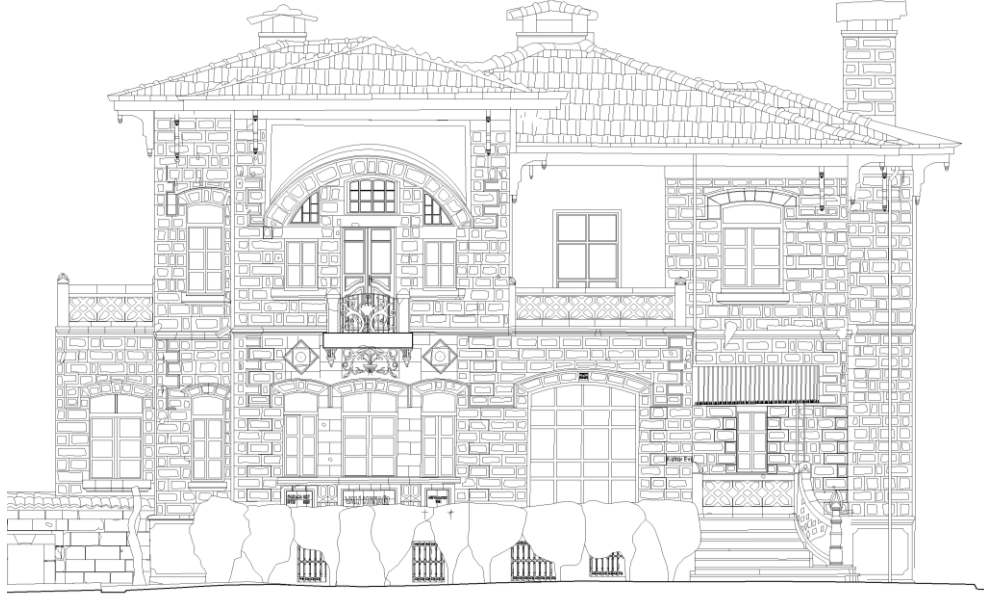
Şekil 4.98. Konut-8 doğu cephe rölöve çizimi (Mutlu arşivinden düzenlenmiştir.)
