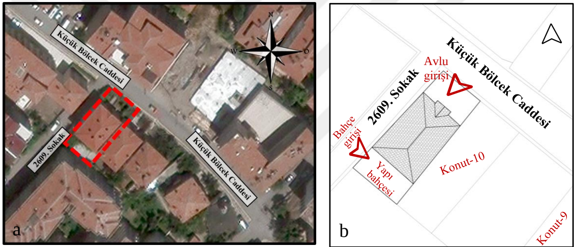
Şekil 4.123. a) Yapı konumu (Yandex Maps görüntüsü üstüne işlenmiştir.), b) yapı vaziyet planı
