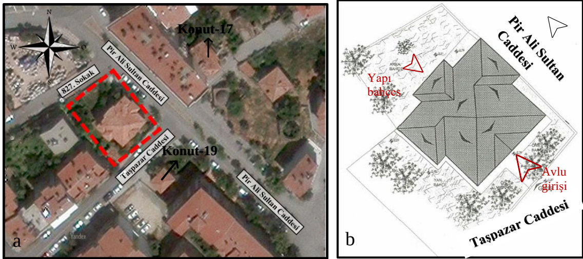
Şekil 4.182. a) Yapı konumu (Yandex Maps görüntüsü üstüne işlenmiştir.), b) yapı vaziyet planı rölöve çizimi (Karadayı Yenice, 2012)
