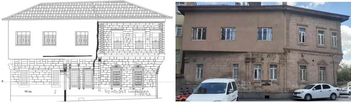
Şekil 4.58. Konut-4 batı cephesi rölöve çizimi (Karadayı Yenice, 2012) ve cephe görünüşü
