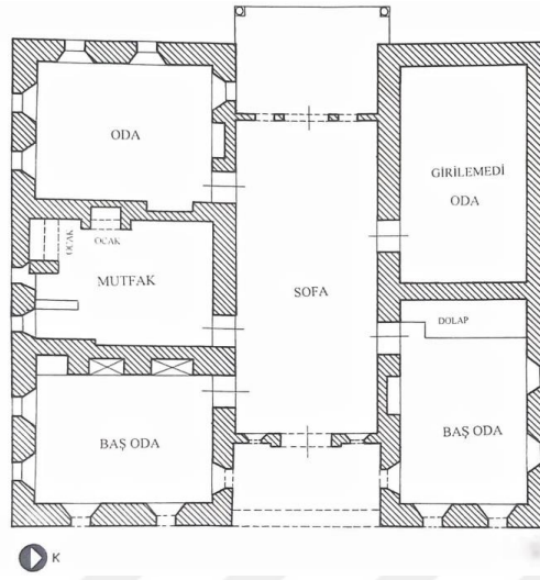
Şekil 4.86. Konut-7 rölöve planı (Erdal, 2016)
