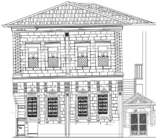
Şekil 4.49. Konut-4 güney cephesi rölöve çizimi (Karadayı Yenice, 2012) ve cephe görüntüsü
