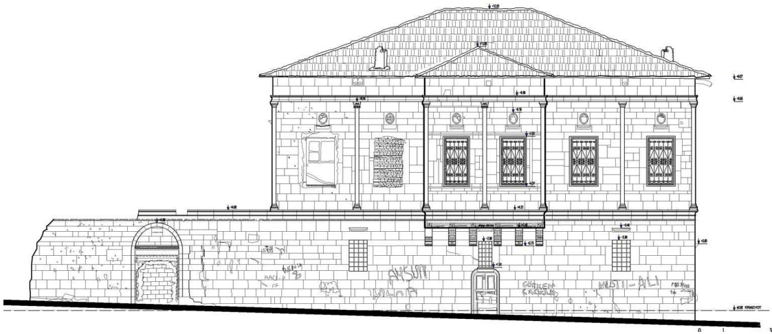
Şekil 4.14. Konut-1 batı cephesi rölöve çizimi (Karadayı Yenice, 2012)
