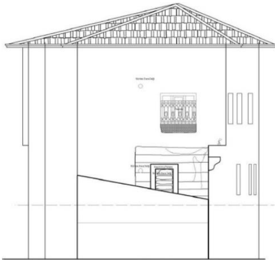
Şekil 4.56. Konut-4 kuzey cephesi (Karadayı Yenice, 2012) ve kuzeybatı cephesi
