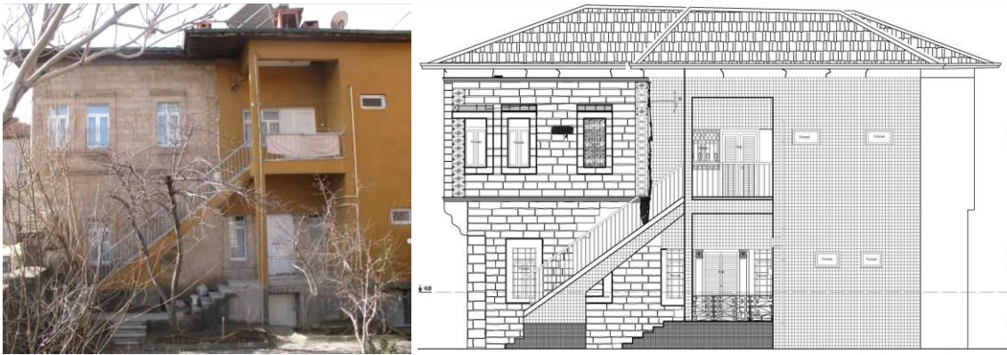
Şekil 4.55. Konut-4 doğu cephesi ve rölöve çizimi (Karadayı Yenice, 2012)
