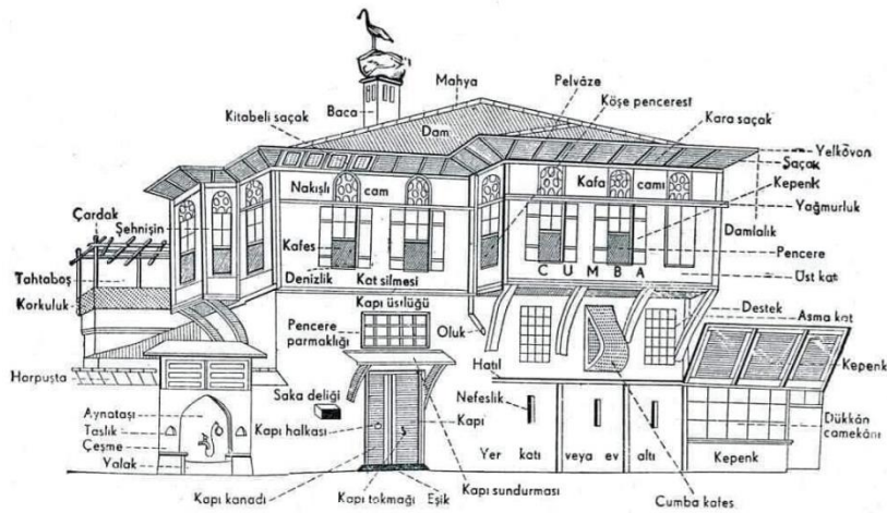
Şekil 3.9. Türk evi cephe elemanları gösterimi (Arseven, 1947'den düzenlenmiştir.)
