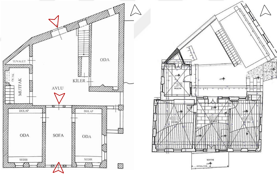
Şekil 4.134. Konut-12 zemin kat planı rölöve çizimi (Erdal, 2016) ve Birinci kat planı rölöve çizimi (Karadayı Yenice, 2012)
