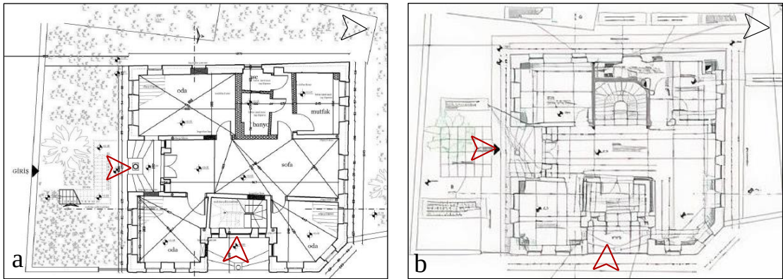
Şekil 4.64. Konut-5 zemin kat rölöve(a) ve restorasyon(b) çizimi (Karadayı Yenice ve Dülgerler, 2014)
