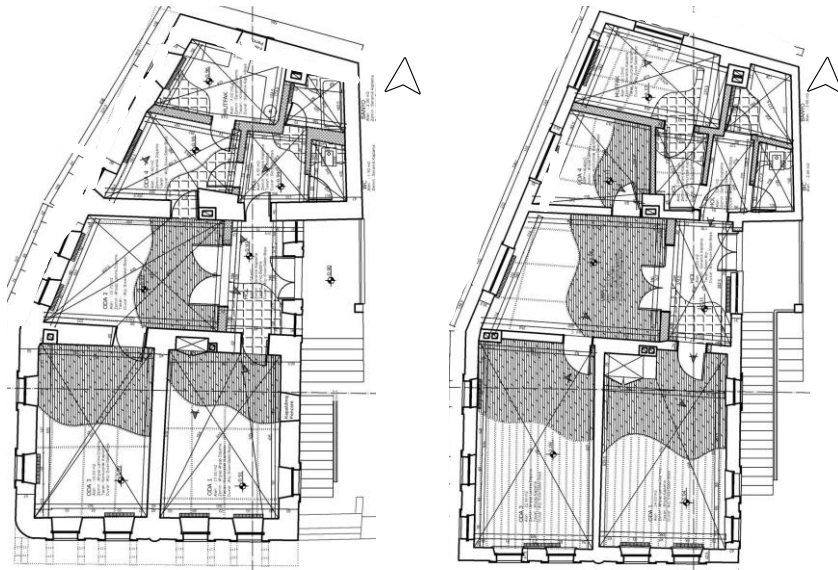
Şekil 4.46. Konut-4 muhdes ekli zemin(solda) ve birinci kat planı (Karadayı Yenice, 2012)
