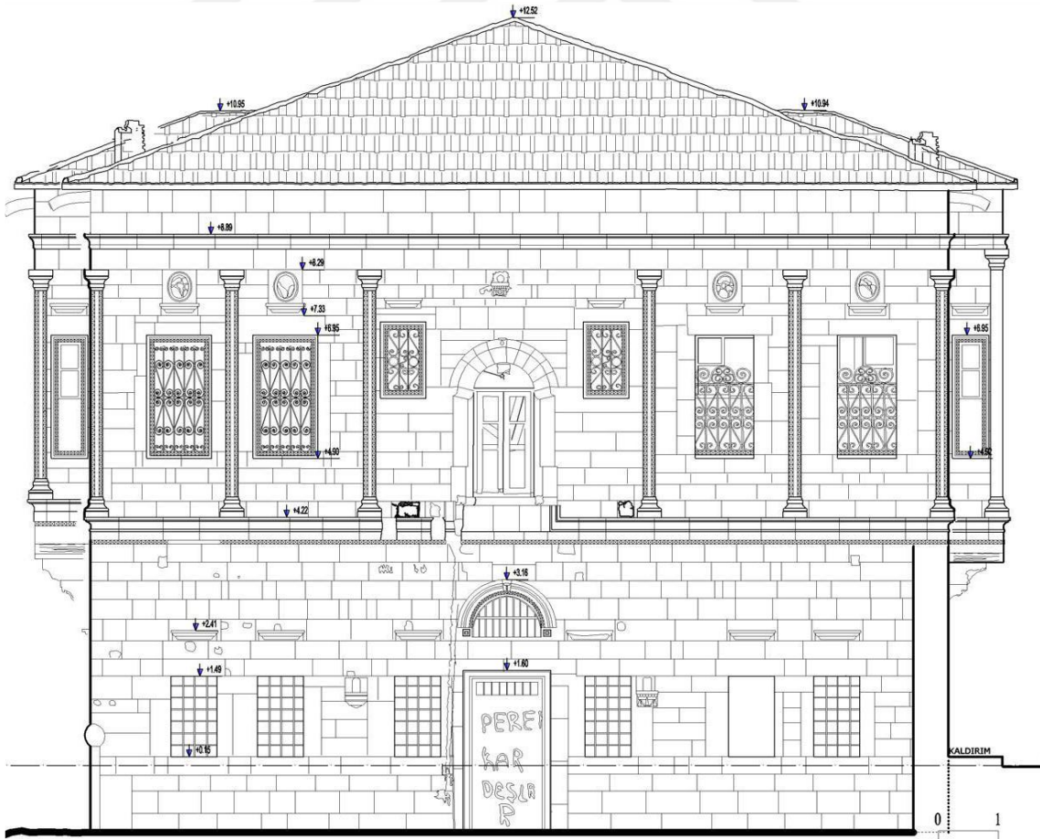
Şekil 4.18. Konut-1 kuzey cephesi rölöve çizimi (Karadayı Yenice, 2012)
