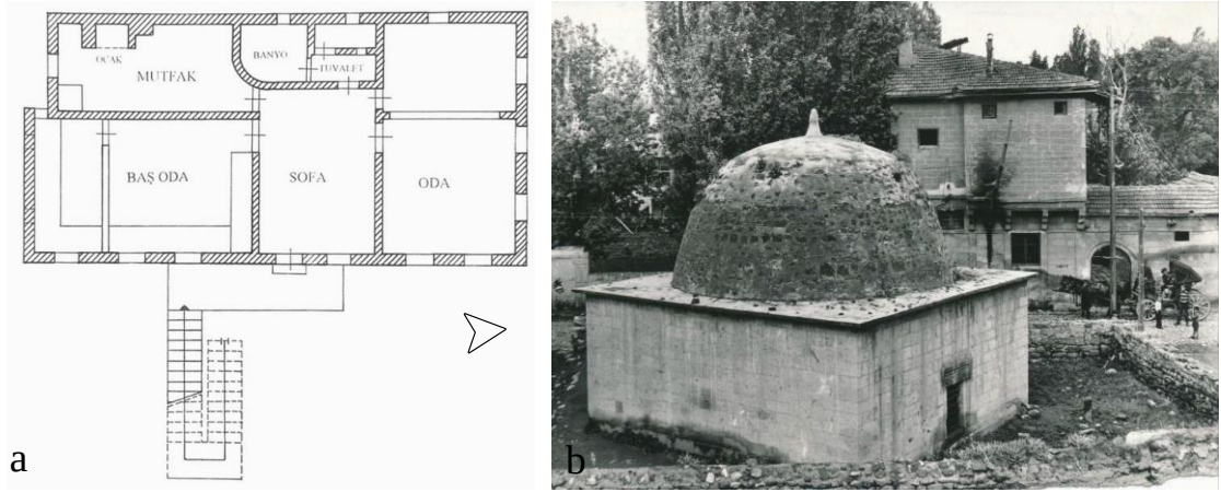
Şekil 4.178. a) Konut-17 Birinci kat planı rölöve çizimi (Erdal, 2016), b) Geleneksel konutun Pir Ali Sultan türbesinden güney cephesi tarihi görünümü (Aksaray İl Kültür ve Turizm Müdürlüğü arşivi)
