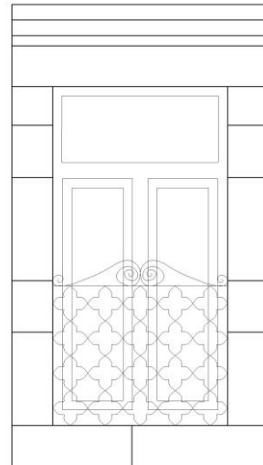
Şekil 4.54. Güney cephe birinci kat penceresi ve köşebendi
