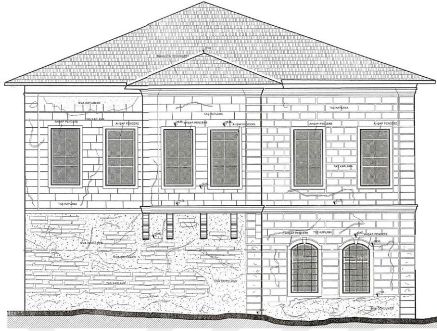
Şekil 4.188. Konut-18 batı cephe rölöve çizimi (Karadayı Yenice, 2012)
