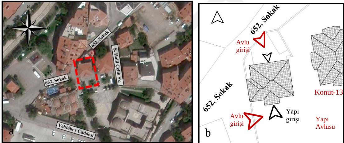
Şekil 4.132. a) Yapı konumu (Yandex Maps görüntüsü üstüne işlenmiştir.), b) yapı vaziyet planı
