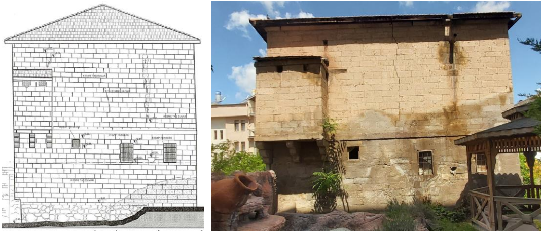
Şekil 4.200. Konut-19 güney cephesi rölöve çizimi (Karadayı Yenice, 2012) ve cephe görünüşü
