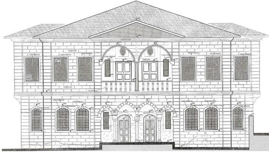
Şekil 4.185. Konut-18 güney cephesi rölöve çizimi (Karadayı Yenice, 2012)
