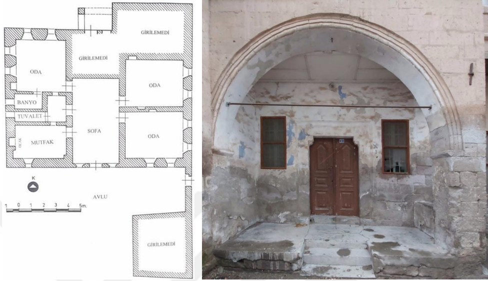
Şekil 4.75. Konut-6 zemin kat planı (Erdal, 2006) ve kemerli girişi
