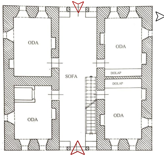
Şekil 4.109. Konut-9 zemin kat rölöve planı (Erdal, 2016)
