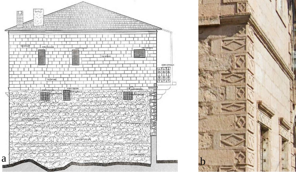
Şekil 4.169. a) Batı cephesi rölöve çizimi (Karadayı Yenice, 2012), b) geometrik bezemeli köşebent
