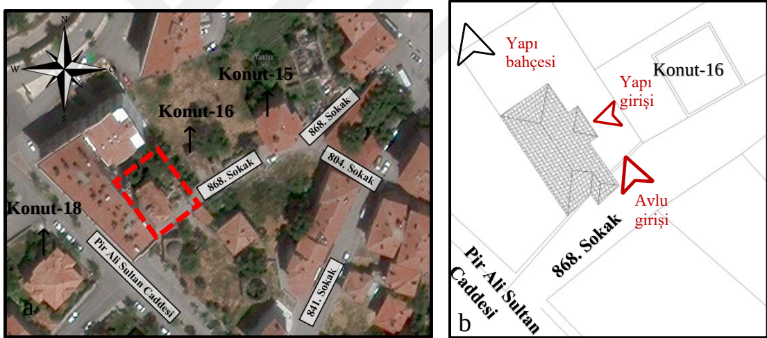
Şekil 4.177. a) Yapi konumu (Yandex Maps görüntüsü üstüne işlenmiştir.), b) yapı vaziyet planı
