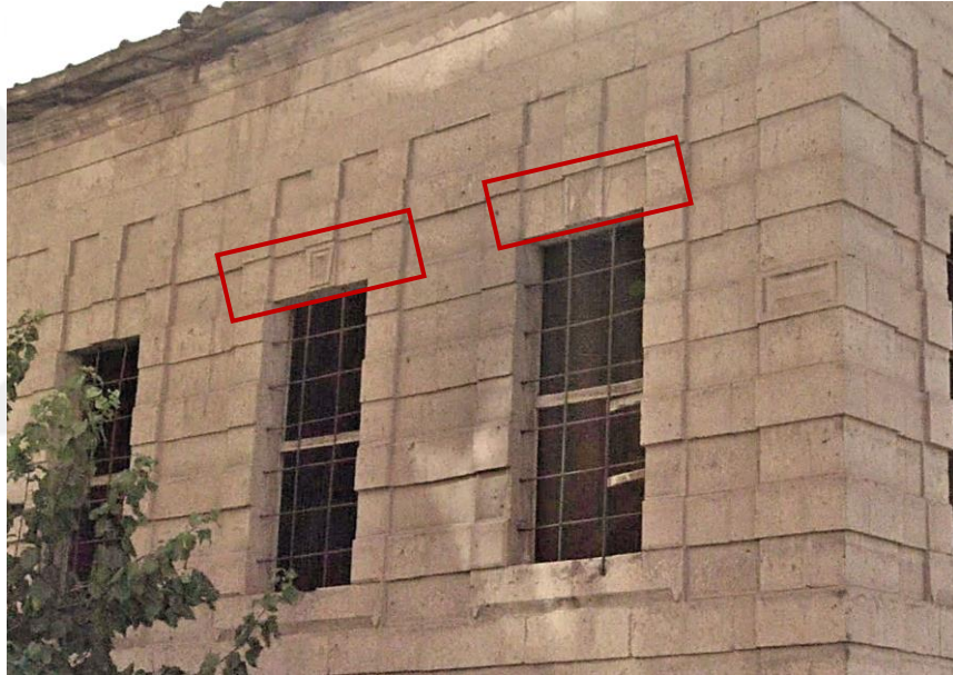
Şekil 4.209. Pencere lentosundaki taş bezemeler
