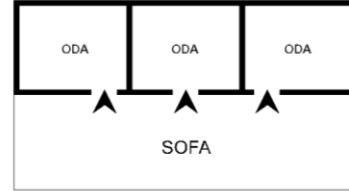
Şekil 3.3. Dış sofalı plan tipi
