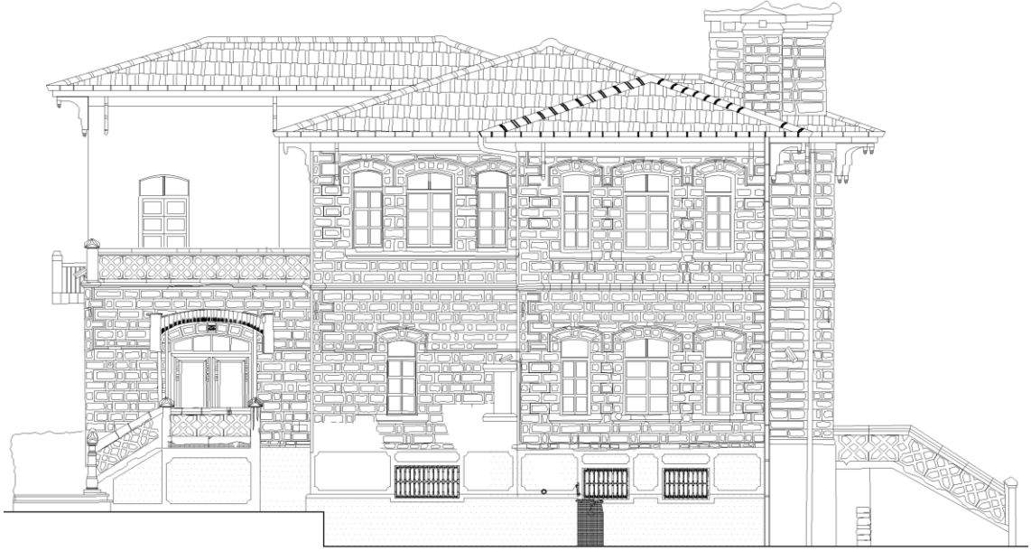
Şekil 4.106. Konut-8 kuzey cephe rölöve çizimi (Mutlu arşivinden düzenlenmiştir.)
