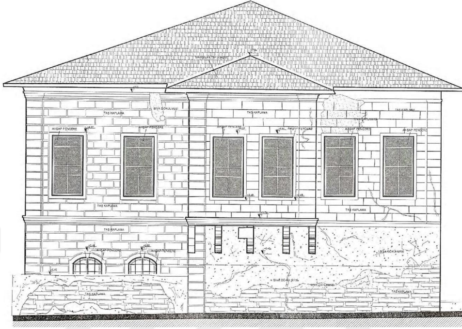
Şekil 4.192. Konut-18 doğu cephe rölöve çizimi (Karadayı Yenice, 2012)
