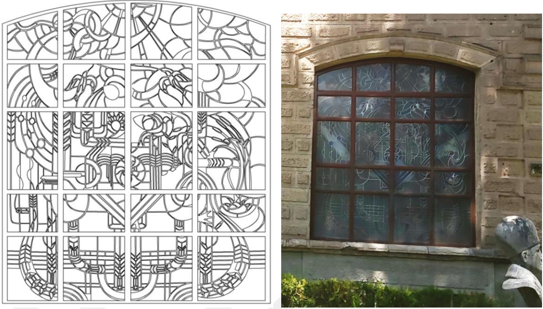
Şekil 5.52. Konut-8 cephesindeki vitray deseni detayı (Mutlu arşivinden düzenlenmiştir.) ve görünüşü
