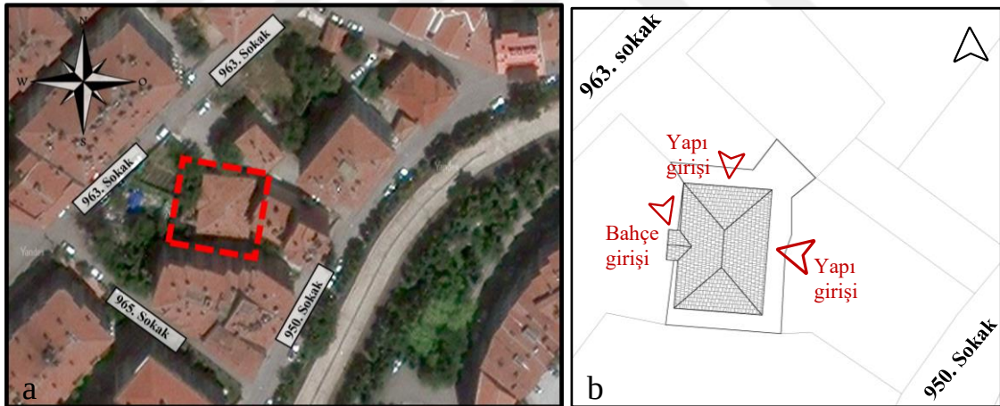
Şekil 4.85. a) Yapı konumu (Yandex Maps görüntüsü üstüne işlenmiştir.), b) yapı vaziyet planı
