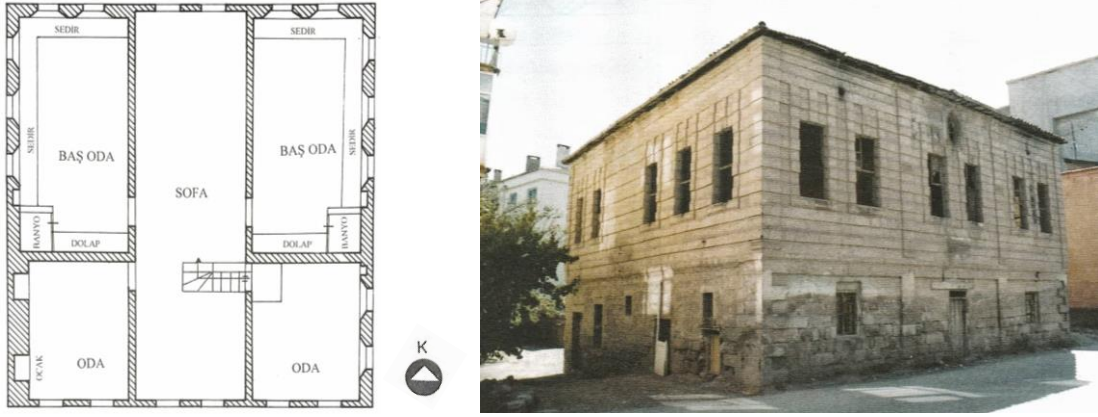
Şekil 4.204. Konut-20'nin birinci kat planı ve genel görünüşü (Erdal, 2016)
