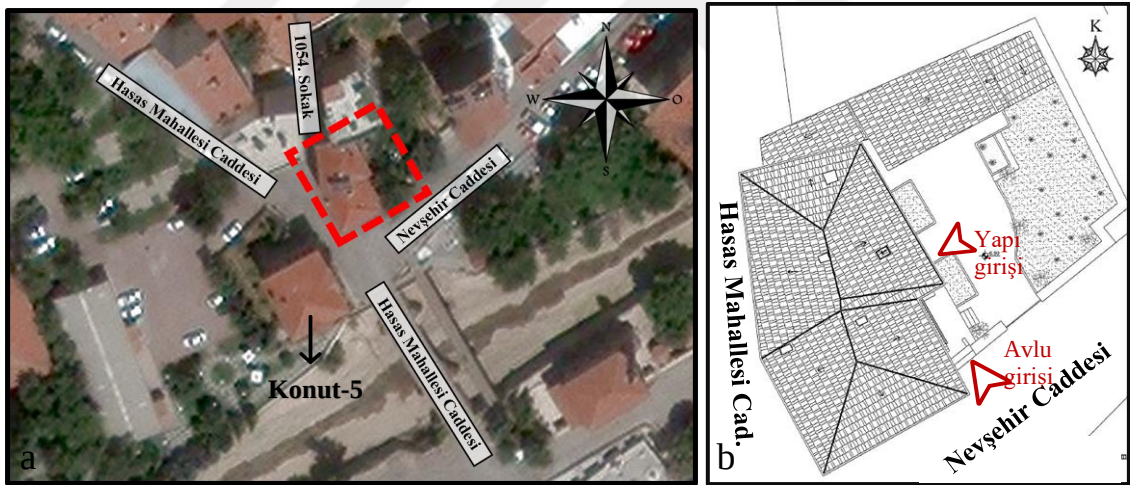
Şekil 4.44. a) Yapı konumu (Yandex Maps görüntüsü üstüne işlenmiştir.), b) Konut-1 rölöve vaziyet planı (Karadayı Yenice, 2012)
