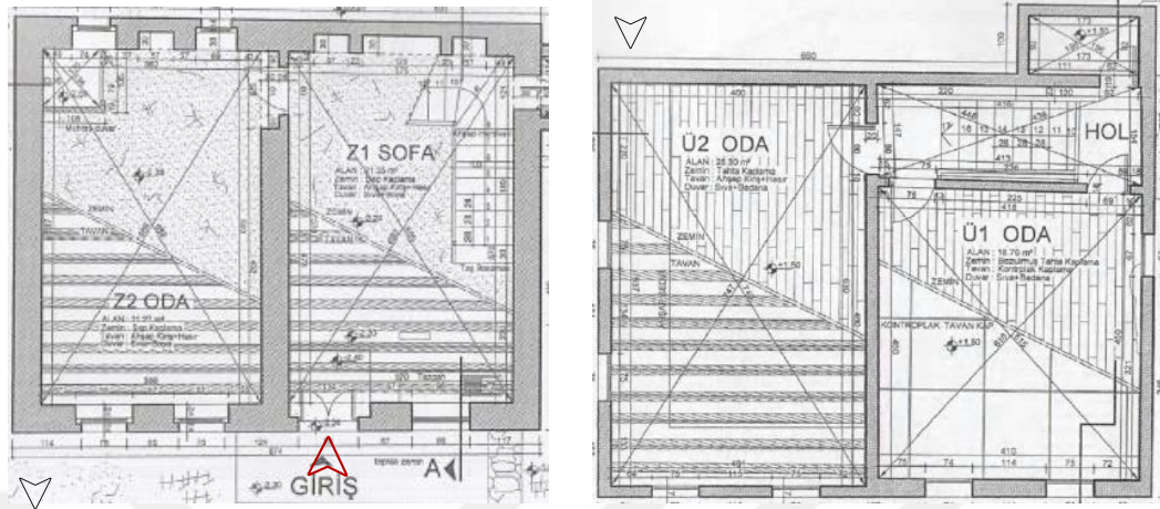
Şekil 4.196. Konut-19 zemin kat (solda) ve birinci kat (sağda) planı rölöve çizimi (Karadayı Yenice, 2012)
