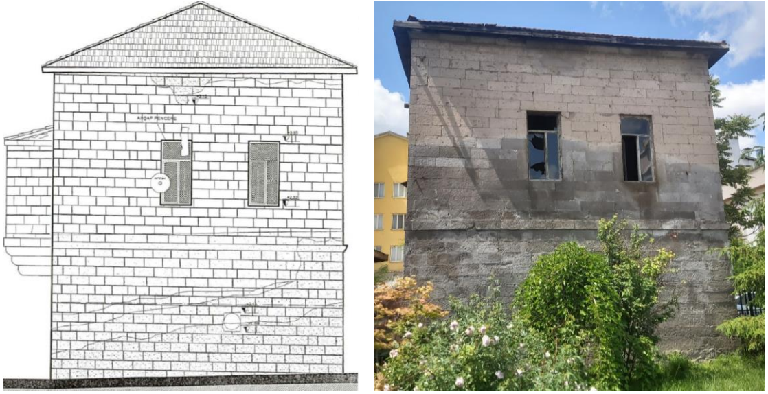
Şekil 4.199. Konut-19 doğu cephe rölöve çizimi (Karadayı Yenice, 2012) ve cephe görünüşü
