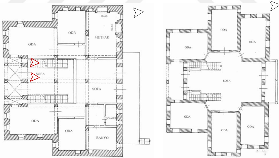
Şekil 4.183. Konut-18 zemin kat (solda) ve birinci kat (sağda) planı rölöve çizimi (Erdal, 2016)
