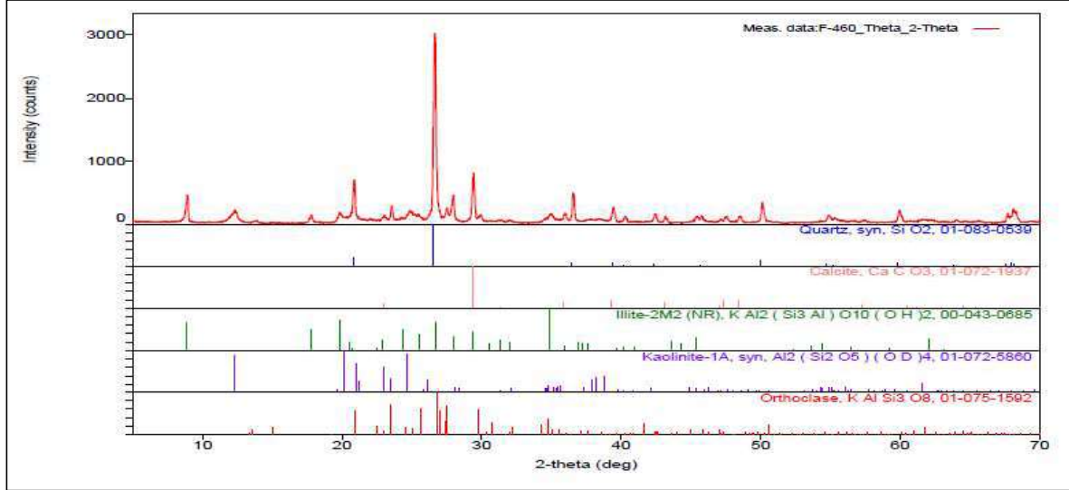
Şekil 6.12. DK-D Duvar Karo bünyesinin (%10 FPA-1 atıklı) XRD analizi
