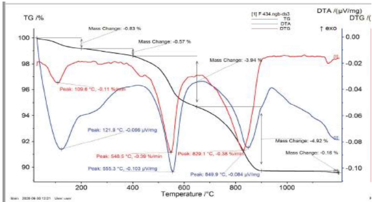
Şekil 6.14 DK-D bünye granülü TG-DTA analizi
