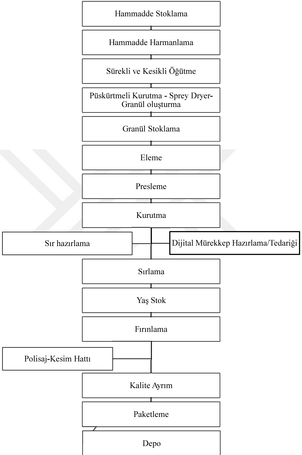
Şekil 2.1. Seramik Karo Üretim Aşamaları
