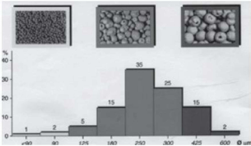
Şekil 2.9. Püskürtmeli kurutucu tane boyut dağılımına karşı farklı boyutlardaki taneciklerin morfolojik görünüşleri (Anonim, 2002a)
