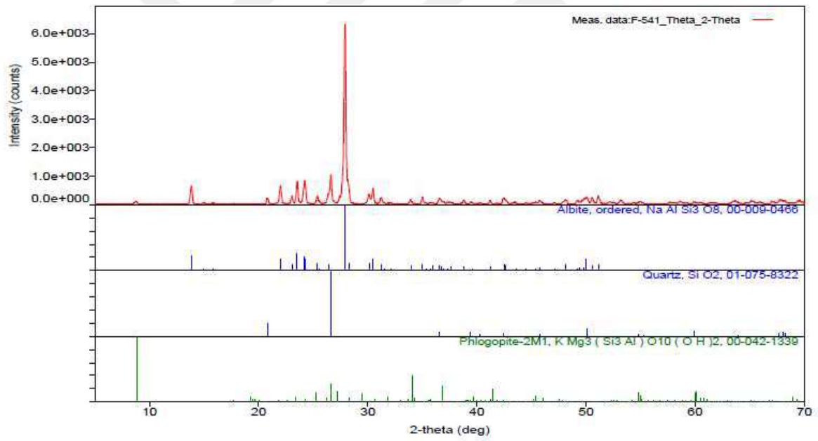
Şekil 6.10 Çine Feldspat XRD Analizi
