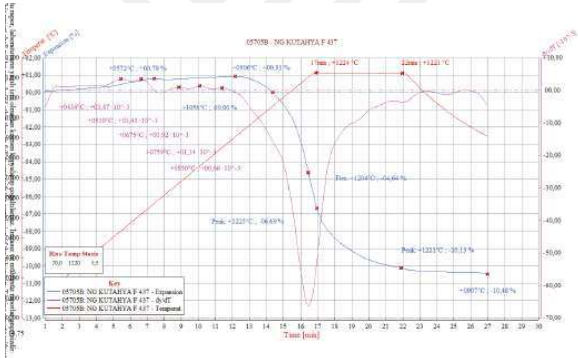
Şekil 6.17 YK-03 bünye granülü optik dilatometre analizi (Tepe sıcaklığında kalma süresi 5,5 dakika)
