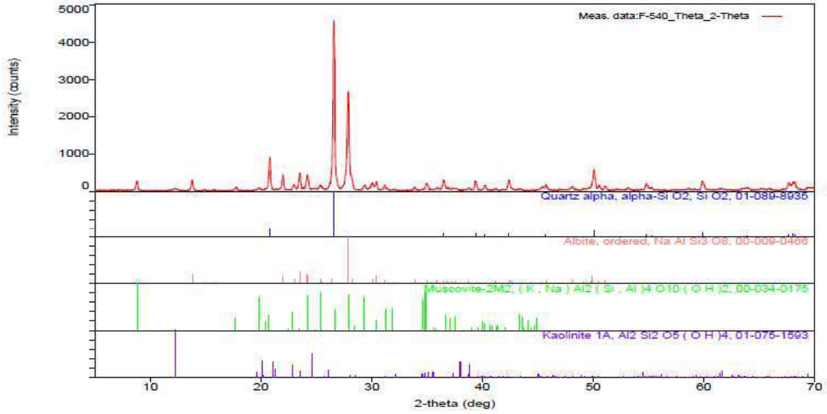
Şekil 6.8. Söğüt Feldspat 1 XRD Analizi
