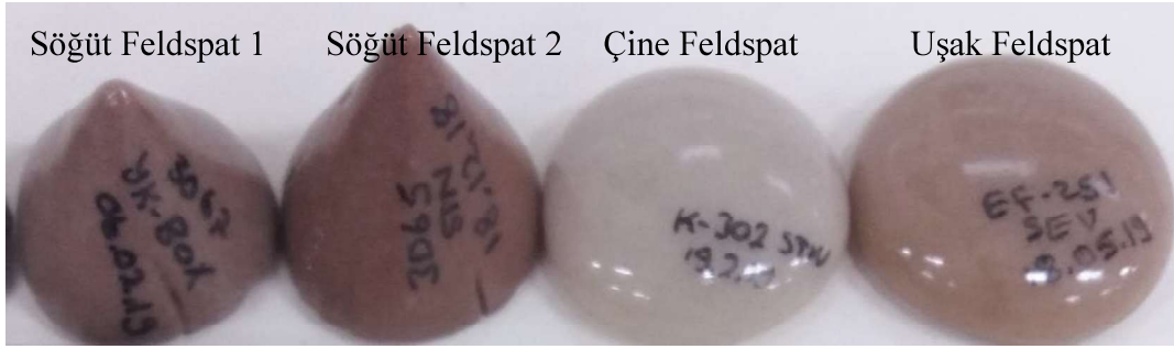
Şekil 6.7. Feldspatların Koni Testleri
