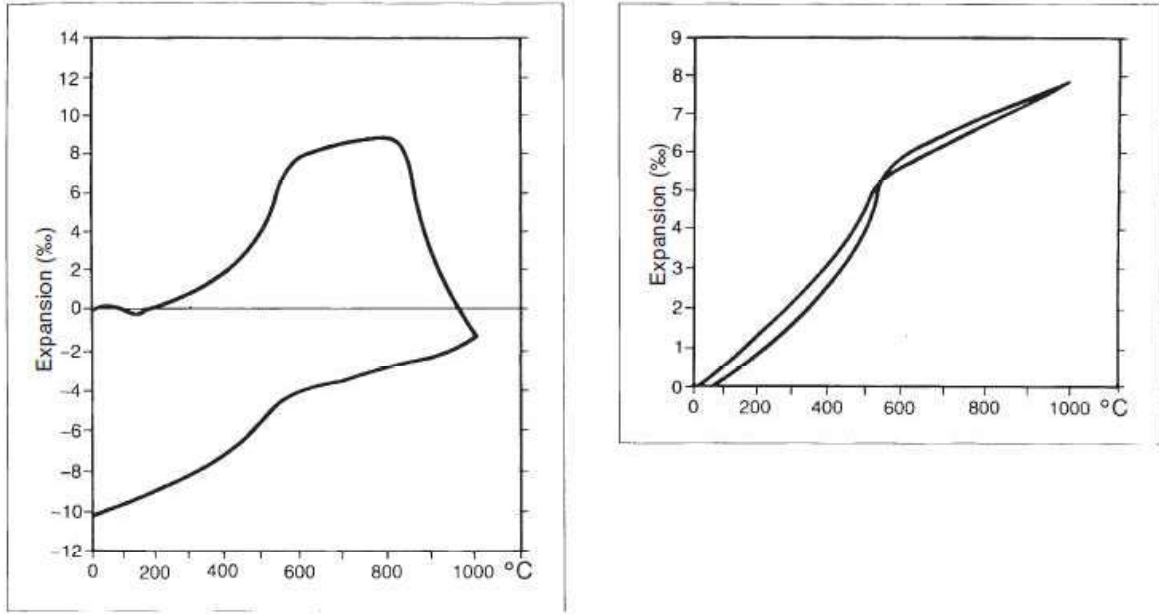
Şekil 2.17. Pişmiş ve pişmemiş karoların ısı işlem boyunca genleşme eğrileri
