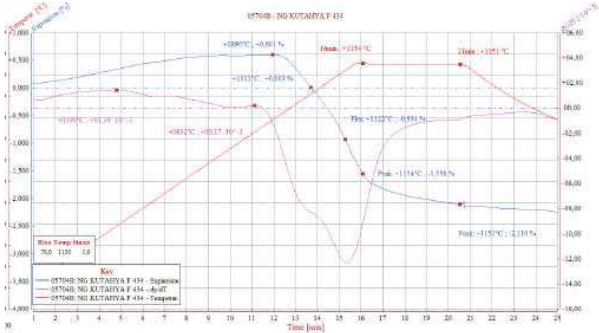
Şekil 6.15 DK-D bünye granülü optik dilatometre analizi
