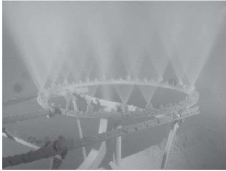
Şekil 2.8. Püskürtmeli kurutucu nozzle halkası görünümü (Anonim, 2002a)
