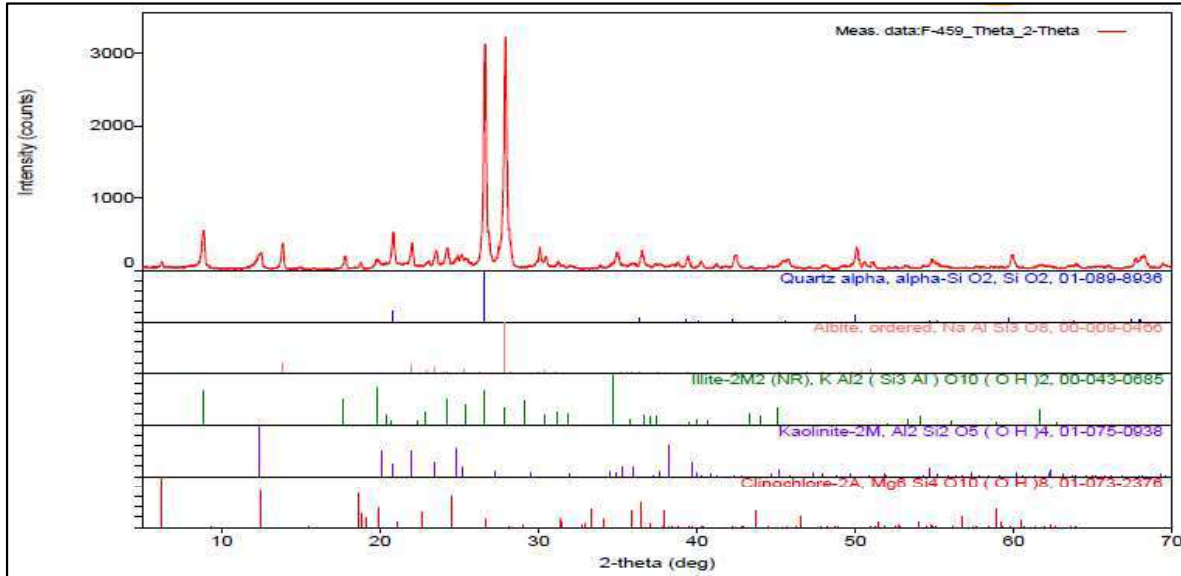
Şekil 6.13. YK-03 Sırlı Porselen bünyesinin (%12 FPA-1+%6 FPA-2 atıklı) XRD analizi
