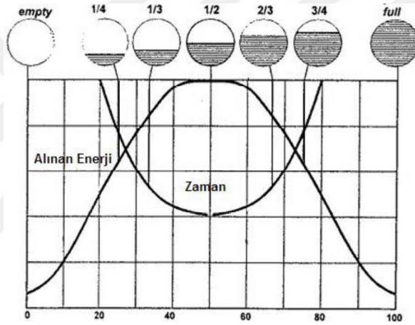
Şekil 2.5. Öğütme zamanına bağlı enerji ve değirmen doluluk oran fonksiyonu
