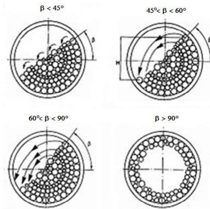
 ekil 2.4. De irmen D n   Hızı ile    tme Ta larının Hareket A ısı
