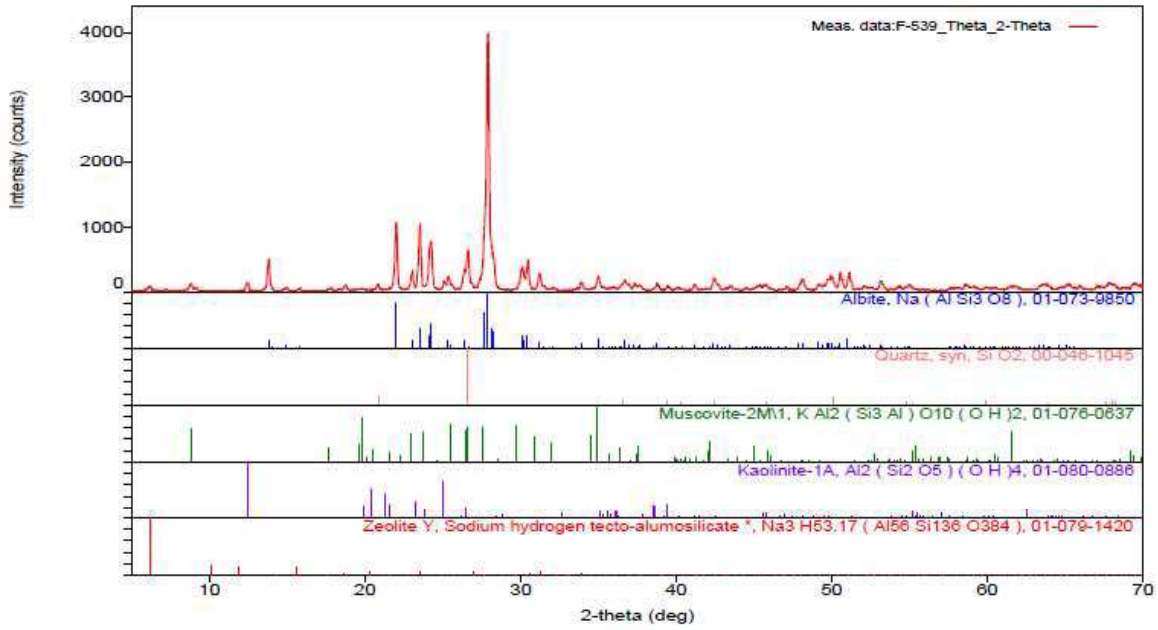
Şekil 6.11 Uşak Feldspat XRD Analizi
