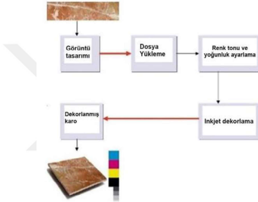
Şekil 2.15. Dijital mürekkep baskı uygulaması akış şeması (Varışlı, 2019)
