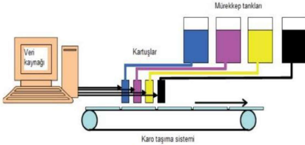
Şekil 2.16. Sırlama bantında dijital mürekkep baskı uygulama sistemi (Varışlı, 2019)
