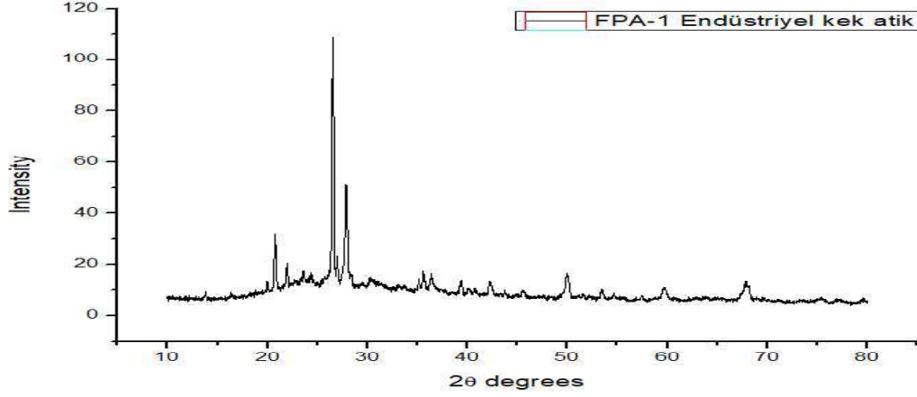
Şekil 6.4 FPA-1 Endüstriyel Kek Atık XRD
