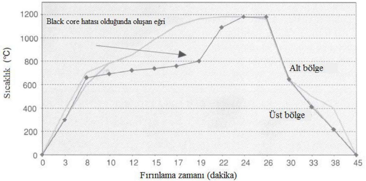
Şekil 2.18. Hızlı tek pişirim rejim döngüsü (Anonim, 2002b)
