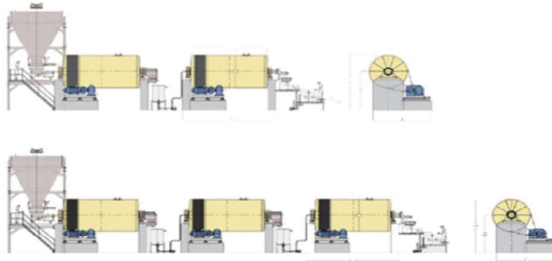
Şekil 2.3. Sıralı Sürekli (Continue) Öğütme Sistemleri (Anonim,2012)
