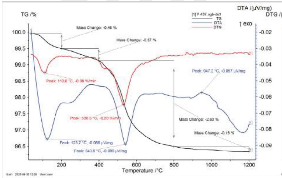
Şekil 6.16 YK-03 bünye granülü TG-DTA analizi
