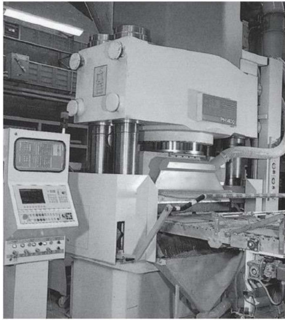
Şekil 2.10. Hidrolik Pres örneği (Anonim, 2002a)
