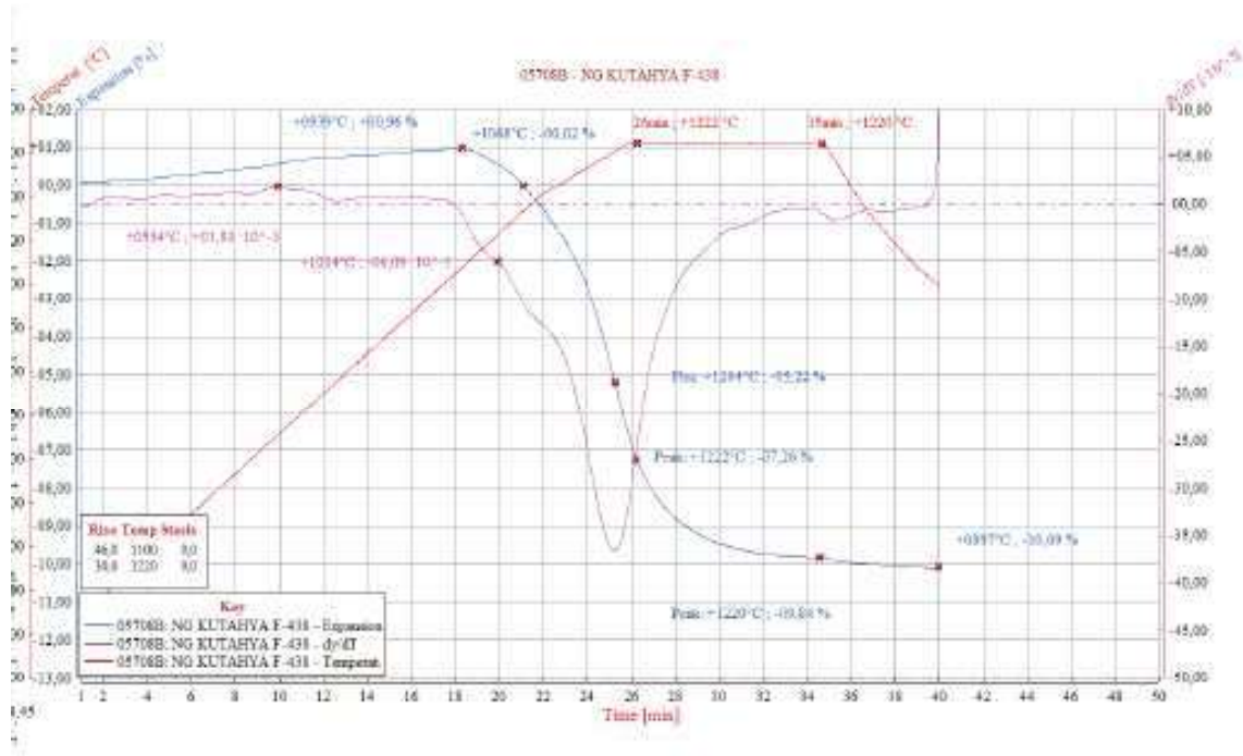
Şekil 6.18 YK-03 bünye granülü optik dilatometre analizi (Tepe sıcaklığında kalma süresi 9 dakika)
