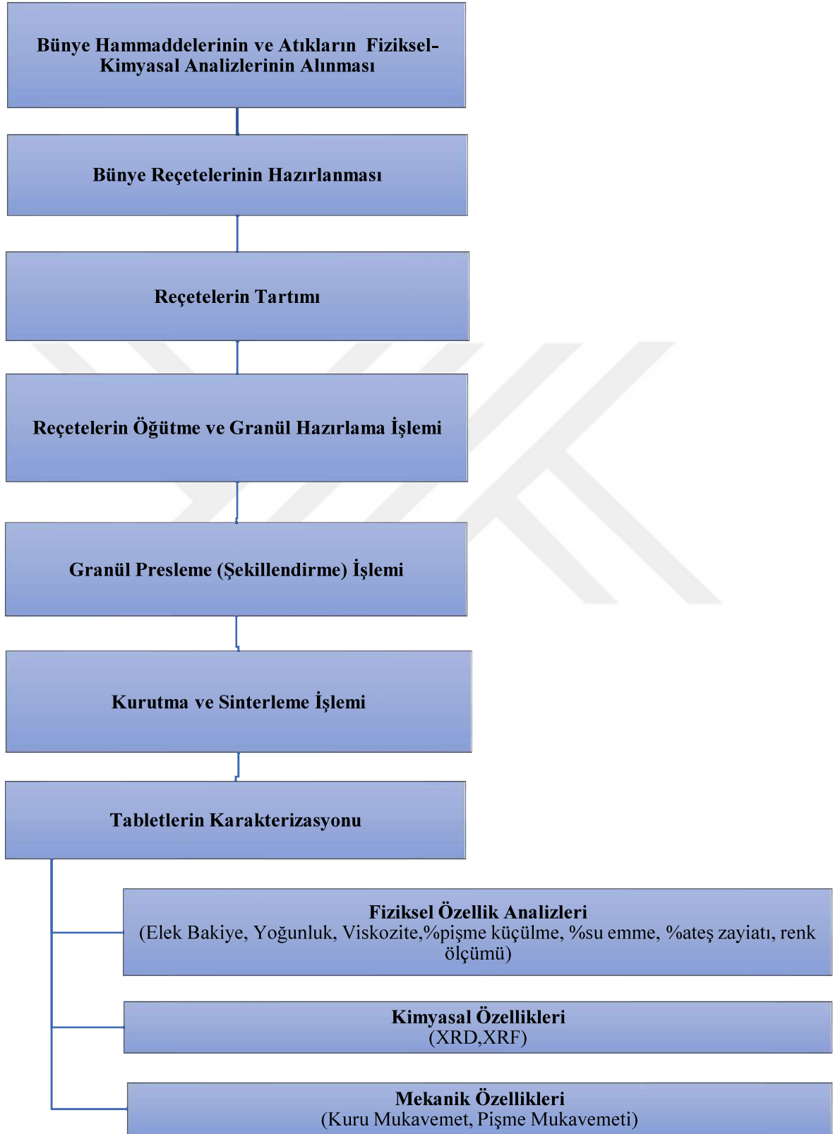
Şekil 5.1. Deneysel Çalışmalara Ait İşlemlerin Akış Şeması
