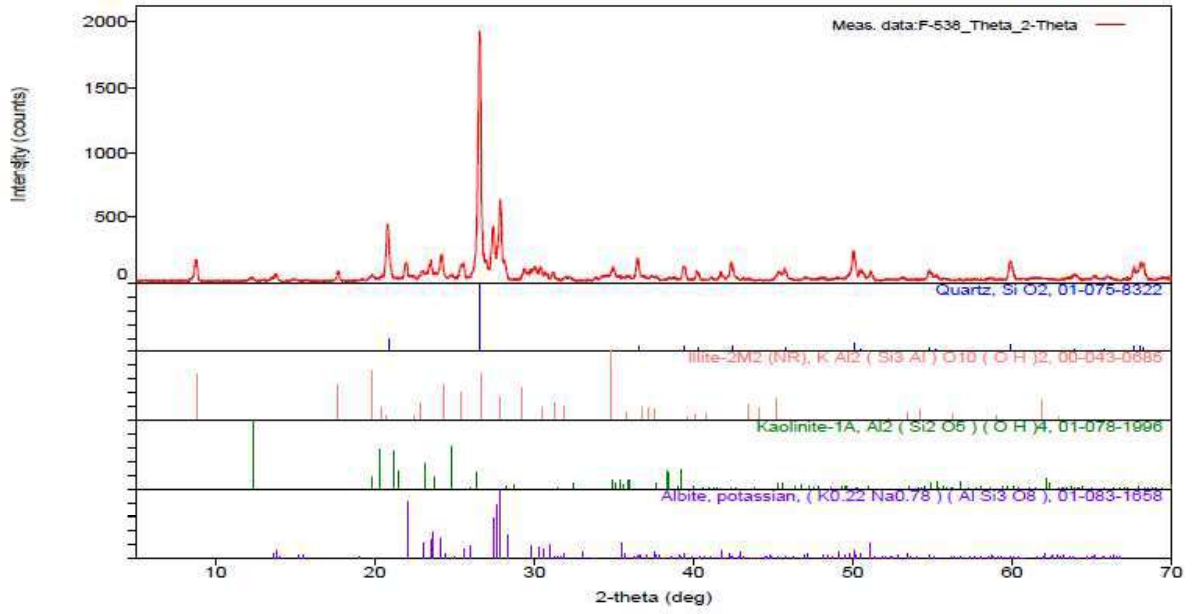
Şekil 6.9 Söğüt Feldspat 2 XRD Analizi
