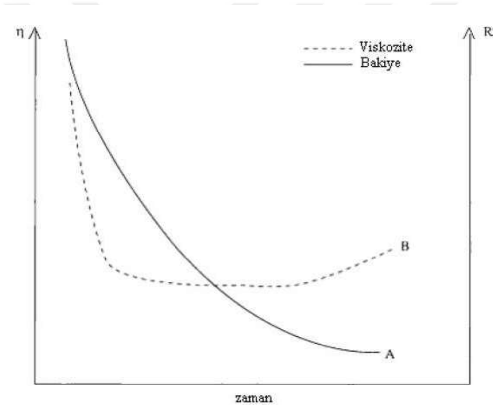
Şekil 2.6. Öğütme Sürecinde Elek bakiye-viskozite ve zaman ilişkisi
