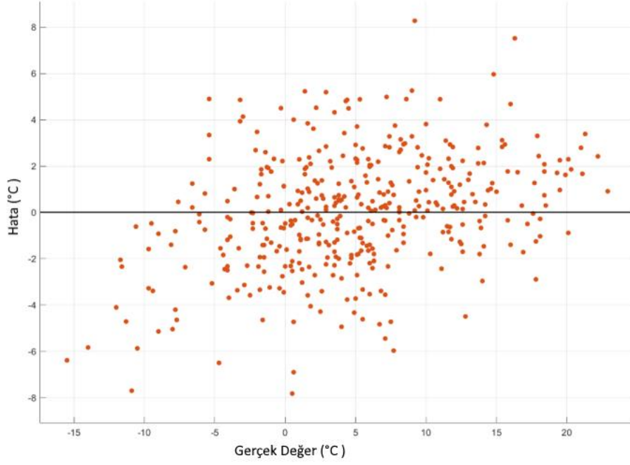
Şekil 6.33 Eğitim-11 Sonucu Elde Edilen Hata Grafiği
