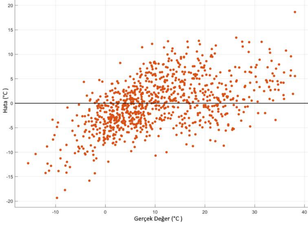
Şekil 6.21 Eğitim-7 Sonucu Elde Edilen Hata Grafiği
