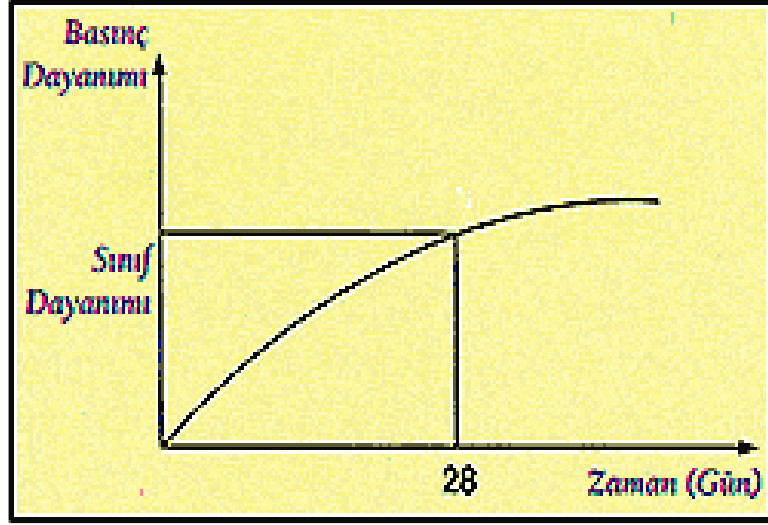
Şekil 3.4 Basınç dayanımı-Zaman İlişkisi (Hasan 2006).
