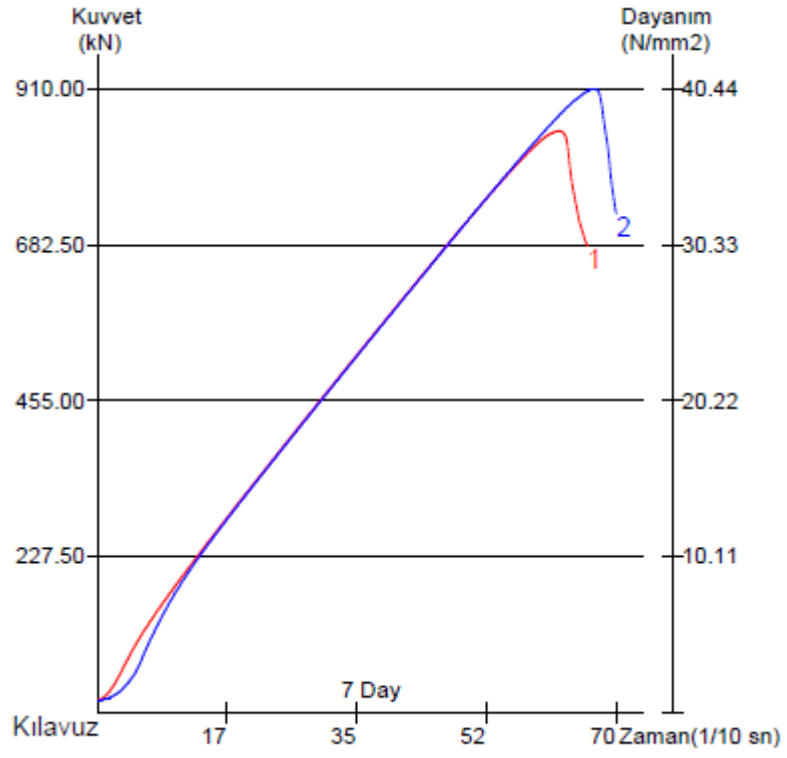
Şekil 5.1 3gün boyunca sertleşme saf (Cüruf 0 %)
