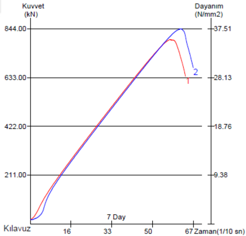
Şekil 5.4 7gün boyunca sertleşme saf (Cüruf 0 %)
