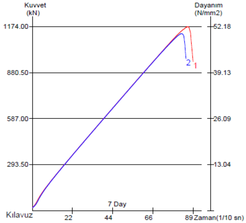
Şekil 5.7 28gün boyunca sertleşme saf (Cüruf 0 %)
