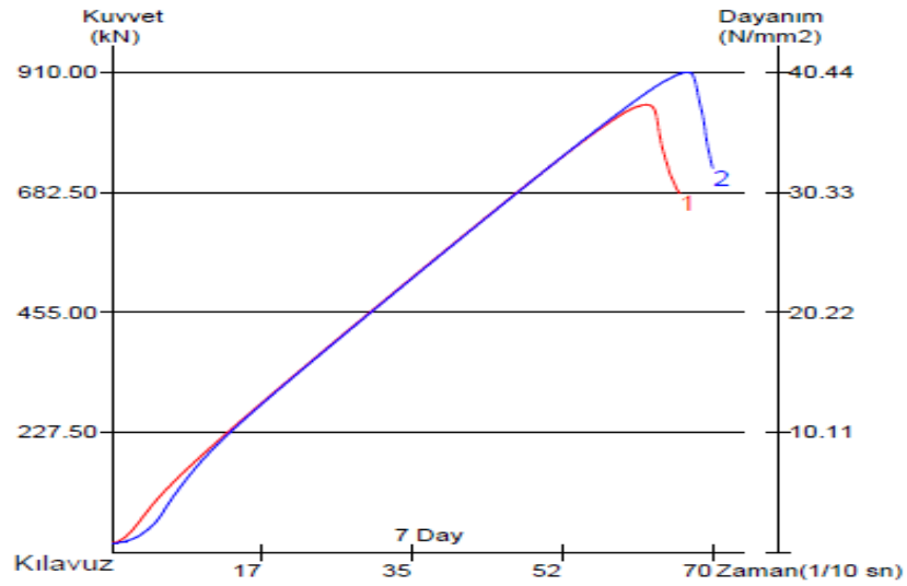
Şekil 5.5 7gün boyunca sertleşme (Cüruf 10%)
