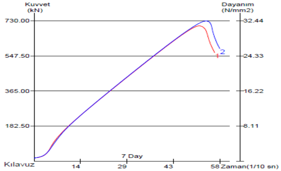
Şekil 5.3 3gün boyunca sertleşme (Cüruf 15 %)
