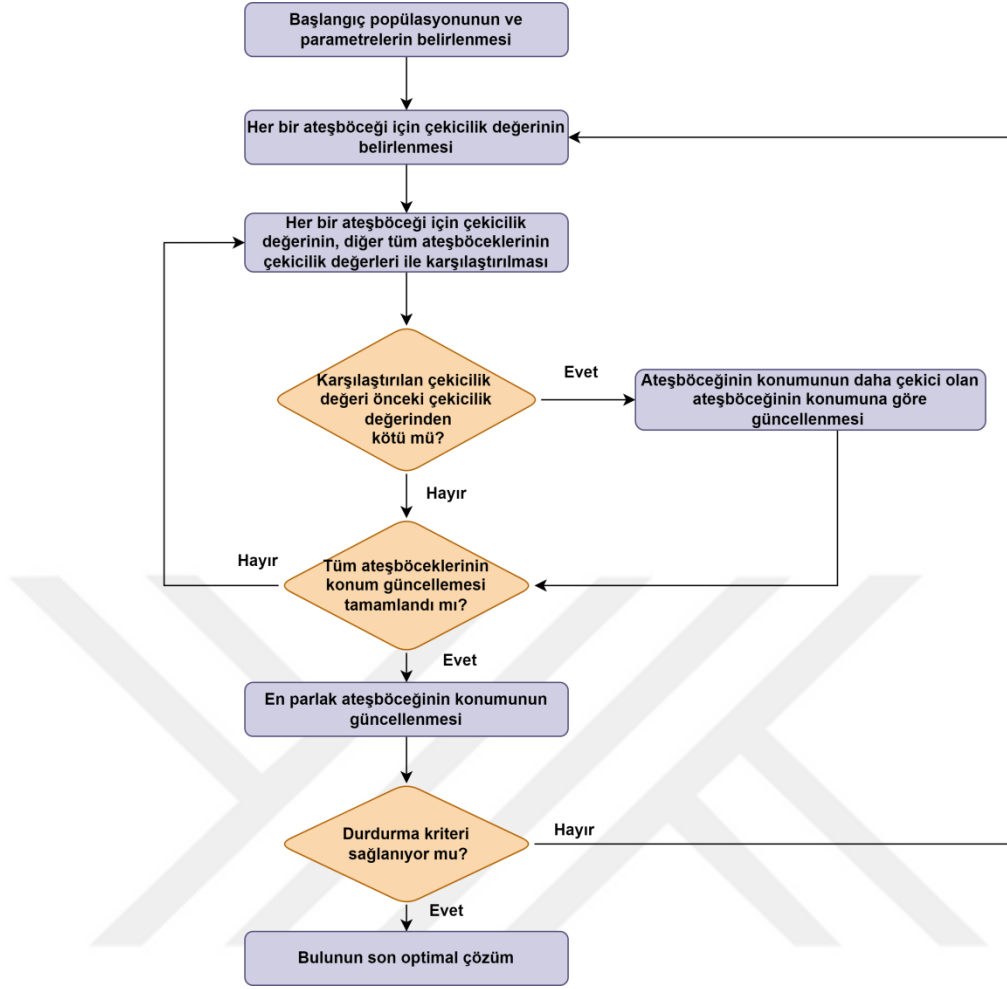
Şekil 3.8. FA Akış Diyagramı
