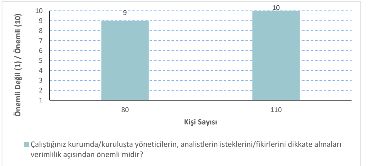
Şekil 5.13. Hipotez 11 grafiği.
