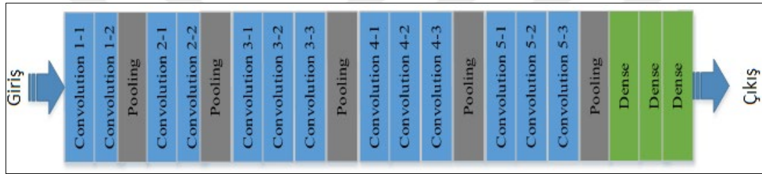
Şekil 3.3. VGGNet-16 mimarisi
