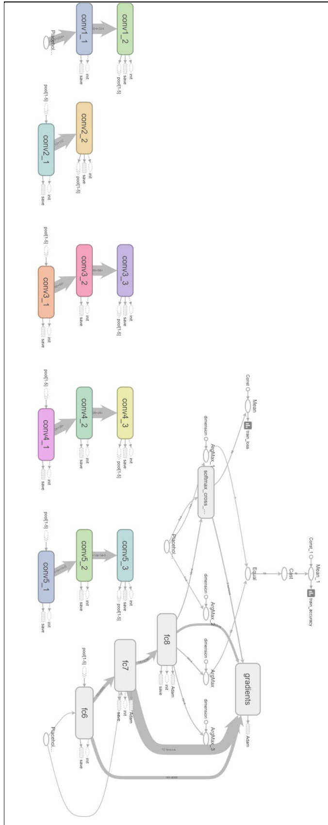
Şekil 1.1. VGGNet-16 ağı
