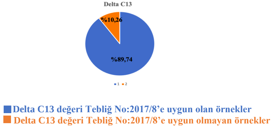
Şekil 26 Örneklerin Delta C13 analiz sonuçlarının Tebliğ No:2017/8'e % uygunluk değerlendirmesi
