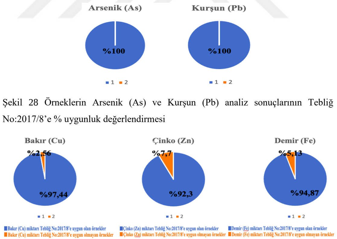
Şekil 29 Örneklerin Bakır (Cu), Çinko (Zn) ve Demir (Fe) analiz sonuçlarının Tebliğ No:2017/8'e % uygunluk değerlendirmesi
