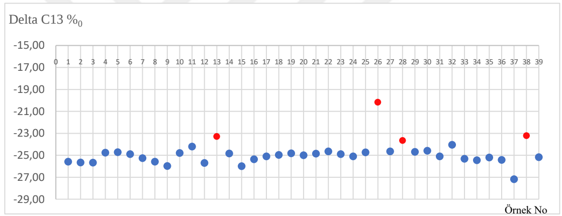
Şekil 27 Örneklerin Delta C13 (‰) değerlerini gösteren grafik
