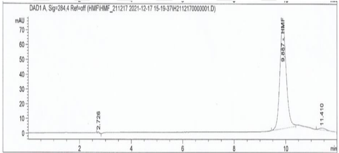
Şekil 20 10 ppm konsantrasyonundaki HMF standartının kromatogram görüntüsü
