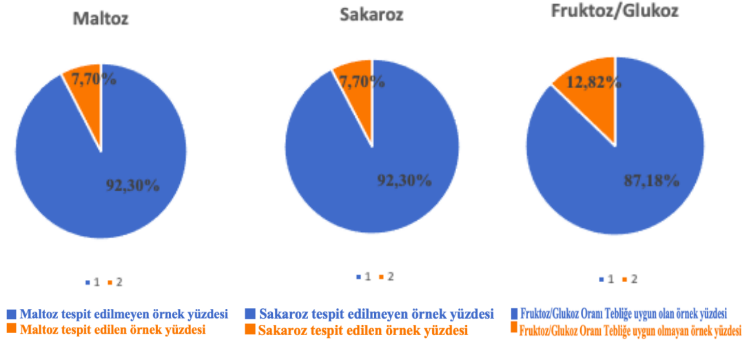
Şekil 21 Şeker Bileşenleri analiz sonuçlarının Tebliğ No:2017/8'e % uygunluk değerlendirmesi
