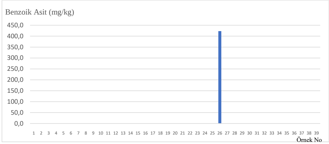
Şekil 40 Benzoik asit analiz sonuçlarını gösteren grafik
