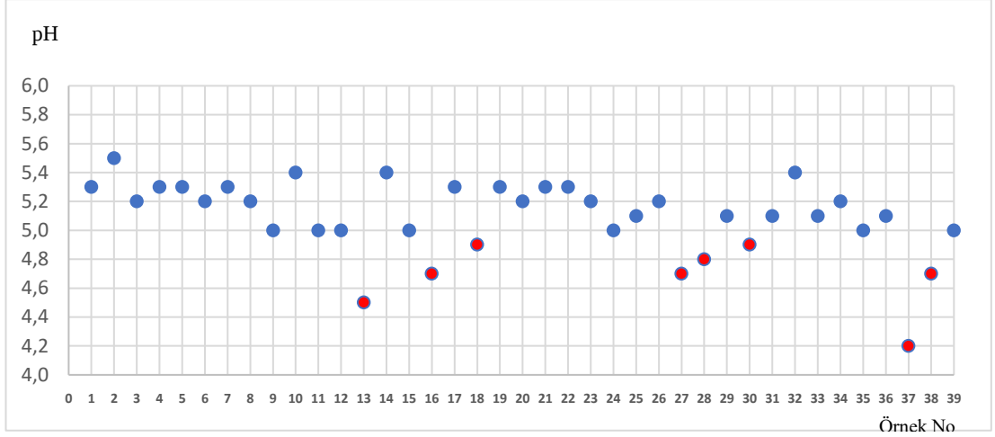
Şekil 13 Örneklerin pH değerlerini gösteren grafik
