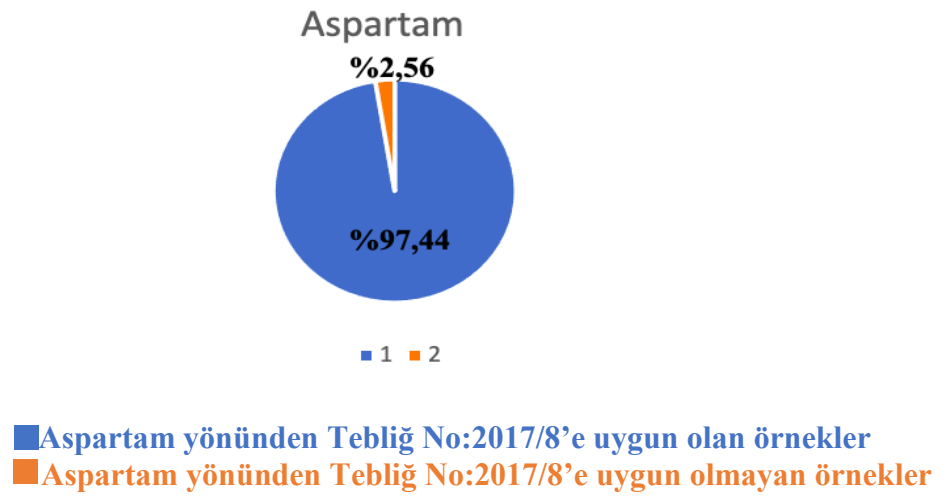
Şekil 44 Aspartam analiz sonuçlarının % uygunluk değerleri
