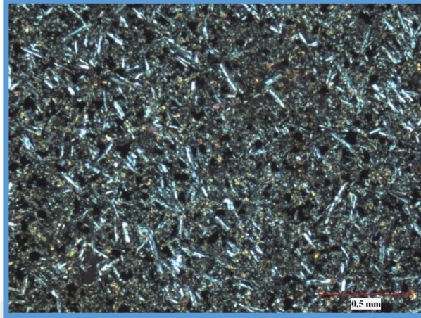
Şekil 3.12. Örnek AS2; çift nikol, hamurda bulunan plajiyoklaz ve olivin mineralleri.
