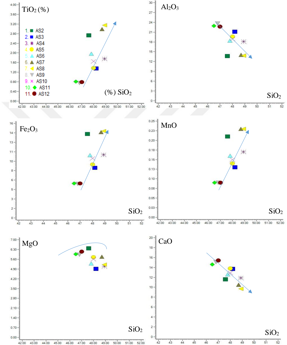
Şekil 3.17. Asal-Ghoubet volkanik kayaçlarının Harker major element diyagramları (TiO 2 , Al 2 O 3 , Fe 2 O 3 , MnO, MgO, CaO – SiO 2 ).
