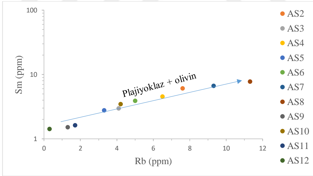
Şekil 4.3. Asal-Ghoubet alanındaki volkanik kayaların Sm - Rb log-log diyagramı.
