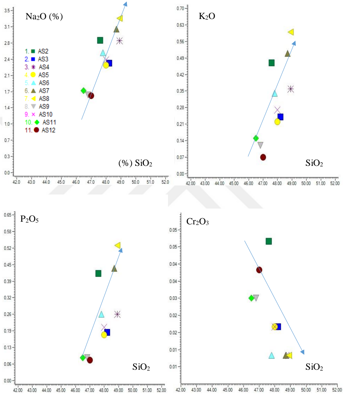
Şekil 3.18. Asal-Ghoubet volkanik kayaların Harker major element diyagramlarına göre değerlendirilmesi (Na 2 O, K 2 O, P 2 O 5 , Cr 2 O 3 – SiO 2 ).
