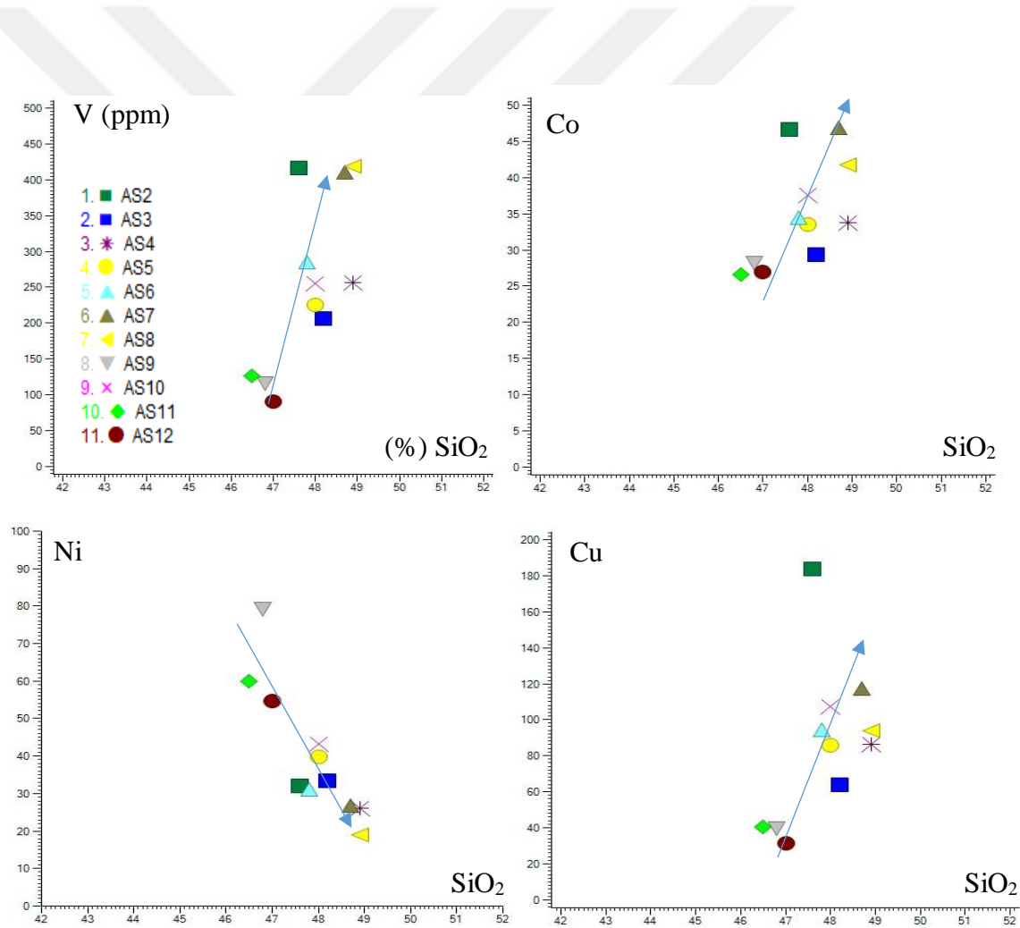
Şekil 3.19. Asal-Ghoubet volkanik kayalarının Harker iz elementler diyagramlarına göre değerlendirilmesi (V, Co, Ni, Cu – \text{SiO}_2 ).
