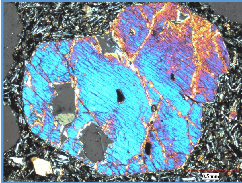
Şekil 3.10. Örnek AS10; çift nikol: iri taneli olivin ve mikrolitik plajiyoklazlar bulunmaktadır.
