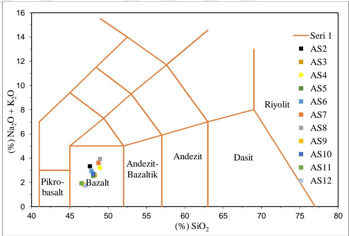
Şekil 3.13. Le Bas vd. (1986)'nin toplam alkali - SiO 2 diyagramında Asal-Ghoubet volkanik kayalarının konumu.
