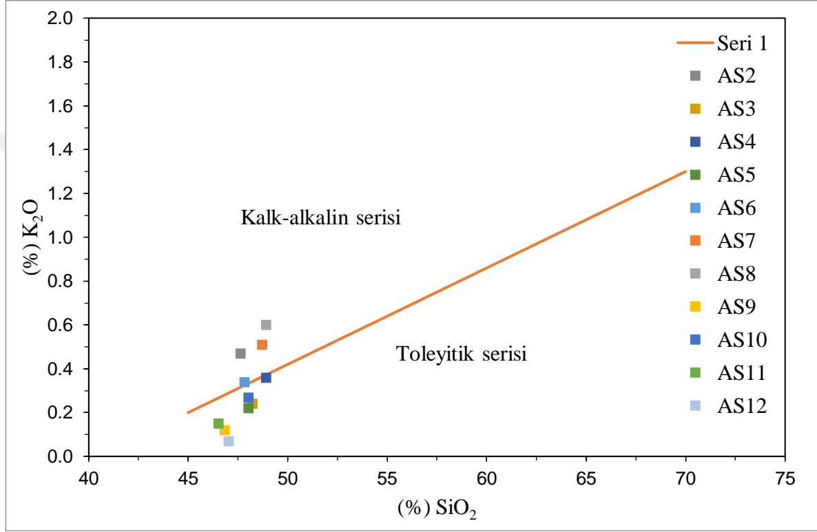
Şekil 3.15. Asal-Ghoubet volkanik kayalarının K_2O - SiO_2 diyagramına göre sınıflandırılması (Peccerilo ve Taylor 1976).
