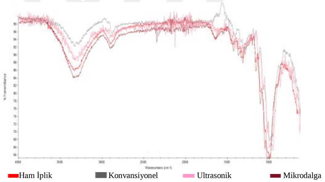
Şekil 33: 10 g/L NaOH ile Konvansiyonel, Ultrasonik, Mikrodalga Yöntemleriyle yüzey işlemi uygulanan Isırgan İpliğinin FTIR analizi
