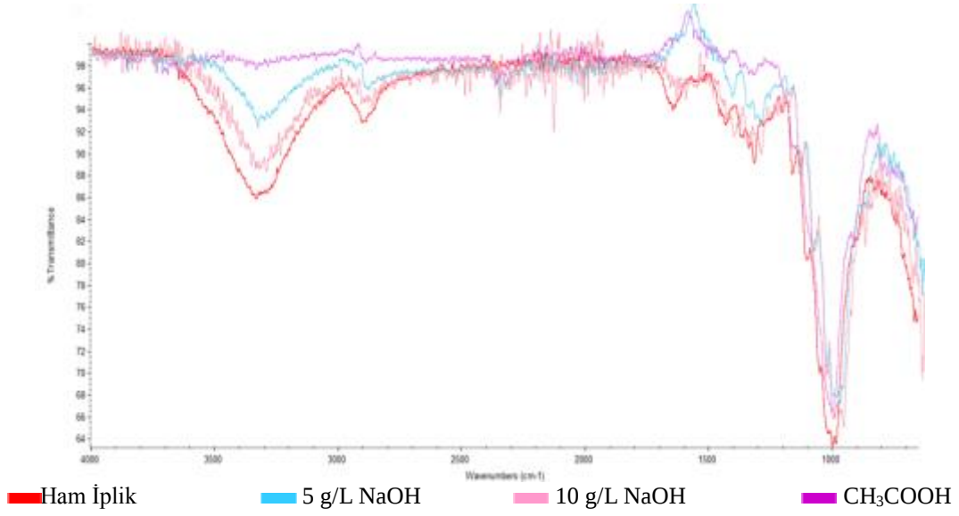
Şekil 30: Ultrasonik enerji yöntemiyle yüzey işleme uygulanan ısrıgan ipliđinin FTIR analizi
