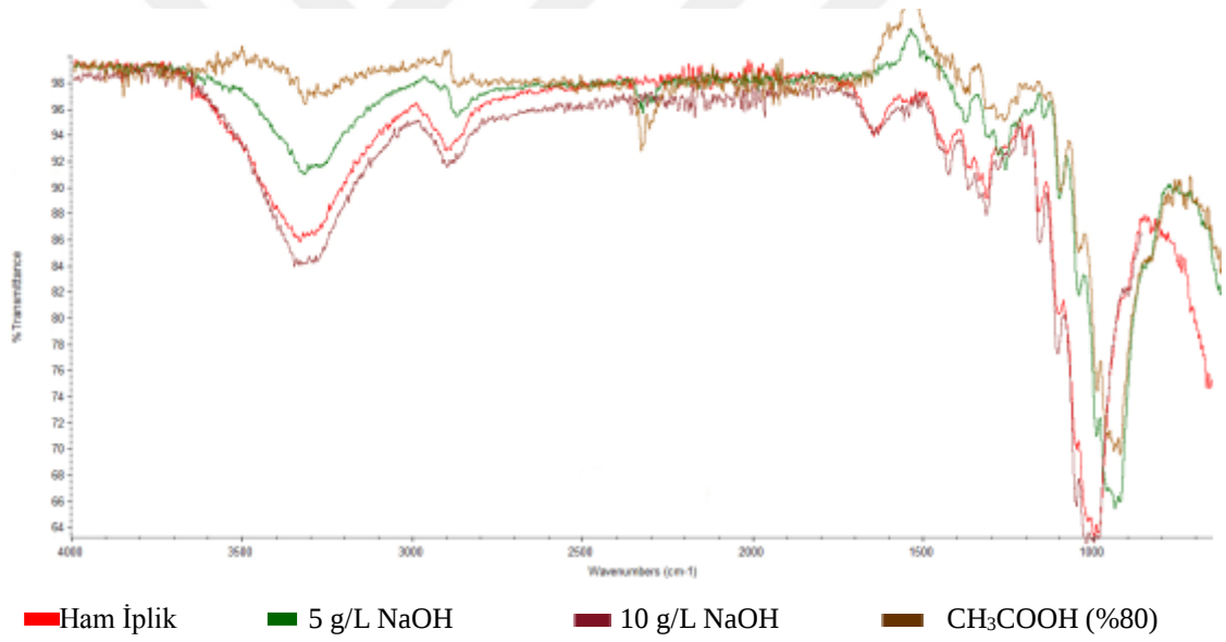
Şekil 31: Mikrodalga yöntemiyle yüzey işleme uygulanan ısrıgan ipliđinin FTIR analizi.
