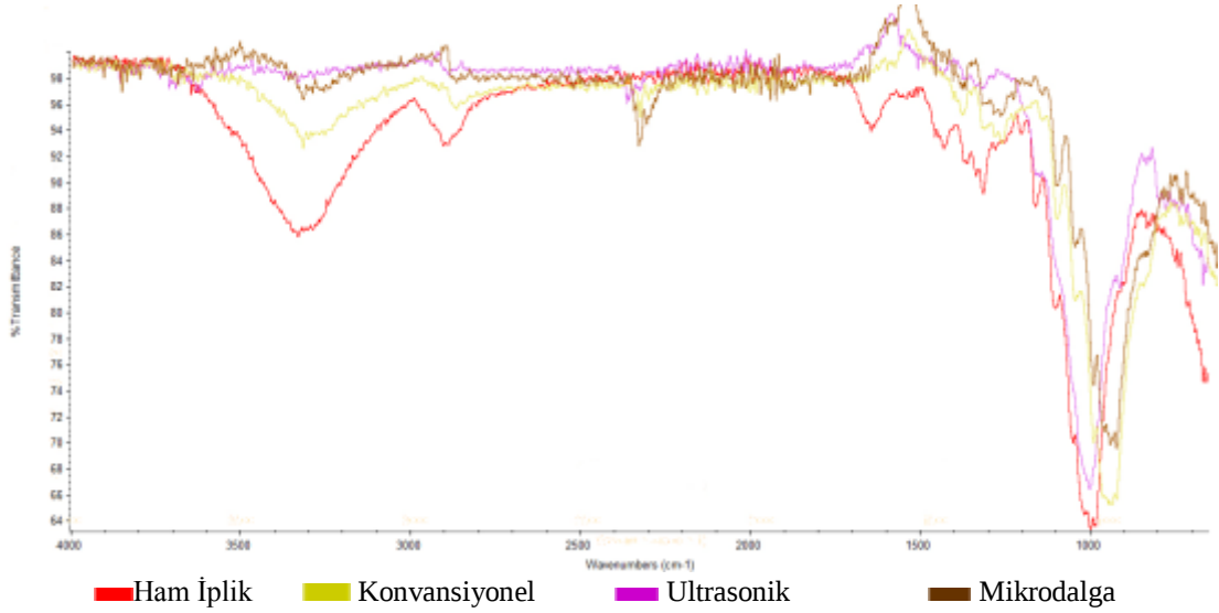
Şekil 34: CH 3 COOH (%80) ile Konvansiyonel, Ultrasonik, Mikrodalga Yöntemleriyle yüzey işleme uygulanan ısırgan ipliğinin FTIR analizi
