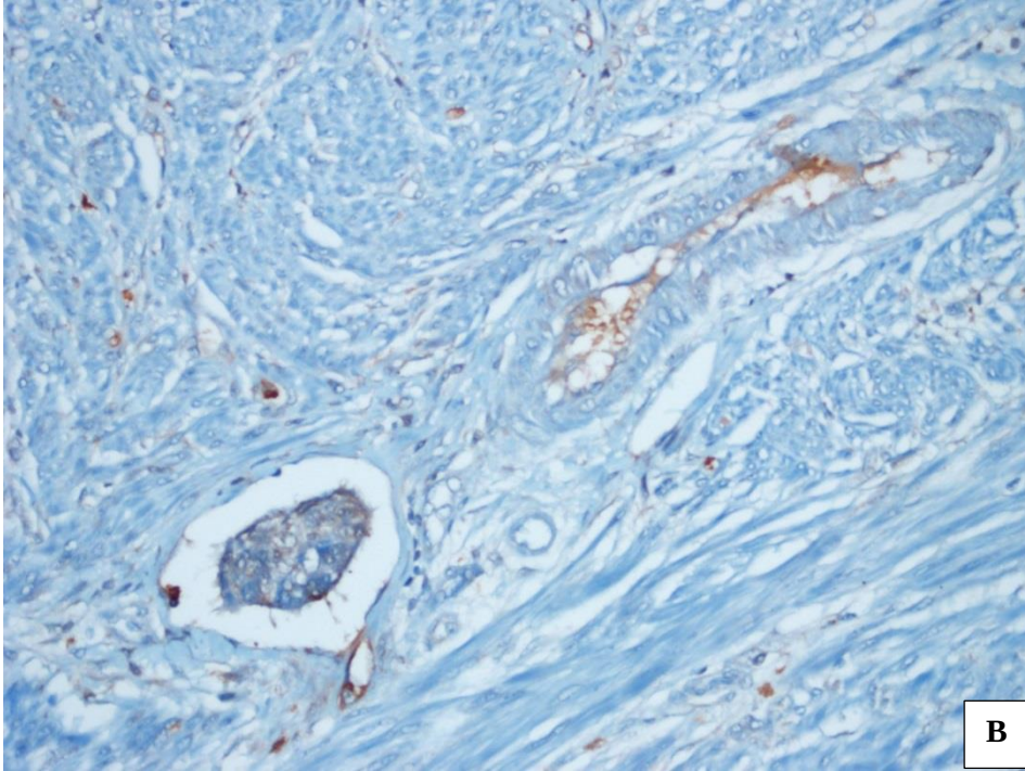
Şekil 4.2. Yüksek dereceli endometrioid karsinom, irice bir arterin yanında lenfovasküler invazyon odağı (HE, x100) (A) , aynı olguda yaygın olan lenfovasküler invazyon odaklarından birinde hafif yoğunlukta sitoplazmik MMP9 ekspresyonu (İHK, x200) (B)
