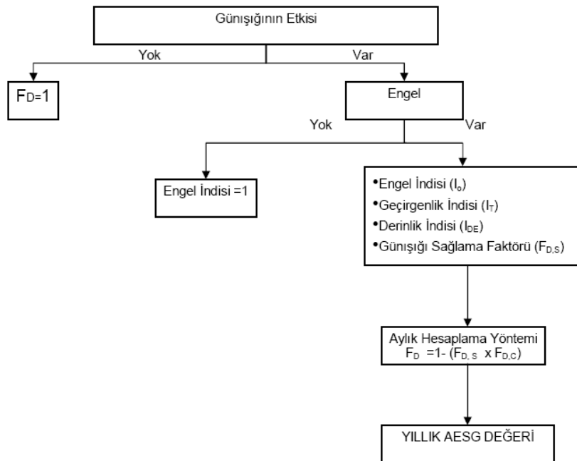
Şekil 3.3. Günişığı bağımlılık faktörünün hesaplanmasına dair akış diyagramı (Anonim, 2010)
