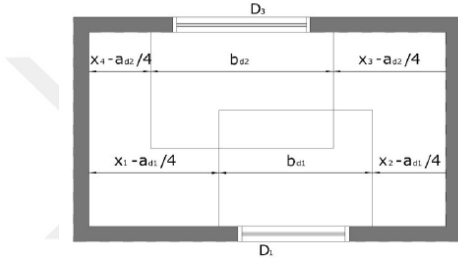
Şekil 3.9. Birinci ve üçüncü duvarlarda birer pencere bulunması durumu
