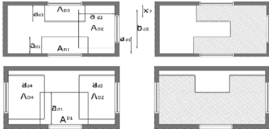
Şekil 3.11. Üç farklı duvarda bir veya birden fazla duvar olması durumu
