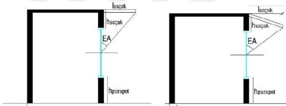
Şekil 3.15. Pencereye dik durumda yatay engel olması durumu (Anonim, 2010)
