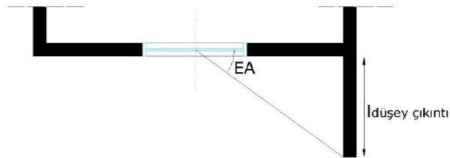
Şekil 3.16. Pencereye dik bir engelin olması durumu
