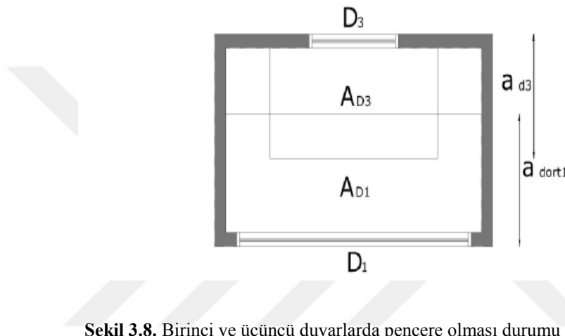
Şekil 3.8. Birinci ve üçüncü duvarlarda pencere olması durumu (Anonymous, 2007)
