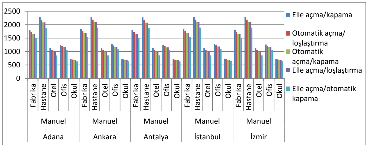
Şekil 4.2. Günışığına bağlı aydınlatma kontrol sisteminin manuel olduğu durum için beş farklı şehir ve bina türünde kontrol sistem senaryolarına bağlı olarak yıllık tüketilen toplam aydınlatma enerjisi miktarları
