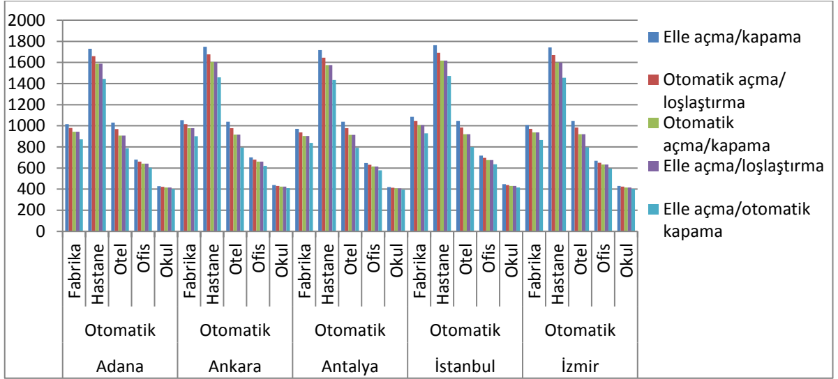
Şekil 4.3. Günişliğine bağlı aydınlatma kontrol sisteminin otomatik olduğu durum için beş farklı şehir ve bina türünde kontrol sistem senaryolarına bağlı olarak yıllık tüketilen toplam aydınlatma enerjisi miktarları
