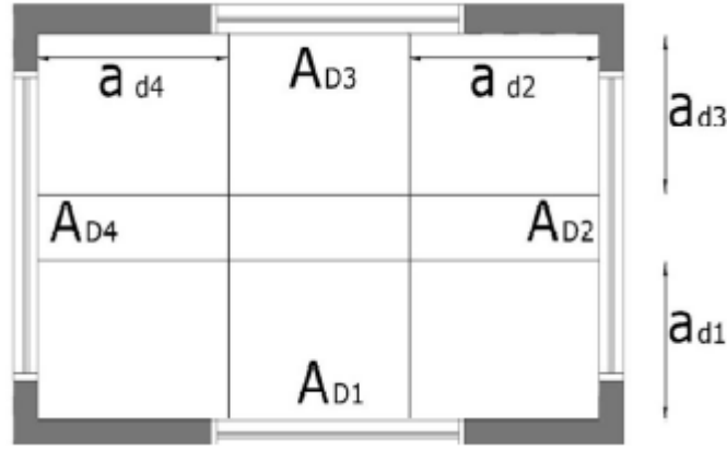
Şekil 3.12. Dört duvarda bir veya birden fazla pencere olması durumu (Anonim, 2010)
