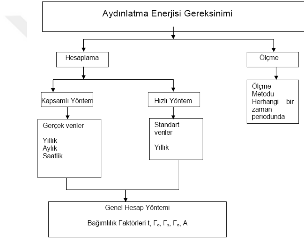
Şekil 3.1. Aydınlatma Enerjisi Gereksinimi Hesaplama Yöntemleri (Anonim,2010)
