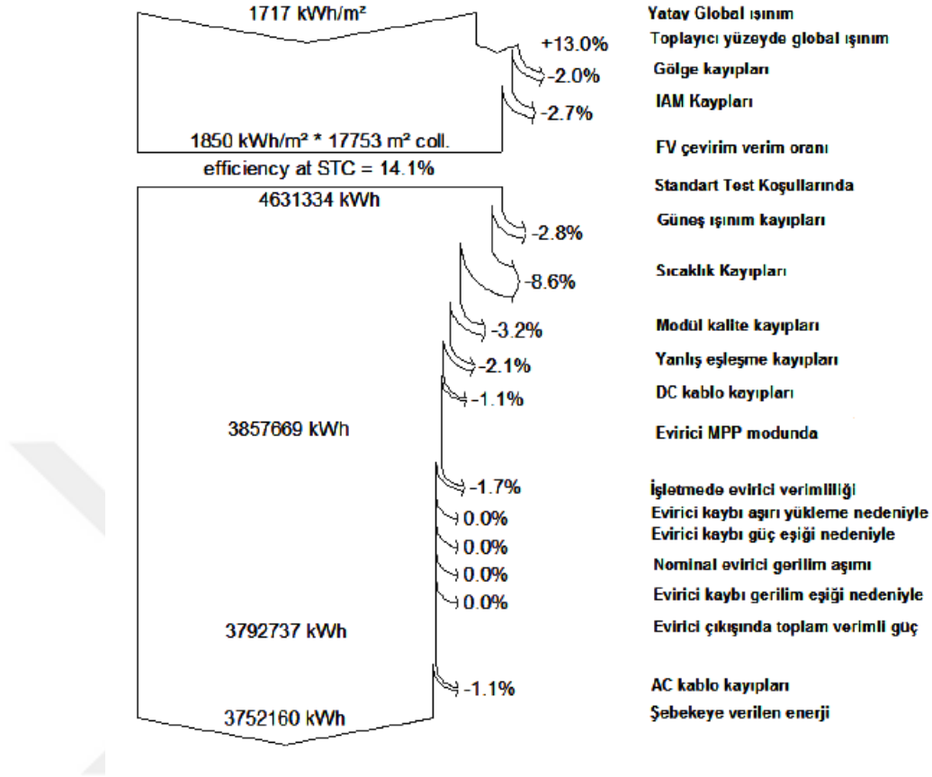
Şekil 4.4. PVsyst programının kayıp diyagramı [7].
