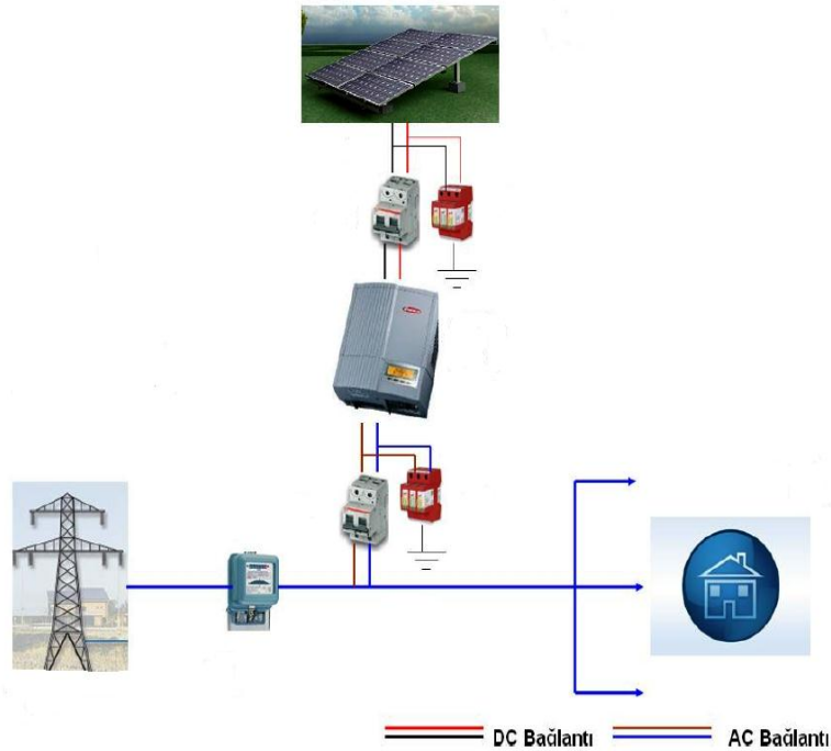
Şekil 3.1. FV sistem şeması [5].
