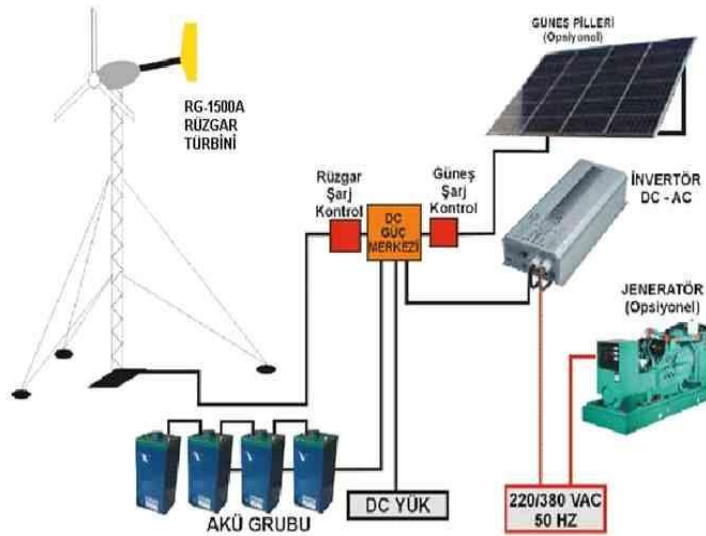
Şekil 3.5.Hibrit fotovoltaik sistem [28].
