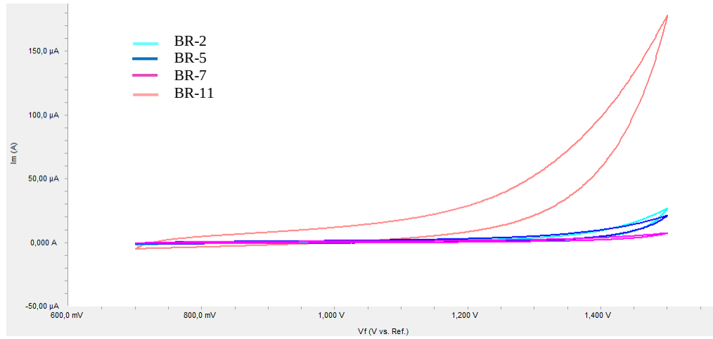
Şekil 4.25. Optimum pH'yı belirlemek amacıyla farklı pH'lardaki BR tamponlarının kıyaslanması
