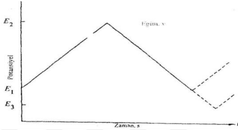
Şekil 1.2. Dönüşümlü voltametri ve doğrusal taramalı tekniklerinde zamanla potansiyel taramanın değişimi
