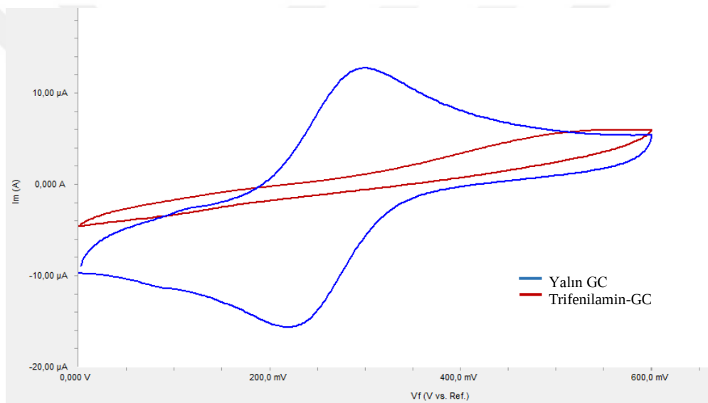
Şekil 4.36. GC'nin ve pH=5 BR ortamında elde edilen trifenilaminin HCF (III) ile yüzey testi
