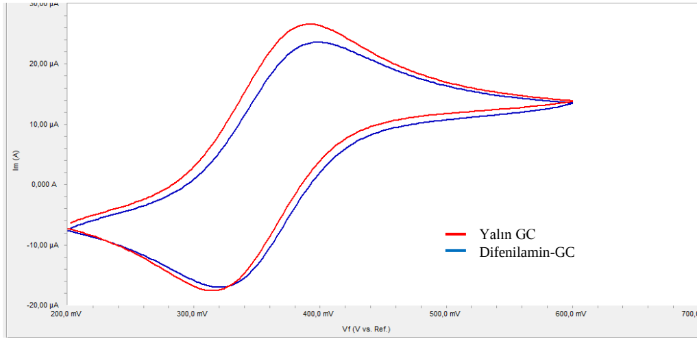
Şekil 4.23. GC'nin ve pH=7 BR ortamında elde edilen difenilaminin Ferrosen ile yüzey testi
