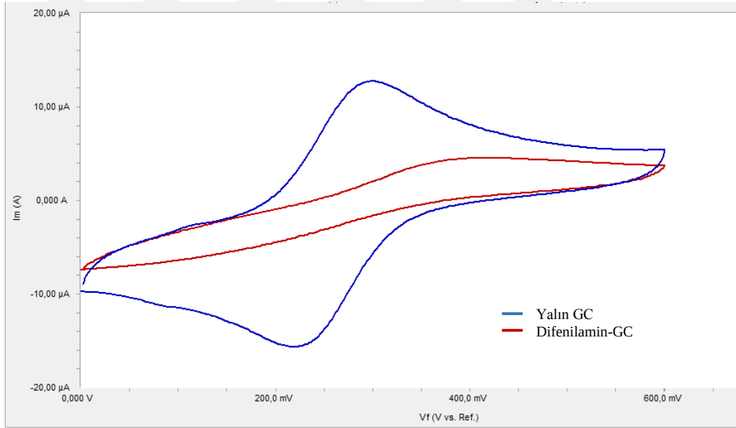
Şekil 4.20. GC'nin ve pH=5 BR ortamında elde edilen difenilaminin HCF (III) ile yüzey testi
