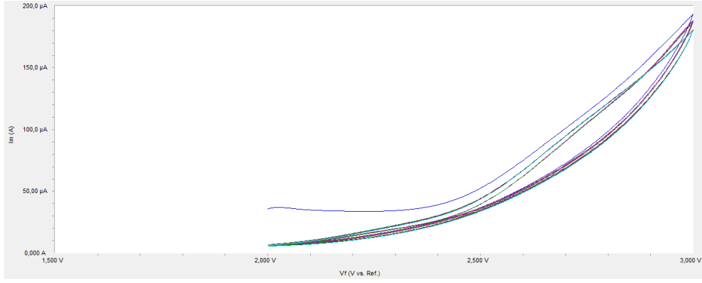
e. 1 mM difenilamin için (2, 3) V potansiyel aralığında alınan voltamogram
