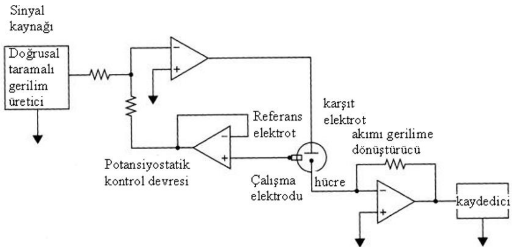
Şekil 1.4. Üçlü elektrot sisteminde doğrusal taramalı voltametri sistemi (Maraba, 2008; Tekin, 2008)
