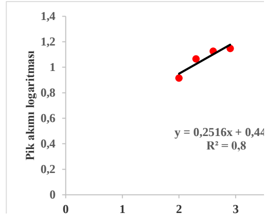
Şekil 4.28. Yalın GC'nin Difenilamin ile modifikasyonunda tarama hızı logaritmasına karşı pik akım logaritması grafiği
