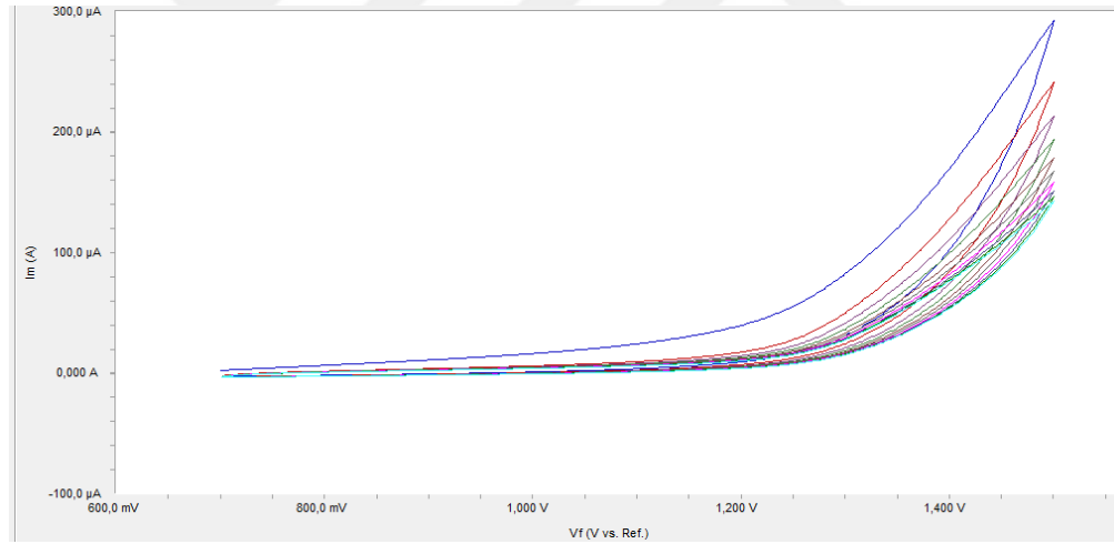
Şekil 4.56. Trifenilfosfinin pH=11 BR ortamında GC elektrot yüzeyindeki 100 mV/s tarama hızında 10 döngülü voltamogramı
