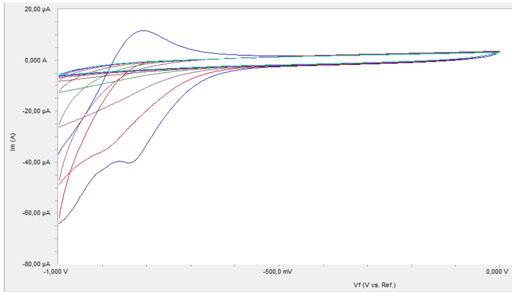
b. 1 mM difenilamin için (-1, 0) V potansiyel aralığında alınan voltamogram
