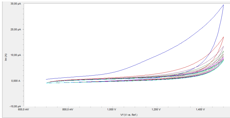
Şekil 4.48. Trifenilfosfinin pH=5 BR ortamında GC elektrot yüzeyindeki 100 mV/s tarama hızında 10 döngülü voltamogramı
