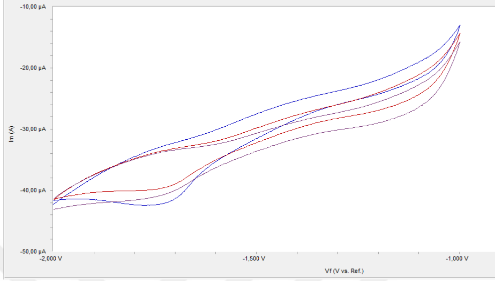
a. 1 mM trifenilamin için (-2, -1) V potansiyel aralığında alınan voltamogram
