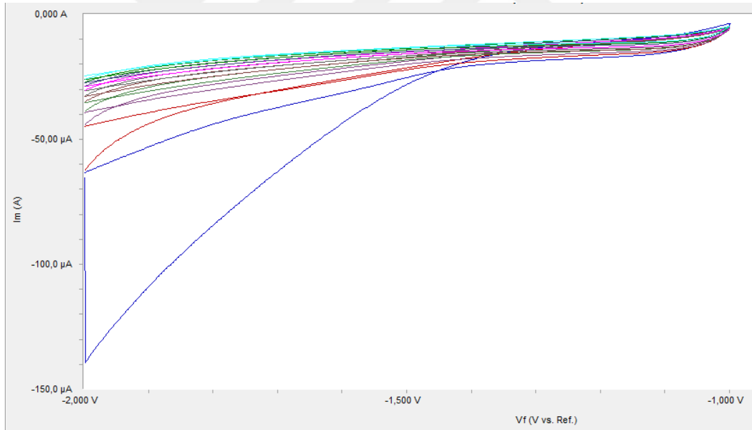
a. 1 mM difenilamin için (-2, -1) V potansiyel aralığında alınan voltamogram
