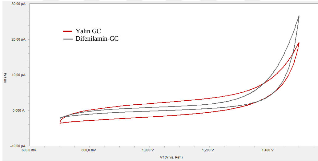
Şekil 4.14. GC’nin ve pH=2 BR ortamında elde edilen difenilaminin yüzey voltamogramı
