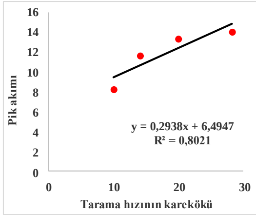
Şekil 4.27. Yalın GC'nin Difenilamin ile modifikasyonunda tarama hızı kareköküne karşı pik akım grafiği
