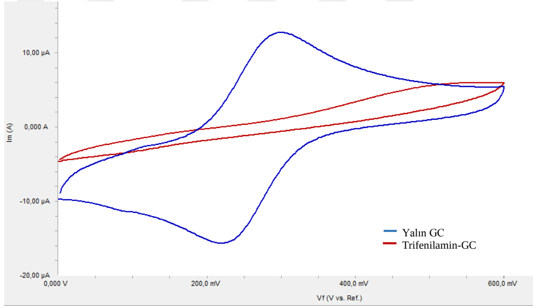
Şekil 4.32. GC'nin ve pH=2 BR ortamında elde edilen trifenilaminin HCF (III) ile yüzey testi
