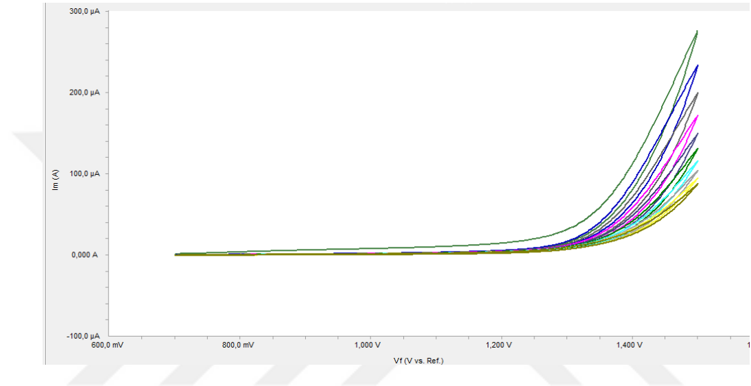
Şekil 4.41. Trifenilaminin pH=11 BR ortamında GC elektrot yüzeyindeki 100 mV/s tarama hızında 10 döngülü voltamogramı
