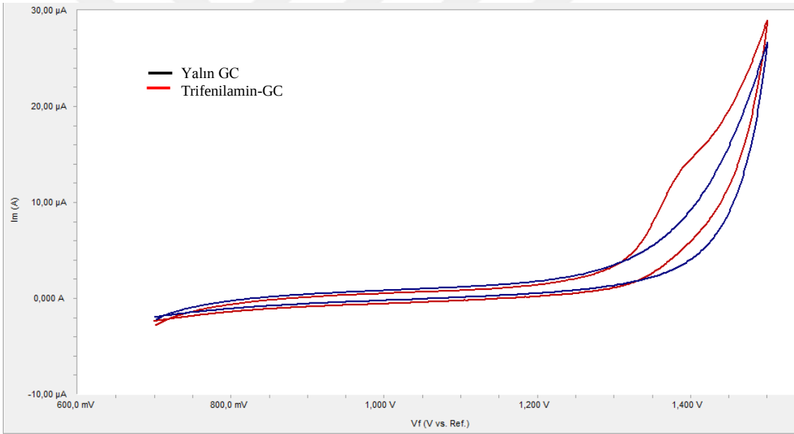
Şekil 4.30. GC'nin ve pH=2 BR ortamında elde edilen trifenilaminin yüzey voltamogramı
