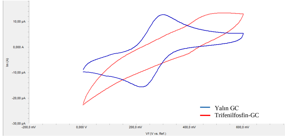
Şekil 4.47. GC'nin ve pH=2 BR ortamında elde edilen trifenilfosfin-GC'nin HCF (III) ile alınan voltamogramları
