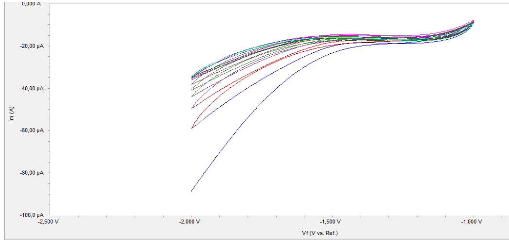
a. 1 mM trifenilfosfin ile (-2, -1) V potansiyel aralığında elde edilen voltamogram
