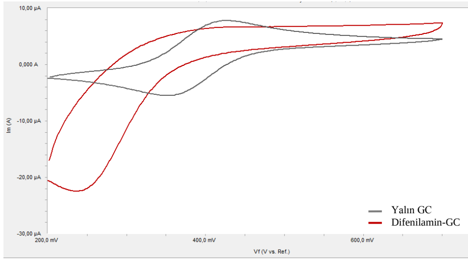
Şekil 4.15. GC'nin ve pH=2 BR ortamında elde edilen difenilaminin Ferrosen ile yüzey testi
