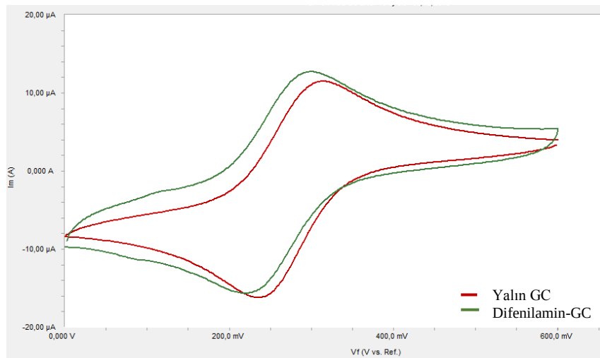
Şekil 4.8. Yalın GC ve Difenilamin-GC elektrodun HCF (III) çözeltisi içinde (0- 0,6) V potansiyel aralığındaki voltamogramları
