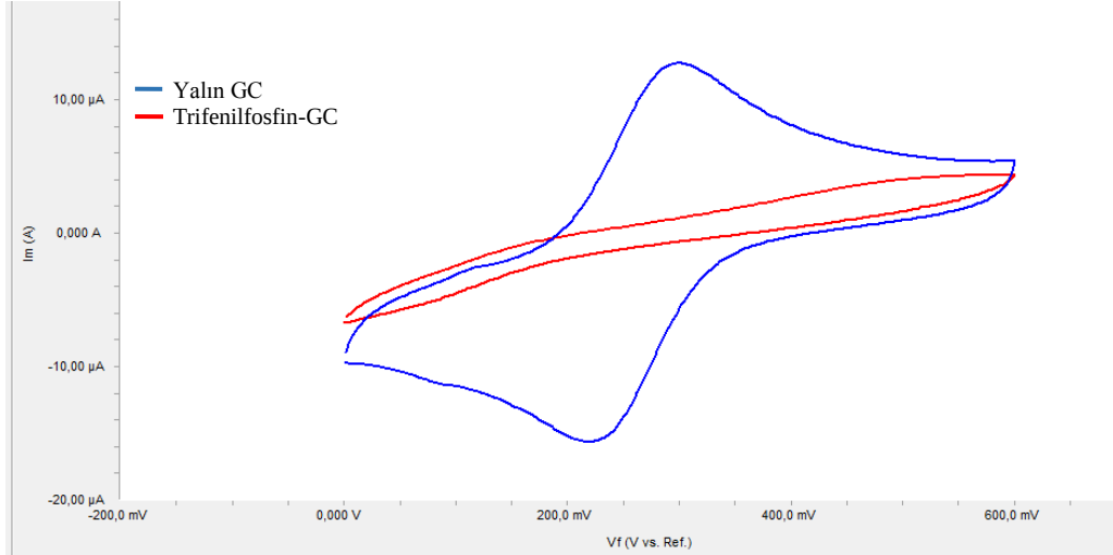
Şekil 4.51. GC'nin ve pH=5 BR ortamında elde edilen trifenilfosfin-GC'nin HCF (III) ile alınan voltamogramları
