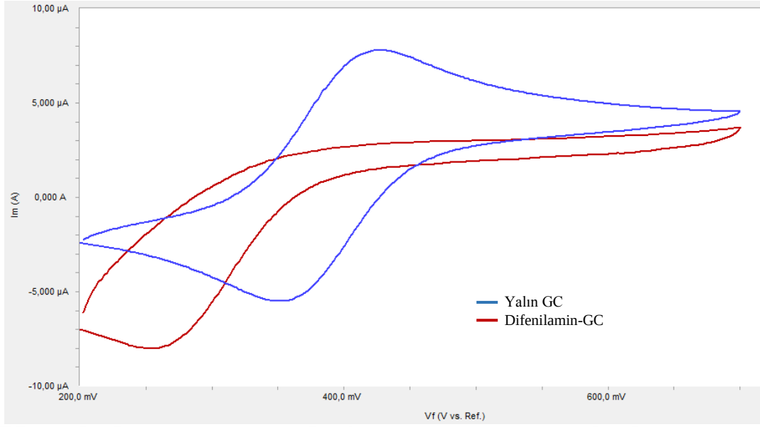
Şekil 4.19. GC'nin ve pH=5 BR ortamında elde edilen difenilaminin Ferrosen ile yüzey testi
