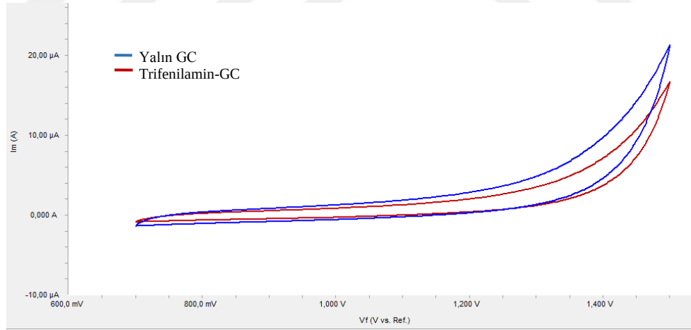
Şekil 4.34. GC'nin ve pH=5 BR ortamında elde edilen trifenilaminin yüzey voltamogramı
