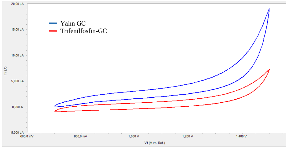
Şekil 4.53. GC'nin ve pH=7 BR ortamında elde edilen trifenilfosfinin yüzey voltamogramı
