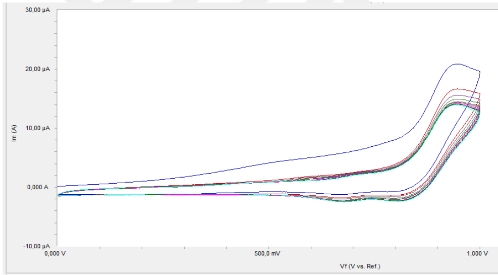
b. 1 mM trifenilamin için (0, 1) V potansiyel aralığında alınan voltamogram
