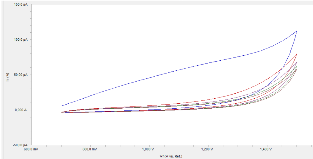
Şekil 4.52. Trifenilfosfinin pH=7 BR ortamında GC elektrot yüzeyindeki 100 mV/s tarama hızında 10 döngülü voltamogramı
