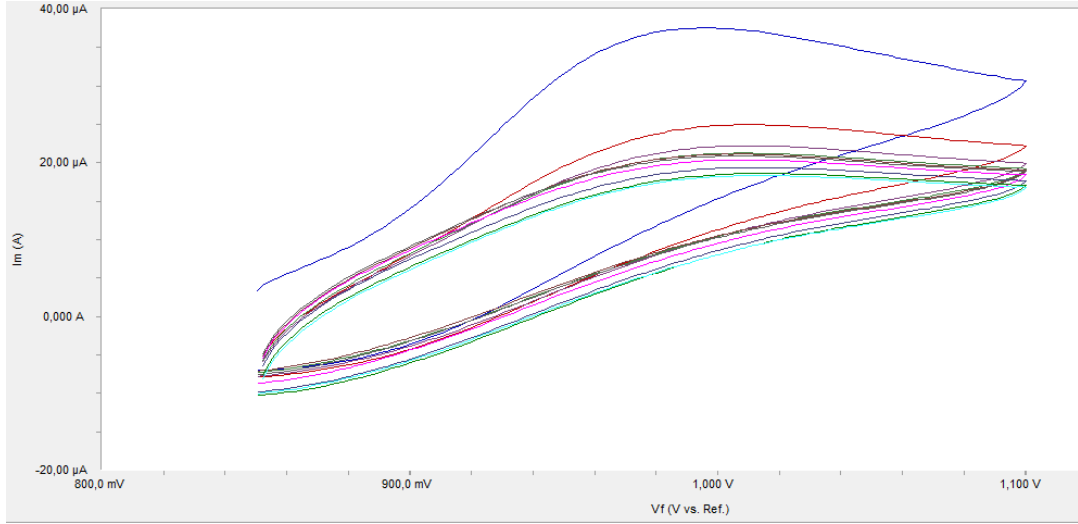
Şekil 4.4. 1 mM triphenilaminin (0.85, 1.1) V potansiyel aralığındaki voltamogramı
