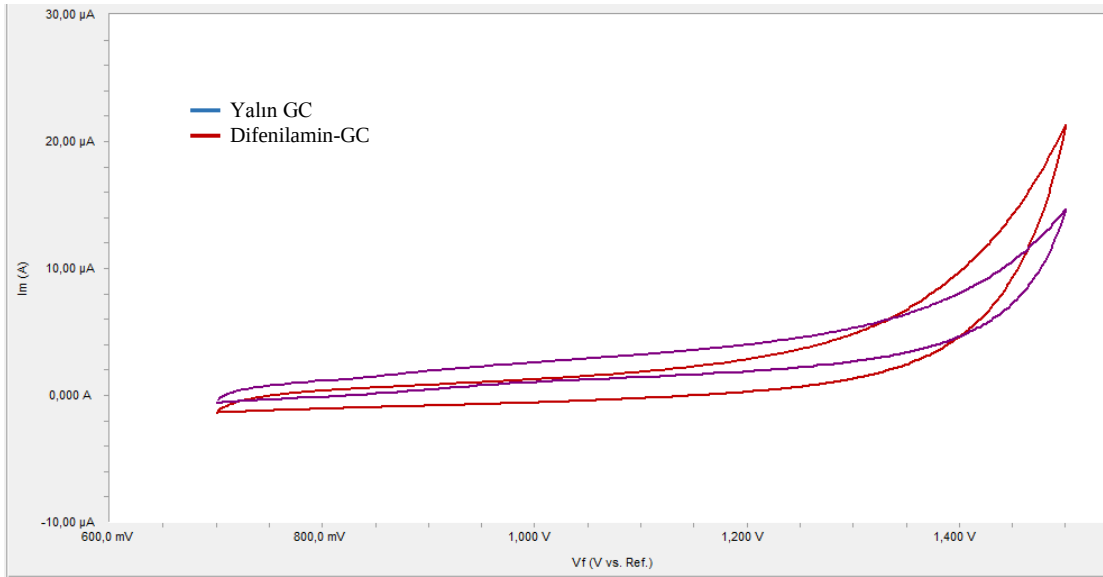
Şekil 4.18. GC’nin ve pH=5 BR ortamında elde edilen difenilaminin yüzey voltamogramı
