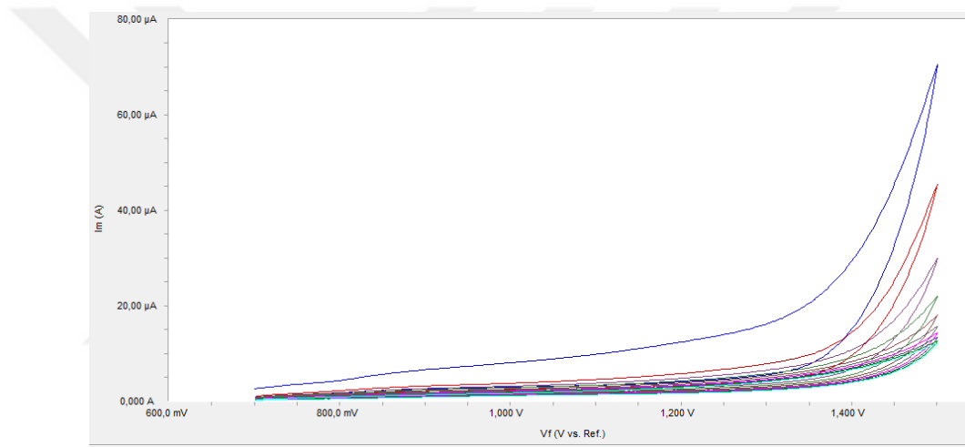
Şekil 4.26. Difenilaminin pH=11 BR ortamında GC elektrot yüzeyindeki 100 mV/s tarama hızında 10 döngülü voltamogramı
