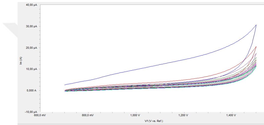
Şekil 4.21. Difenilaminin pH=7 BR ortamında GC elektrot yüzeyindeki 100 mV/s tarama hızında 10 döngülü voltamogramı
