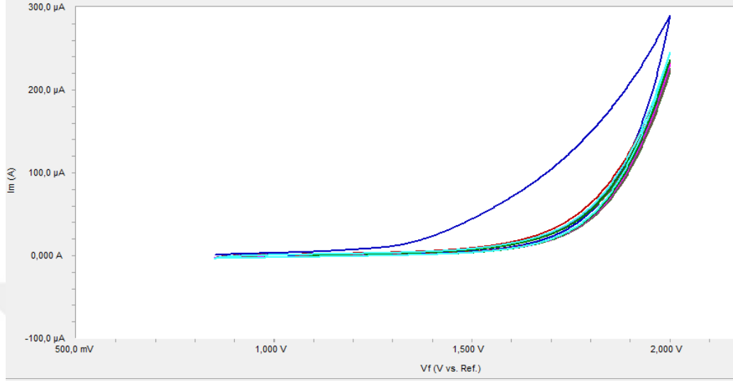
Şekil 4.13. Difenilaminin pH=2 BR ortamında GC elektrot yüzeyindeki 100 mV/s tarama hızında 10 döngülü voltamogramı
