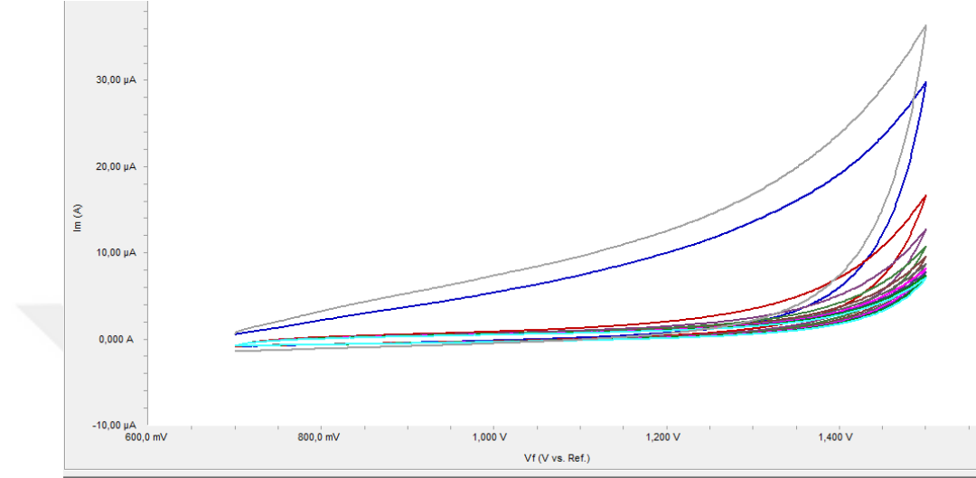
Şekil 4.33. Trifenilaminin pH=5 BR ortamında GC elektrot yüzeyindeki 100 mV/s tarama hızında 10 döngülü voltamogramı
