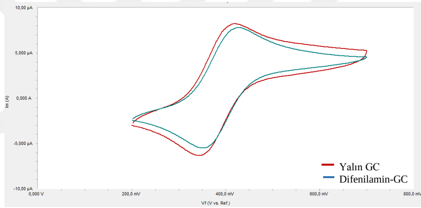
Şekil 4.7. Yalın GC ve Difenilamin-GC elektrodun Ferrosen çözeltisi içindeki dönüşümlü voltamogramı
