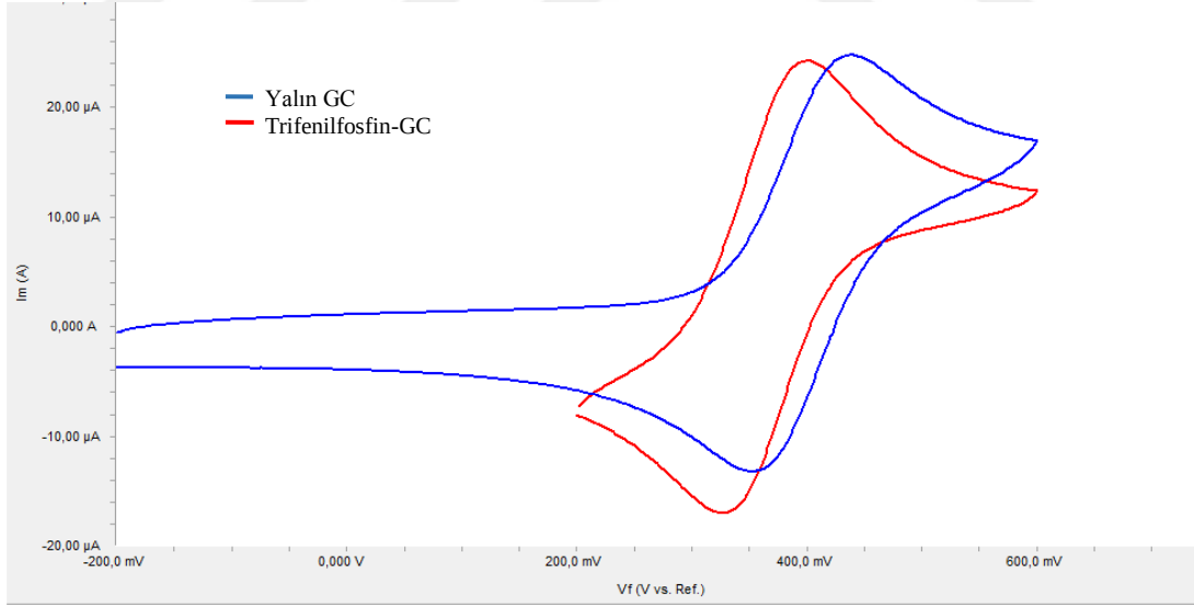
Şekil 4.50. GC'nin ve pH=5 BR ortamında elde edilen trifenilfosfin-GC'nin Ferrosen ile alınan voltamogramları
