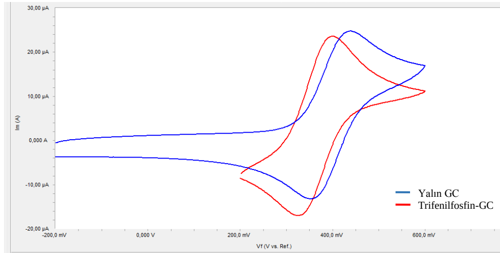
Şekil 4.46. GC'nin ve pH=2 BR ortamında elde edilen trifenilfosfin-GC'nin Ferrosen ile alınan voltamogramları
