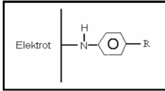
Şekil 1.7. Amin oksidasyonu yöntemi ile elde edilen yüzey
