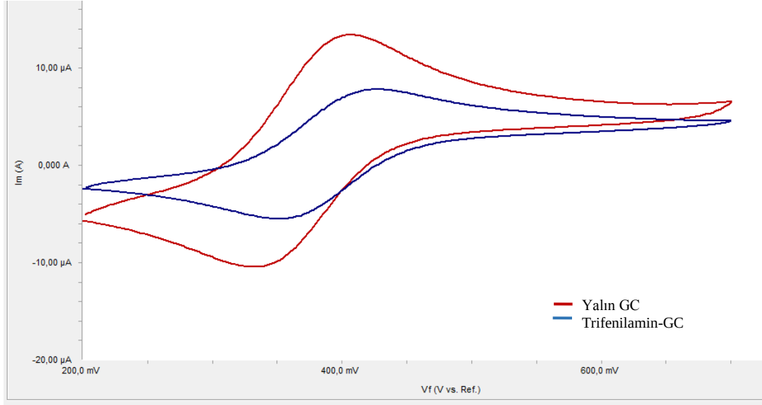
Şekil 4.31. GC'nin ve pH=2 BR ortamında elde edilen trifenilaminin Ferrosen ile yüzey testi
