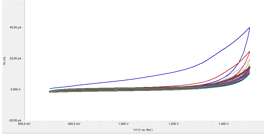
Şekil 4.44. Trifenilfosfinin pH=2 BR ortamında GC elektrot yüzeyindeki 100 mV/s tarama hızında 10 döngülü voltamogramı
