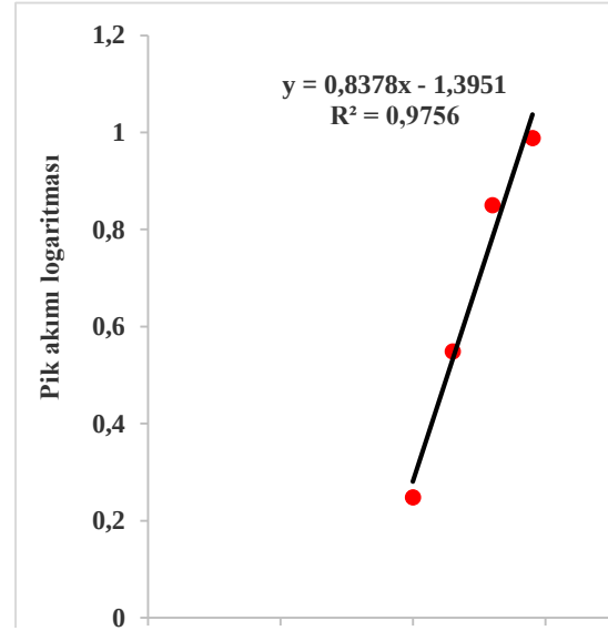
Şekil 4.43. Yalın GC'nin Trifenilamin ile modifikasyonunda tarama hızı logaritmasına karşı pik akım logaritması grafiği
