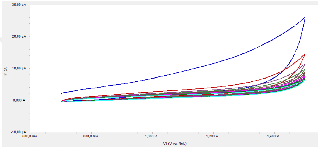
Şekil 4.17. Difenilaminin pH=5 BR ortamında GC elektrot yüzeyindeki 100 mV/s tarama hızında 10 döngülü voltamogramı
