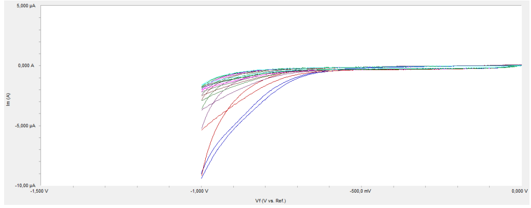
b. 1 mM trifenilfosfin ile (-1, 0) V potansiyel aralığında elde edilen voltamogram
