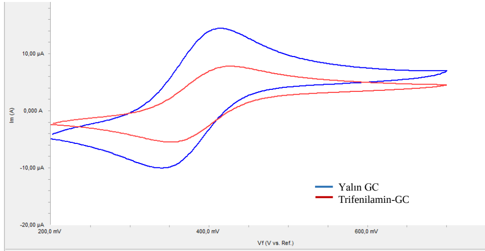
Şekil 4.35. GC'nin ve pH=5 BR ortamında elde edilen trifenilaminin Ferrosen ile yüzey testi
