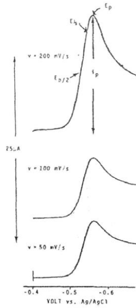
Şekil 1.3. Doğrusal taramalı voltametri de akım–potansiyel eğrileri ve akımın tarama hızıyla değişimi
