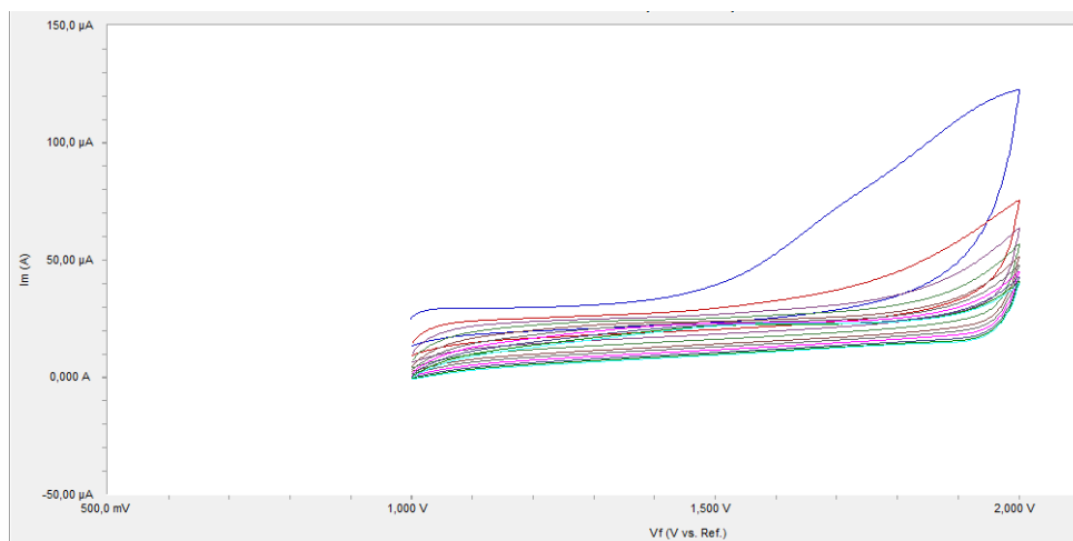
d. 1 mM difenilamin için (1, 2) V potansiyel aralığında alınan voltamogram
