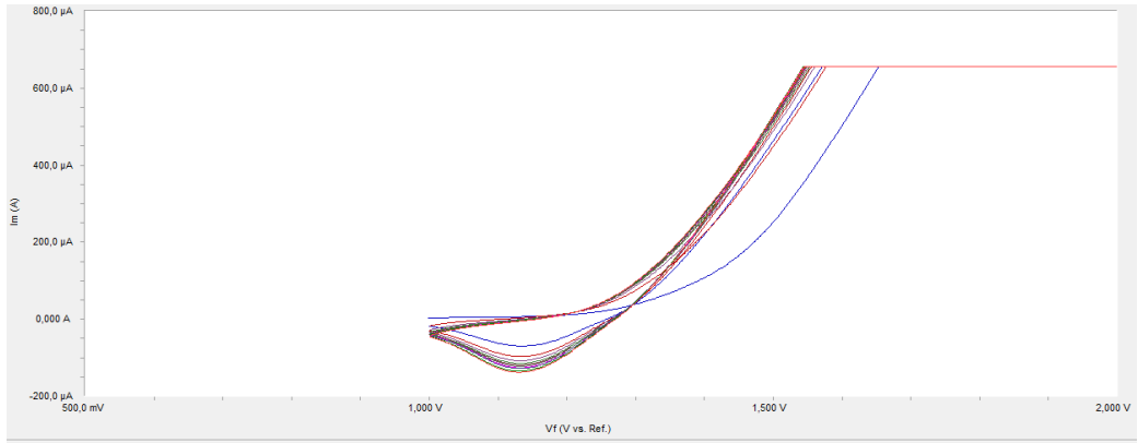
d. 1 mM trifenilfosfin ile (1, 2) V potansiyel aralığında elde edilen voltamogram
