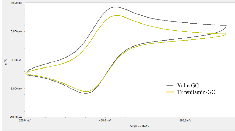
Şekil 4.9. Yalın GC ve Trifenilamin-GC elektrodun Ferrosen çözeltisindeki voltamogramları
