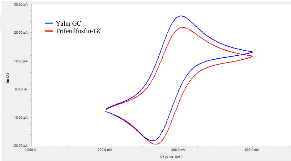
Şekil 4.54. GC'nin ve pH=7 BR ortamında elde edilen trifenilfosfin-GC'nin Ferrosen ile alınan voltamogramları
