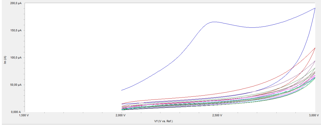
e. 1 mM trifenilfosfin ile (2, 3) V potansiyel aralığında elde edilen voltamogram
