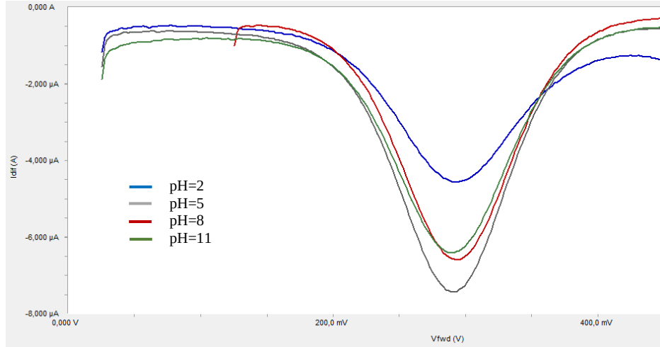
Şekil 4.59. Yalın GC'de farklı pH'larda tutulan 1.10^{-2} M \text{Cu}^{2+} 'nin DPV ile sıyırılma voltagramları
