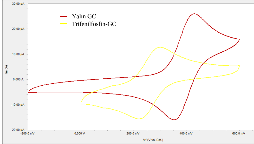
Şekil 4.12. Yalın GC ve Trifenilfosfin-GC elektrodun HCF (III) çözeltisi içindeki voltamogramları
