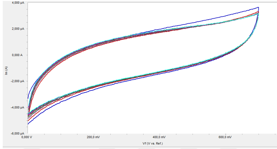
Şekil 4.37. Trifenilaminin pH=7 BR ortamında GC elektrot yüzeyindeki 100 mV/s tarama hızında 10 döngülü voltamogramı
