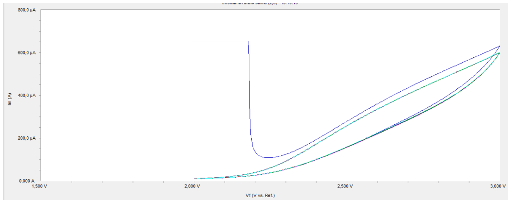
e. 1 mM trifenilamin için (2, 3) V potansiyel aralıklarında alınan voltamogram
