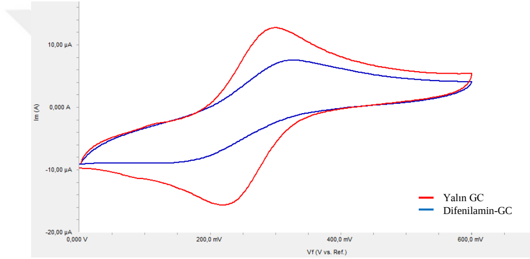
Şekil 4.24. GC'nin ve pH=7 BR ortamında elde edilen difenilaminin HCF (III) ile yüzey testi
