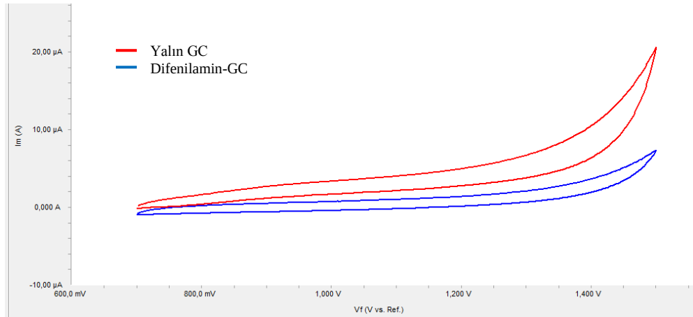
Şekil 4.22. Difenilamin ile kaplanan GC ve yalın GC ile pH=7 BR ortamında alınan voltamogramların kıyaslanması
