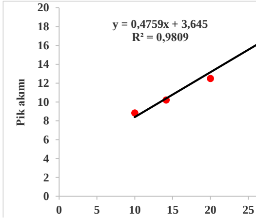
Şekil 4.57. Yalın GC'nin Trifenilfosfin ile modifikasyonunda tarama hızı kareköküne karşı pik akım grafiği
