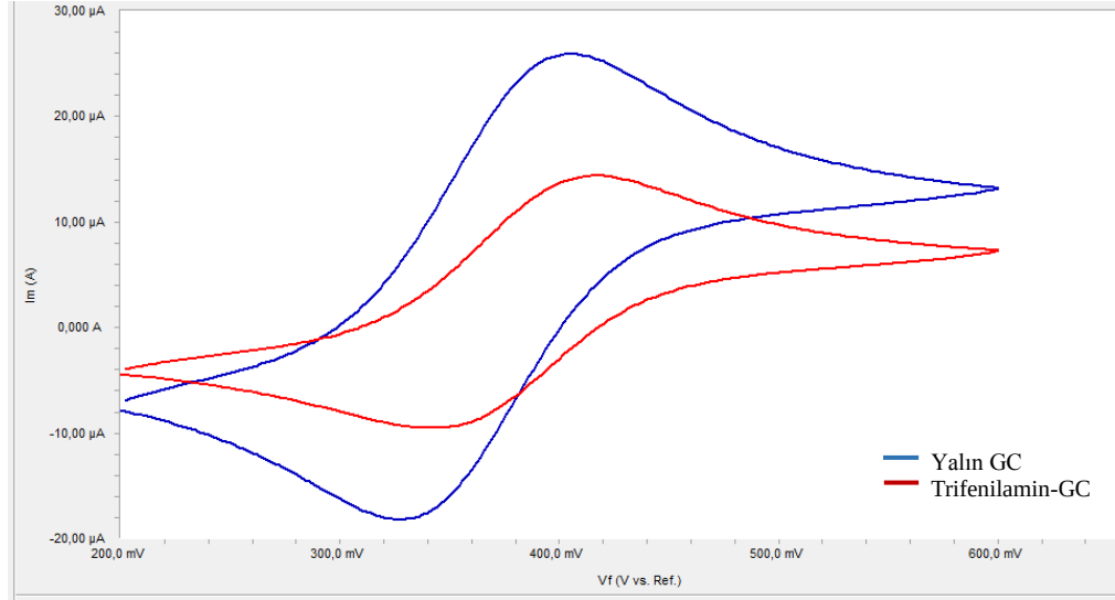
Şekil 4.39. GC'nin ve pH=7 BR ortamında elde edilen trifenilaminin Ferrosen ile yüzey testi
