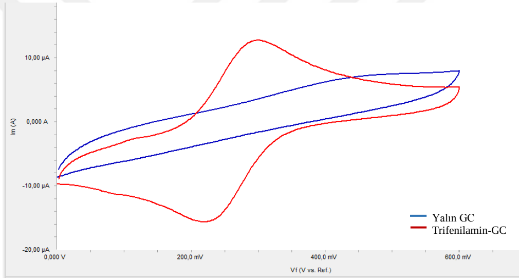
Şekil 4.40. GC'nin ve pH=7 BR ortamında elde edilen trifenilaminin HCF (III) ile yüzey testi
