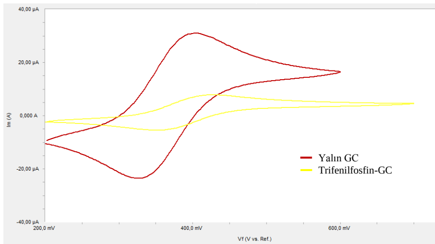
Şekil 4.11. Yalın GC ve Trifenilfosfin-GC elektrodun Ferrosen çözeltisindeki voltamogramları
