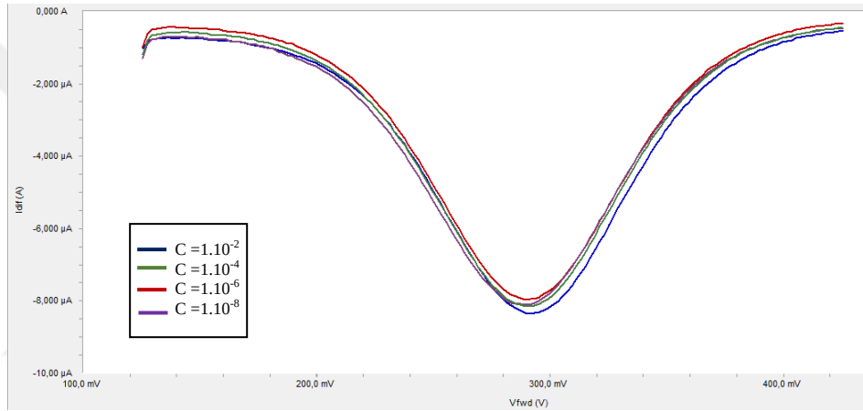
Şekil 4.60. Yalın GC'de pH=5 olan farklı derişimlerde tutulan \text{Cu}^{2+} 'nin DPV ile sıyırılma voltagramları
