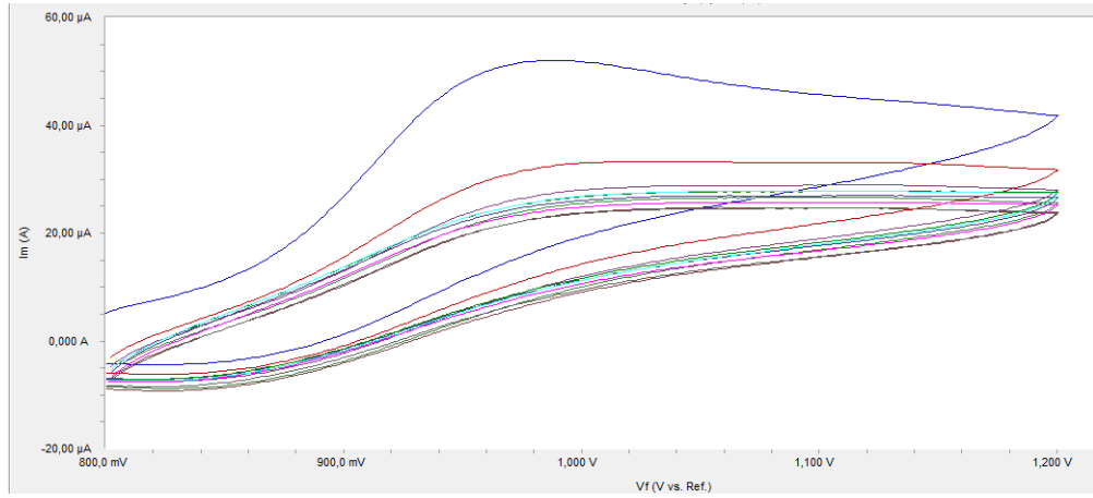
c. 1 mM trifenilamin için (0.8, 1.2) V potansiyel aralığında alınan voltamogram
