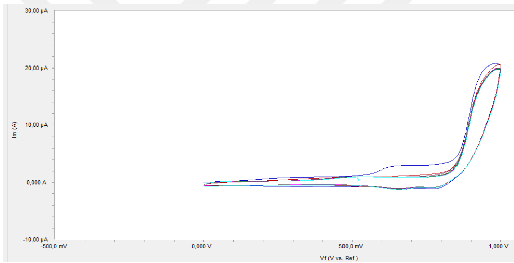
c. 1 mM difenilamin için (0, 1) V potansiyel aralığında alınan voltamogram
