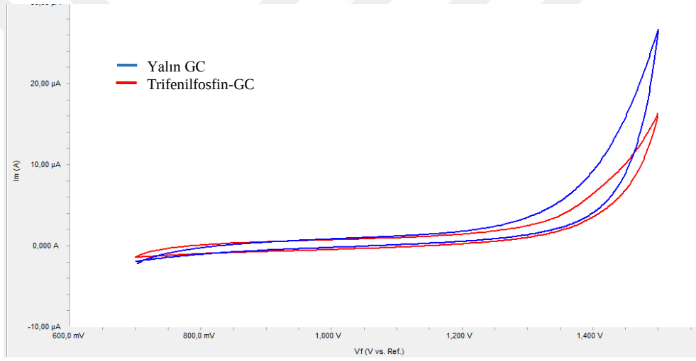
Şekil 4.45. GC'nin ve pH=2 BR ortamında elde edilen trifenilfosfinin yüzey voltamogramı
