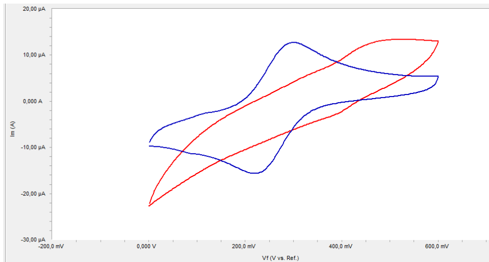
Şekil 4.55. GC'nin ve pH=7 BR ortamında elde edilen trifenilfosfin-GC'nin HCF (III) ile alınan voltamogramları
