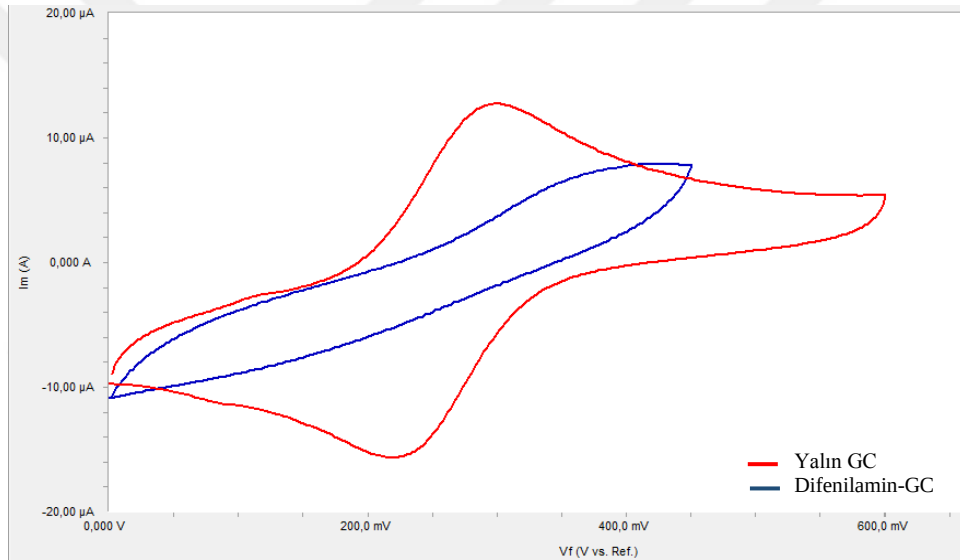
Şekil 4.16. GC'nin ve pH=2 BR ortamında elde edilen difenilaminin HCF (III) ile yüzey testi
