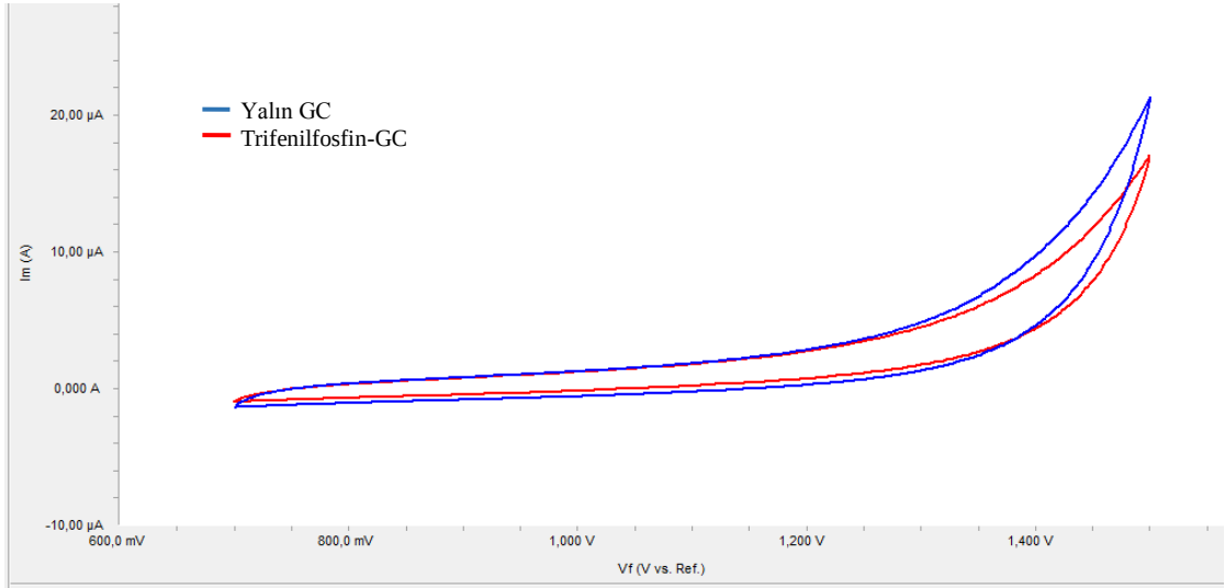
Şekil 4.49. GC'nin ve pH=5 BR ortamında elde edilen trifenilfosfinin yüzey voltamogramı
