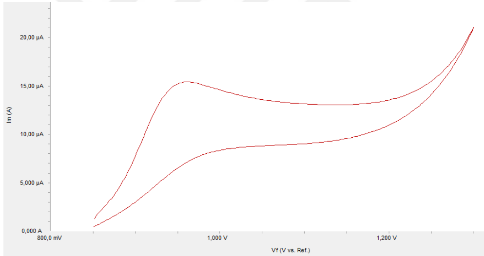
Şekil 4.2. (0.85, 1.3) V potansiyel aralığında alınan 1 mM difenilaminin voltamogramı
