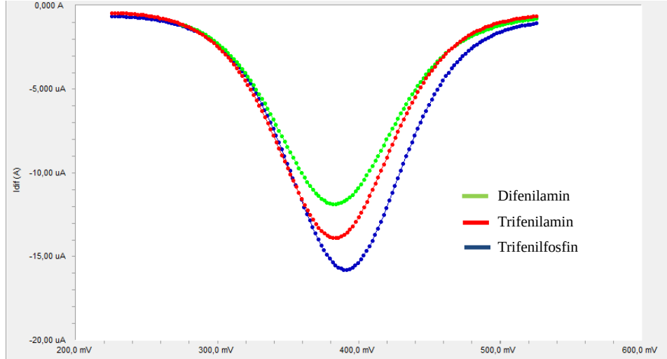
Şekil 4.61. 1.10^{-2} M derişimde ve pH=5 ortamında aminli bileşiklerin metal tutma kapasitelerinin karşılaştırılması
