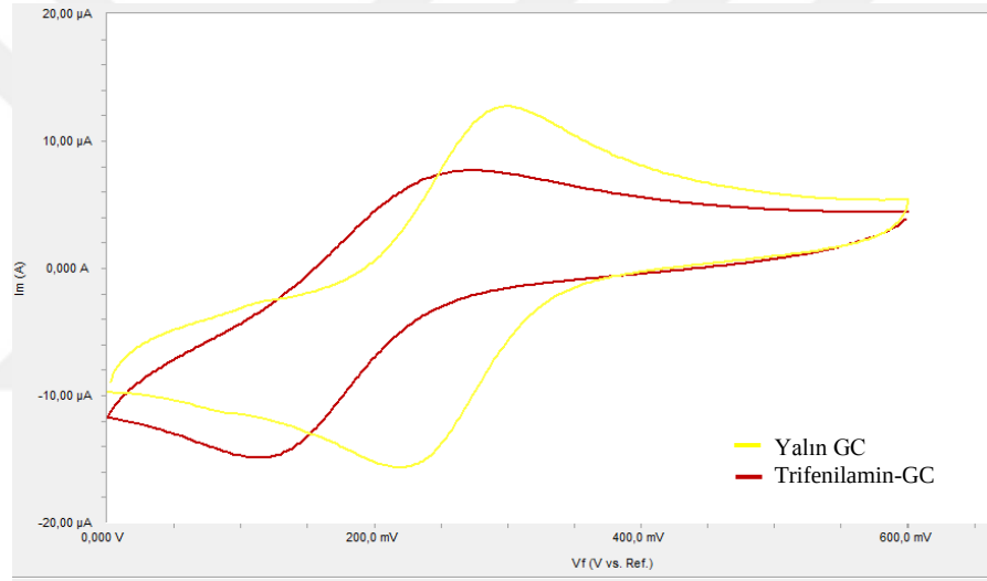
Şekil 4.10. Yalın GC ve Trifenilamin-GC elektrodun HCF (III) çözeltisindeki voltamogramları
