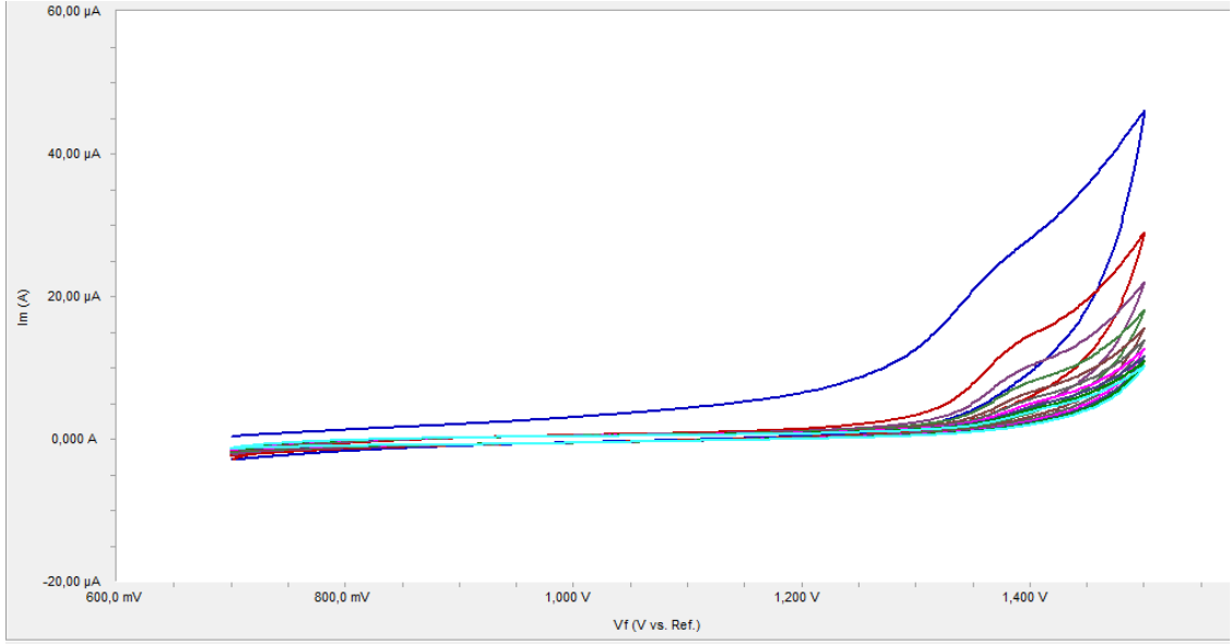
Şekil 4.29. Trifenilaminin pH=2 BR ortamında GC elektrot yüzeyindeki 100 mV/s tarama hızında 10 döngülü voltamogramı
