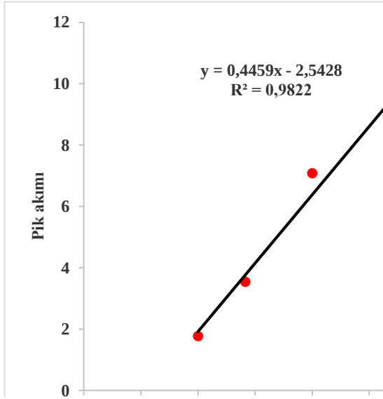
Şekil 4.42. Yalın GC'nin Trifenilamin ile modifikasyonunda tarama hızı kareköküne karşı pik akım grafiği
