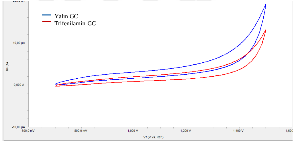
Şekil 4.38. GC’nin ve pH=7 BR ortamında elde edilen trifenilaminin yüzey voltamogramı
