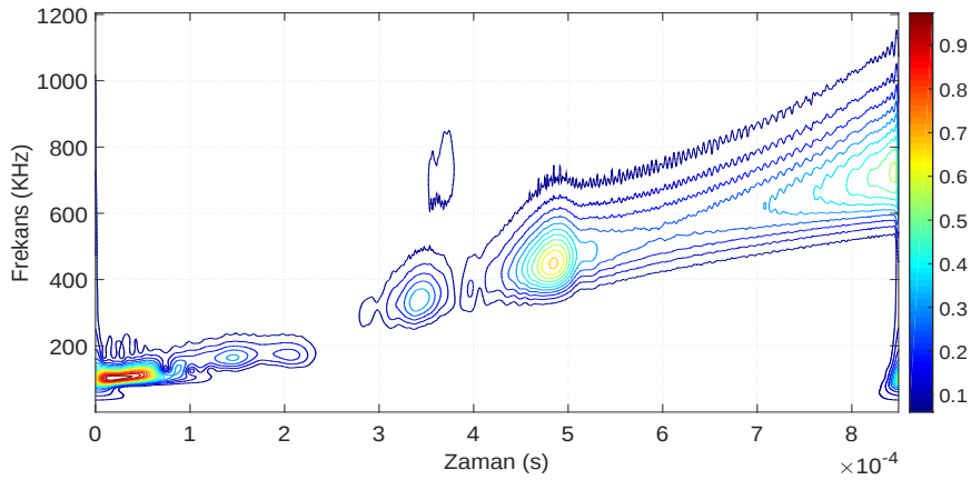
Şekil 4.9. Sinüs dalga, Genlik: 0.2V-Ofset: 0
