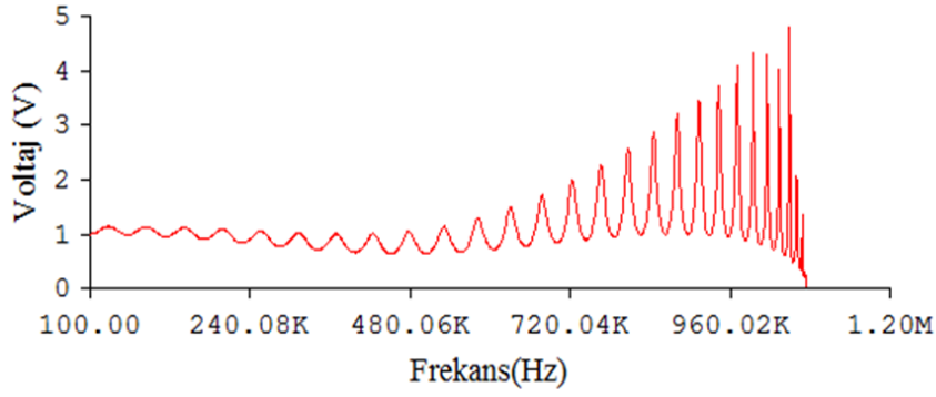
Şekil 2.22. Kiplerin frekans dağılımı
