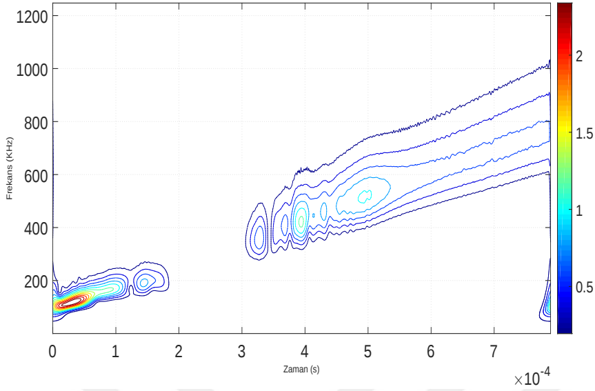
Şekil 4.23. Sinüs dalga, Genlik: 0.5V-Ofset: 1
