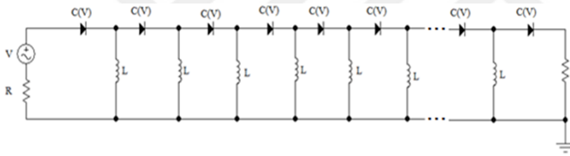
Şekil 2.23. Nonlinear sol elli iletim hattı
