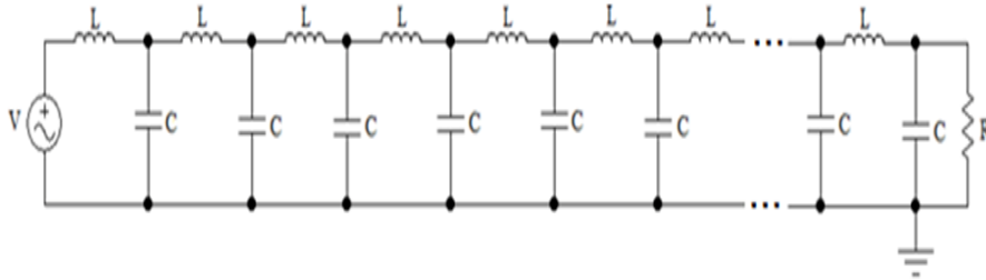
Şekil 2.1. Sağ elli lineer LC iletim hattı
