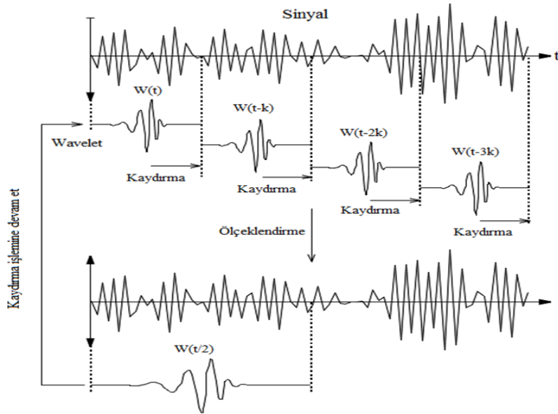
Şekil 3.6. Wavelet dönüşüm işlemleri
