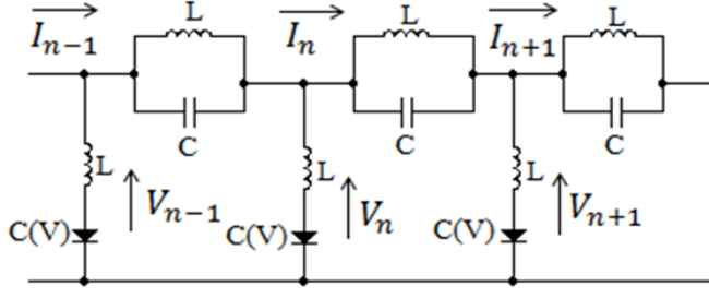
Şekil 2.28. Nonlinear birleşik iletim hattı kesiti
