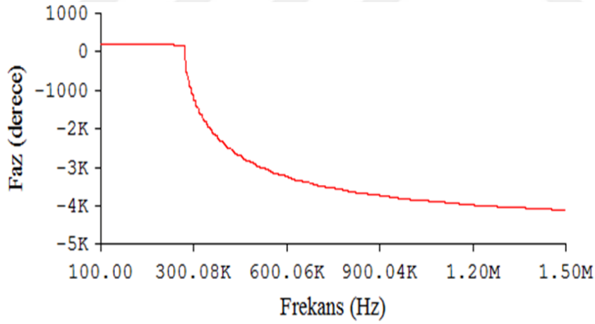
Şekil 2.10. \omega(k) dağıtım grafiği
