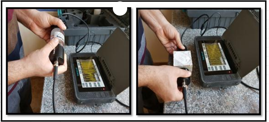
Şekil 3.12 Sertleşmiş betonda ultrases hız ölçümü
