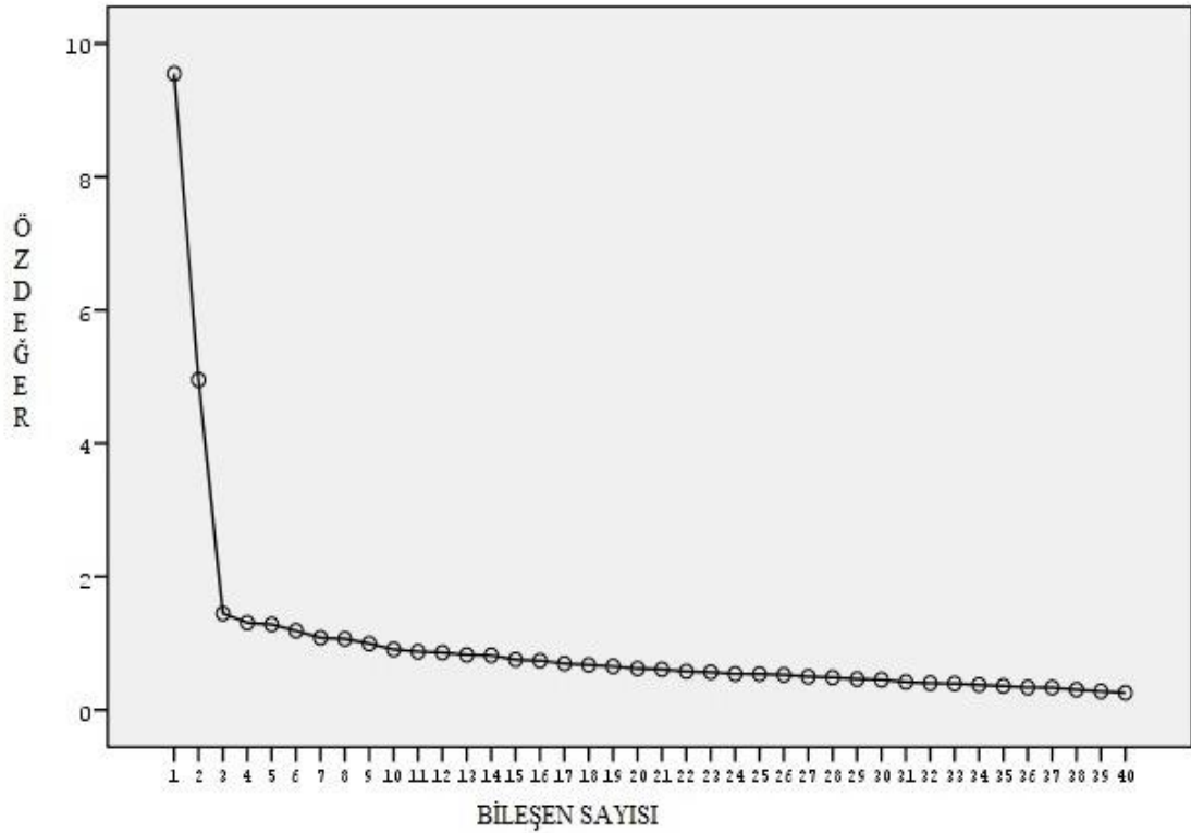
Şekil 1. Varimaks Döndürme Sonrası Yamaç Birikinti Grafiği
