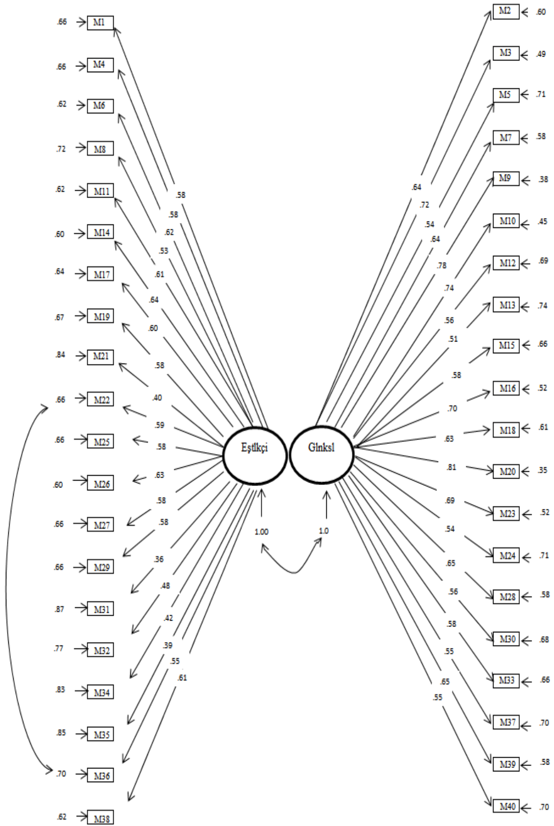
Şekil 2. Modifikasyonlar sonrası ERBÖ Modeli Standart Değerleri
