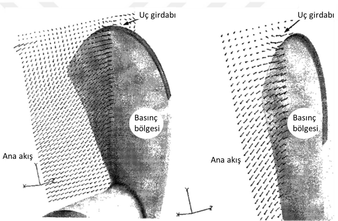
Şekil 2. 15 Basınç bölgesindeki hız dağılımı [11]
