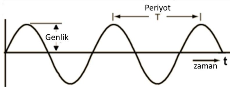
Şekil 3. 1 Basit harmonik bir dalgaının ses basıncının zamanla değişimi
