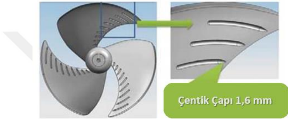
Şekil 2. 9 Yiv açılmış fan kanatları [6]
